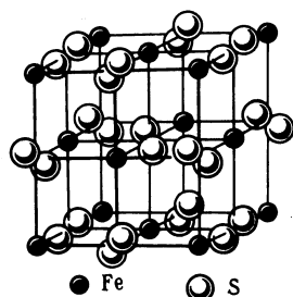
Р и с. 155. Кристаллическая решетка пирита \text{FeS}_2
