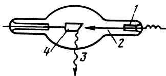
Р и с. 86. Схема рентгеновской трубки
