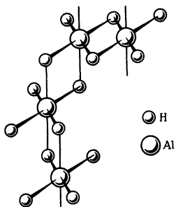
Р и с. 196. Фрагмент структуры гидроида алюминия (\text{AlH}_3)_n
