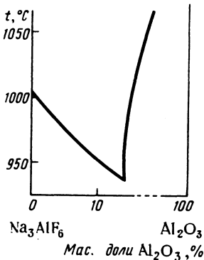
Рис. 190. Фрагмент диаграммы плавкости системы \text{Na}_3\text{AlF}_6 - \text{Al}_2\text{O}_3
