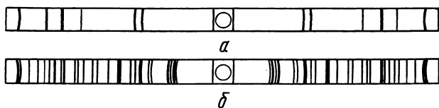
Р и с. 101. Рентгенограммы: a – алмаз; b – графит
