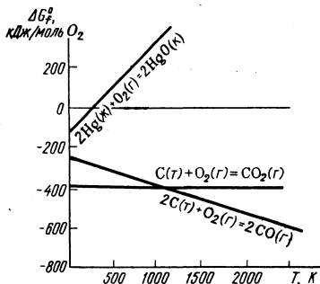
Р и с. 113. Зависимость \Delta G_f^\circ ряда оксидов от температуры
