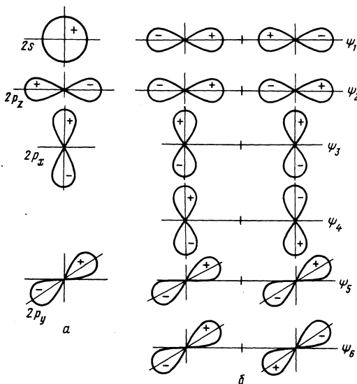
Р и с. 38. Орбитали центрального атома (а) и групповые орбитали (б) для трехцентровой линейной молекулы \text{CO}_2
