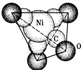
Рис. 242. Строение молекулы тетракарбонила никеля Ni(CO) 4
