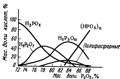
Р и с. 168. Состав фосфорных кислот в зависимости от содержания в растворе P 2 O 5
