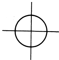
Р и с. 3. Сечение границной поверхности
