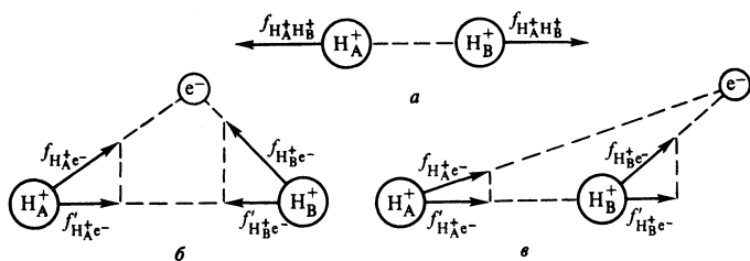
Р и с. 18. Силы взаимодействия между протонами и электроном в молекулярном ионе H_2^+
