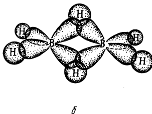
Р и с. 185. Строение (а) и схема перекрывания атомных орбиталей (б) в молекуле \text{B}_2\text{H}_6
