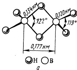
Р и с. 185. Строение (а) и схема перекрывания атомных орбиталей (б) в молекуле \text{B}_2\text{H}_6
