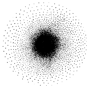
Р и с. 2. Электронное облако
