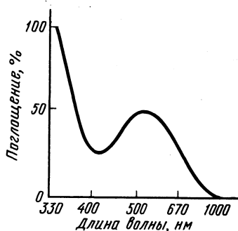
Р и с. 223. Спектр поглощения комплекса [\text{Ti}(\text{OH}_2)_6]^{3+}
