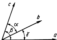
Р и с. 63. Система кристаллографических координат
