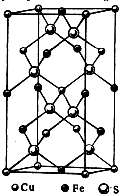
Рис. 135. Кристаллическая решетка халькопирита \text{CuFeS}_2
