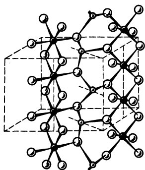
Р и с. 181. Структура сурика Pb_3O_4 ( Pb_2PbO_4 )
