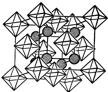
Р и с. 68. Кристаллическая решетка соединений типа: M_2[ЭНal_6] или [M^+(NH_3)_6]X_2 : октаэдры — ионы SiF 6 2- , TiCl 6 2- , Ni(NH 3 ) 6 2+ ; кружки — ионы NH 4 + , K + , Cl - , Br - и др.
