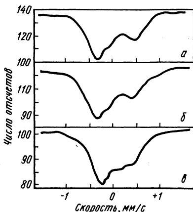
Р и с. 241. \gamma -Спектры берлинской лазури (а) и турбуллевой сини (б) и солей \text{KFe}^{+3}\text{Fe}^{+2}(\text{CN})_6 и \text{KFe}^{+2}\text{Fe}^{+3}(\text{CN})_6 (в)
