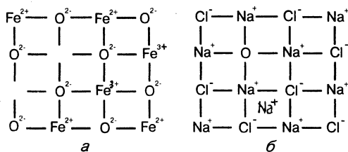
Р и с. 138. Катионный дефект в кристалле FeO ( a ) и анионный дефект в кристалле NaCl, легированном натрием ( б )
