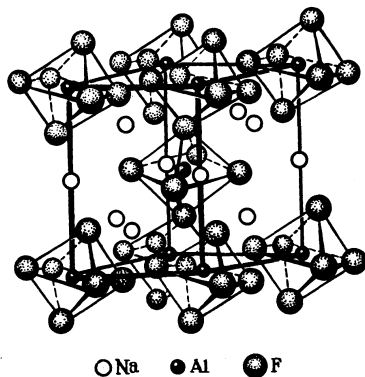
Р и с. 195. Структура криолита \text{Na}_3\text{AlF}_6
