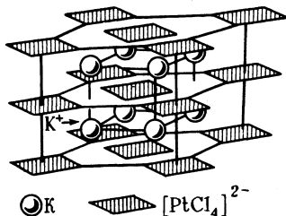
Р и с. 247. Структура \text{K}_2[\text{PtCl}_4]
