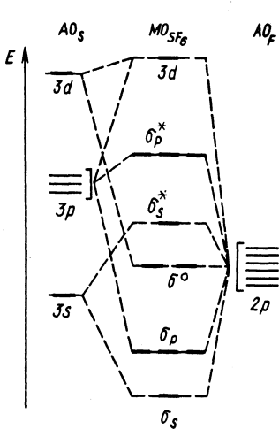
Р и с. 144. Энергетическая диаграмма орбиталей октаэдрической молекулы SF 6
