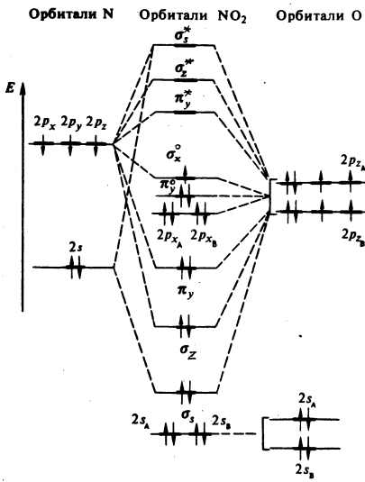
Р и с. 163. Энергетическая диаграмма орбиталей молекулы NO 2 и делокализованной \pi -связи ( \pi_y -орбиталь).
