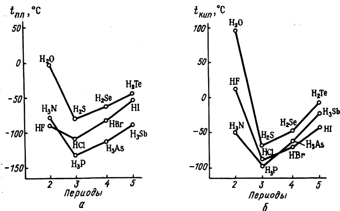
Р и с. 148. Температуры плавления (а) и кипения (б) водородных соединений р-элементов VII, VI, V групп
