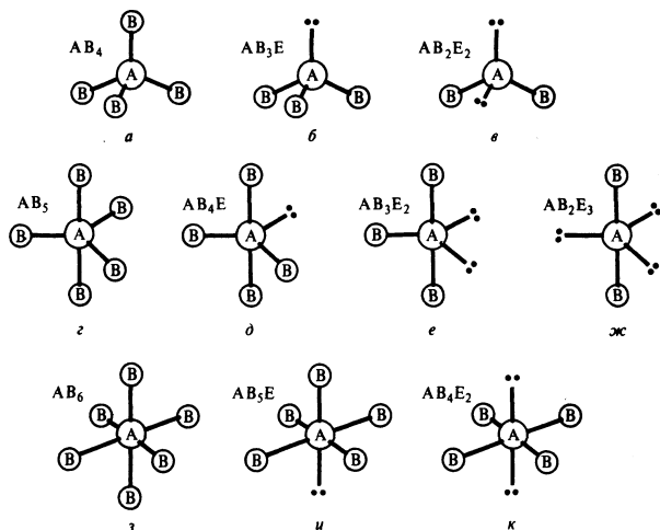
Р и с. 51. Влияние связывающих и несвязывающих электронных пар (E) центрального атома на пространственную конфигурацию молекул:
