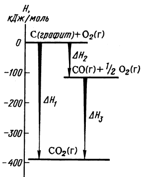
Рис. 109. Энтальпийная диаграмма окисления графита
