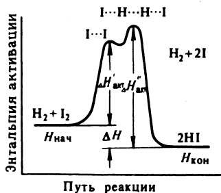
Р и с. 118. Энергетическая схема хода реакции H_2(r) + I_2(r)
