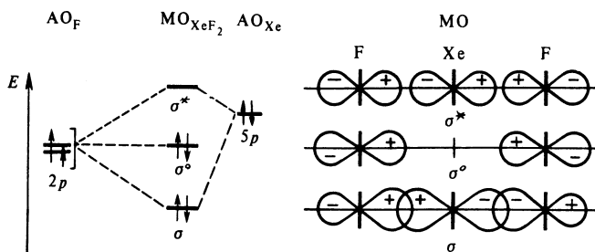
Р и с. 208. Трехцентровые орбитали молекулы \text{XeF}_2
