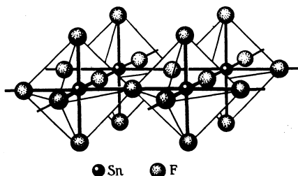
Рис. 182. Структура \text{SnF}_4
