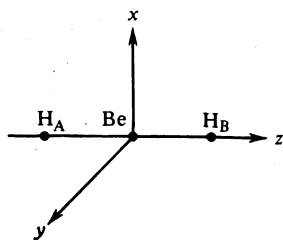
Р и с. 32. Взаимное расположение атомов в молекуле \text{BeH}_2
