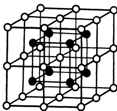
CsCl
