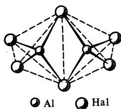
Р и с. 194. Строение молекулы \text{Al}_2\text{Hal}_6
