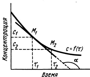
Рис. 114. Изменение концентрации исходных веществ в процессе реакции
