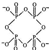
(PO_3)_4^{4-} тетраметафосфат-ион
