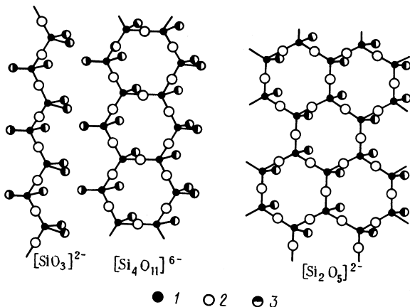
Р и с. 179. Полимерные оксосиликатные ионы:
