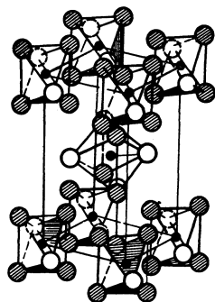
Р и с. 249. Строение кристалла [\text{Pt}(\text{NH}_3)_2\text{Cl}_4]
