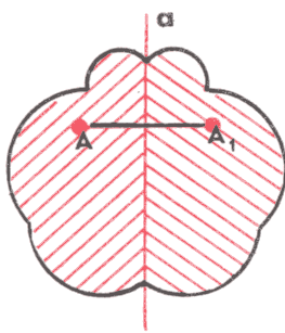
Рис. 36. Прямая a — ось симметрии фигуры
