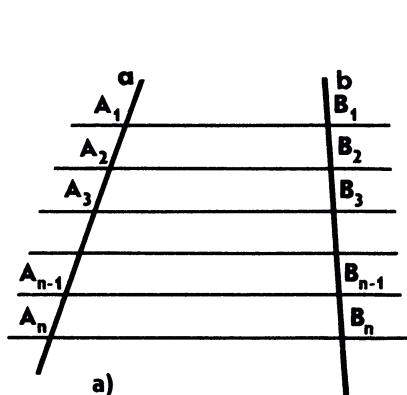
а) Теорема Фалеса:
