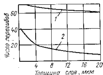
Рис. 3. Окрупчивание пружинистой стали при покрытии в различных электролитах;
