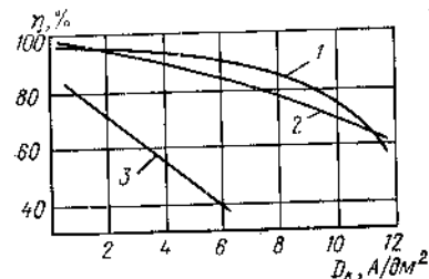
Рис. 6. Зависимость выхода по току от плотности тока в электролитах лужения:
