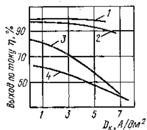
Рис. 2. Зависимость выхода по току от плотности тока в электролитах цинкования: 1 — борфтористоводородном; 2 — аммиачном; 3 — цианистом; 4 — пирофосфатном
