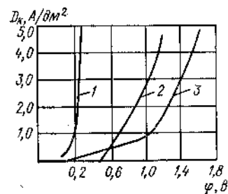
Рис. 4. Катодная поляризация в электролитах кадмирования:
