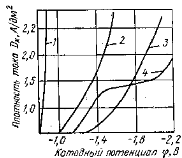
Рис. 1. Катодная поляризация в электролитах цинкования: 1 — сульфатном; 2 — аммиачном; 3 — цианистом; 4 — цинкатном
