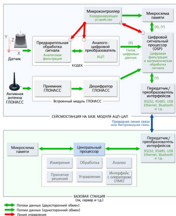
Рис. 5. Схема потоков данных. Источник информации – сейсмоматчик. Антенна ГЛОНАСС в составе спутниковой системы необходима для синхронизации данных между разными сейсмостанциями.
