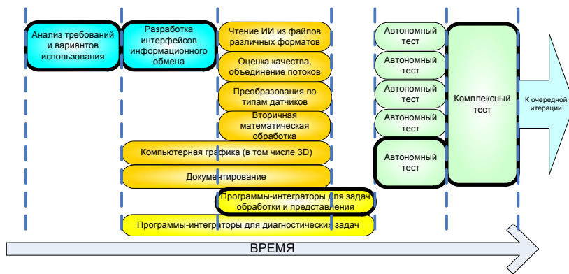
Рис. 6. Итерация разработки ПО системы графического анализа
