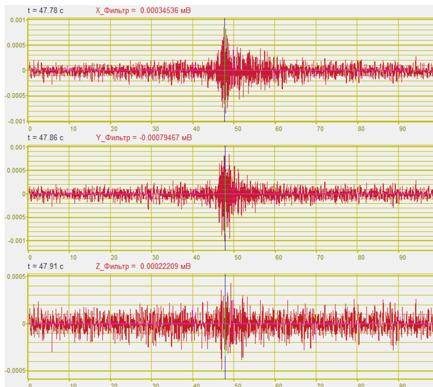
Рис. 10. Сейсмограммы. Компоненты одного из сейсмоматчиков: X-верхний, Y-средний, Z-нижний графики. Показания после полосовой фильтрации. Данные представлены в относительном времени.
