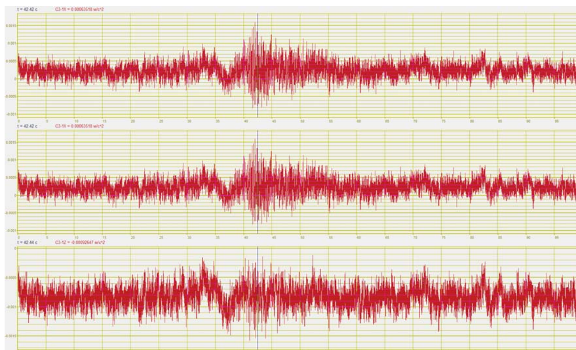
Рис. 6. Сейсмограммы. Компоненты одного из сейсмоматчиков: X-верхний, Y-средний, Z-нижний графики. Показания до полосовой фильтрации. Данные представлены в относительном времени.
