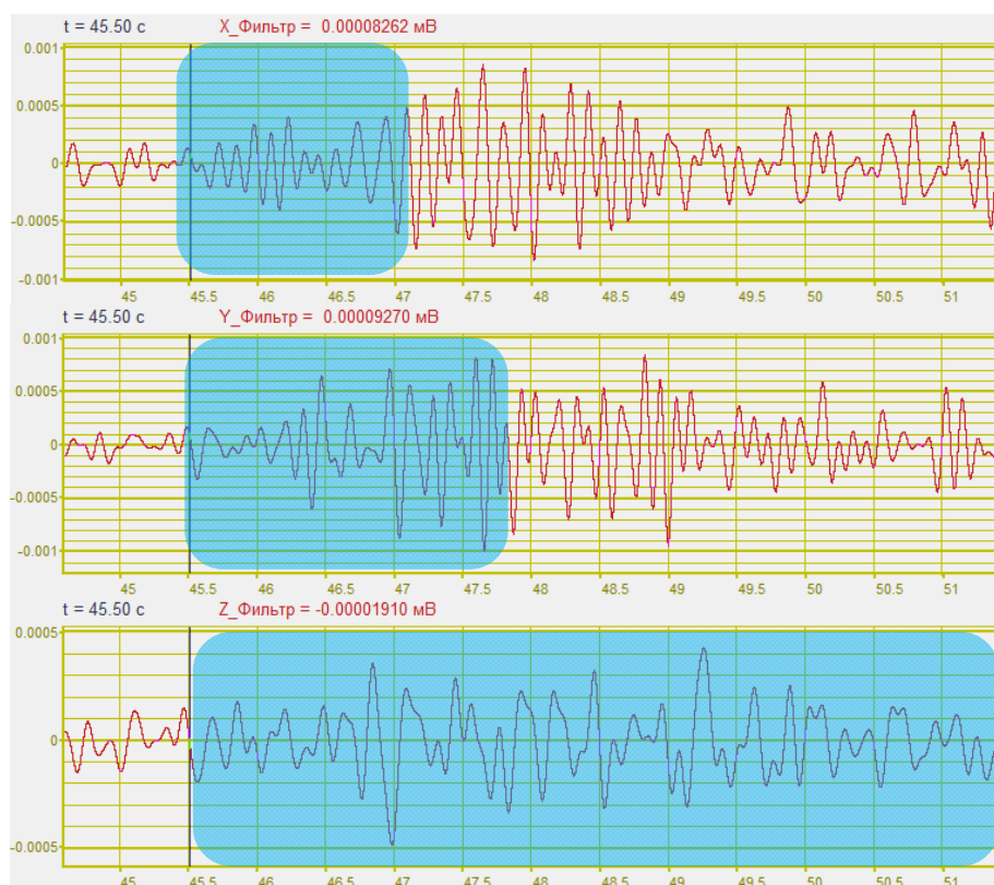
Рис. 11. Компоненты одного из сейсмоматчиков: X-верхний, Y-средний, Z-нижний графики. Увеличение масштаба по оси времени. Данные представлены в относительном времени. Зона неопределенности подсвечена голубой рамкой.
