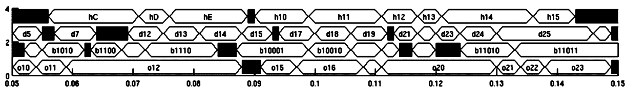
Рис. 2. Временных диаграмм изменения цифровых сигналов, построенная при помощи ПО vmodel
