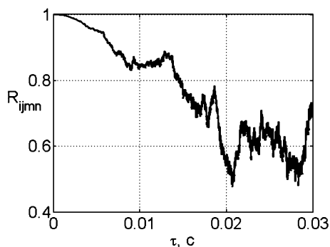
Рис. 5. Корреляционная функция
