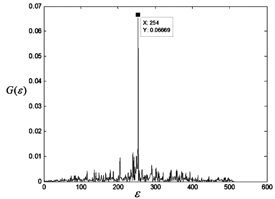
Рис. 4. Пример функции G(\varepsilon) для фактического значения \varepsilon_i = -2 ( q=0 дБ, N=256 )
