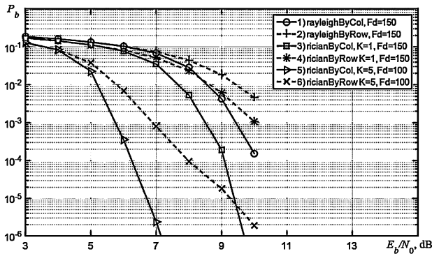
Рис. 3. Характеристики МПД в канале с замираниями при последовательной и параллельной передаче бит
