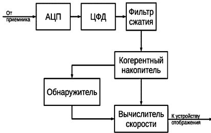
Рис. 1. Общая функциональная схема тракта цифровой обработки РЛС
