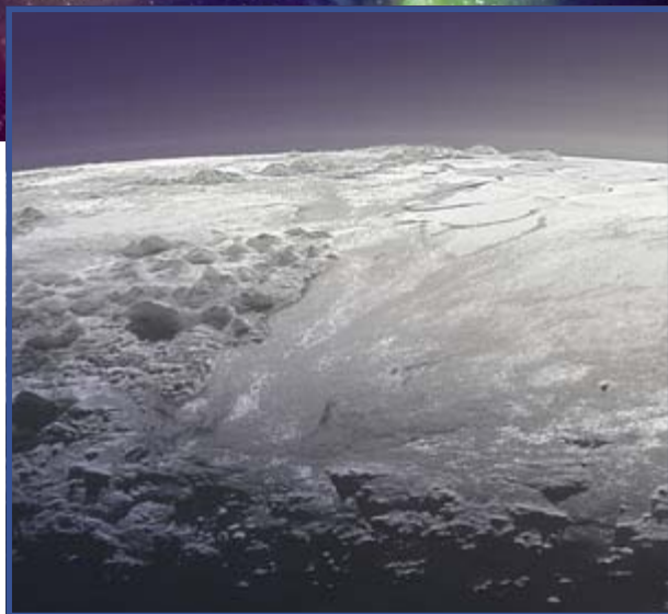
Закат на Плуtone. Снимок сделан пролетевшим мимо автоматическим зондом New Horizons
