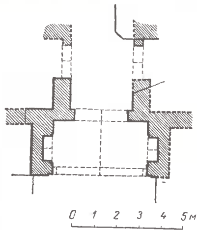
40. Караван-сарай. Общий вид и план портала (обмерный чертёж)
