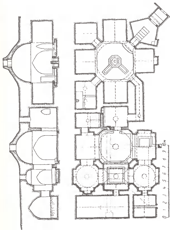
25. Древние бани у ворот Кырхляр-Капы. План и разрез (обмерный чертеж)
