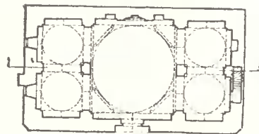
28. Кыхляр-мечеть. Фасад, разрез и план (обмерный чертеж)
