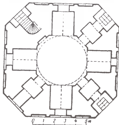
39. Мавзолей Тути-Бикв. Деталь, план (обмерный чертеж)
