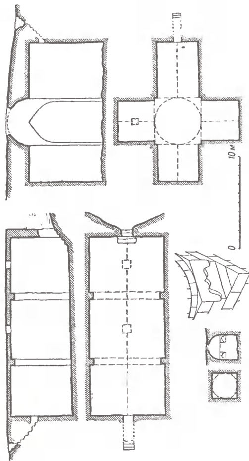
34. Три цистерны в цитадели. Планы и разрезы (обмерный чертеж)
