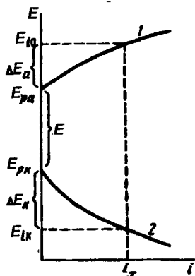
Рис. 9.10. Поляризация анода (1) и катода (2) при электролизе
