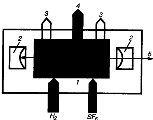
Рис. 9.2. Схема химического лазера: 1 — реактор; 2 — зеркало; 3 — отвод теплоты; 4 — отвод продуктов реакции; 5 — лазерный луч
