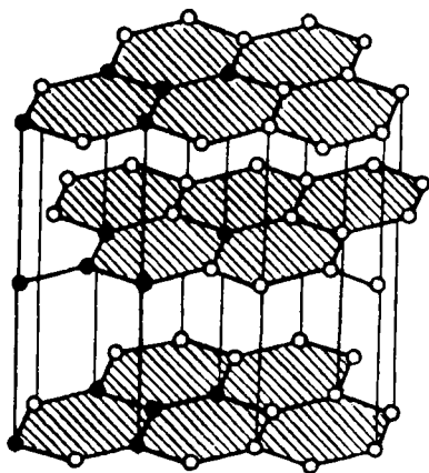
Р и с . 4.9. Структура графита
