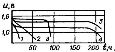
Рис. 9.14. Разрядные кривые первичных элементов одинаковой массы: марганцево-цинковых с солевым (1) и щелочным (2) электролитом, серебряно-цинкового (3), воздушно-цинкового (4) и сульфиджелезнодорожно-литиевого с неводным раствором электролита (5)
