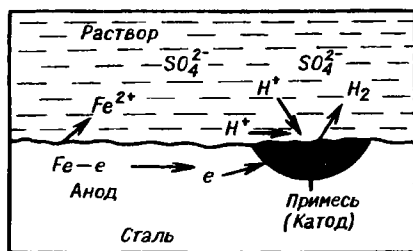
Рис. 10.5. Схема коррозии стали в растворе \text{H}_2\text{SO}_4 с выделением водорода
