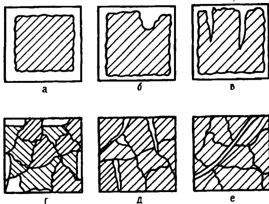
Рис.10.1. Виды коррозионных разрушений: а — равномерное; б — местное; в — точечное; г — избирательное; д — межкристаллическое; е — транскристаллическое
