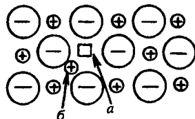
Рис. 4.13. Точечный дефект в ионном кристалле в узле решетки (а) при переходе иона в междоузлие (б)
