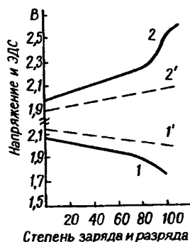
Рис. 9.16. Типичные разрядные (1 и 1') и зарядные (2 и 2') кривые свинцового аккумулятора: 1 и 2 — напряжение; 1' и 2' — ЭДС
