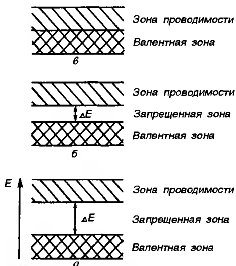
Рис. 4.11. Зонная структура диэлектриков (а), полупроводников (б) и металлов (в)
