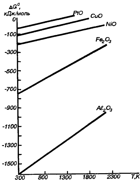
Рис. 10.2. Энергия Гиббса образования некоторых оксидов металлов при p_{\text{O}_2} = 1
