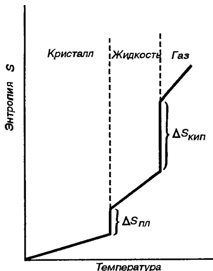
Рис. 5.3. Изменение энтропии вещества с увеличением температуры
