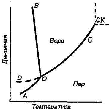
Р и с . 6.1. Диаграмма состояния воды
