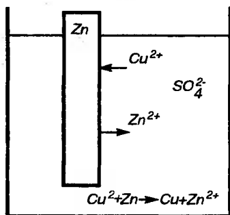
Р и с . 9.1. Взаимодействие цинка с ионами меди (контактное осаждение меди на цинке) в растворе
