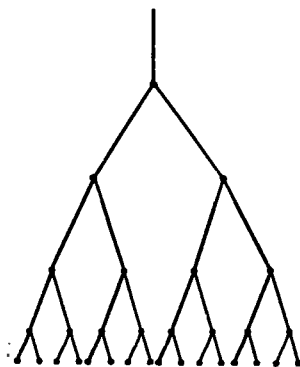
Р и с . 7.5. Схема реакции с разветвленными цепями
