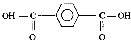
терефталевая кислота
