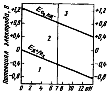
Рис. 9.6 Зависимости потенциалов водородного и кислородного электродов от pH среды при p_{O_2} = p_{H_2} = 1 (100 кПа)
