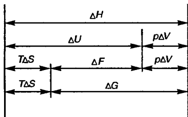
Рис. 5.4. Соотношение термодинамических функций
