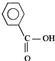
бензойная кислота
