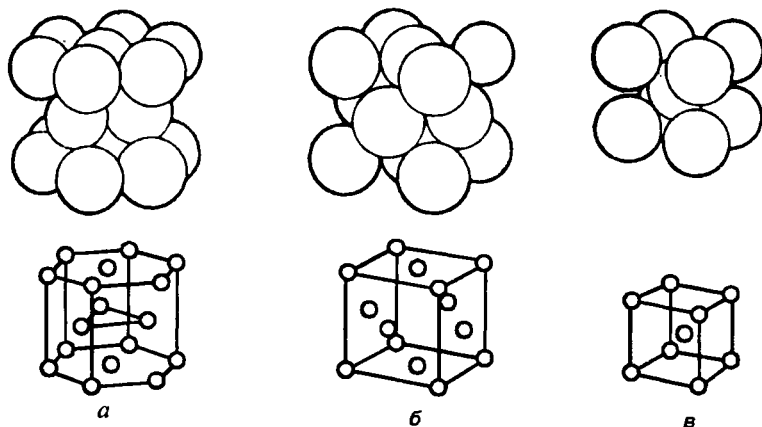
Р и с . 4.6. Трехмерное изображение упаковок шаров: а — гексагональная; б — кубическая гранецентрированная; в — кубическая объемно центрированная
