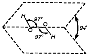
Р и с. 12.7. Структура пероксида водорода
