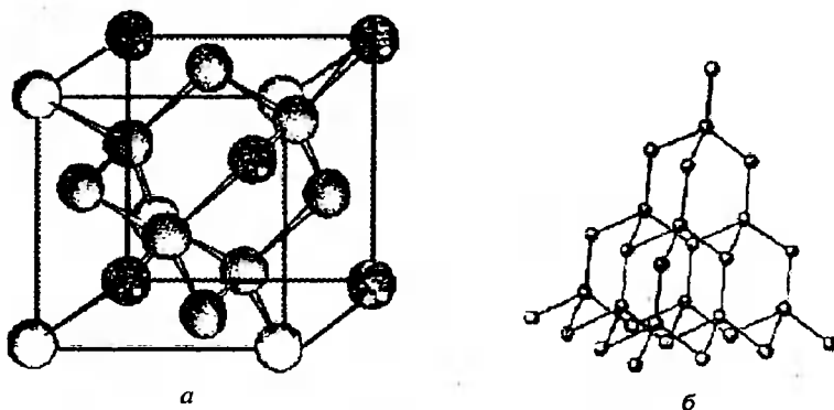
Рис. 4.7. Структура алмаза:
