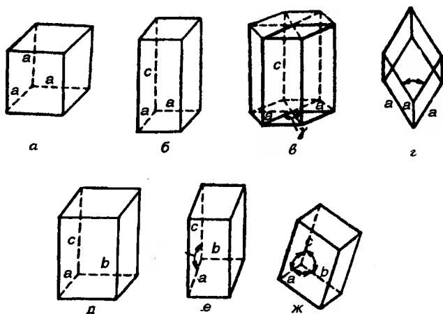
Р и с. 4.5. Геометрические фигуры, отвечающие элементарным ячейкам:
