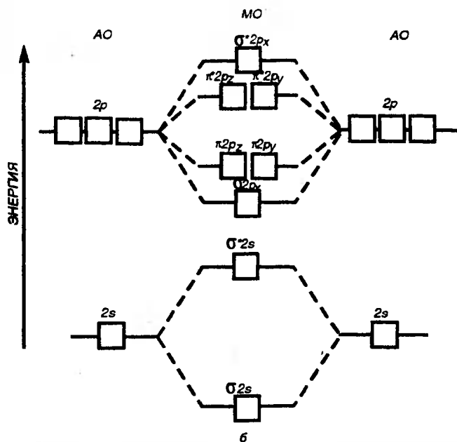
Р и с . 2.16. Диаграмма энергетических уровней АО и МО двухатомных молекул элементов от начала (до N_2 ) (а) и до конца (от O_2 до F_2 ) (б) второго периода
