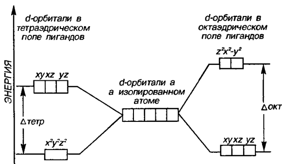
Р и с . 3.5. Энергия d -орбиталей в изолированном атоме и в полях лигандов
