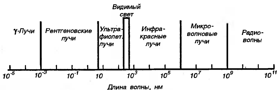
Р и с . 1.1. Спектр электромагнитного излучения
