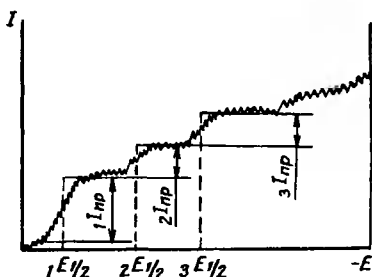
Рис. 16.1. Полярограмма раствора, содержащего несколько катионов
