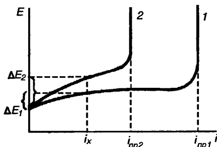
Р и с. 9.8. Кривые потенциал-плотность тока при концентрационной поляризации с перемешиванием (1) и без перемешивания (2)
