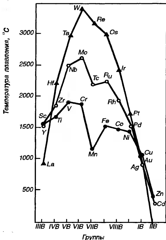
Р и с. 11.10. Изменение температуры плавления d -элементов по группам
