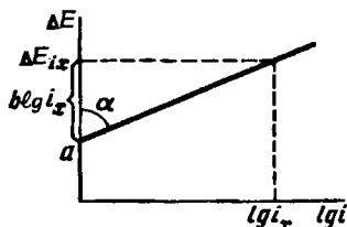
Рис. 9.9. Зависимости электрохимической поляризации электродов от \lg i
