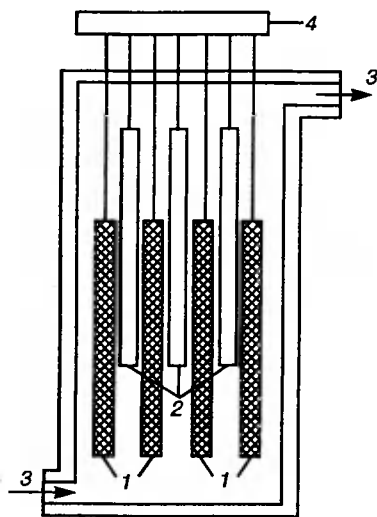
Рис. 17.4. Схема активной зоны атомного реактора:
