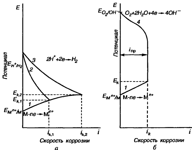
Р и с. 10.6. Коррозионные диаграммы для коррозии с поглощением кислорода (б) и с выделением водорода (а): 1 — анодные кривые растворения металла; 2, 3 — катодные кривые выделения водорода на участках с большим (2) и небольшим (3) перенапряжением; 4 — катодная кривая восстановления кислорода
