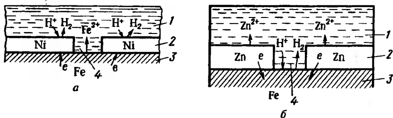
Р и с . 10.8. Схема коррозии железа в кислотном растворе в порах катодного (а) и анодного (б) покрытий:
