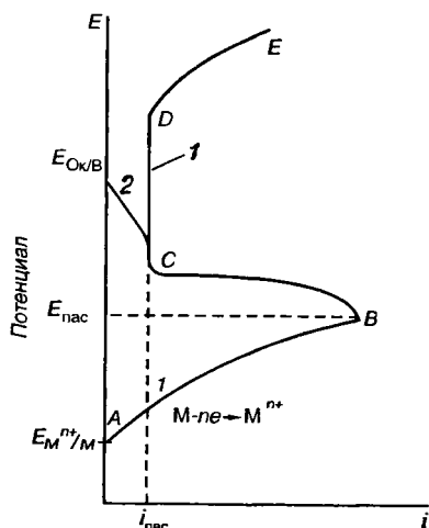
Рис. 10.7. Коррозионная диаграмма для коррозии пассивирующегося металла:
