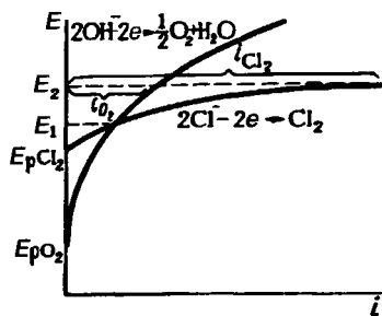
Рис. 9.12. Поляризационные кривые анодного выделения кислорода и хлора
