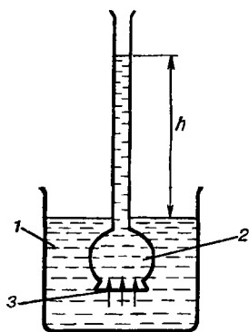
Рис. 8.2. Схема осмометра: 1 — вода; 2 — раствор; 3 — полупроницаемая мембрана
