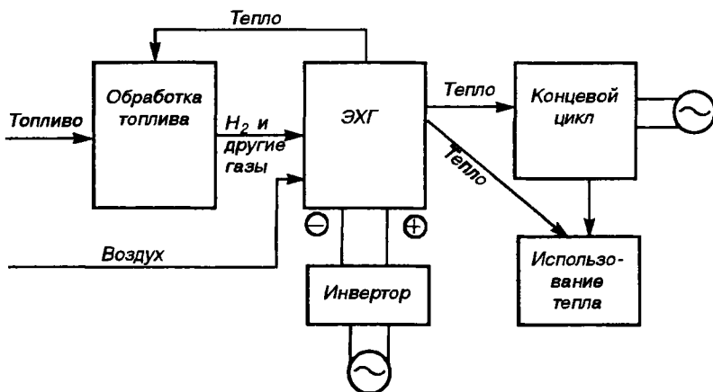
Р и с . 15.6. Блок-схема электрохимической энергоустановки
