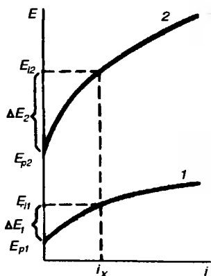
Р и с. 9.7. Поляризационные кривые двух электродов
