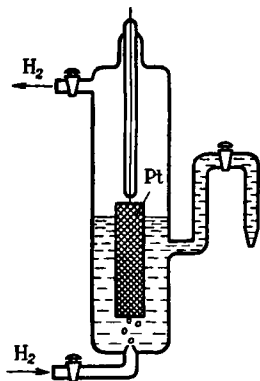
Р и с . 9.5. Схема водородного электрода
