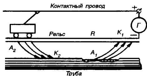
Рис. 10.10. Схема коррозии трубопровода блуждающими токами
