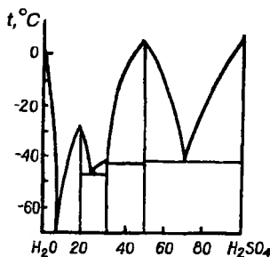
Рис. 6.6. Диаграмма плавления системы \text{H}_2\text{O} - \text{H}_2\text{SO}_4
