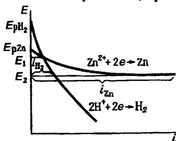
Рис. 9.11. Поляризационные кривые катодного выделения водорода и цинка
