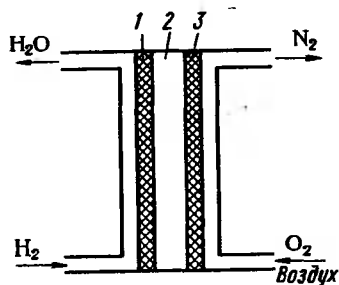
Рис. 9.15. Схема кислородно-водородного топливного элемента:
