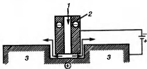
Рис. 9.13. Схема электрохимической обработки металлов:
