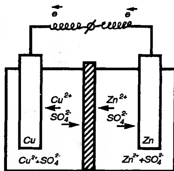
Р и с . 9.4. Схема гальванического элемента Даниэля — Якоби
