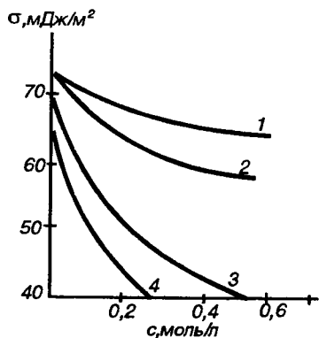
Рис. 6.8. Зависимость поверхностного натяжения \sigma карбоновых кислот от их концентрации:
