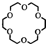
18-Краун-6
