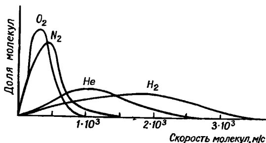
Р и с . 4.1. Распределение молекул по скоростям Максвелла — Больцмана при температуре 298 К
