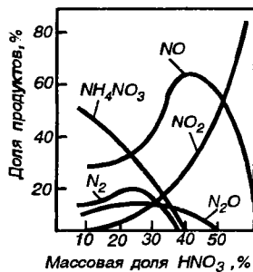
Рис. 12.6. Влияние концентрации HNO_3 на состав продуктов ее восстановления железом
