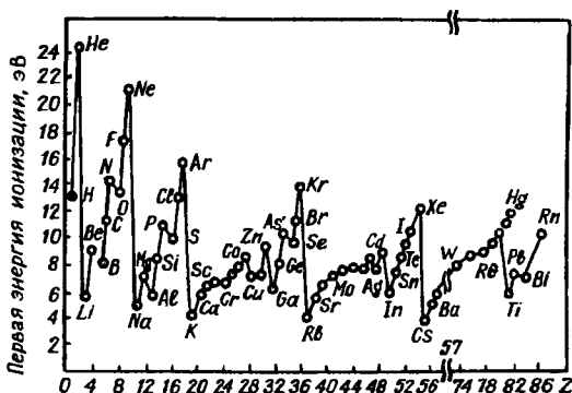
Р и с. 1.6. Зависимость первой энергии ионизации от порядкового номера элемента Z
