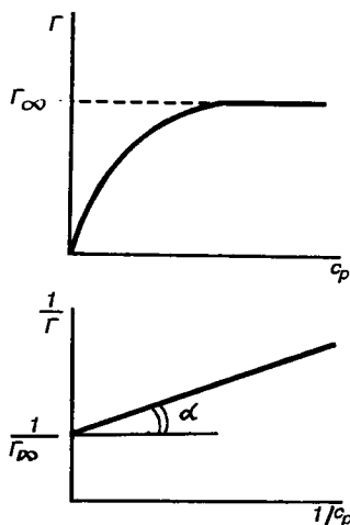
Р и с . 6.7. Изотерма Лэнгмюра в двух формах
