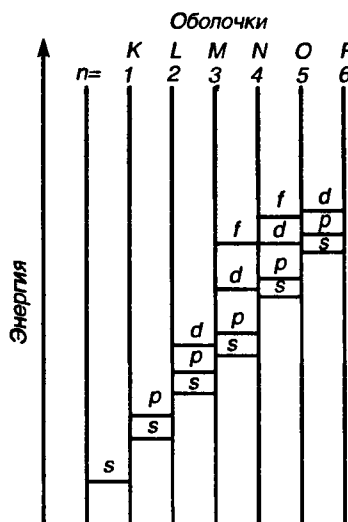
Рис. 1.5. Примерная схема относительного расположения энергетических подуровней в многоэлектронных атомах
