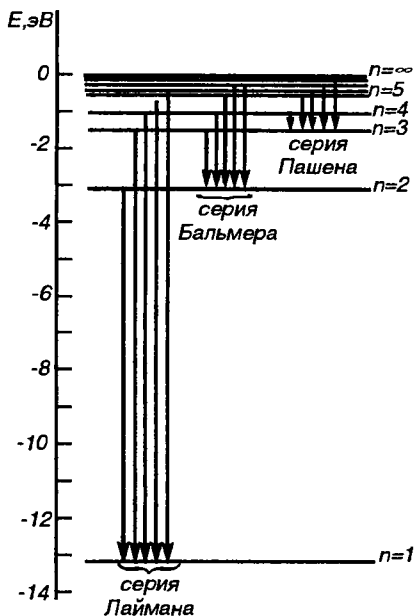
Рис. 1.3. Схема энергетических уровней и квантовые переходы атома водорода
