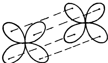
Рис. 2.5. Направления перекрывания атомных d -орбиталей при образовании \delta -связей
