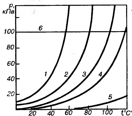
Рис. 4.4. Давление насыщенных паров некоторых жидкостей: ацетона (1), этанола (2), воды (3), уксусной кислоты (4) и этиленгликоля (5). Температура кипения при нормальном давлении (6)
