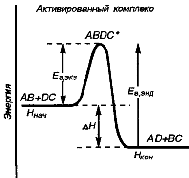
Р и с . 7.3. Энергетическая диаграмма хода реакции с образованием активированного комплекса
