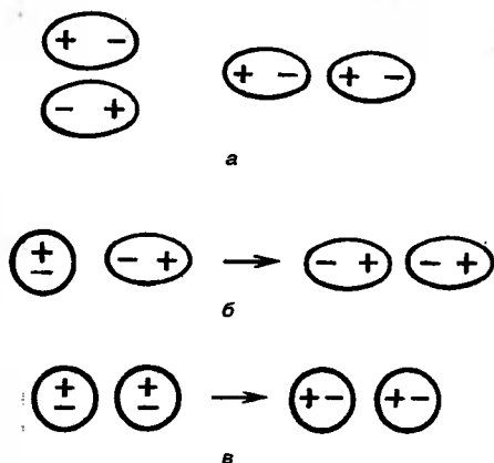
Рис. 3.1. Вандерваальсовы взаимодействия молекул:
