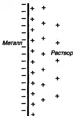
Р и с . 9.3. Двойной электрический слой на границе раздела металл — раствор
