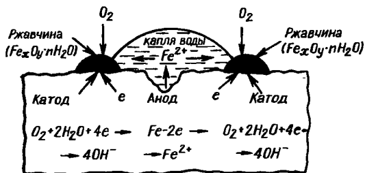
Рис. 10.4. Схема коррозии стали при контакте с водой с поглощением кислорода (атмосферная коррозия)
