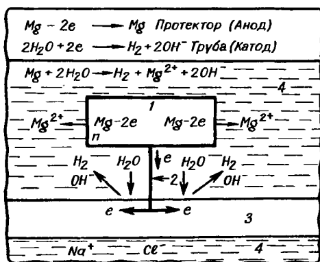
Рис. 10.9. Схема протекторной защиты стального трубопровода магнием в морской воде:
