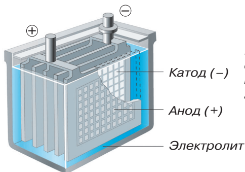
Устройство свинцово- кислотного аккумулятора.
