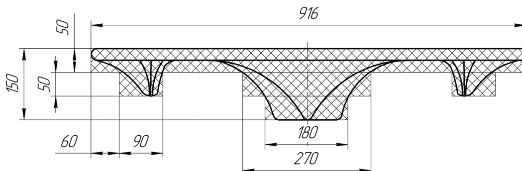
Рис. 4. Схема наклейки пластин «Пеноплэкса».
