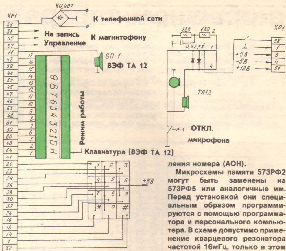
На рисунке изображена схема подключения к плате АОН телефонного аппарата и периферийных устройств.
