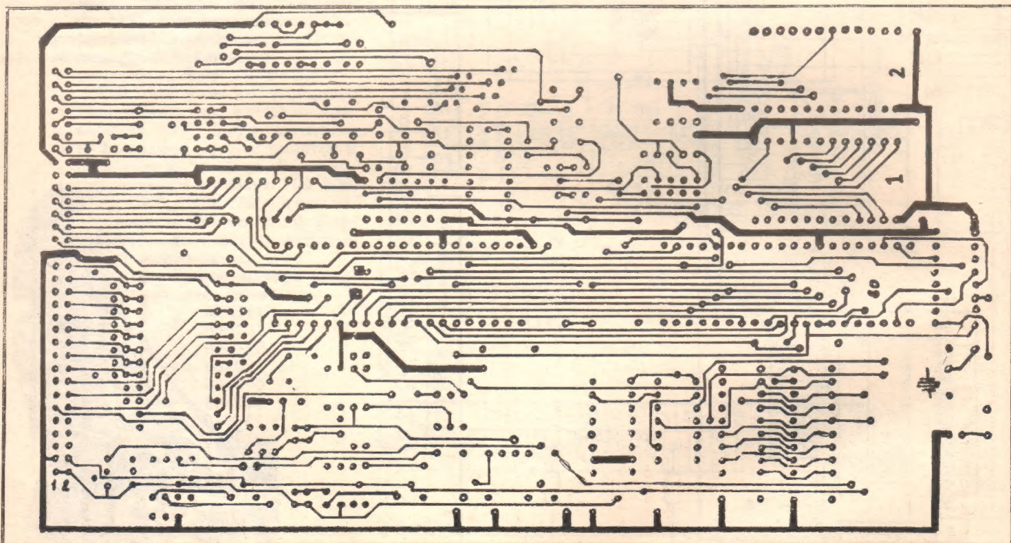
На странице 10 изображена лицевая сторона печатной платы, а на странице 11 — тыльная.
