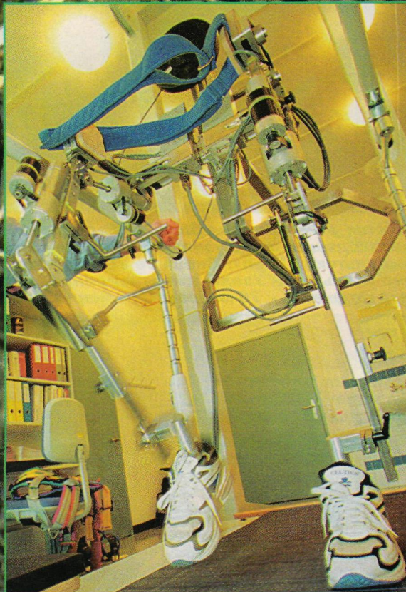
Этот шагающий робот для инвалидов, разработанный в Швейцарии, испытывается на бегущей дорожке университетской клиники в Цюрихе. Устройство не только заменяет инвалидам собственные ноги, но и оказывает им существенную психологическую поддержку.
