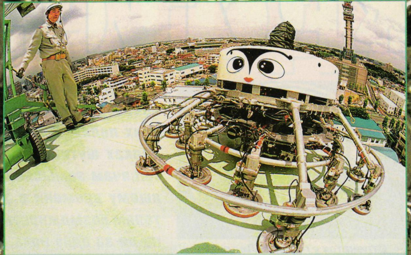
Паукообразный робот фирмы «Токио Газ» обследует громадную емкость для сжиженного газа на предмет выявления трещин. Робот снабжен 16-ю вакуумными присосками и микроволновым поисковым локатором.
