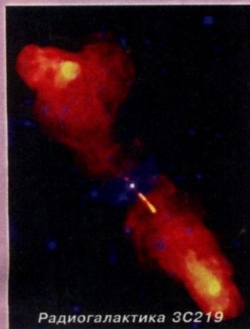
Радиогалактика 3C 219
