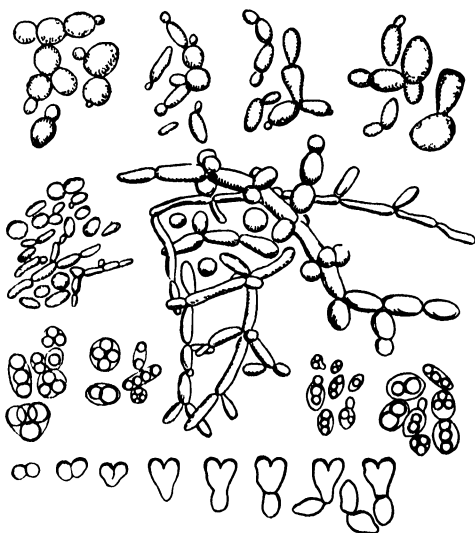
Рис. 4. Почкование.
