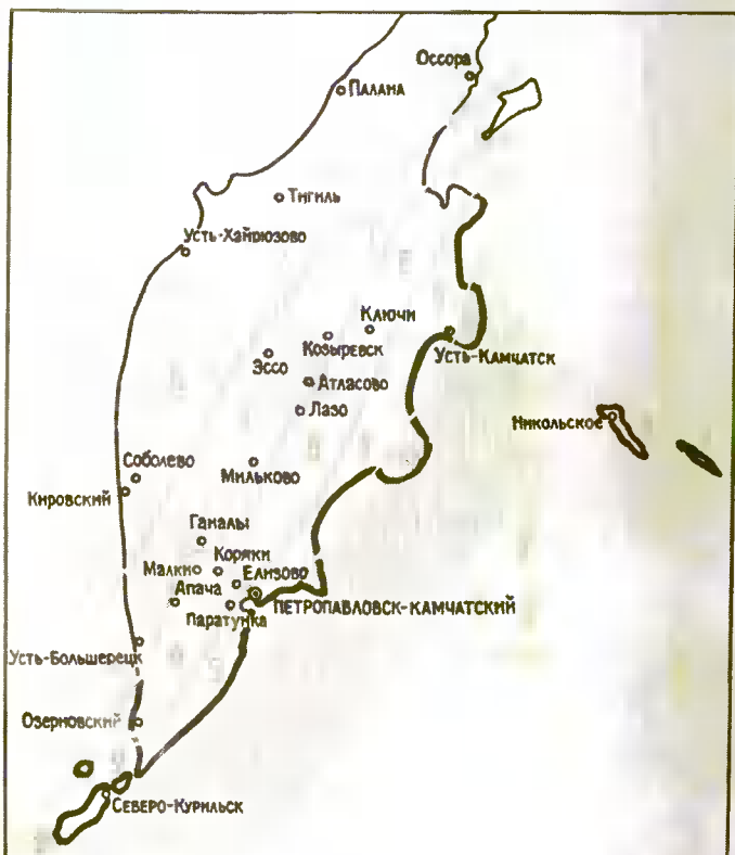
Карта Камчатки с указанием сейсмоопасности (в баллах) различных регионов.
