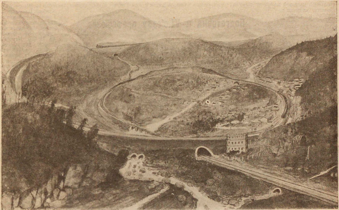
Общий вид Хингайской станции. Если поезд будет длиной в 2½ версты, то паровоз будет находиться под последними вагонами состава.
