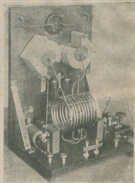
Передатчик коротких волн для любительских целей. Вид сзади.
