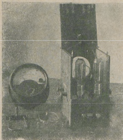
Передатчик для волн в 2\frac{1}{2} метра.
