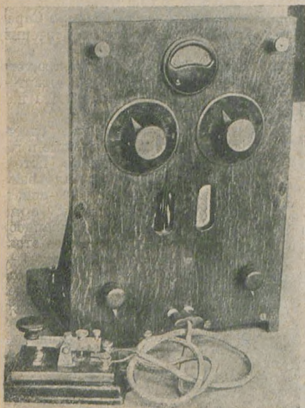
Передатчик коротких волн для любительских целей. Вид спереди.
