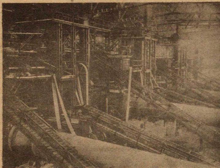
Недавно закончен постройкой Подпильский фосфоритный завод, первый по мощности не только в СССР, но и в Европе. Несмотря на трудности снабжения завод благодаря усилии рабочих и персонала построен за одиннадцать месяцев. На снимках: слева—общий вид размольного и машинного отделений завода; справа—вид на восемь силосов для хранения фосфоритной муки
