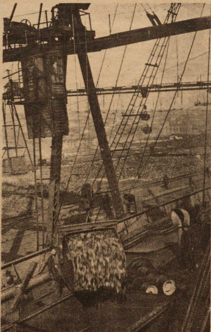
В Мариупольском порту. Механическая подача бадь с углем в трюм парохода
