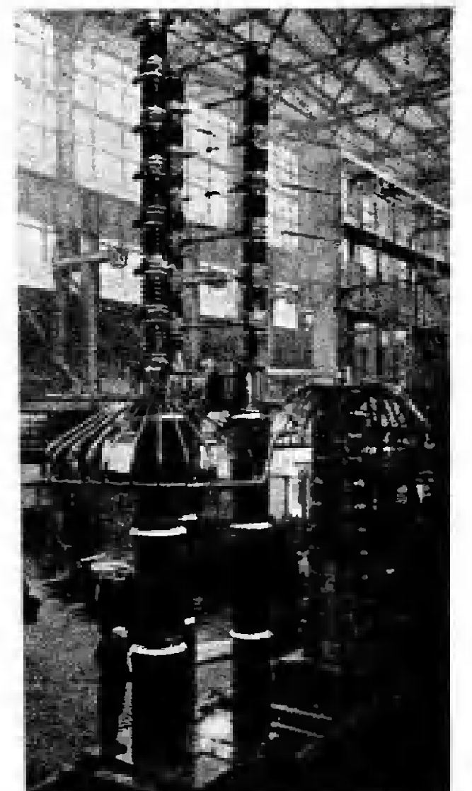
На сборке воздушных выключателей для линии электропередач Куйбышев — Москва.
