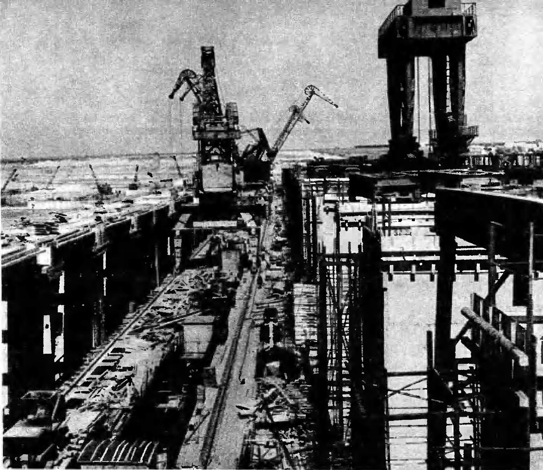
Заканчивается строительство здания Каховской ГЭС.
