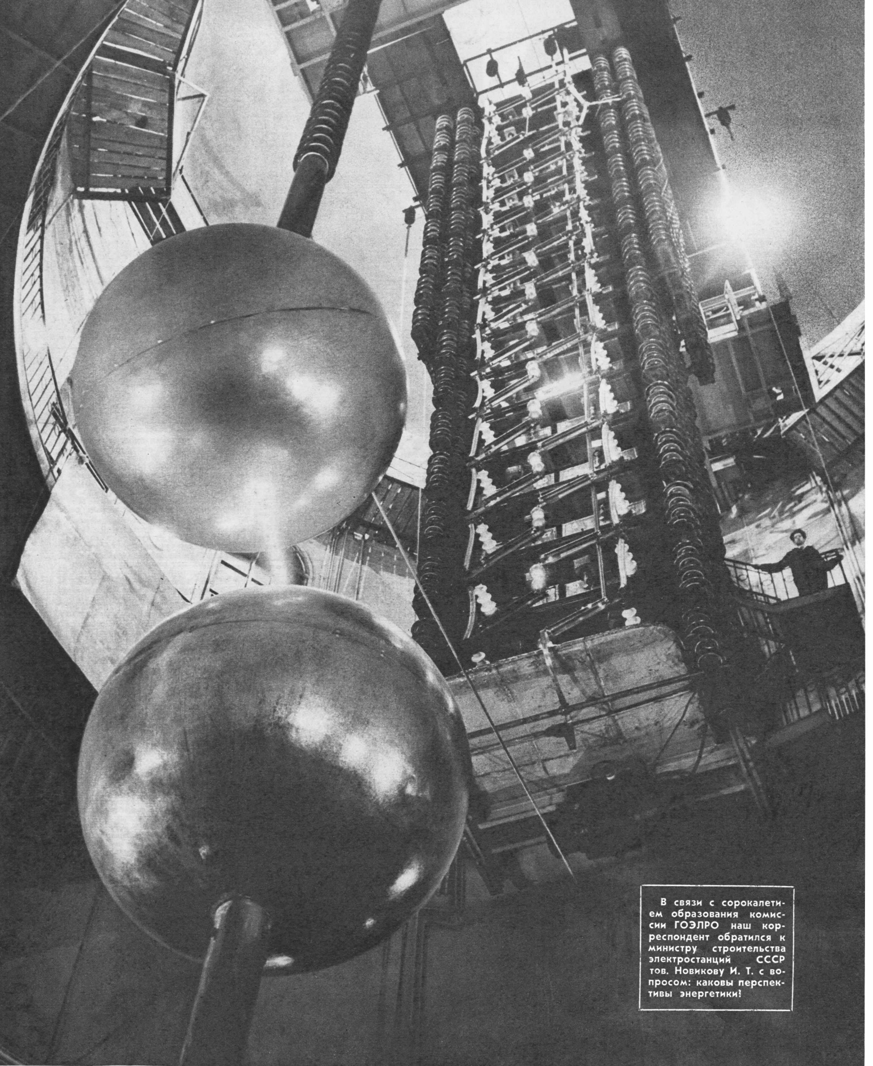
В лаборатории высоковольтного газового разряда Энергетического института имени Г. М. Кржижановского Академии наук СССР. Фото Д. Шоломовича.
