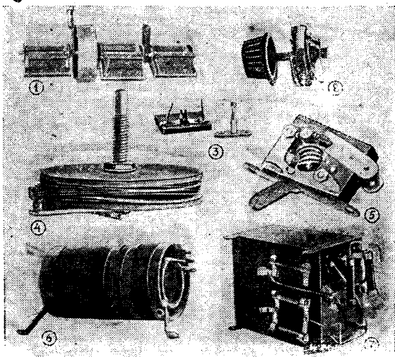
„Объяснимые“ детали: 1. Агрегат (строенный конденсатор). 2. Волном-контроль (регулятор громкости). 3. Ш. выключатель (выключатель анодного напряжения). 4. Конденсатор обратной связи. 5. Выключатель сети. 6. Катушки сеточного контура и обратной связи. 7. Конденсатор фильтра и сцепляющий
