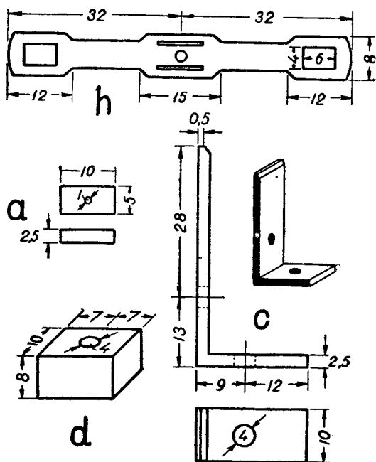
Рис. 2. Детали пружины d , полюсных наконечников С , бруска d и пластинки а .
