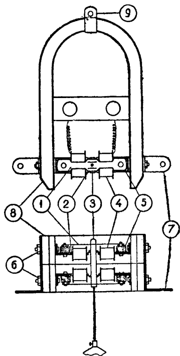
Рис. 1. Собранный механизм. 1—пружина h , 2—полюсные наконечники С , 3—якорь, 4—катушки, 5—деревянные бруски d , 6—болтики, 7—плаки для скрепления магнитов, 8—магниты, 9—петля подвески.
