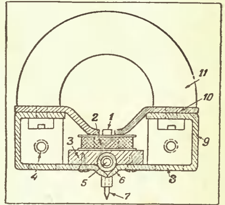
Рис. 3. 1 — вибратор лопатки, 2 — катушка, 3 — планка (латунь), 4 — отверстие для крепления, 5 — отверстие для крепежного винта, 6 — резиновая трубка, 7 — игла, 8 — отверстие для отверстия, 9 — коробка магнитопровода, 10 — полюсные наконечники, 11 — магнит
