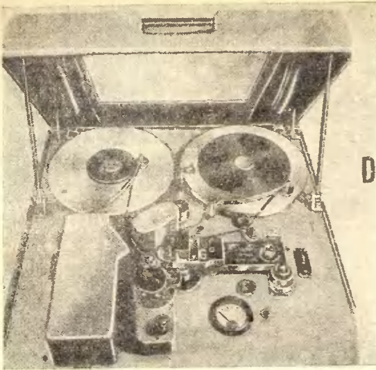
Рис. 2. Общий вид аппарата для записи на зачерненной пленке
