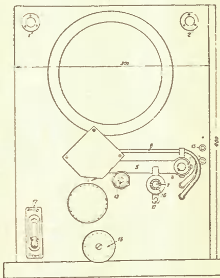
Рис. 5. Расположение деталей на передней панели: 1 и 2 — сигнальные лампочки; 3 — отверстие для динамика; 4 — рекордер; 5 — тонарм рекордера; 6 — токоподводящие шнуры; 7 — направляющая втулка рекордера; 8 — направляющая; 9 — винт смещения; 10 — гайка смещения; 11 — направляющая, предохраняющая гайку от вращения; 12 — щека, ведущая тонарм; 13 — ручка переключателя; 14 — барабан для записи и воспроизведения; 15 — гнезда адаптера; 16 — направляющий ролик; 17 — выключатель мотора
