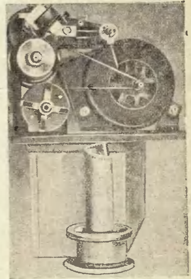
Рис. 8. Установка т. Мени. Вид сбоку
