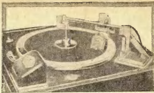
Рис. 3. Звукозаписывающая приставка в действии
