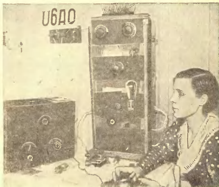
Секретарь Азово-Черноморской секции коротких волн т. Кожарина у своего передатчика
