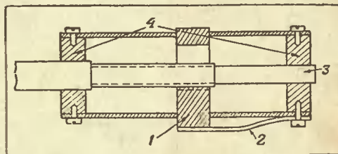
Рис. 26. Супорт т. Трушина: 1—полугойка; 2—пружина, сцепляющая полугойку с резьбой винта; 3 — направляющая с винтом; 4 — направляющие втулки
