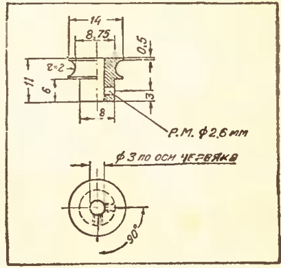
Рис. 2. Шкив а
