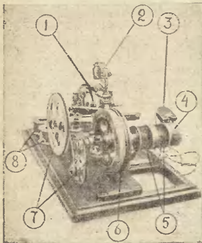
Рис. 9. Установка т. Минакова: 1 — мотор; 2 — рекордер; 3 — адаптер; 4 — барабан для воспроизведения; 5 — барабаны для записи; 6 — шкив-маховик на валу барабана; 7 — ременной перебор механизма смещения рекордера; 8 — натяжные ролики
