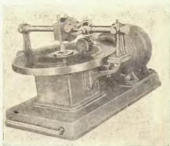
Аппарат шорнограф для записи звука на целлулозные диски
