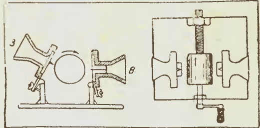
Рис. 1. Фонограф Эдисона
