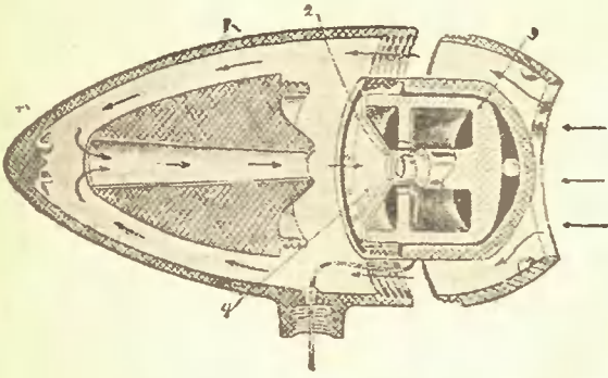
Рис. 1. Устройство «микродуктора»: 1—бакелитовый каркас, 2 — катушка, 3 — постоянный магнит, 4 — мембрана
