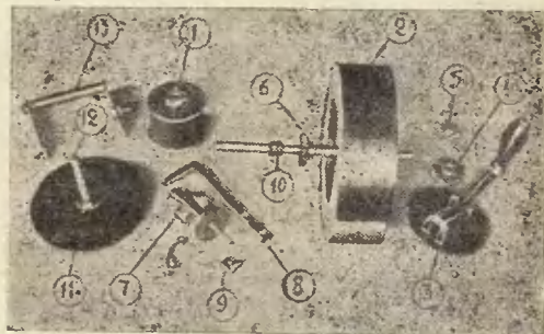
Рис. 13. Детали установки т. Успенского: 1 — барабан для записи; 2 — маховик; 3 и 4 — шестерни зубчатого механизма; 5 — нит крепление большой шестерни; 6 — червячная шестерня центробежного регулятора; 7 — центробежный регулятор; 8 — стойка крепления центробежного регулятора; 9 — подпятник центробежного регулятора; 10 — резиновое кольцо фрикционного перебора механизма смещения рекордера; 11 и 12 — фрикционный диск и нит смещения рекордера; 13 — кровштейн крепления винта смещения
