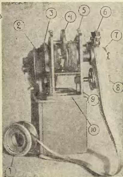
Рис. 7. Установка т. Мени. Вид спереди: 1 — натяжной ролик; 2 — мотор; 3 — ремennая передача механизма смещения рекордера; 4 — шестерня зубчатого перебора смещения рекордера; 5 — крепление шестерни зубчатого перебора; 6 — рекордер; 7 — барабан для записи и воспроизведения; 8 — направляющий ролик; 9 — станина
