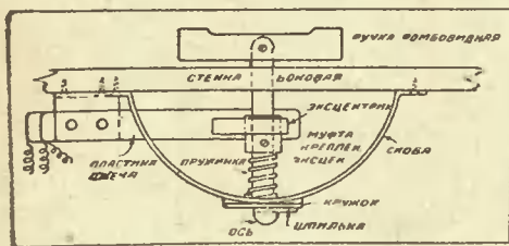
Рис. 23. Переключатель т. Грудева
