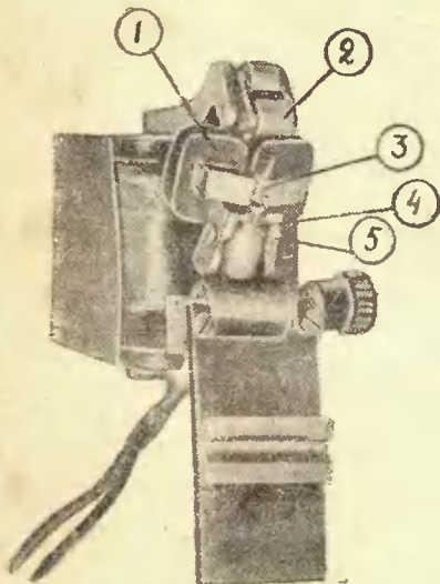
Рис. 18. Рекордер т. Федорова: 1 — модуляционные катушки; 2 — роляковый ограничитель глубины борозды; 3 — якорь; 4 — пружина крепления якоря; 5 — лапы для изменения степени демпфирования
