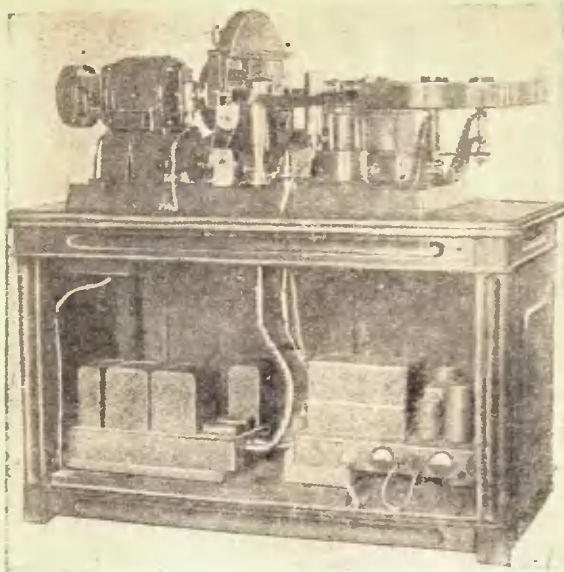
Общий вид телекинопередатчика
