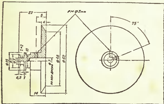
Рис. 5. Шкив в
