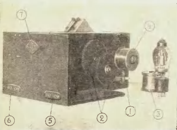
Рис. 3. Установка т. Татаржицкого. Вид со стороны барабана воспроизведения и фрикционного перебора механизма перебора: 1 — рычаг выключения фрикционного перебора; 2 — эбонитовые диски фрикционного перебора; 3 — натяжной ролик; 4 — барабан для звуковоспроизведения; 5 — гнезда выхода адаптера; 6 — гнезда для подачи переменного тока к мотору; 7 — панель для подачи звуковой частоты и подмагничивания на рекордер
