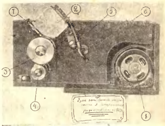
Рис. 2. Установка т. Татаржицкого. Вид со стороны барабана записи: 1 — мотор; 2 — рекордер; 3 — барабан для записи; 4 — направляющий ролик; 5 — крепление рекордера к направляющей; 6 — подшипники винта подачи; 7 — ограничитель глубины борозды
