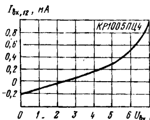
Типовая зависимость входного тока по выводу 12 от напряжения на выводе 12 при T=+25^\circ С
