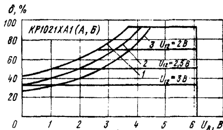
Типовые зависимости коэффициента заполнения \delta = t/T от напряжения обратной связи на выводе 8:
