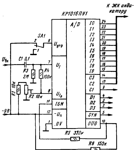
Типовая схема включения микросхемы КР1016ПУ1
