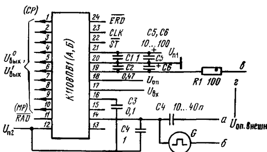
Типовая схема включения АЦП К1108ПВ1 (А, Б). Конденсаторы C2 и C4 керамические
