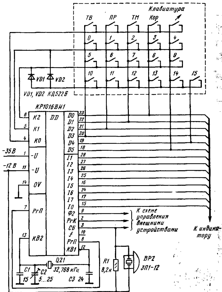
Типовая схема включения микросхемы КР1016ВИ1
