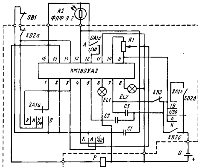
Типовая схема включения микросхем КМ189ХА2, КС189ХА2, КР189ХА2 в фотоаппарате «Силуэт-электрон»
