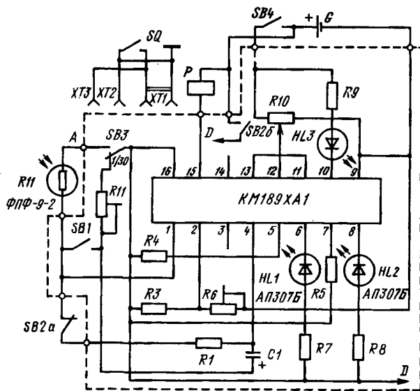
Принципиальная электрическая схема включения микросхем KM189XA1, KC189XA1, KP189XA1 в фотоаппарате «Силуэт-автомат» с сигнализацией «мало — норма» (1/30)
