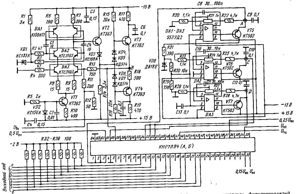
ипловая схема включения АЦП К1107ПВ4 (А, Б) с входными буферными усилителями формирователей регулируемых опорных напряжений и гистерезиса
