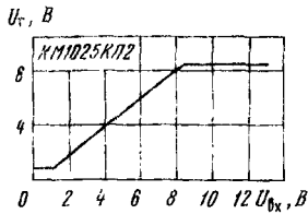
Типовая зависимость напряжения питания генератора от входного напряжения КМ1025КП2
