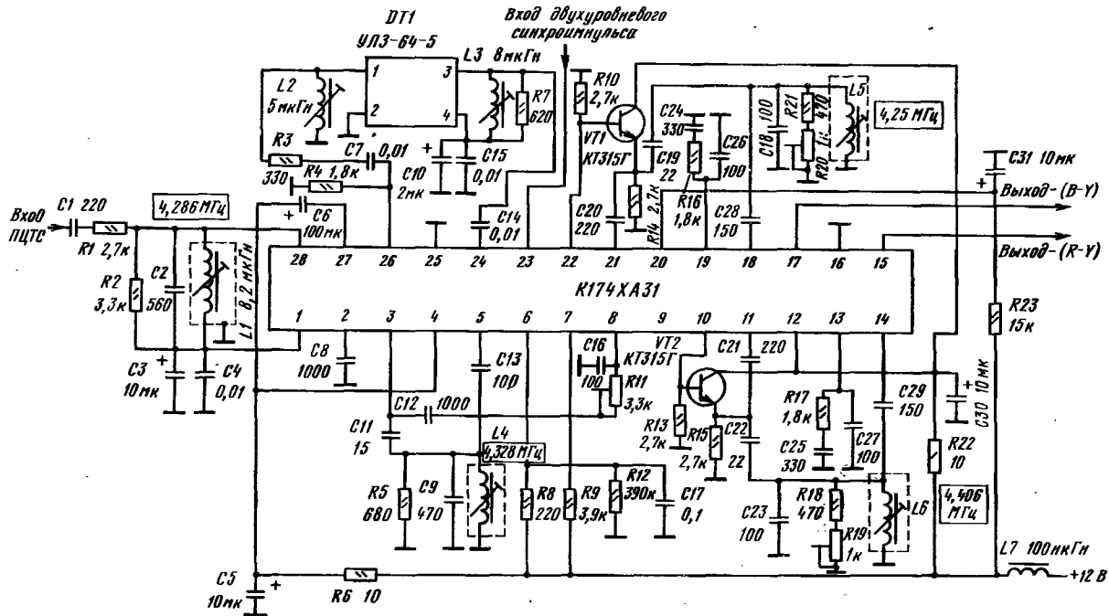
Типовая схема включения микросхемы К174ХА31:
