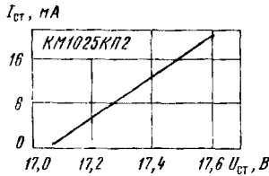
Типовая зависимость тока стабилизатора от напряжения стабилизации КМ1025КП2
