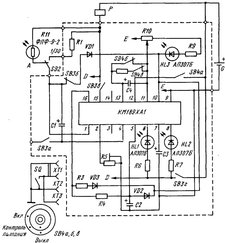
Принципиальная электрическая схема включения микросхем КМ189ХА1, КС189ХА1, КР189ХА1 в фотоаппарате «Силут» с сигнализацией в импульсном режиме
