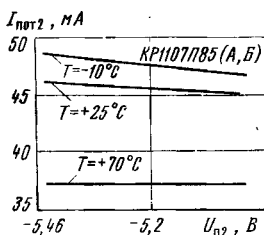
Типовые зависимости тока потребления I_{пот2} от напряжения питания U_{п2} при различных температурах окружающей среды и U_{п1} = 5 В
