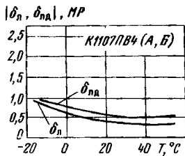
Типовые зависимости нелинейности \delta_n и дифференциальной нелинейности \delta_{нд} от температуры окружающей среды АЦП К1107ПВ4 (А, Б)
