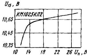
Типовая зависимость напряжения на выходе стабилизатора от напряжения питания КМ1025КП2
