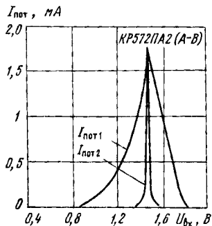
Типовые зависимости токов потребления КР572ПА2 (А—В) от напряжения на цифровых входах при U_{\text{н1}} = 5 В, U_{\text{н2}} = 15 В
