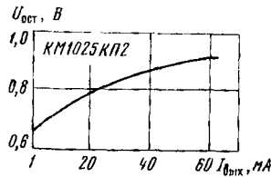
Типовая зависимость остаточного напряжения от выходного тока КМ1025КП2 при U_n = 15 В для малых значений выходных токов
