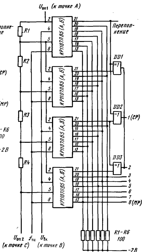
Схема включения входов и выходов четырех БИС КР1107ПВ5 (А, Б) при увеличении числа разрядов АЦП до восьми. Точки подключения А, В, С указаны на типовой схеме включения
