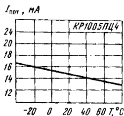
Типовая зависимость тока потребления от температуры окружающей среды при U_n=9 В
