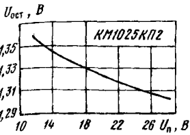
Типовая зависимость остаточного напряжения от напряжения питания КМ1025КП2 при выходном токе 200 мА
