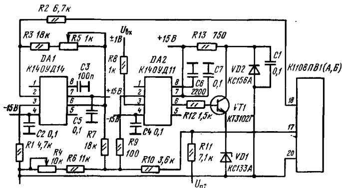
Принципиальная электрическая схема подключения аналоговых входов АЦП К1108ПВ1 для работы в режиме преобразования биполярного аналогового сигнала
