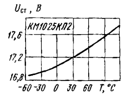
Типовая зависимость напряжения на выходе стабилизатора КМ1025КП2 от температуры окружающей среды
