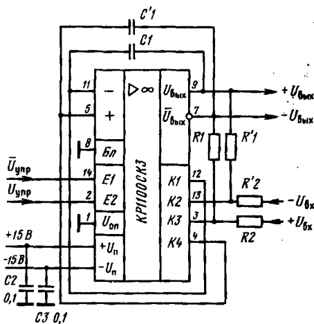
Типовая схема включения микросхемы КР1100СК3 с симметричными входом и выходом
