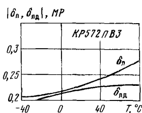
Типовая зависимость нелинейности и дифференциальной нелинейности АЦП КР572ПВ3 от температуры окружающей среды
