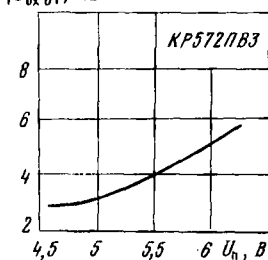
|U_{вх0}|, мВ
