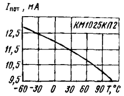
Типовая зависимость тока потребления КМ1025КП2 от температуры окружающей среды при U_n = 18 В
