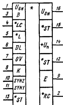
КМ1025КП2
