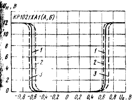
Типовые зависимости напряжения на выходе микросхемы (вывод 11) от напряжения на выводе 6:
