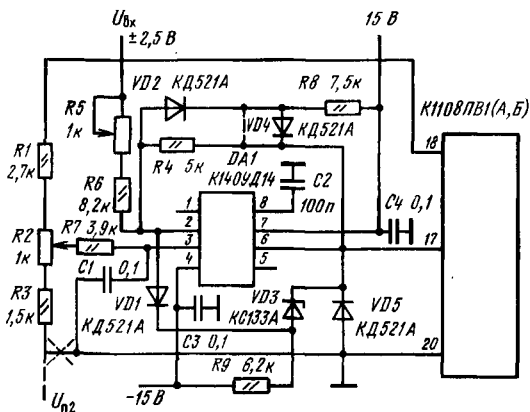
Принципиальная электрическая схема подключения аналоговых входов АЦП К1108ПВ1 для преобразования однополярного и биполярного (соединение показано штриховой линией) сигналов с помощью входного ОУ в инвертирующем режиме усиления:
