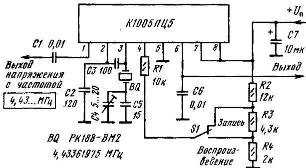
Типовая схема включения микросхемы К1005ПЦ5
