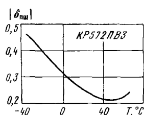
Типовая зависимость абсолютной погрешности преобразования в конечной точке шкалы АЦП КР572ПВ3 от температуры окружающей среды
