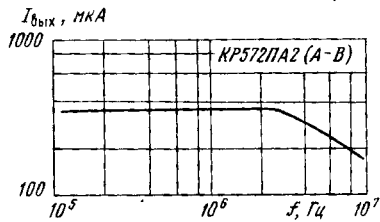
Типовая зависимость выходного тока ЦАП КР572ПА2 (А—В) от частоты изменения опорного напряжения при T = +25^\circ \text{C}
