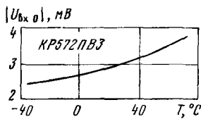
Типовая зависимость напряжения смещения нуля АЦП КР572ПВ3 от температуры окружающей среды
