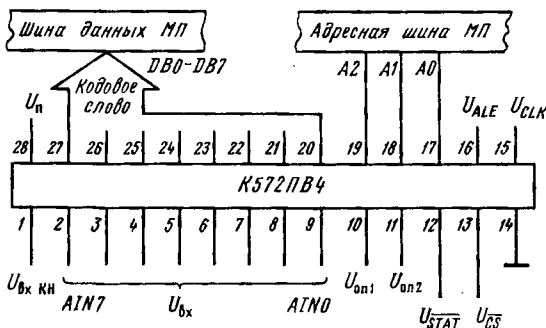
Типовая схема включения БИС АЦС К572ПВ4
