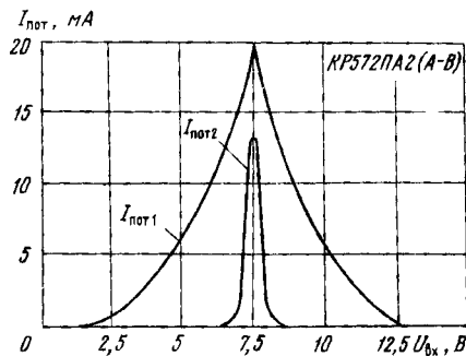
Типовые зависимости токов потребления КР572ПА2 (А—В) от напряжения на цифровых входах при U_{\text{н1}} = U_{\text{н2}} = 15 В
