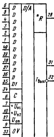
КР572ПА2 (А—В)
