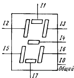
Коды сегментов десятичной цифры на семисегментном индикаторе
