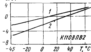
U_{вх0} , мВ
