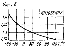
Типовая зависимость напряжения на выходе стабилизатора КМ1025КП2 от температуры окружающей среды
