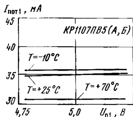
Типовые зависимости тока потребления I_{пот1} от напряжения питания U_{п1} при различных температурах окружающей среды и U_{п2} = -5,2 В
