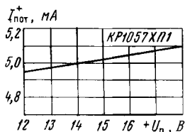
Типовая зависимость тока потребления от положительного источника питания от его напряжения при T = +25^\circ С
