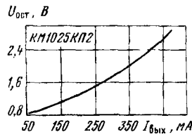
Типовая зависимость остаточного напряжения от выходного тока КМ1025КП2 при U_n = 15 В для больших значений выходных токов
