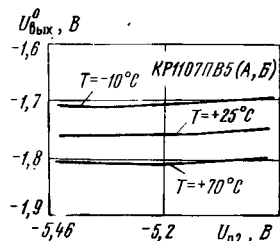
Типовые зависимости выходного напряжения низкого уровня от напряжения питания U_{п2} при различных температурах окружающей среды и U_{п1} = 5 В
