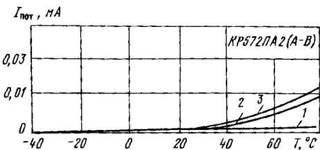
Типовые зависимости токов потребления КР572ПА2 (А—В) от температуры окружающей среды:
