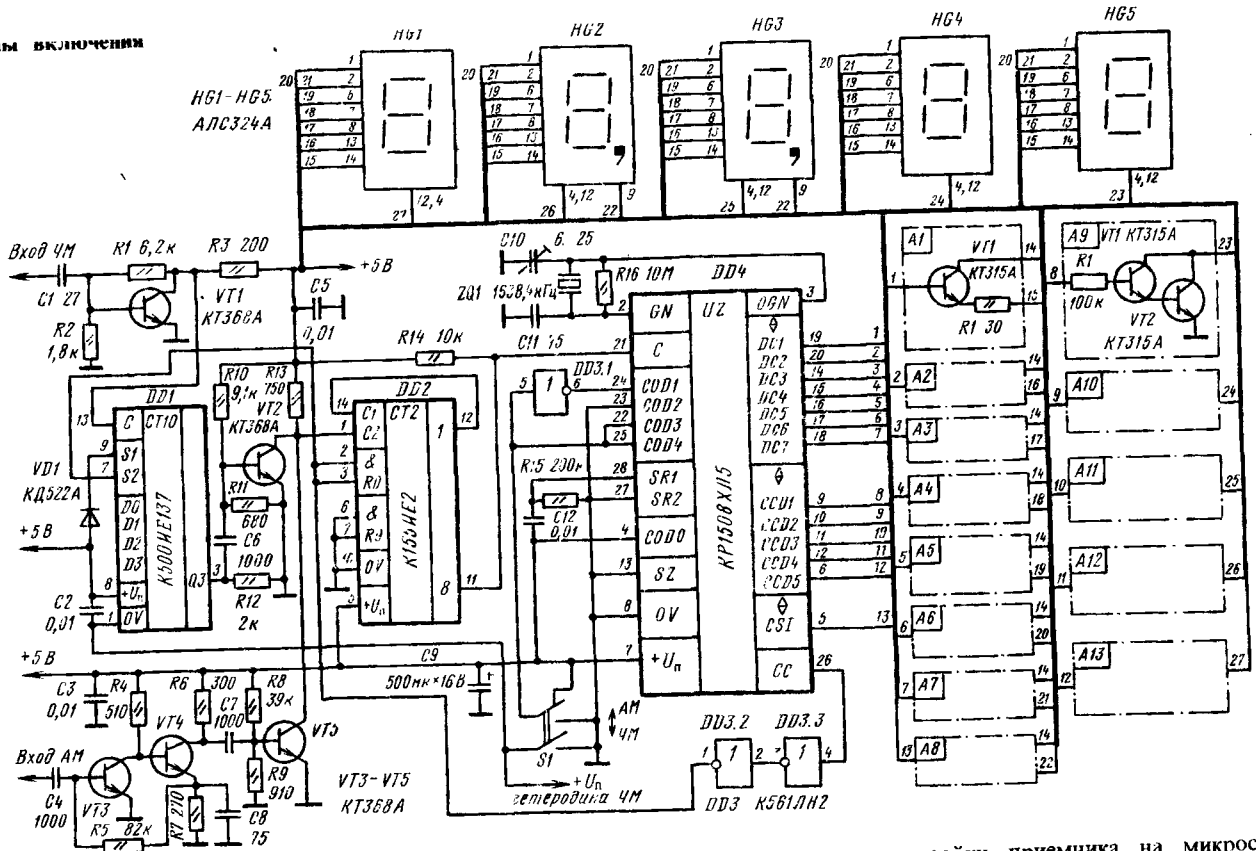
Принципиальная электрическая схема устройства цифрового отсчета частоты настройки приемника на микросхеме KP150BXL5 [12]
