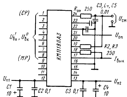
Типовая схема включения ЦАП КМ1118ПАЗ (КР1118ПАЗ) с расширенным диапазоном выходного тока
