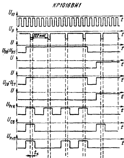
Временные диаграммы выходных (а) и входных (б) импульсов на выходах D0—D5 по входу К0 микросхемы КР1016ВИ1
