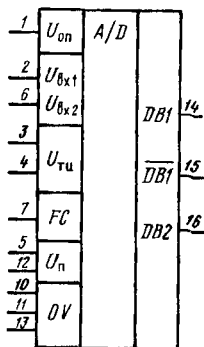
КМ1126ПВ1, КМ1126ПВ1
