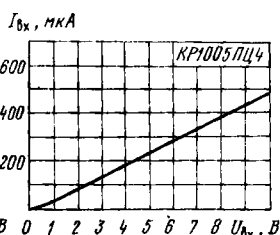
Типовая зависимость входного тока выводов управления 3, 4, 6, 7, 8, 10, 11 от входного напряжения на этих выводах при T=+25^\circ С
