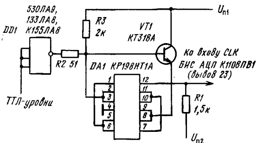
Принципиальная электрическая схема узла сопряжения БИС АЦП К1108ПВ1 с цифровыми ТТЛ-микросхемами по входу CLK
