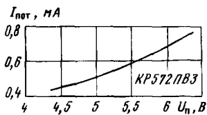
Типовая зависимость тока потребления КР572ПВ3 от напряжения питания
