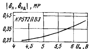
Типовая зависимость нелинейности и дифференциальной нелинейности АЦП КР572ПВ3 от напряжения питания
