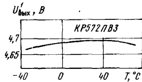
Типовая зависимость выходного напряжения высокого уровня АЦП КР572ПВ3 от температуры окружающей среды
