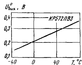
Типовая зависимость выходного напряжения низкого уровня АЦП КР572ПВ3 от температуры окружающей среды
