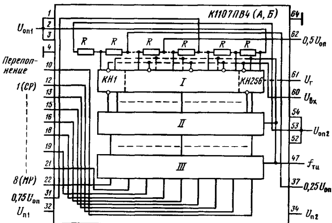
Функциональная электрическая схема БИС АЦП считывания К1107ПВ4 (А, Б)
