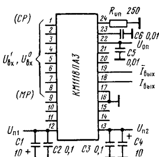
Типовая схема включения ЦАП КМ1118ПАЗ (КР1118ПАЗ)
