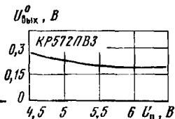
Типовая зависимость выходного напряжения низкого уровня АЦП КР572ПВ3 от напряжения питания
