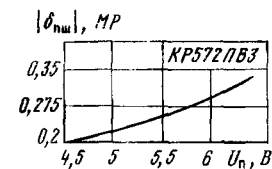
Типовая зависимость абсолютной погрешности преобразования в конечной точке шкалы АЦП КР572ПВ3 от напряжения питания
