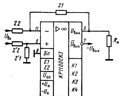
Схема включения парафазного операционного усилителя с симметричным входом и несимметричным выходом
