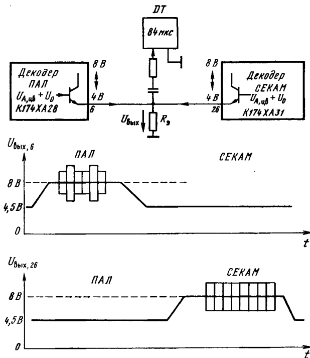
Эпюры выходных напряжений усилителей сигналов цветности микросхем K174XA28 и K174XA31 в двухстандартном декодере сигналов цветности ПАЛ/СЕКАМ с общей линией задержки
