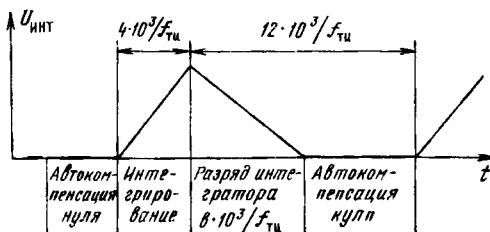
Временная диаграмма работы БИС АЦП КР572ПВ5
