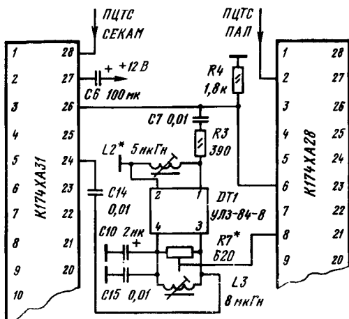
Схема включения общей линии задержки и двухстандартном декодере сигналов цветности ПАЛ и СЕКАМ на микросхемах K174XA28 и K174XA31
