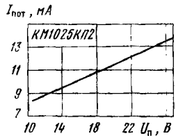
Типовая зависимость тока потребления от напряжения питания КМ1025КП2
