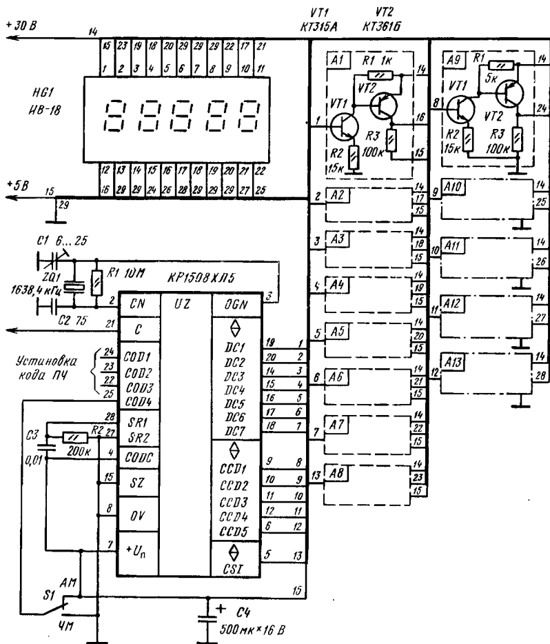
Принципиальная электрическая схема включения вакуумно-люминесцентного цифрового индикатора совместно с микросхемой КР1508ХЛ5 [12]
