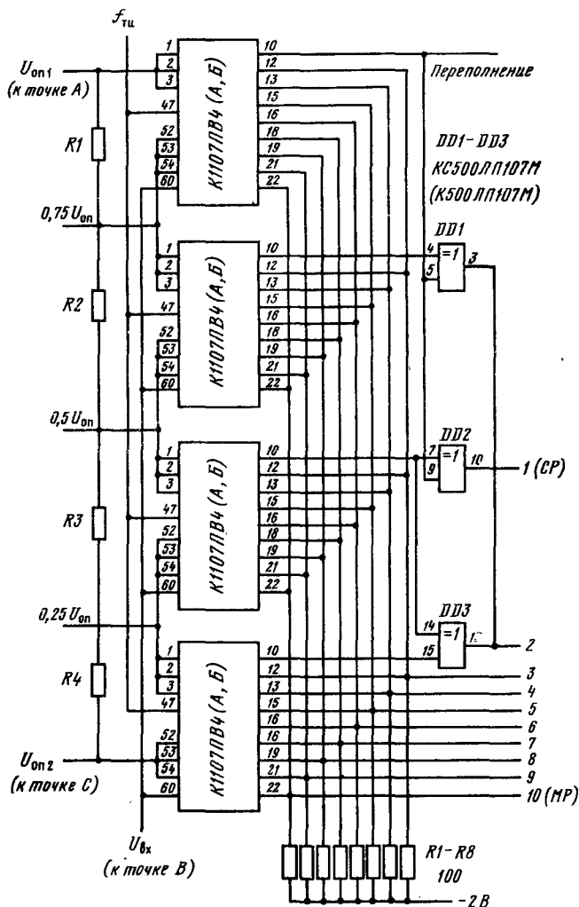
Схема включения входов и выходов четырех БИС К1107ПВ4 (А, Б) при увеличении числа разрядов АЦП до десяти. Точки подключения А, В, С указаны на типовой схеме включения
