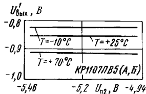
Типовые зависимости выходного напряжения высокого уровня от напряжения питания U_{п2} при различных температурах окружающей среды и U_{п1} = 5 В
