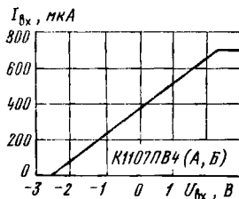
Типовая зависимость входного тока от входного напряжения АЦП К1107ПВ4 (А, Б)
