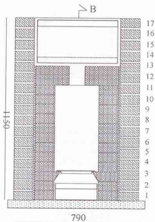
Сечение А
