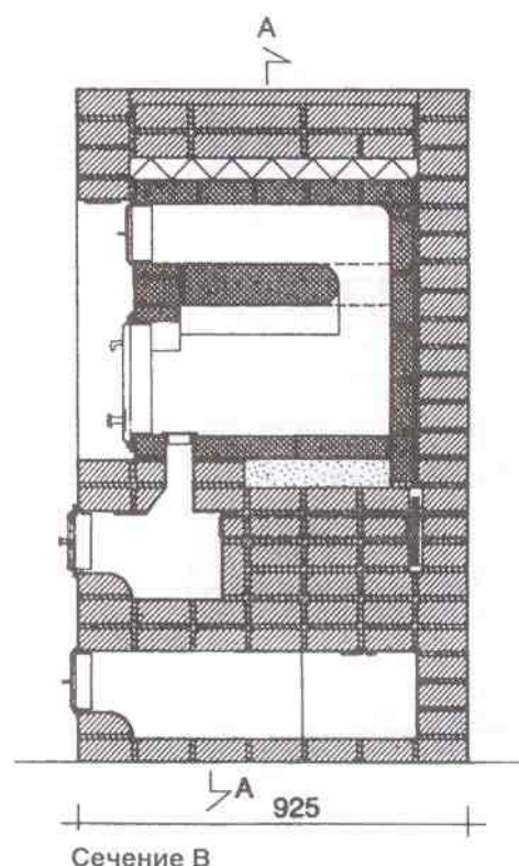
Сечение В
