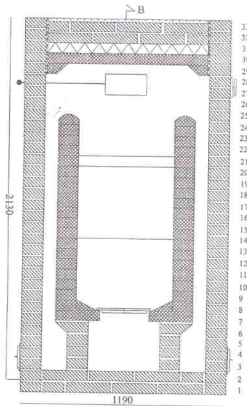
Сечение А
