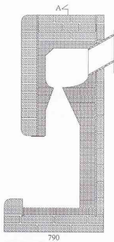
Сечение В
