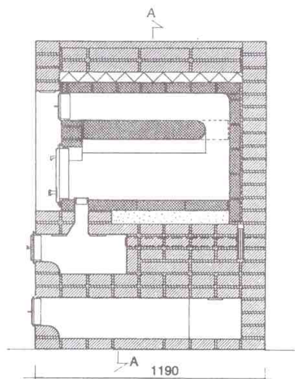
Сечение В
