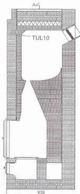
Сечение В
