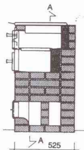
Сечение В
