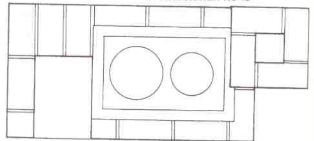
14-й ряд кладки
