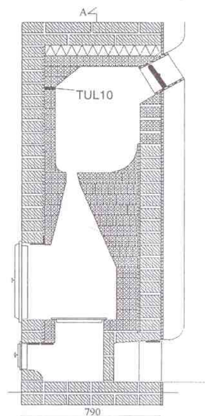
Сечение В
