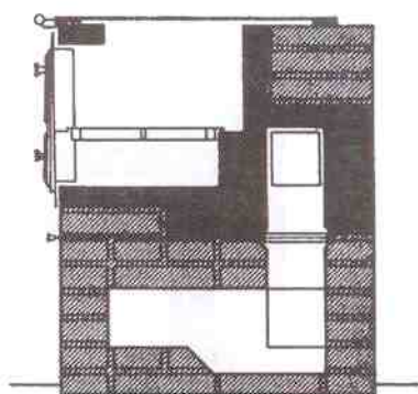
Сечение В1 - В1 (вариант)
