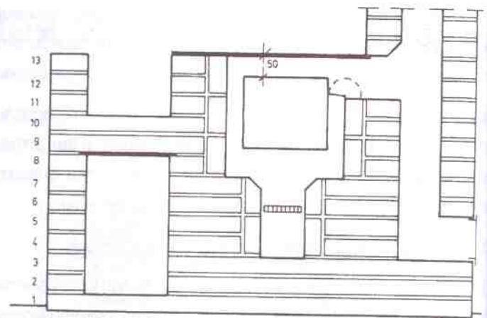
Продольный разрез 1060 Коптильная печь
