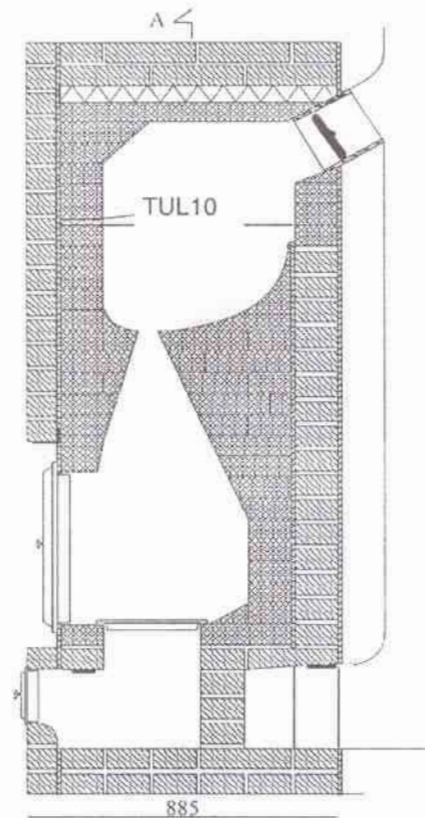
Сечение В
