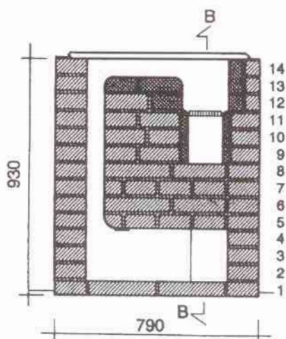
Сечение А
