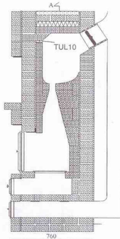
Сечение В
