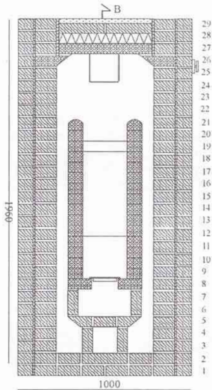
Сечение А
