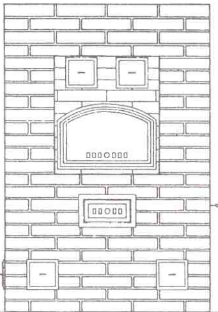
Хлебная печь, вид спереди
