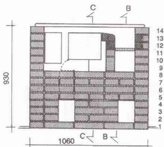
Плита, вид спереди
