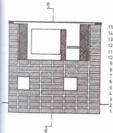
Сечение А
