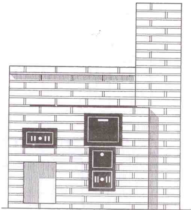
Вид спереди
