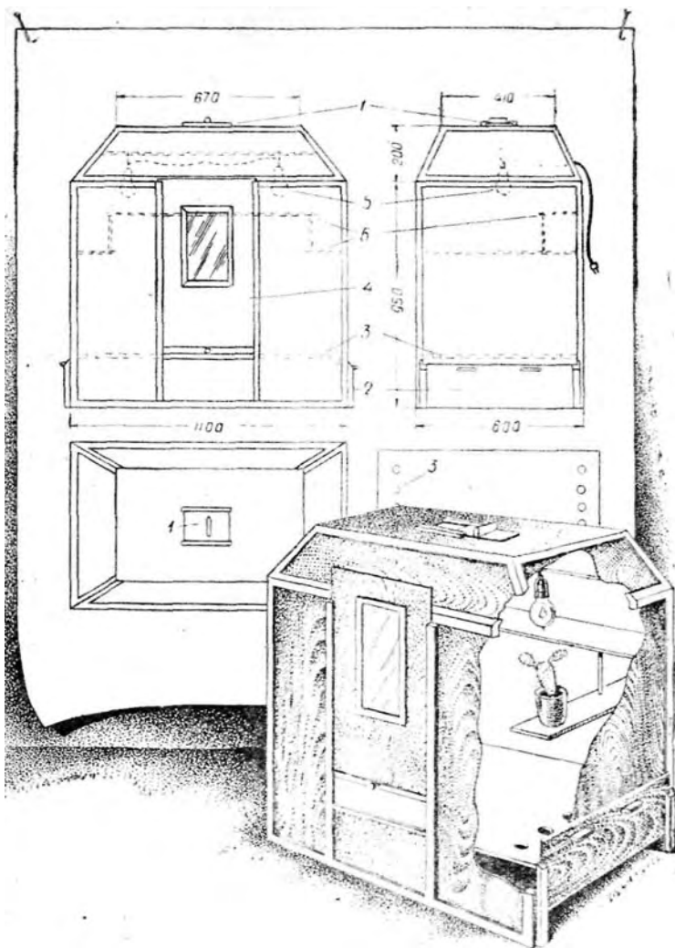
Электрокамера Н. М. Верзилина и ее чертеж с указанием размеров в миллиметрах:
