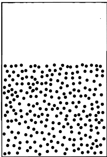
Рис. 2. Оседающий туман.
