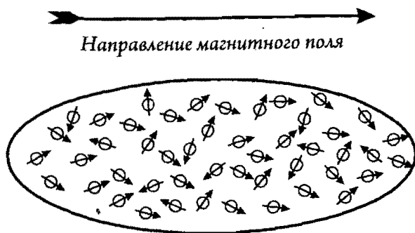
Рис. 1. Парамагнетизм.
