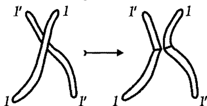
Рис. 6. Кроссинговер. Слева — две гомологичные хромосомы в контакте; справа — после обмена и разделения.
