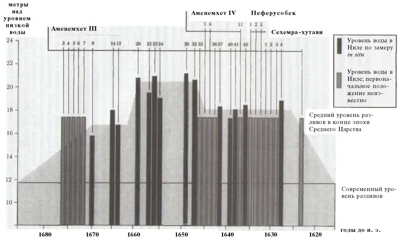
Диаграмма высоких разливов Нила с четко выраженным максимумом с 20 по 32 год правления Аменемхета III.
