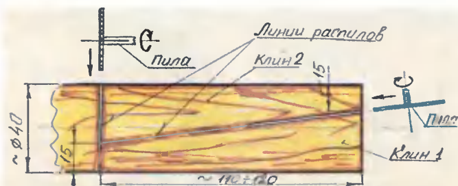
Рис. 2. Схема изготовления клинышков.
