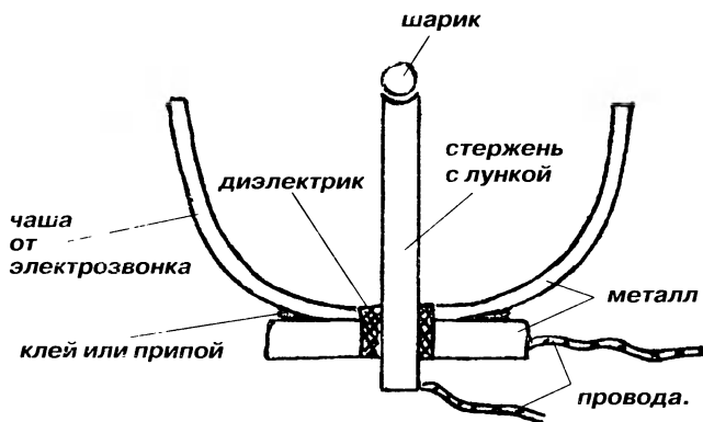
Рис. 1. Отпугивающее устройство.
