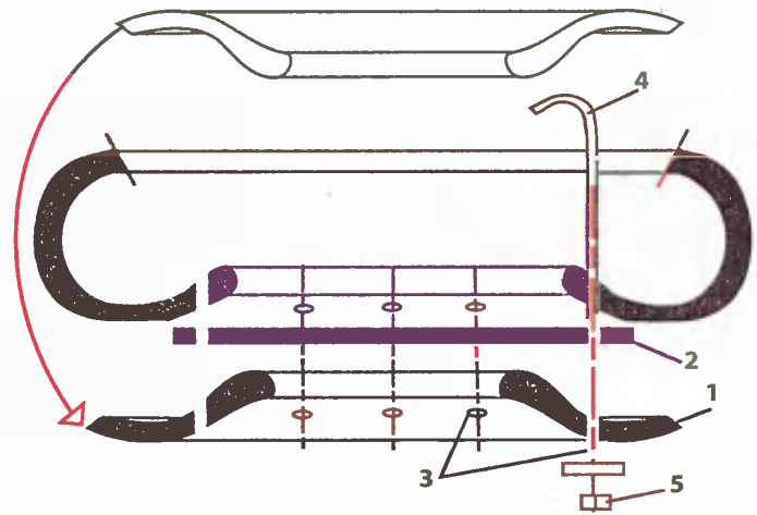
1 — вырезанная боковина, 2 — стальное днище, 3 — сквозные отверстия, 4 — болты М10, 5 — гайки с шайбами
