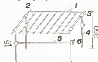
Рис. 1 Подставка для костра в рабочем положении
