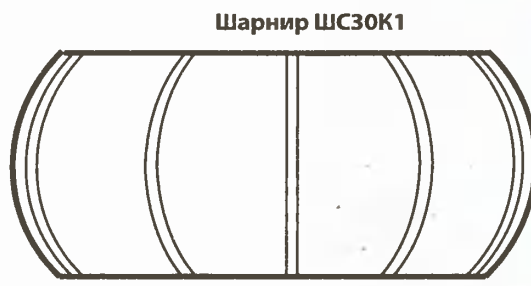
Шарнир ШС30К1 Внутренняя обойма Пазы 1,1 мм (6 шт.) через 60 градусов
