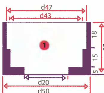
Рис. 1 Стакан
