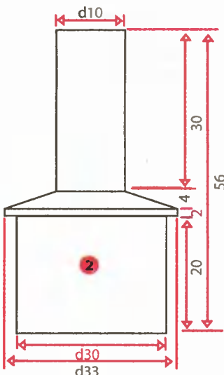
Рис. 2 Хвостовик
