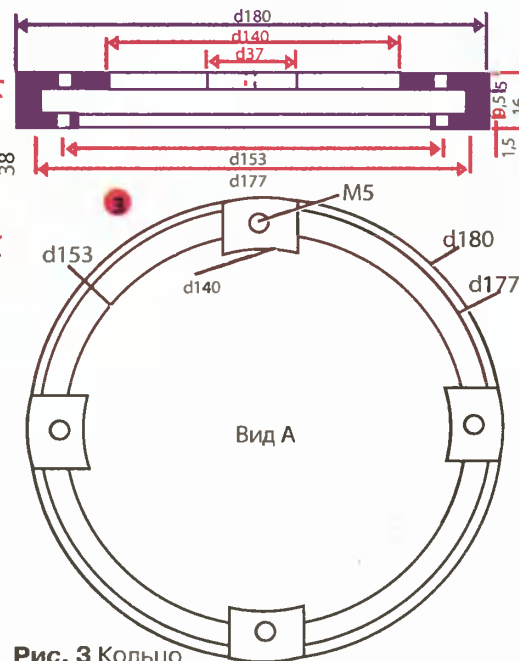
Рис. 3 Кольцо
