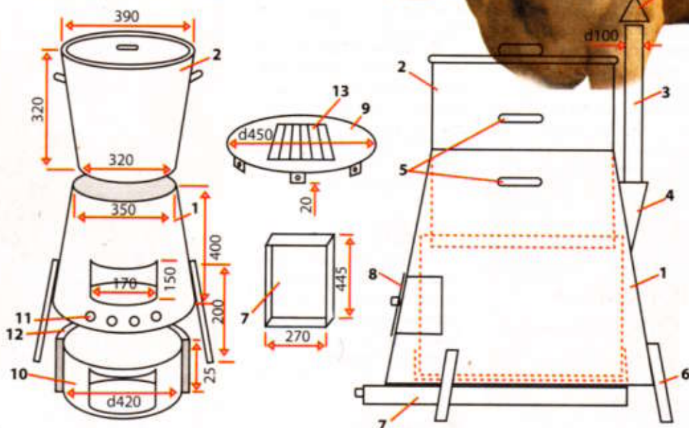
Общий вид печи 1 — кожух, 2 — бак, 3 — труба, 4 — карман с патрубком, 5 — ручки, 6 — ножки, 7 — зольник, 8 — дверка, 9 — поддон, 10 — вставка, 11 — отверстия поддувала, 12 — асбест, 13 — колосники, 14 — ветрогаситель
