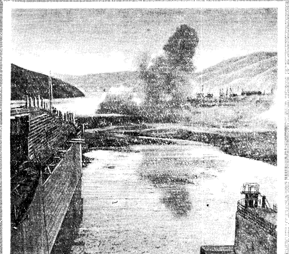
Строители Бухтарминской ГЭС одержали большую победу: в котловане первой очереди закончены работы по сооружению подводящей части водосливной плотины. Двадцать восьмого сентября 1957 года правобережный котлован был затоплен. На снимке вы видите, как при помощи взрывчатки разрушена нижняя стенка перемычки. Фото Г. Емельянова.
