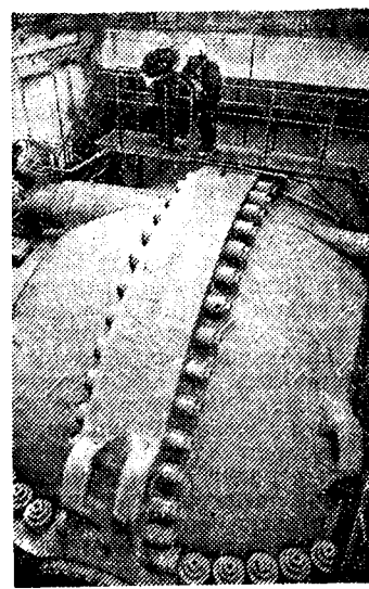
ТАДЖИКСКАЯ ССР. Около 11 миллионов киловатт-часов электроэнергии выработали с момента пуска шесть агрегатов Нурекской ГЭС. Шестой агрегат мощностью 300 тысяч киловатт недавно досрочно поставлен под промышленную нагрузку. На снимке: шаровый затвор шестого агрегата, который позволяет регулировать напор воды, поступающей на рабочее колесо турбины. Фото Р. НЕТЕЛЕВА. (ТАСС).
