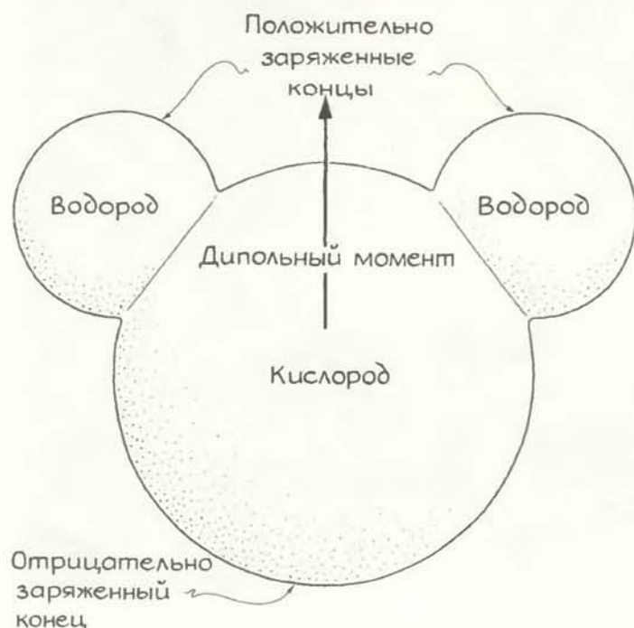
Молекула воды
