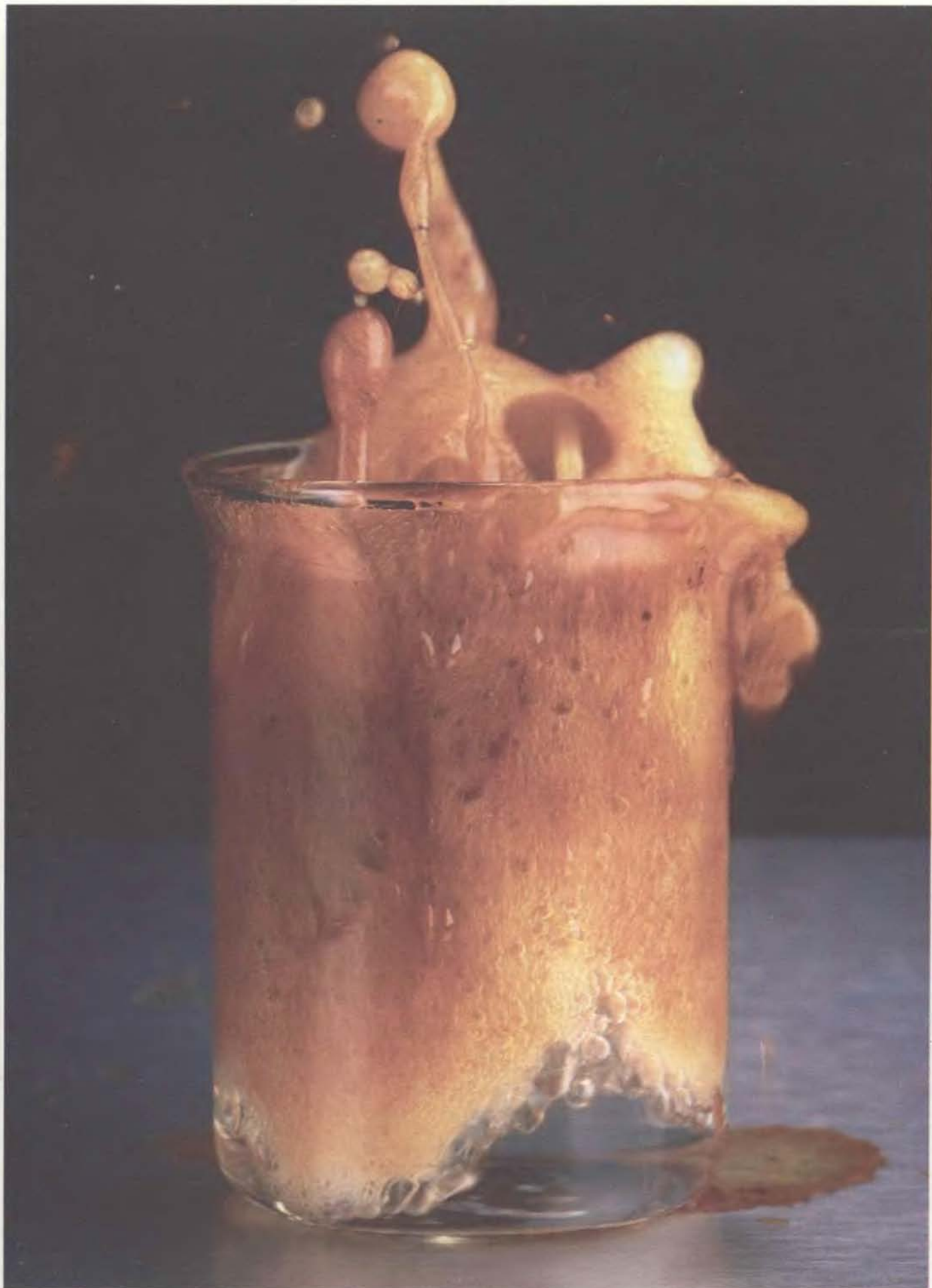
Порошок вызывает закипание перегретой воды в микроволновой печи
