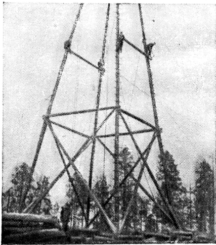
Постройка тригонометрической вышки (сигнала) геодезистами. Фото В. Зубакина.
