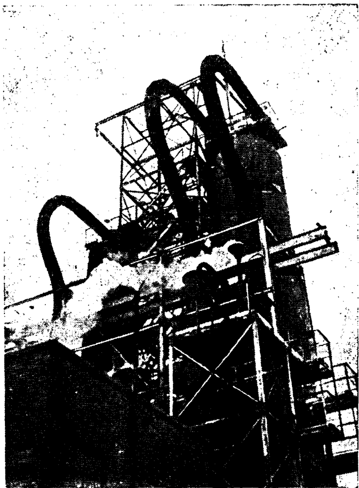
Трубочатка „Фостер-Биллер“ (Грозненский нефтеперерабатывающий завод)
