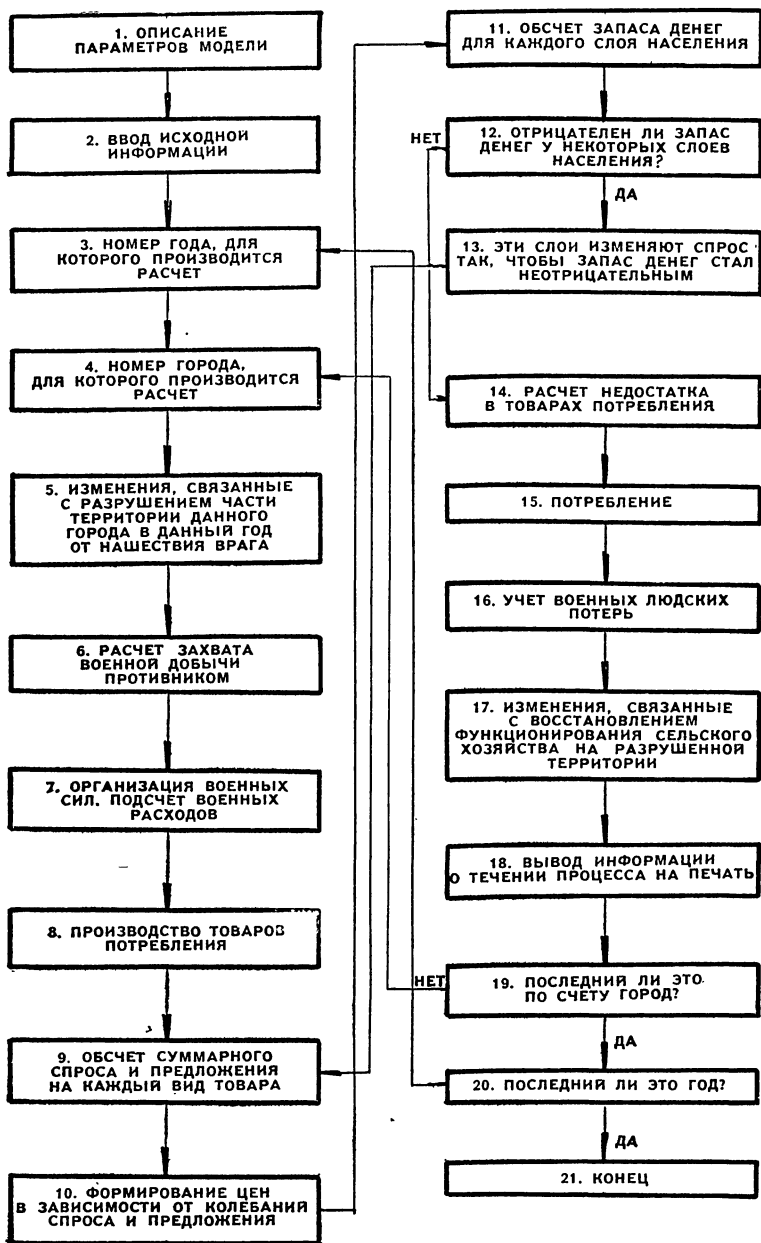
Рис. 2. Блок-схема вычислительного процесса
