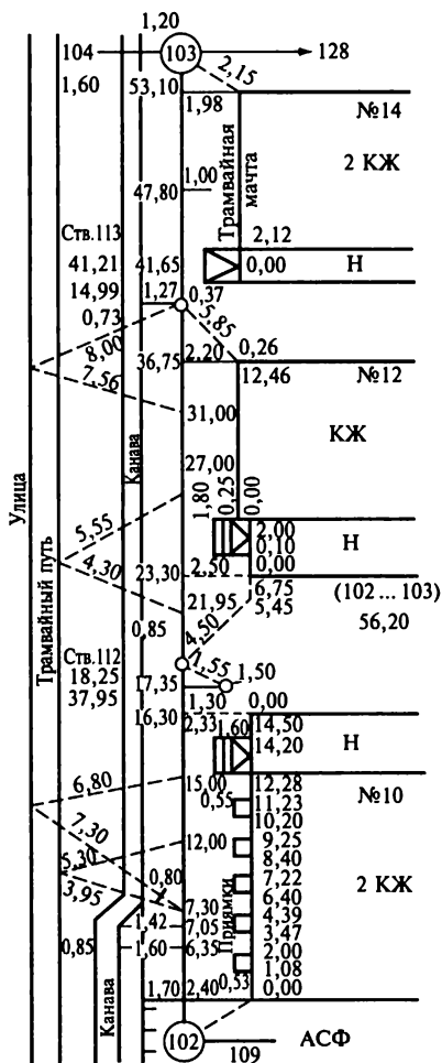
Рис. 11.1. Пример абриса
