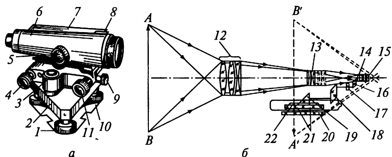
Рис. 7.6. Нивелир Н-3:
