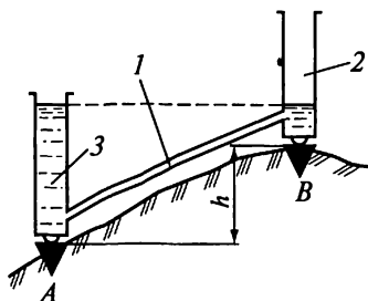
Рис. 7.13. Схема гидростатического нивелирования:
