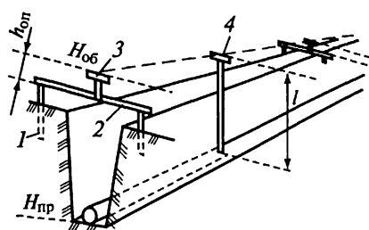
Рис. 19.1. Обноска для применения способа визирок при рытье траншей: 1 — деревянный столб; 2 — горизонтальная доска; 3 — опорная визирка; 4 — ходовая визирка
