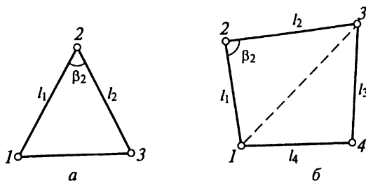
Рис. 23.1. Геометрические фигуры для определения площадей участков: а — треугольник; б — четырехугольник
