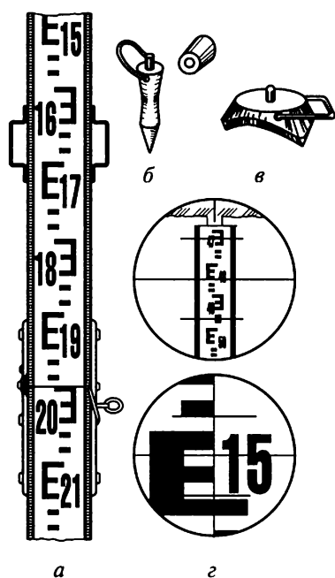
Рис. 7.8. Нивелирная рейка: а — внешний вид; б — костыль; в — башмак; з — отсчеты по рейке
