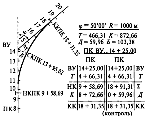
Рис. 25.4. Расчет пикетажа:
