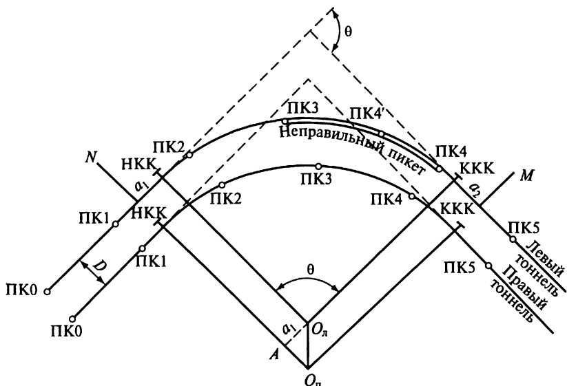
Рис. 27.4. Схемы расположения пунктов на кривых двухпутного тоннеля: НКК — начало круговой кривой; ККК — конец круговой кривой
