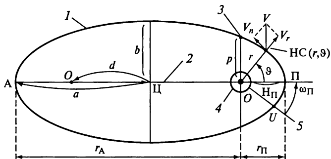
Рис. 14.11. Эллиптическая орбита спутника: 1 — эллиптическая орбита НС; 2 — линия апсид; 3 — НС ( r = p , \vartheta = 90^\circ ); 4 — Земля; 5 — линия узлов
