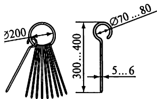
Рис. 6.4. Набор шпилек
