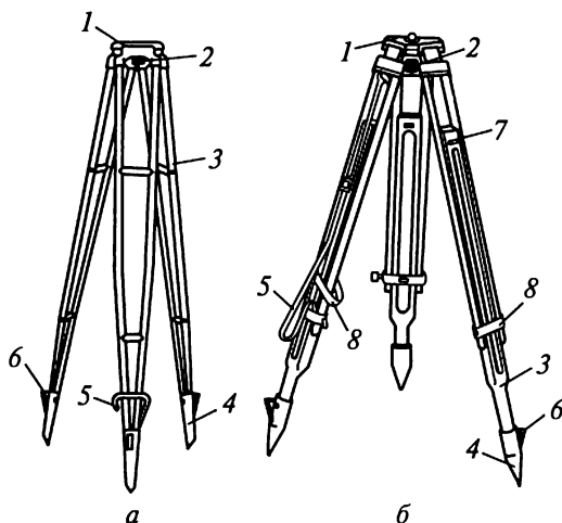
Рис. 8.7. Штанитивы:
