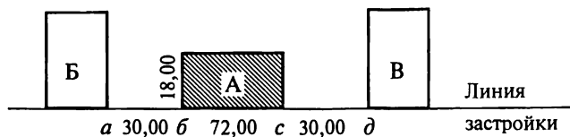
Рис. 17.3. Графический способ определения размещения здания для разбивки: a \dots d — углы зданий
