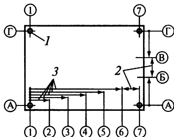
Рис. 20.22. Схема разбивки и контроля блочного здания: 1 — точка пересечения габаритных осей; 2 — расстояния, измеряемые для контроля; 3 — промежуточные оси
