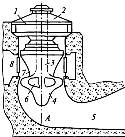
Рис. 26.6. Конструктивная схема гидроагрегата:
