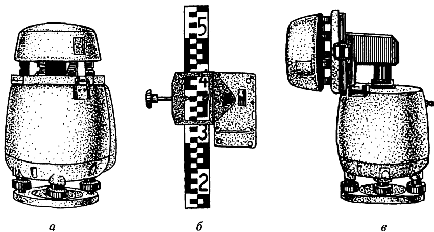
Рис. 9.1. Лазерный нивелир:
