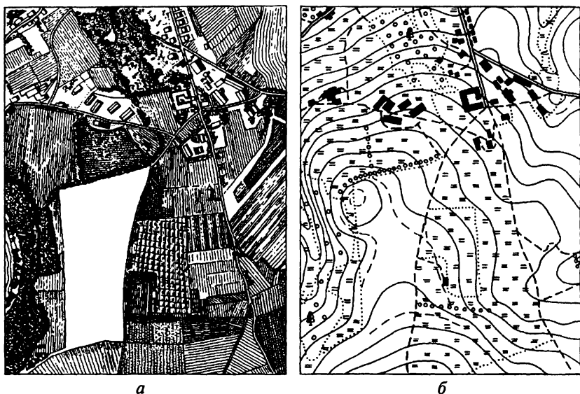
Рис. 11.6. Аэрофотографическое изображение местности ( a ) и составленный по нему план ( б )
