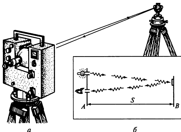
Рис. 6.10. Светодальномер:
