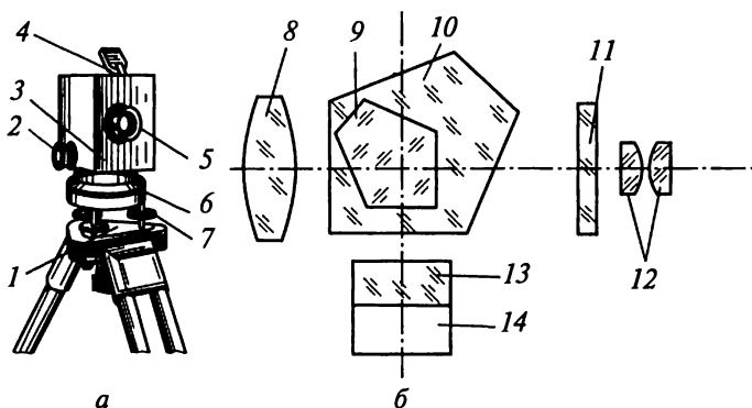
Рис. 7.5. Нивелир Н-10КП:
