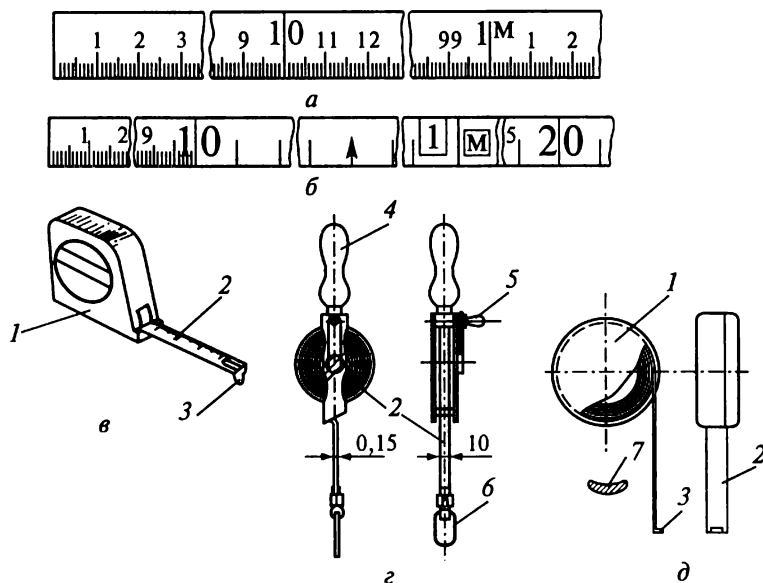
Рис. 6.1. Стальные рулетки:
