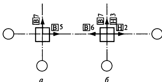
рис. 30.2. Примеры указания действительных отклонений осей элементов от разбивочных осей на плане для свай (а) и колонн (б)
