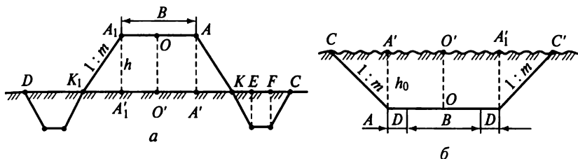
Рис. 25.12. Схемы разбивки дорожного полотна: а — для устройства земляного полотна на насыпи; б — в выемке
