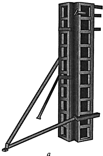
Рис. 20.25. Опалубка для колонн: a — установка опалубки колонн; б — расположение ориентирных рисок; 1 — ориентирные риски
