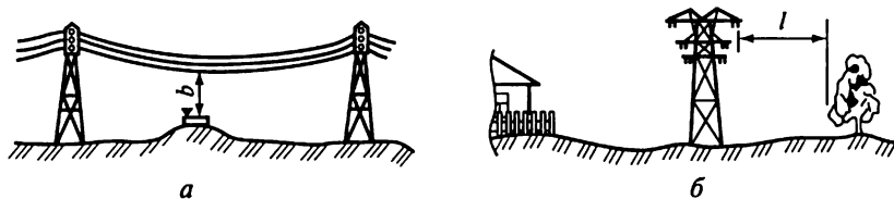
Рис. 29.1. Габаритные размеры приближения проводов: a — вертикальный; b — горизонтальный
