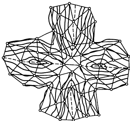
Рис. 4.5. Схема расположения точек цифровой модели в характерных местах рельефа и на горизонталях
