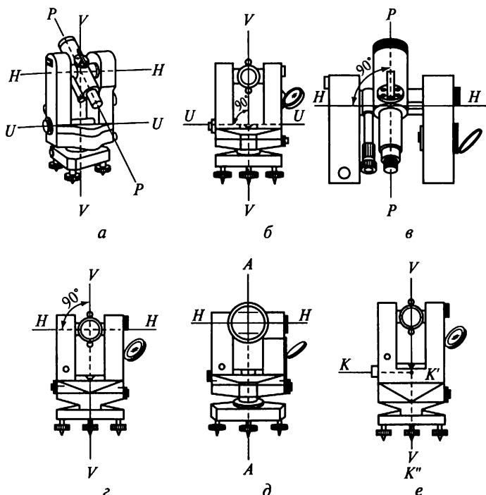
Рис. 8.11. Схемы (а...е) геометрических осей теодолита
