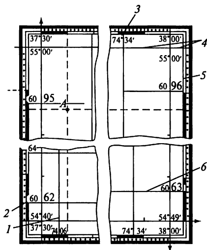
Рис. 3.5. Определение координат точки на топографическом плане: 1 — вертикальная километровая линия; 2 — цифровые обозначения горизонтальных линий координатной сетки; 3 — цифровые обозначения вертикальных линий координатной сетки; 4 — внутренняя рамка; 5 — рамка с минутами; 6 — горизонтальная километровая линия
