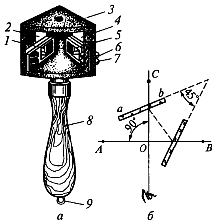
Рис. 8.10. Двухзеркальный ЭГ: а — внешний вид; б — построение прямого угла эккером над точкой O ; 1, 5 — зеркала; 2, 4 — окна; 3 — корпус; 6, 7 — винты; 8 — ручка; 9 — кольцо
