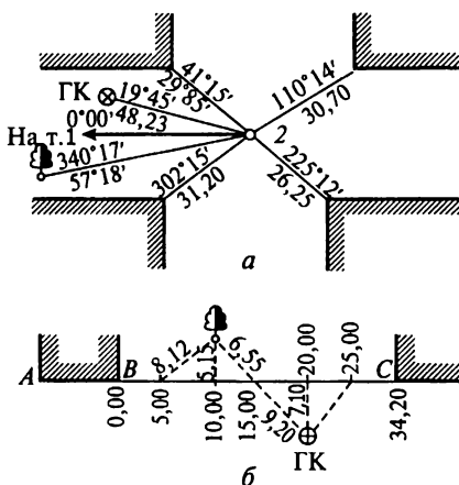
Рис. 11.2. Абрисы съемок, выполненных способами полярных координат (а) и створным (б)
