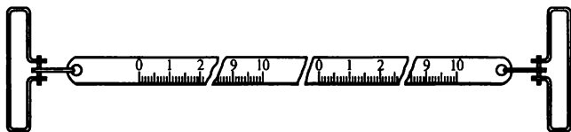
Рис. 6.3. Землемерная лента шкаловая
