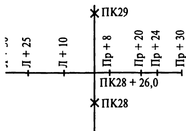
рис. 25.5. Разбивка поперечного профиля трассы
