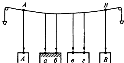
Рис. 22.1. Схема струнного способа установки конструкций
