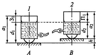
Рис. 22.7. Схема определения превышения при помощи гидростатической системы:
