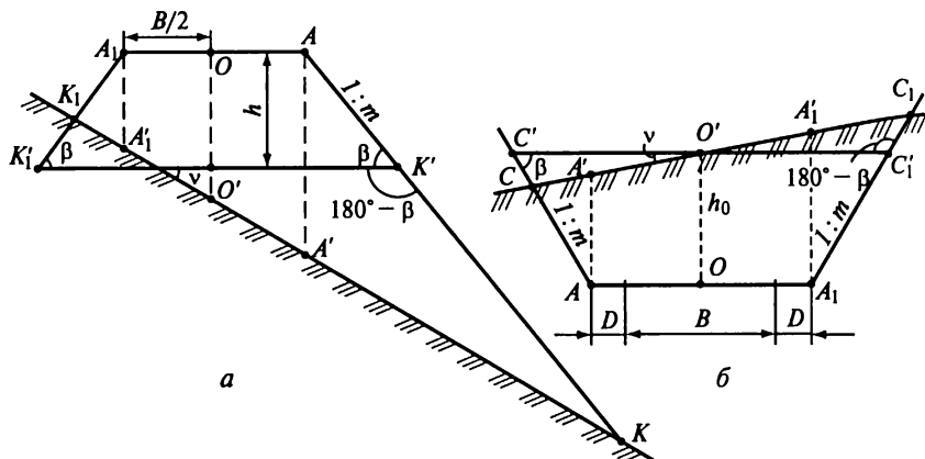
Рис. 25.13. Схемы разбивки дорожного полотна на косогоре: а — для поперечного профиля в насыпи; б — в выемке
