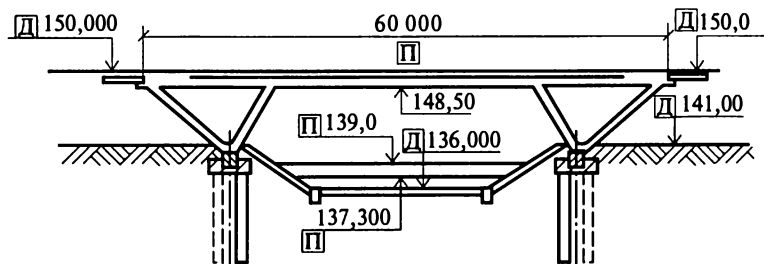
рис. 30.1. Обозначение действительных \Delta и проектных \Pi отметок на фасаде продольного профиля мостового перехода
