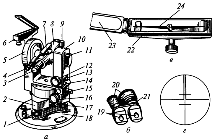
Рис. 8.5. Теодолит 3Т30:
