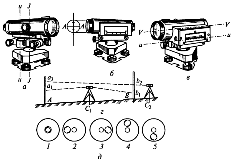
Рис. 7.14. Поверка нивелира:
