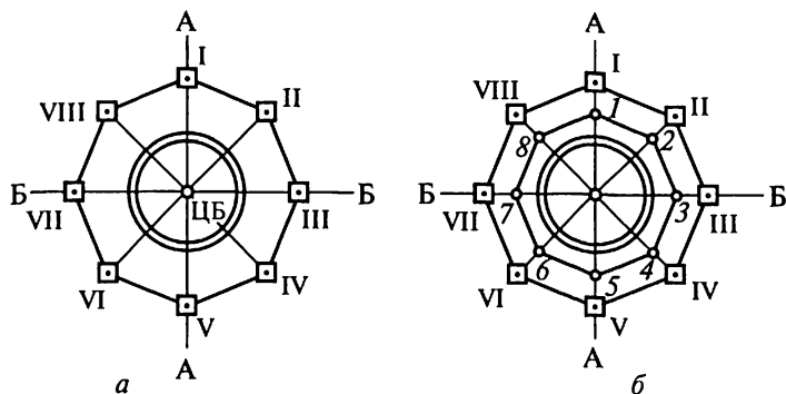
Рис. 21.7. Схемы опорной сети для строительства башенных сооружений: а — равномерное расположение пунктов на одной окружности; б — концентрическое расположение пунктов; 1...8 — ближние пункты; I...VIII — дальние пункты
