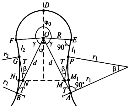
Рис. 25.10. Симметричная серпантина
