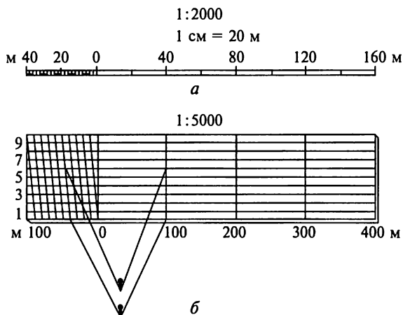
Рис. 1.8. Графические масштабы: а — линейный; б — поперечный
