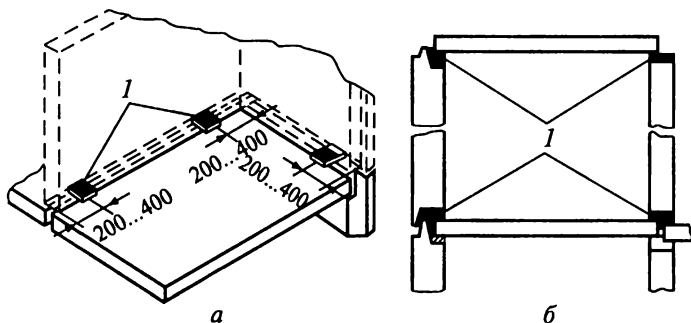
Рис. 20.13. Выравнивание монтажного горизонта: а — установка маяков под панели; б — выравнивание стен и перекрытий; 1 — маяки
