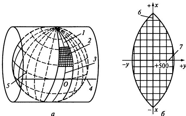
Рис. 3.3. Равноугольное проецирование:
