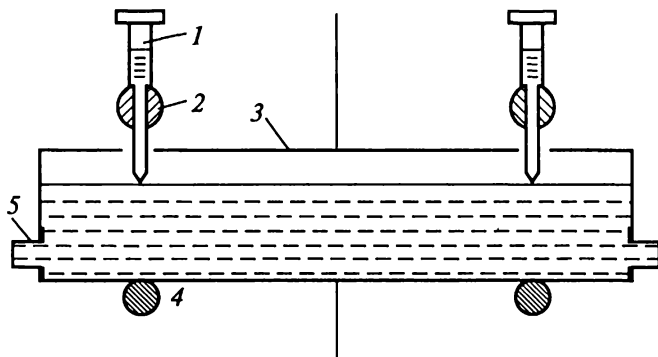
Рис. 24.4. Стационарная гидростатическая система: 1 — измеритель; 2 — марка; 3 — отрезок металлической трубы; 4 — стержень; 5 — шланг
