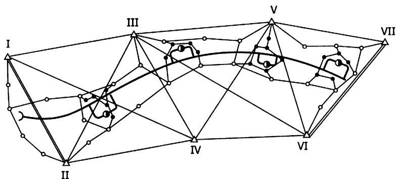
Рис. 27.9. Схема планового геодезического обоснования тоннеля: \Delta — тоннельная триангуляция; \circ — основная полигонометрия; \bullet — переходная полигонометрия; \bigcirc — ствол шахты; \sim — трасса тоннеля
