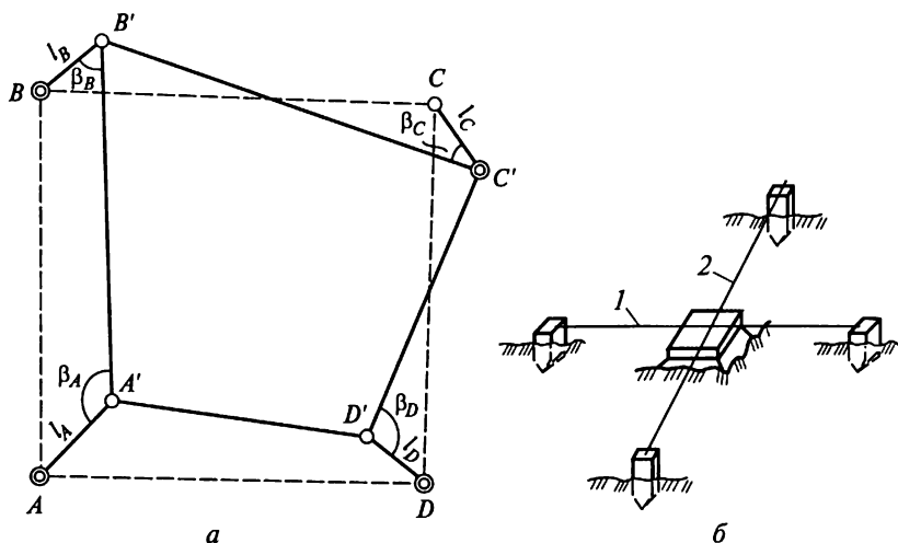
Рис. 13.7. Редуцирование пунктов строительной сетки: а — схема редуцирования; б — закрепление пункта постоянным знаком; 1, 2 — створы
