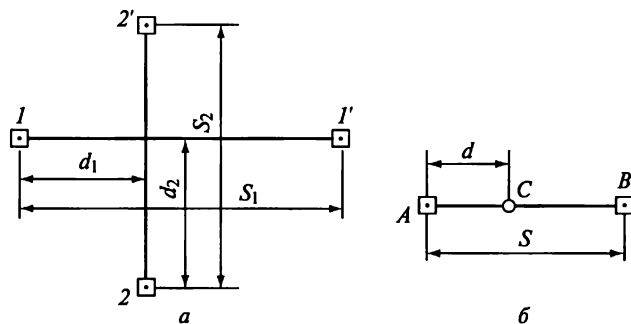
Рис. 16.5. Схемы разбивки способами: a — створной засечки; б — створно-линейной засечки
