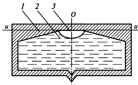
Рис. 7.3. Круглый уровень: 1 — ампула; 2 — жидкость; 3 — пузырек
