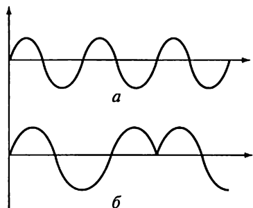
Рис. 14.5. Импульсно-фазовая модуляция:
