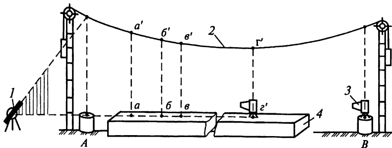
Рис. 22.2. Схема струнно-оптического способа установки конструкций: 1 — теодолит; 2 — струна; 3 — прибор вертикального проектирования; 4 — оборудование
