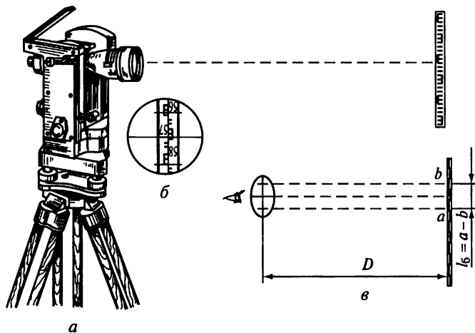
Рис. 6.8. Оптический дальномер: а — внешний вид; б — поле зрения трубы; в — схема измерения
