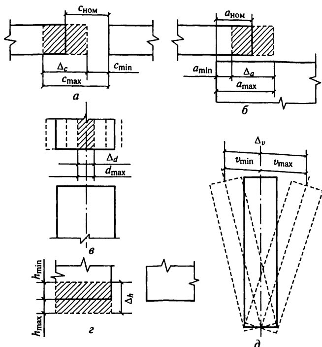
Рис. 22.12. Основные виды функциональных параметров: a — зазор между элементами c_{\text{ном}} ; б — длина опирания элемента a_{\text{ном}} ; в — несоосность элементов d ; г — несовпадение поверхностей элементов h ; д — неперпендикулярность v
