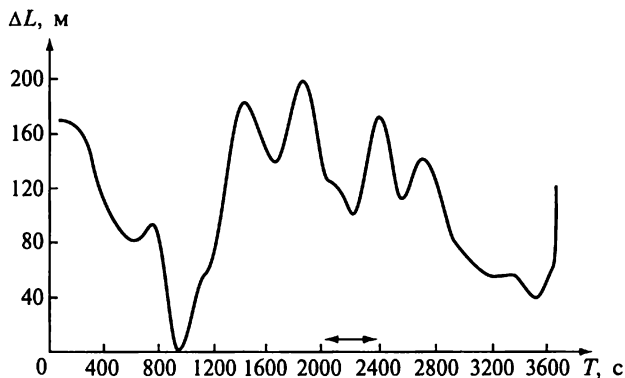
Рис. 14.16. Влияние искажения сигналов
