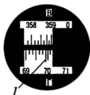
Рис. 8.6. Поле зрения отсчетного микроскопа теодолита 3Т30:
