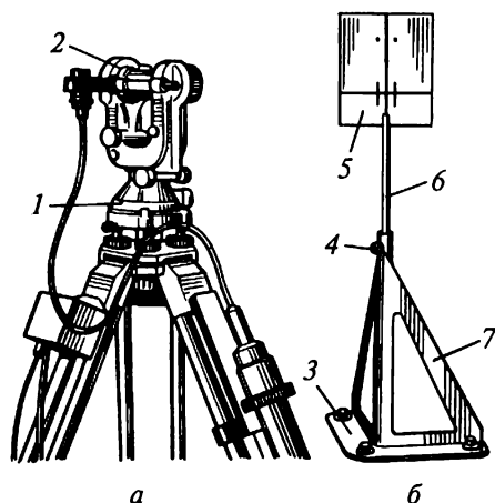
Рис. 9.2. Лазерный теодолит (а) и визирная марка (б): 1, 2 — горизонтальный и вертикальный круги; 3 — опора; 4 — закрепительный винт; 5 — марка; 6 — стержень; 7 — стойка
