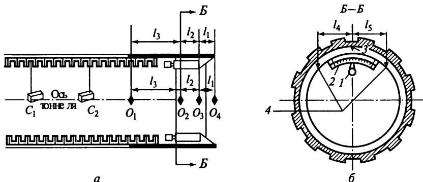
Рис. 27.14. Геодезическое обеспечение щитовой проходки:
