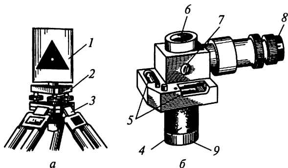
Рис. 8.8. Элементы установки визирных целей:
