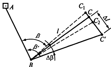
Рис. 15.2. Схема построения в натуре проектного угла
