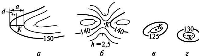
Рис. 4.8. Определение отметок точек по горизонталям: a \dots z — схемы при высоте сечения h = 2,5 м
