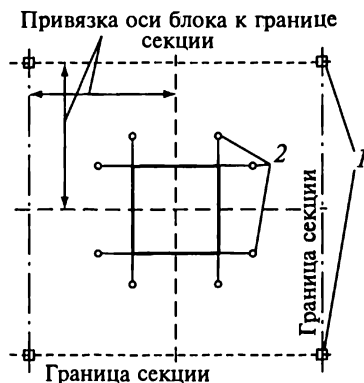
Рис. 26.5. Схема разбивки осей блока плотины: 1 — угловые знаки; 2 — знаки выноски
