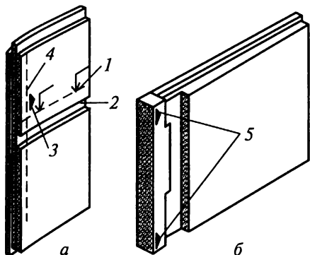
Рис. 20.19. Разметка панелей:
