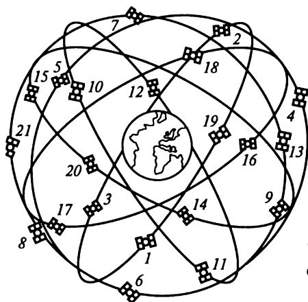
Рис. 14.2. Спутниковая навига- ионная система NAVSTAR GPS: 1...21 — номера спутников
