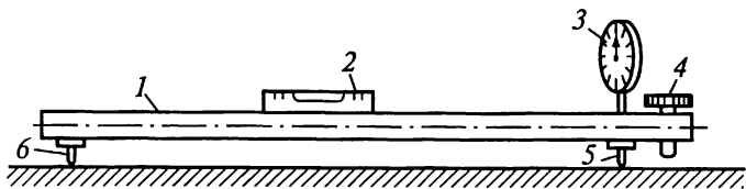
Рис. 22.6. Конструктивная схема микронивелира:
