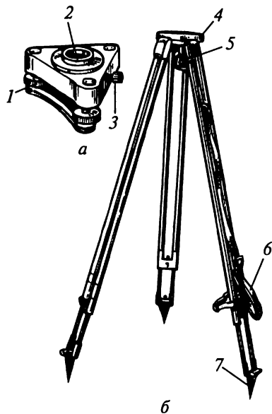
Рис. 7.4. Установка и крепление геодезических приборов: a — подставка; б — штатив; 1, 3, 5 — винты; 2 — отверстие для уста- новки прибора; 4 — столик; 6 — ремень, 7 — наконечник
