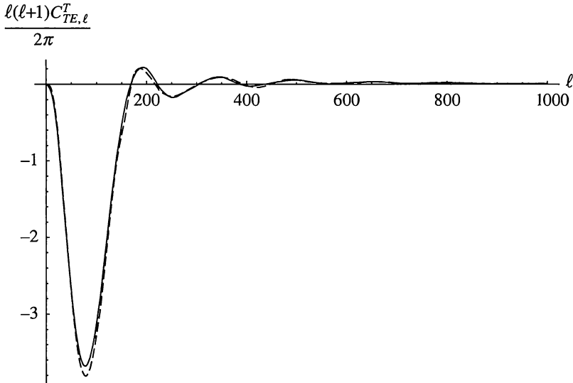
Рис. 7.8. Зависимость мультипольного коэффициента \ell(\ell+1)C_{TE,\ell}^T/(2\pi) , выраженного в квадратных микрокельвинах, от \ell , сноска 55. Сплошная кривая берется на основе точной формулы (7.4.65); пунктирная кривая описывает приближение (7.4.72). В обоих случаях метод вычисления гравитационной амплитуды и функции источника, а также предполагаемых космологических параметров описан в разд. 7.3
