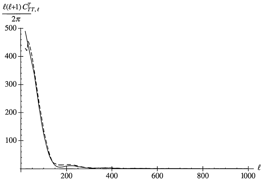
Рис. 7.3. Зависимость тензорного «температура-температура» мультипольного коэффициента \ell(\ell+1)C_{TT,\ell}^T/(2\pi) , выраженного в квадратных микрокельвинах, от \ell из сноски 30. Непрерывная кривая является результатом использования точной формулы (7.3.18); пунктирная кривая описывает результат приближения больших \ell (7.3.25). Используемые в этих вычислениях космологические параметры описываются в тексте
