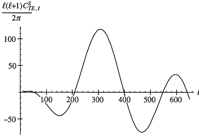
Рис. 7.5. Зависимость мультипольного коэффициента \ell(\ell+1)C_{TE,\ell}^{(S)}/(2\pi) , выраженного в квадратных микрокельвинах, от \ell при космологических параметрах, заданных в (7.2.44) и (7.2.45)
