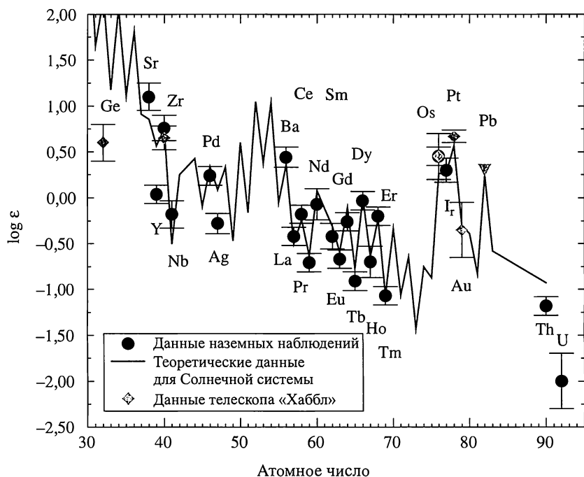
Рис. 1.5. Данные о распространенности порожденных \gamma -процессом элементов для звезды BD+17° 3248, которые получены посредством спектроскопических наблюдений, выполненных наземными обсерваториями и телескопом «Хаббл». Для сравнения сплошной линией показаны теоретические значения исходной распространенности, опирающиеся на данные по Солнечной системе. Обратите внимание на то, что наблюдаемые значения распространенности для тория и урана заметно ниже теоретических значений для исходной распространенности. Это указывает на возраст звезды BD+17° 3248, равный 13,8 \pm 4 млрд лет. (Из J. J. Cowan et al., Astrophys. J. 572 , 861 (2002) [astro-ph/0202429])
