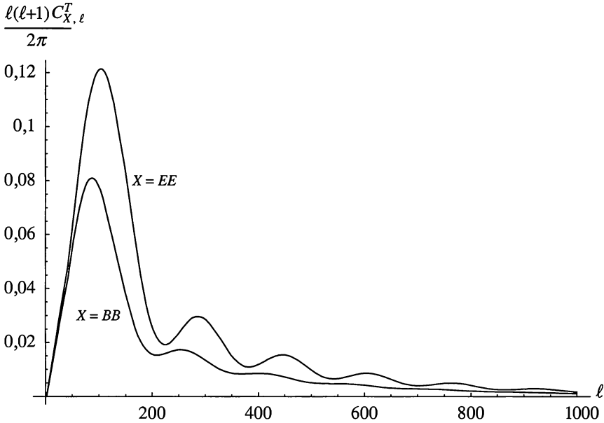
Рис. 7.7. Зависимость мультипольных коэффициентов \ell(\ell+1)C_{EE,\ell}^T/(2\pi) и \ell(\ell+1)C_{BB,\ell}^T/(2\pi) , выраженных в квадратных микрокельвинах, от \ell при космологических параметрах, заданных в разд. 7.2 (см. также сноску 55). Эти результаты согласуются с точностью до 1 % с результатами, полученными (при таких же космологических параметрах) при использовании компьютерных программ CMBfast и CAMB, в которых вместо использования интегрального уравнения (7.3.22), как это сделано здесь, система уравнений Больцмана усечена на максимальном значении \ell . (Результаты двух компьютерных программ отличаются друг от друга примерно с той же точностью)
