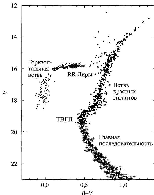
Рис. 1.6. Диаграмма «цвет — звездная величина» для шарового скопления М15. Визуально наблюдаемая видимая звездная величина звезд скопления М15 отложена на вертикальной оси. Поскольку все звезды этого скопления находятся примерно на одном расстоянии от Земли, видимая визуальная звездная величина отличается от абсолютной звездной величины на некоторое постоянное значение при нарастающей при движении вверх абсолютной светимости. Разница между видимой голубой и визуальной звездными величинами отложена на горизонтальной оси. Это служит мерой поверхностной температуры, которая спадает при движении вправо. Если бы скопление М15 было молодым, главная последовательность уходила бы вверх и влево; положение точки выключения главной последовательности (ТВГП) и другие характеристики этой диаграммы указывают на то, что возраст скопления составляет 15 \pm 3 млрд лет. Диаграмма взята из В. Chaboyer, Phys. Rep. 307 , 23 (1998) и опирается на данные из работы Р. R. Durrell and W. E. Harris, Astron. J. 105 , 1420 (1993) [astro-ph/9808200]
