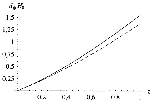
Рис. 1.3. Зависимость фотометрического расстояния от красного смещения для двух космологических моделей. Верхняя сплошная кривая соответствует случаю \Omega_\Lambda = 0,7 , \Omega_m = 0,3 , \Omega_K = \Omega_\Lambda = 0 ; нижняя пунктирная линия отвечает модели пустой Вселенной, в которой \Omega_K = 1 , \Omega_\Lambda = \Omega_m = \Omega_\Lambda = 0 . По вертикали отложено фотометрическое расстояние, умноженное на постоянную Хаббла
