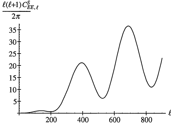
Рис. 7.4. Зависимость мультипольного коэффициента \ell(\ell+1)C_{EE,\ell}^{(S)}/(2\pi) , выраженного в квадратных микрокельвинах, от \ell при космологических параметрах, заданных в (7.2.44) и (7.2.45)
