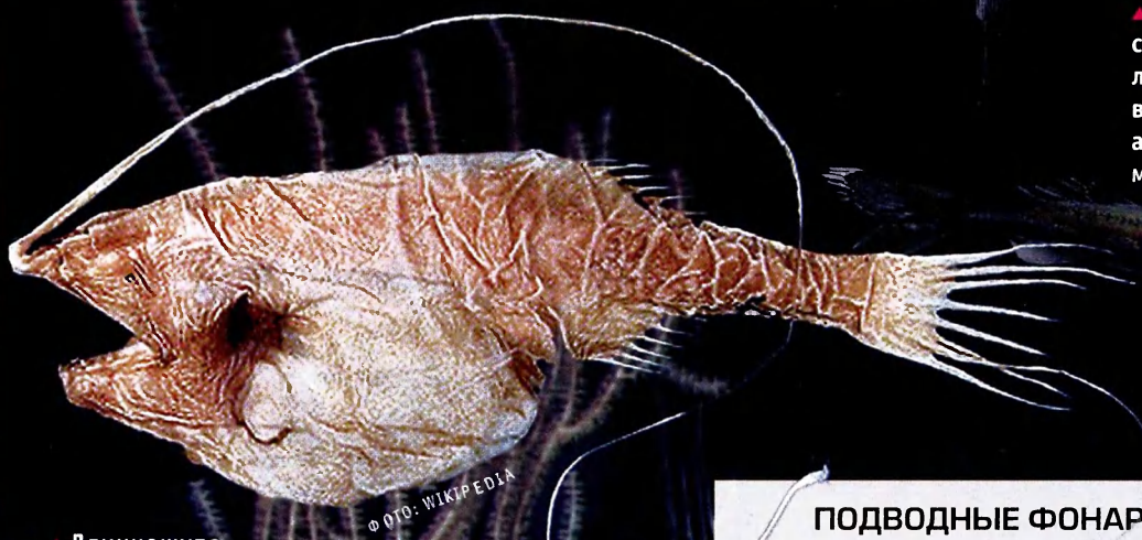
▲ Длиннощуповый удильщик.
