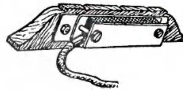
Рис. 3. Крепление электромагнитного звукоснимателя на подставке балалайки или домры.
