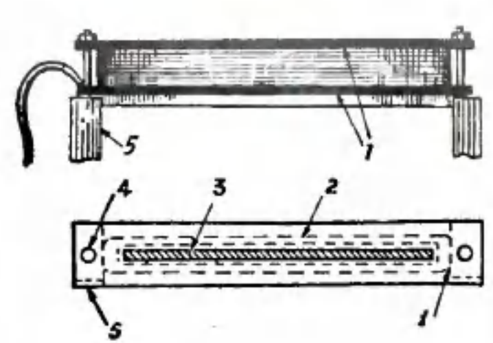
Рис. 4. Разрез электромагнитного звукоснимателя и крепление собранного звукоснимателя на подставке под струнами: 1 — железные планки; 2 — обмотка катушки; 3 — прямоугольный магнит; 4 — отверстия для стяжных болтов; 5 — алюминиевые лапки для крепления звукоснимателя к подставке.
