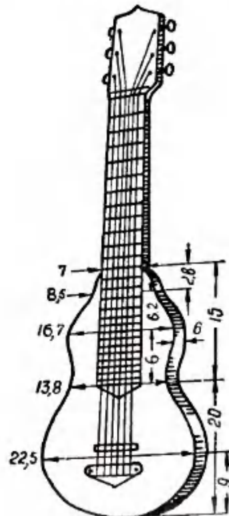
Рис. 1. Корпус «немой» гавайской гитары.
