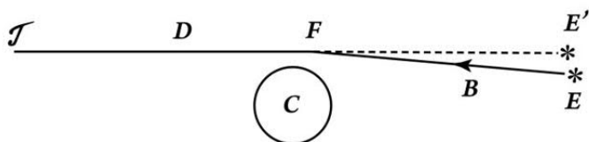
Рис. 56. Одно из следствий общей теории относительности — отклонение световых лучей под влиянием силы тяготения Солнца. Согласно теории относительности земной наблюдатель в T видит звезду в точке E' по направлению прямой TDFE' , между тем как в действительности звезда находится в точке E и посылает свои лучи по искривленному пути EBFDT . При отсутствии Солнца световой луч от звезды E к Земле T направлялся бы по прямой линии
