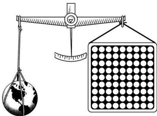
Рис. 89. Земля «весит» в 81 раз больше Луны
