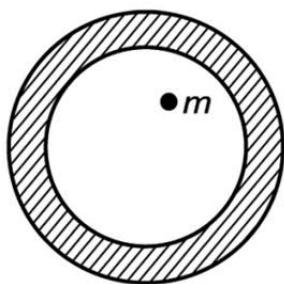
Рис. 91. Тело внутри шаровой оболочки не имеет веса
