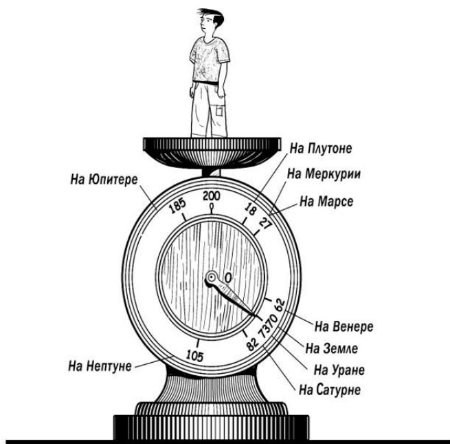
Рис. 90. Сколько весил бы человек на разных планетах. Вес человека на Плуtone — не 18 кг, а всего лишь 3,6 кг (по современным данным)
