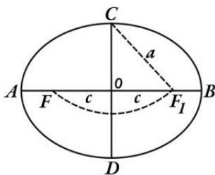
Рис. 18. Как разыскать фокусы эллипса
