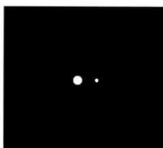
Марс в наибольшей близости и в наибольшем удалении
