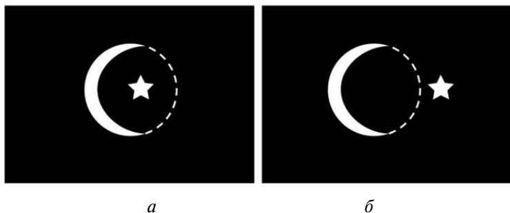
Рис. 31. Почему звезда не может быть видна между рогами месяца
