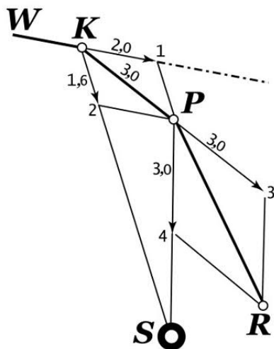
Рис. 84. Как Солнце S искривляет путь планеты WKPR
