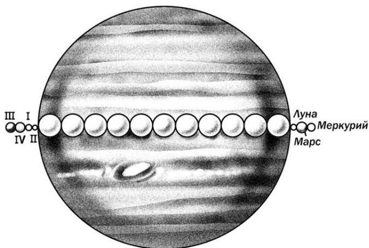
Рис. 65. Размеры Юпитера и его спутников (слева) по сравнению с размерами Земли (вдоль диаметра), Луны, Марса и Меркурия (справа)
