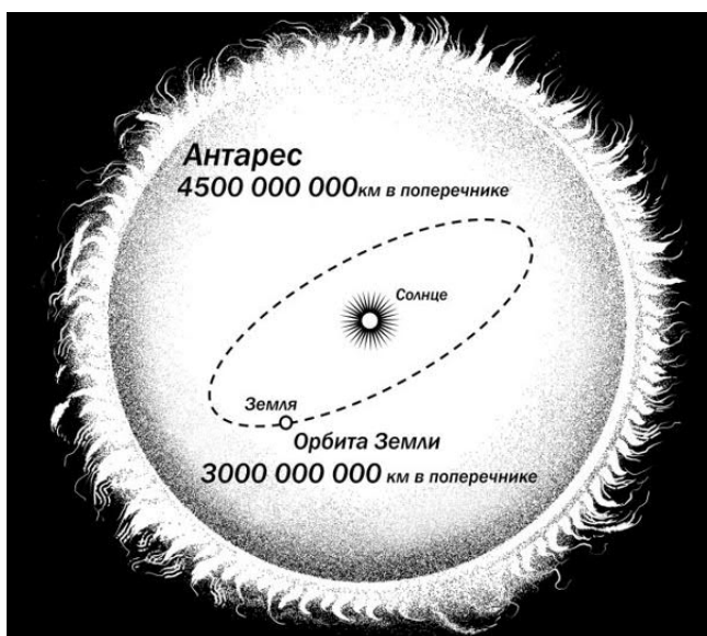
Рис. 73. Звезда-гигант Антарес ( \alpha Скорпиона) могла бы включить в себя наше Солнце с земной орбитой
