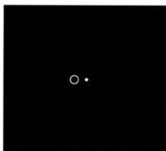
Меркурий в наибольшей близости (невидим) и в наибольшем удалении
