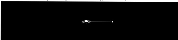
Сатурн с крупнейшим спутником
