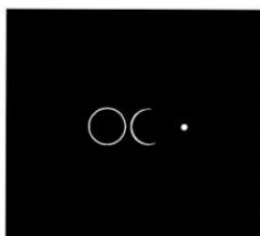
Венера в наибольшей близости (невидима), наибольший видимый серп, в наибольшем удалении
