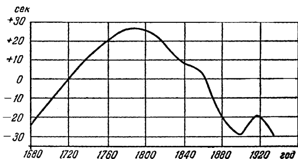
Рис. 29. Кривая поправок, которые надо прибавить к моментам среднего времени, чтобы скомпенсировать влияние колебаний вращения Земли (по Спенсеру Джонсу). Подъемы кривой соответствуют удлинению суток, т.е. замедлению вращения Земли; понижения — ускорению вращения
