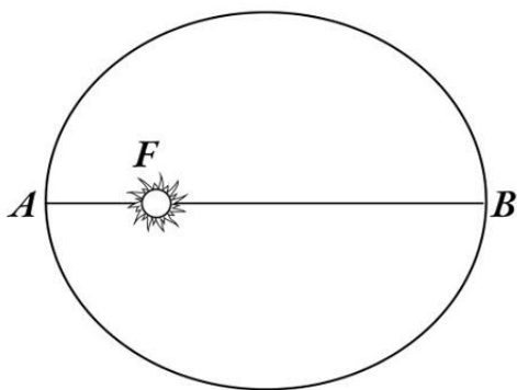
Рис. 19. Какую форму имела бы орбита Земли, если бы эксцентриситет земной орбиты был равен 0,5. В фокусе F — Солнце
