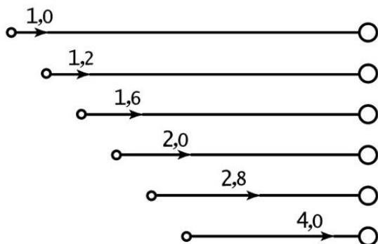
Рис. 83. Сила притяжения планеты Солнцем увеличивается с уменьшением расстояния
