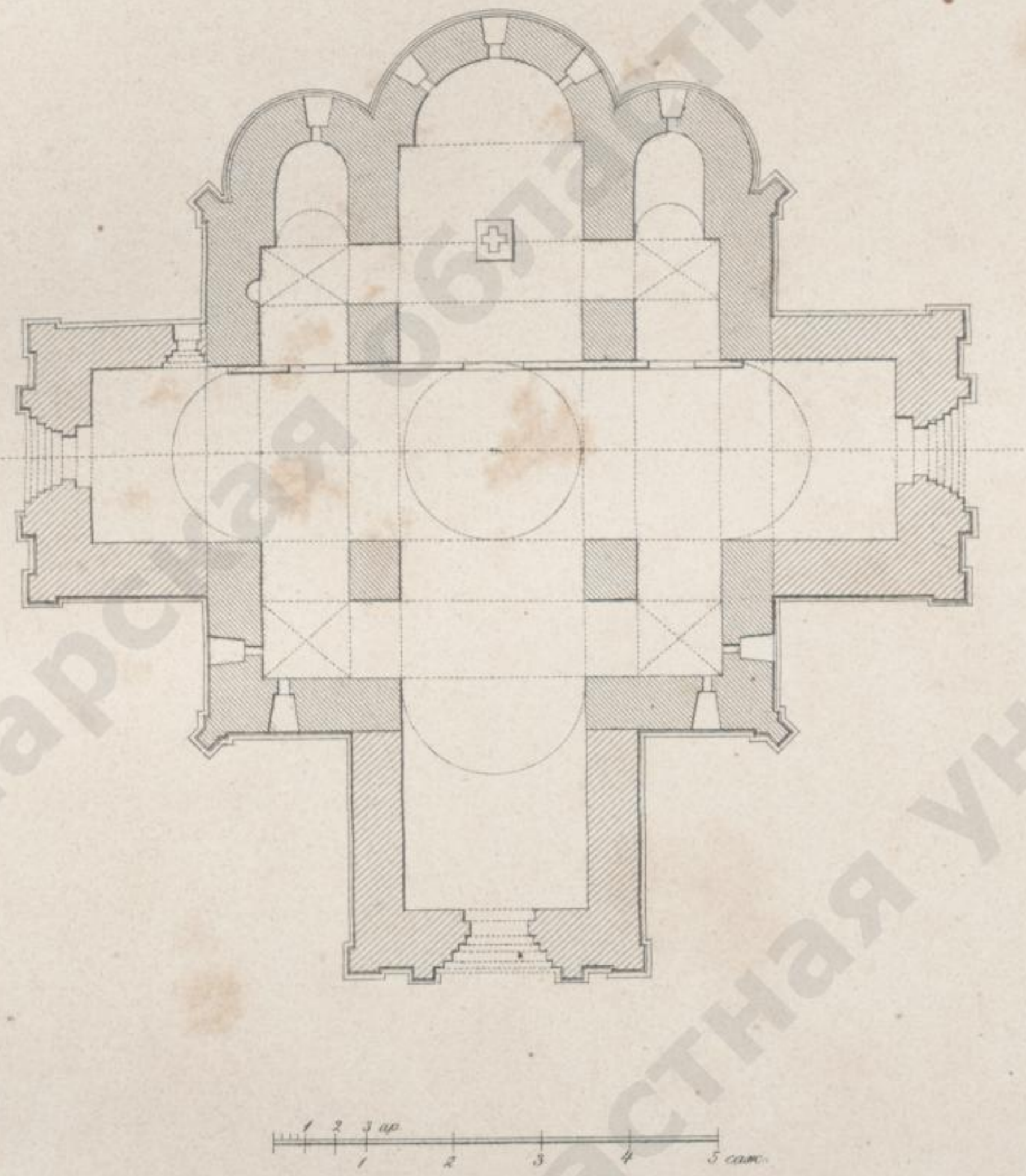
ПЛАНЪ ЦЕРКВИ ПРЕОБРАЖЕНІЯ ВЪ ПЕРЕСЛАВѢ ЗАЛЪССКОМЪ
