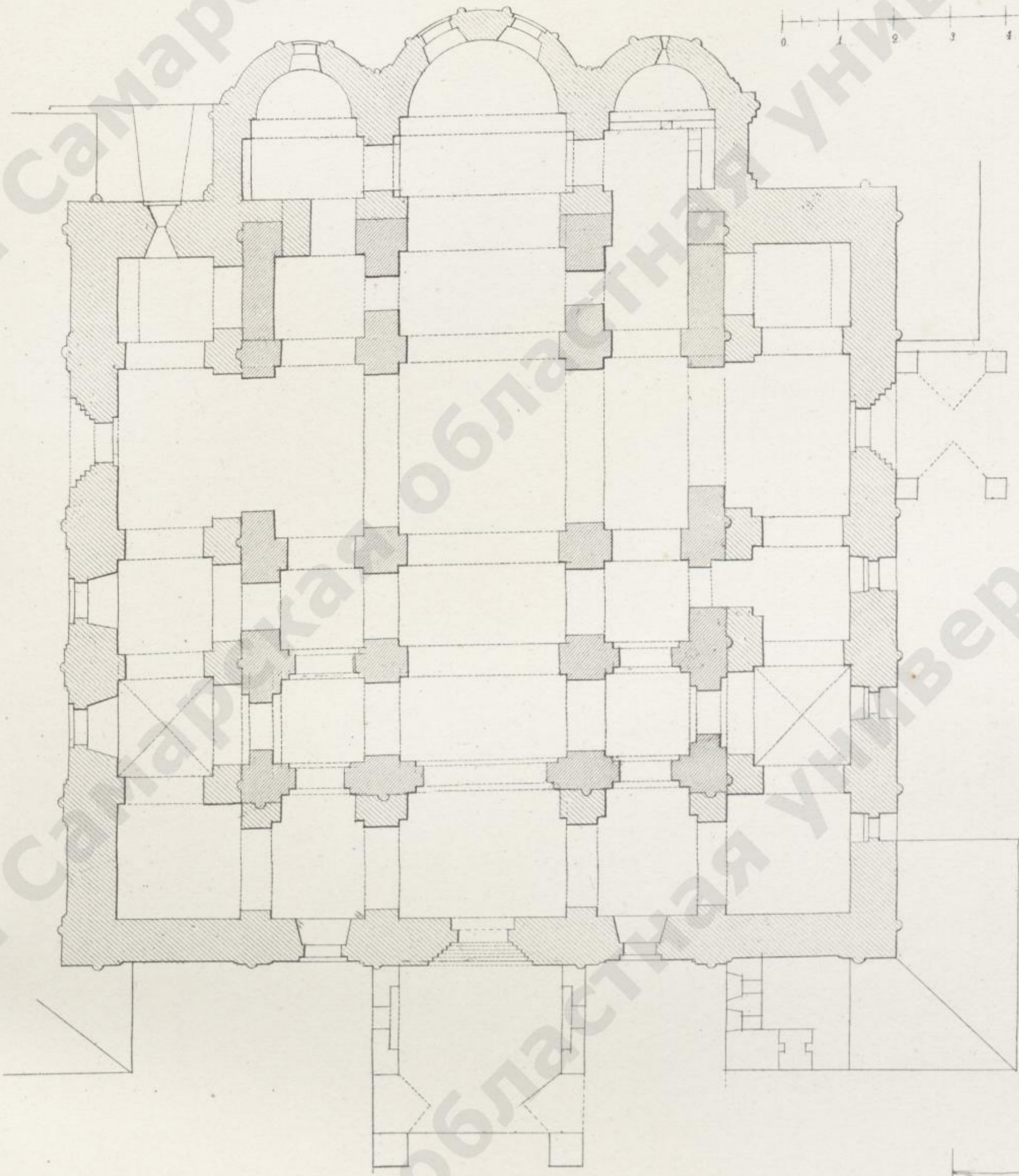
НИЖНИЙ ПЛАНЪ УСПЕНСКАГО СОБОРА
