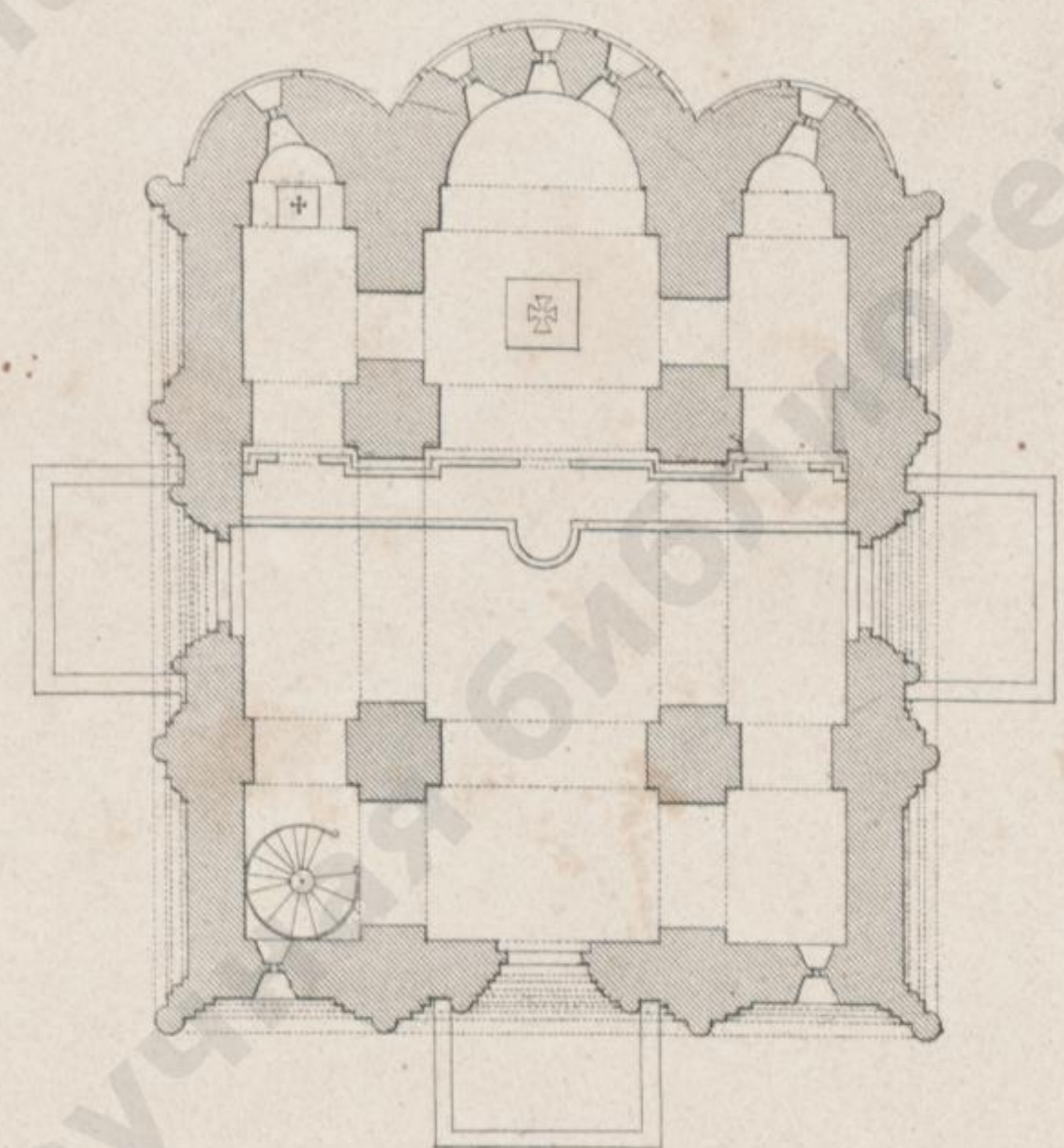
ПЛАНЪ ДМИТРІЕВСКАГО СОБОРА ВО ВЛАДИМИРѢ
