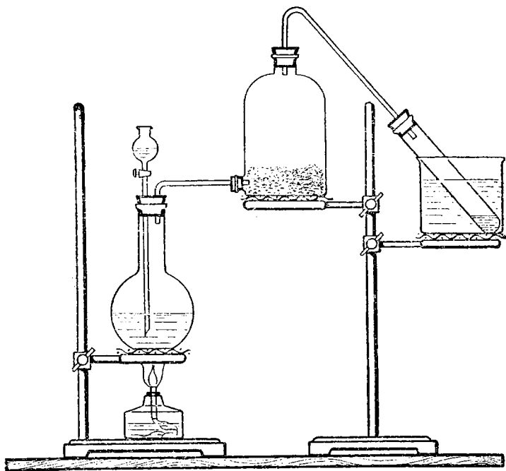
Рис. 1. Получение эфирного масла из плодов тмина.
