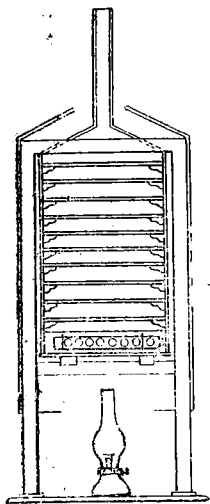
Рис. 4. Сушилка с током воздуха, идущим вверх.
