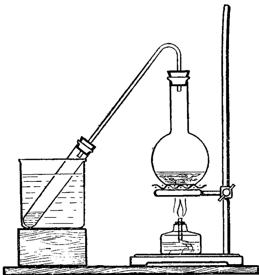
Рис. 2. Добывание эфирного масла из листьев душицы.
