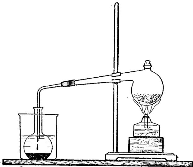
Рис. 3. Получение дегтя из бересты.
