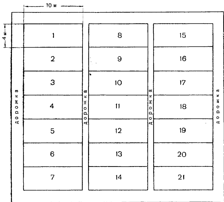
Рис. 7. План производственного участка.
