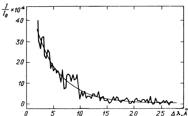
Рис. 28. Профиль линии ртути 2536 Å, полученный с узкой щелью через офсетную диафрагму
