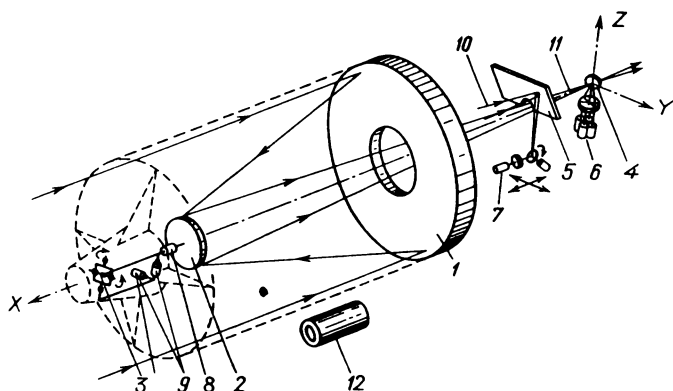
Рис. 13. Оптическая схема телескопа с элементами системы наведения и стабилизации: 1 — главное зеркало, 2 — вторичное зеркало, 3 — нейтральная точка телескопа, 4 — зеркальная пирамида, 5 — плоское диагональное зеркало, 6 — астродатчик ДПЗО, 8 — привод фокусировки, 9 — приводы системы стабилизации, 10 — свет от опорной звезды, 11 — свет от исследуемой звезды, 12 — телевизионная камера опознавания поля
