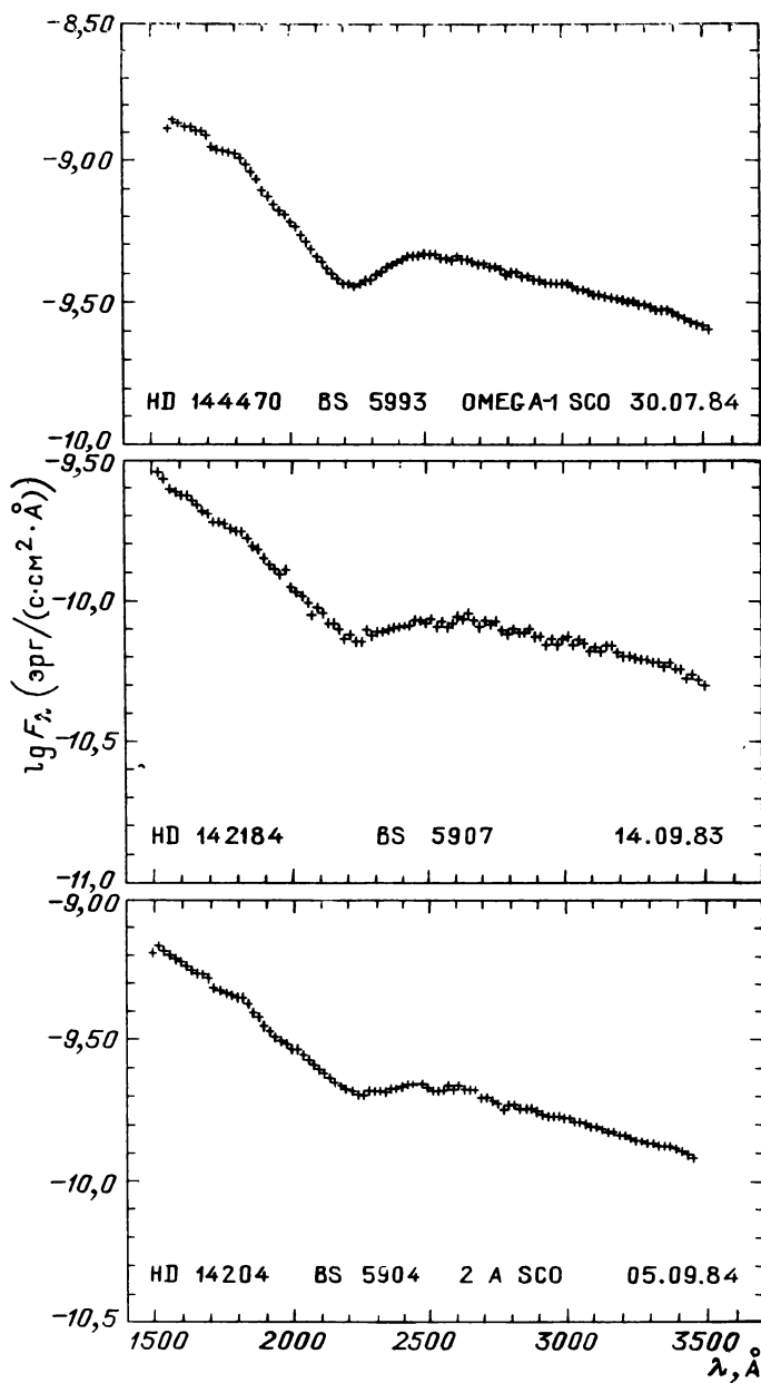
Рис. 31.24. Распределение энергии в спектрах звезд
