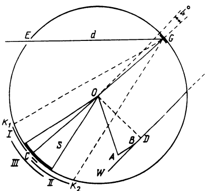
Рис. 14. Общая схема спектрометра: O — центр круга Роуланда, G — торондальная вогнутая решетка, C — центр кривизны дифракционной решетки, E — входная щель спектрометра, OAB — кривошипно-кулисный механизм сканирования, W — микрометрический винт, S — подвижной сектор с выходными щелями и фотоумножителями, K_1 K_2 — пределы перемещения сектора S при сканировании, I, II, III — участки сканирования трех каналов
