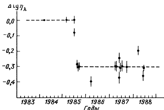
Рис. 23. Изменение абсолютной чувствительности УФС в центральной диафрагме
