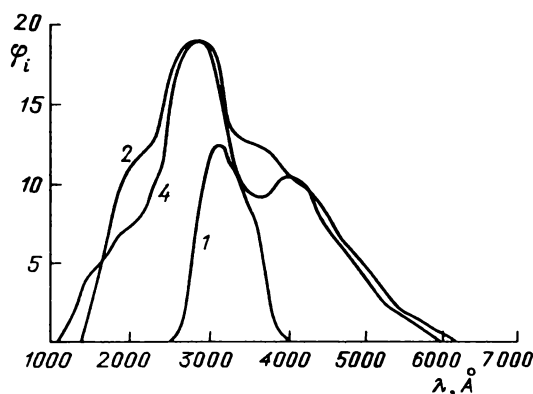
Рис. 30. Кривые реакции 1-го, 2-го, 4-го каналов УФС
