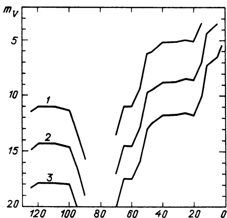
Рис. 12. Зависимость предельной звездной величины гидрочувствительной звезды от угла \alpha между оптической осью телескопа и направлением на Землю для трех положений космической станции на орбите: r = 50\,000 км (1), 100\,000 км — (2), 200\,000 км — (3)
