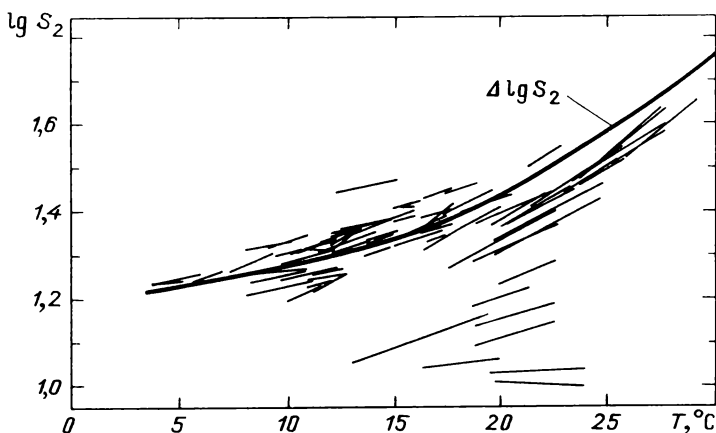
Рис. 26. Зависимость темного тока от температуры ФЭУ 2-го канала
