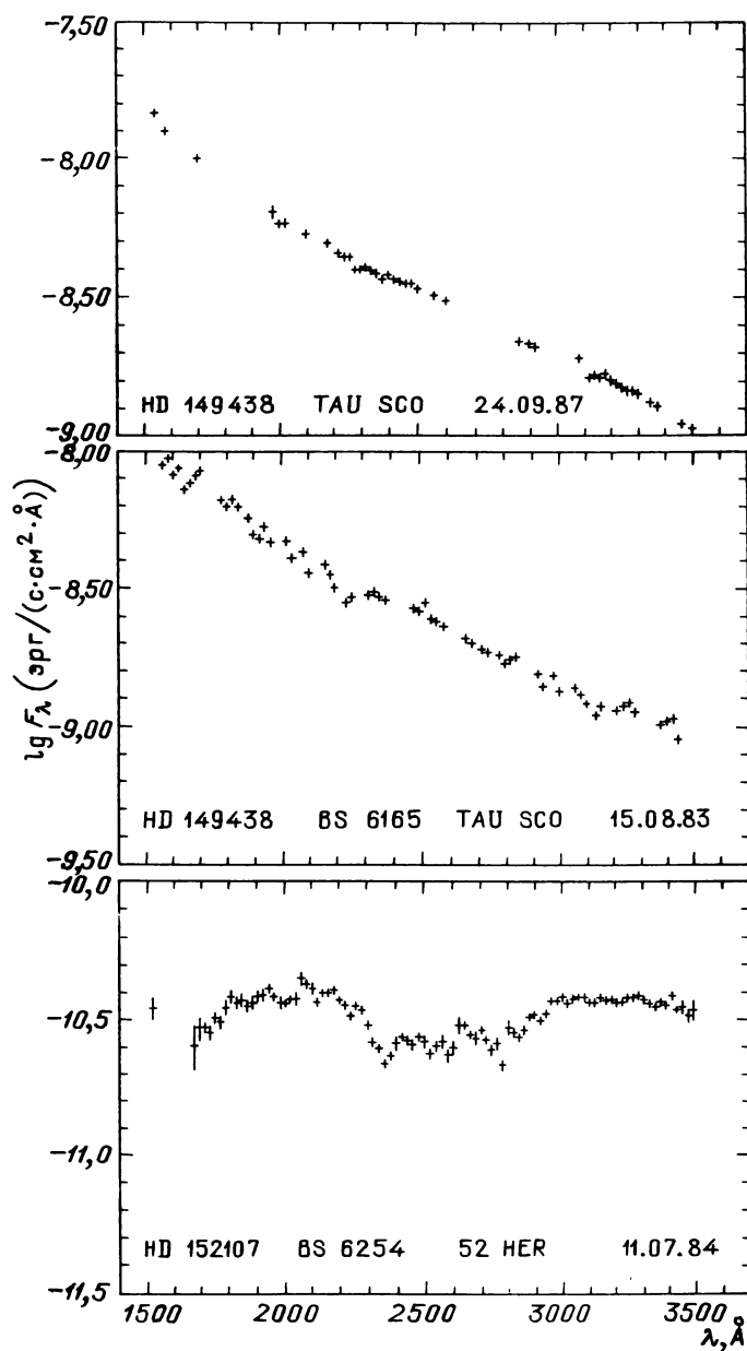
Рис. 31.27. Распределение энергии в спектрах звезд
