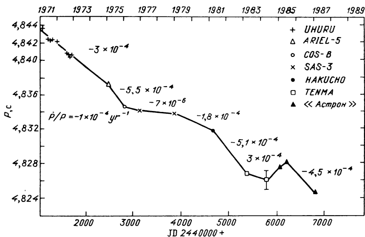
Рис. 78. Изменение периода пульсара Сеп X-3 со временем. Последние три значения получены по данным АС «Астро́н»
