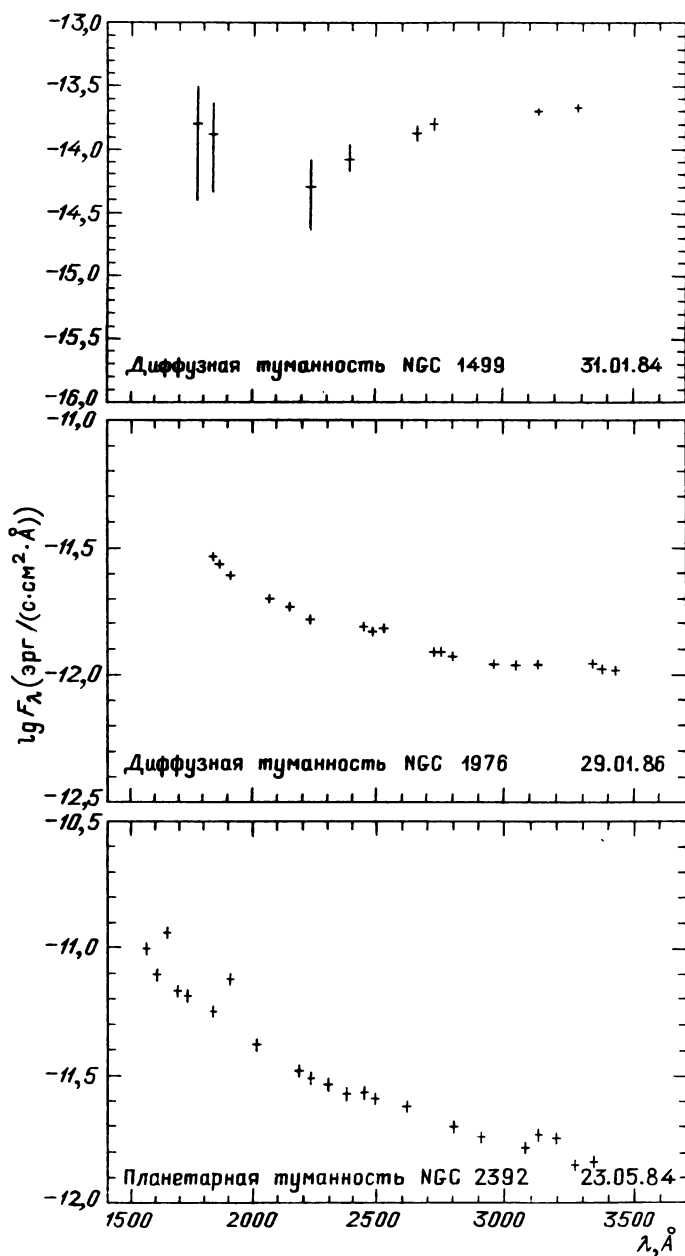
Рис. 64.1. Абсолютные значения потоков излучения газовых туманностей в полосах шириной 28 Å в интервале длин волн 1600–3500 Å
