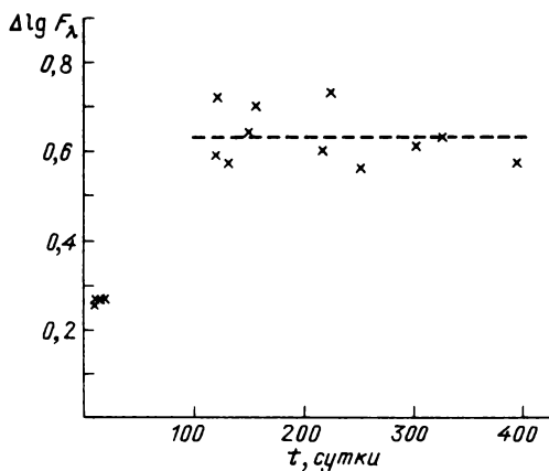
Рис. 42. Эволюция глубины бленды \lambda 3350 Å; штриховая линия соответствует среднему значению при t \geq 120^{\text{д}}
