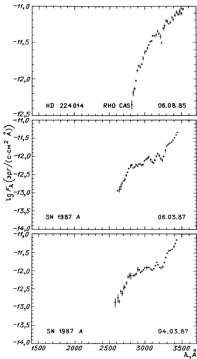
Рис. 31.40. Распределение энергии в спектрах звезд
