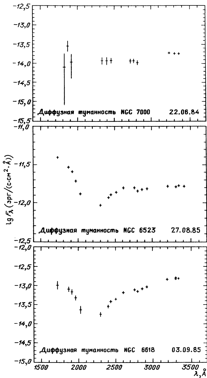
Рис. 64.6. Абсолютные значения потоков излучения газовых туманностей в полосах шириной 28 Å в интервале длин волн 1600–3500 Å
