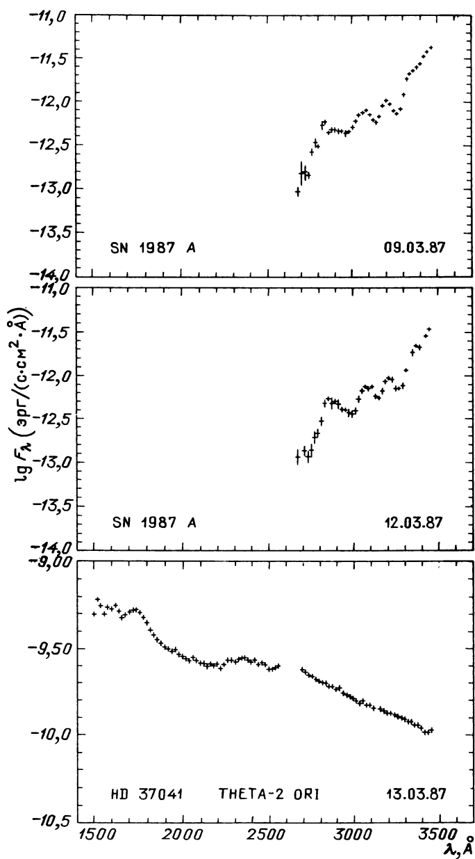
Рис. 31.41. Распределение энергии в спектрах звезд
