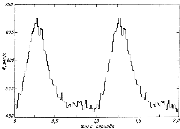
Рис. 79. Кривая блеска пульсара Сеп X-3, полученная 09.01.85
