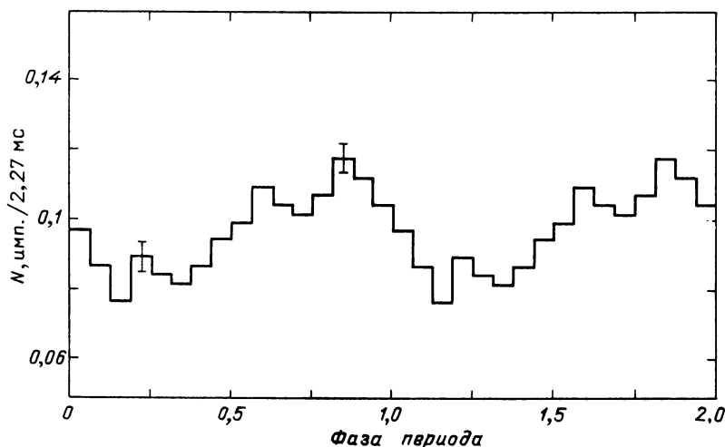
Рис. 90. Кривая блеска пульсара Нег X-1 по данным 08.04.85
