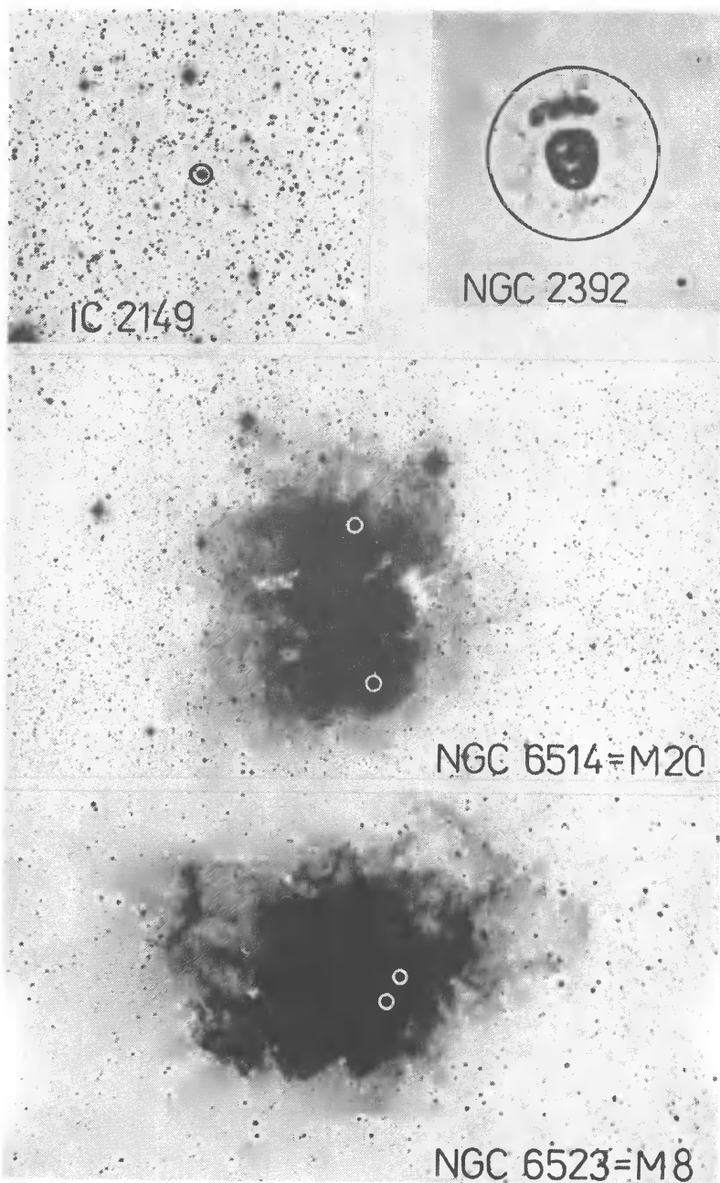
Рис. 63.2. Фотографии газовых туманностей. Размеры и положения колец соответствуют размерам и положениям диафрагм при наблюдениях
