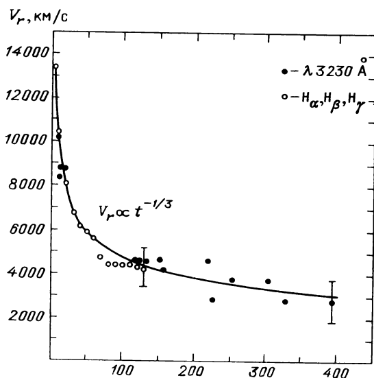
Рис. 38. Лучевая скорость как функция времени
