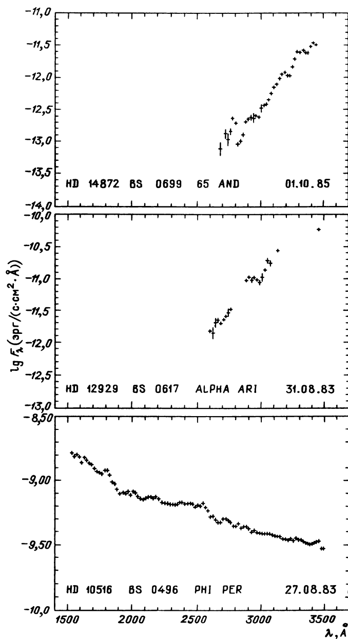
Рис. 31.1. Распределение энергии в спектрах звезд
