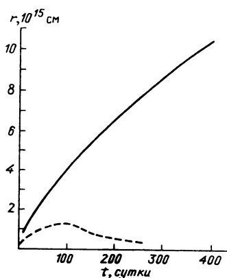
Рис. 39. Расстояние до слоя, где формируется бленда \lambda 3230 Å, как функция времени, штриховая линия — радиус фотосферы Сверхновой
