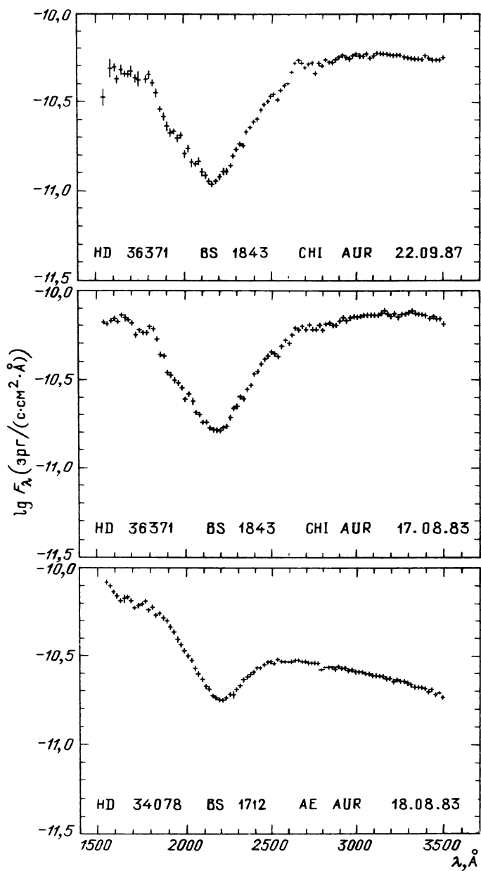
Рис. 31.8. Распределение энергии в спектрах звезд
