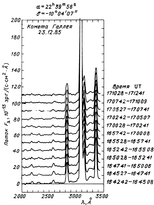
Рис. 65. Серия спектров кометы Галлея, полученных 23.12.85
