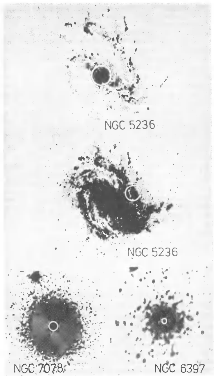
Рис. 48.1. Фотографии наблюдаемых звездных систем. Размеры диафрагмы изображены в виде колец и соответствуют данным столбца «диафрагма» табл. 10: O —офсетная, \Phi —фоновая
