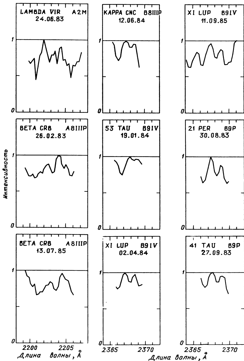
Рис. 47.19. Распределение энергии в спектрах звезд, наблюдавшихся с высоким спектральным разрешением
