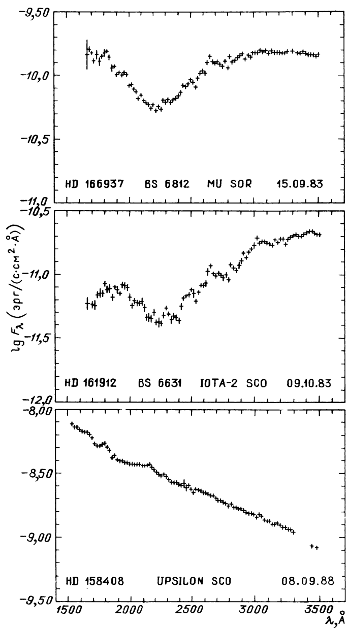
Рис. 31.32. Распределение энергии в спектрах звезд
