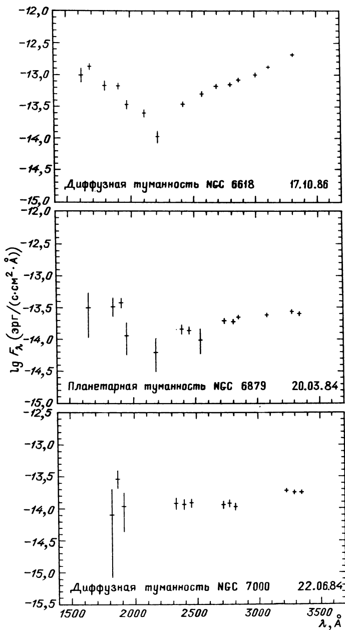
Рис. 64.8. Абсолютные значения потоков излучения газовых туманностей в полосах шириной 28 Å в интервале длин волн 1600–3500 Å
