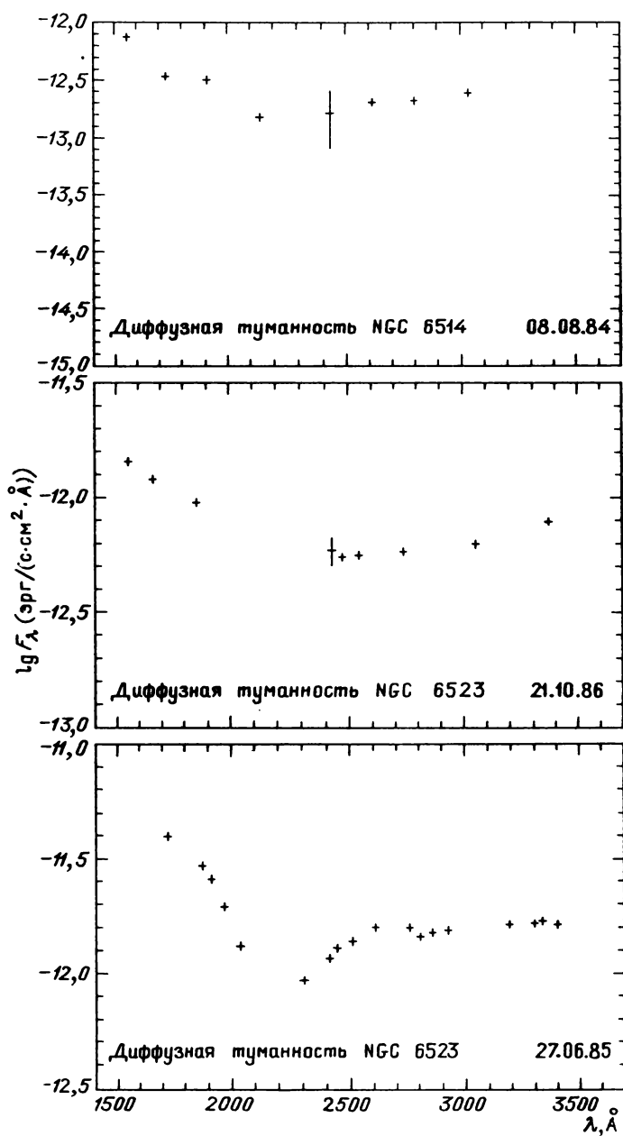
Рис. 64.3. Абсолютные значения потоков излучения газовых туманностей в полосах шириной 28 Å в интервале длин волн 1600–3500 Å
