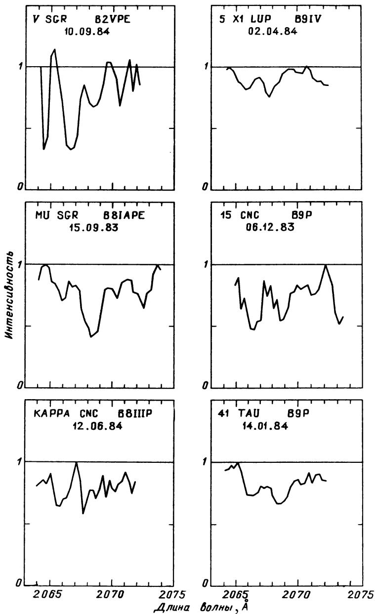
Рис. 47.14. Распределение энергии в спектрах звезд, наблюдавшихся с высоким спектральным разрешением
