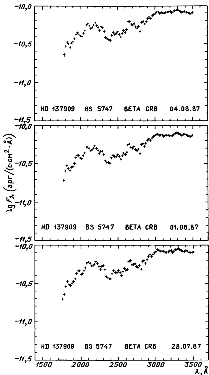
Рис. 31.21. Распределение энергии в спектрах звезд
