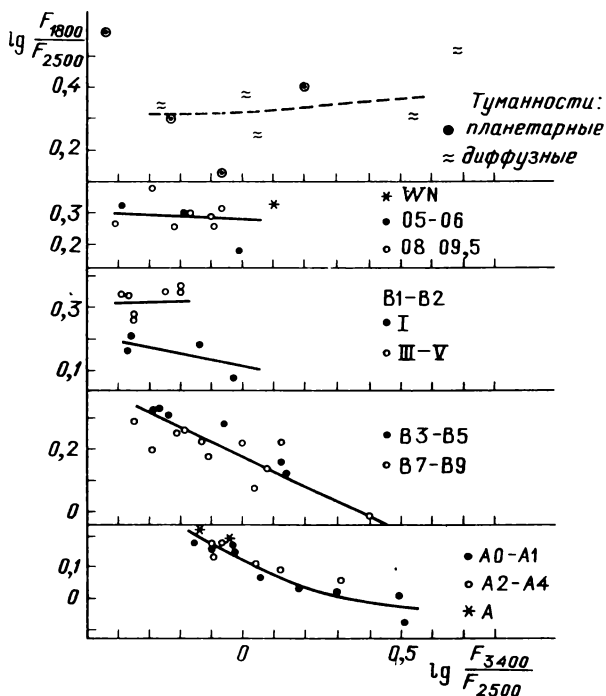
Рис. 60. Двухцветная диаграмма газовых туманностей и звезд спектральных классов 05 — 06, B1 — B2, B3 — B5, A0 — A1
