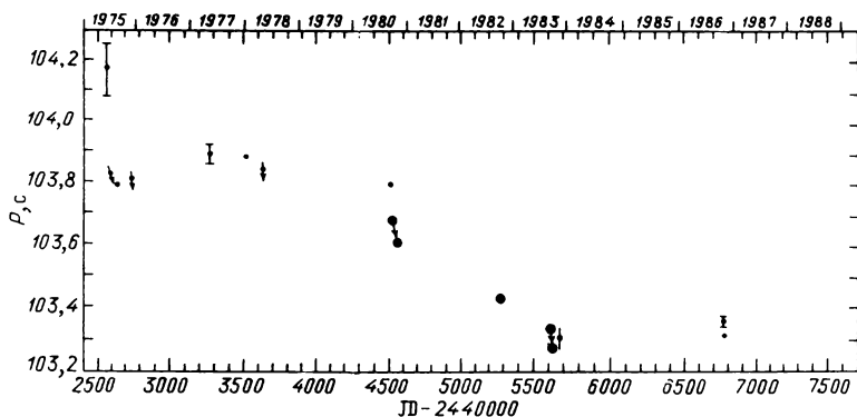
Рис. 77. Изменение периода пульсара A0535+26 со временем (в юлианских днях)
