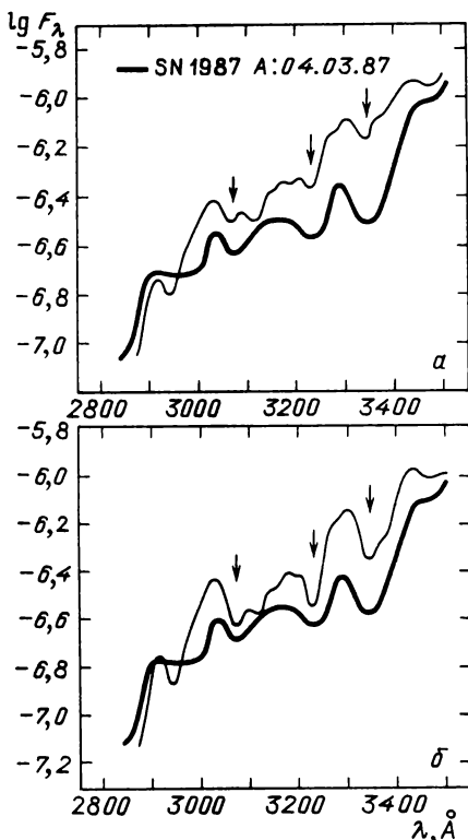
Рис. 41. Сравнение наблюдаемого спектра (толстые линии) с синтетическими (тонкие линии), вычисленными при нормальном (а) и повышенном (б) содержании металлов; стрелками указаны три бленды, полностью сформированные линиями TiII
