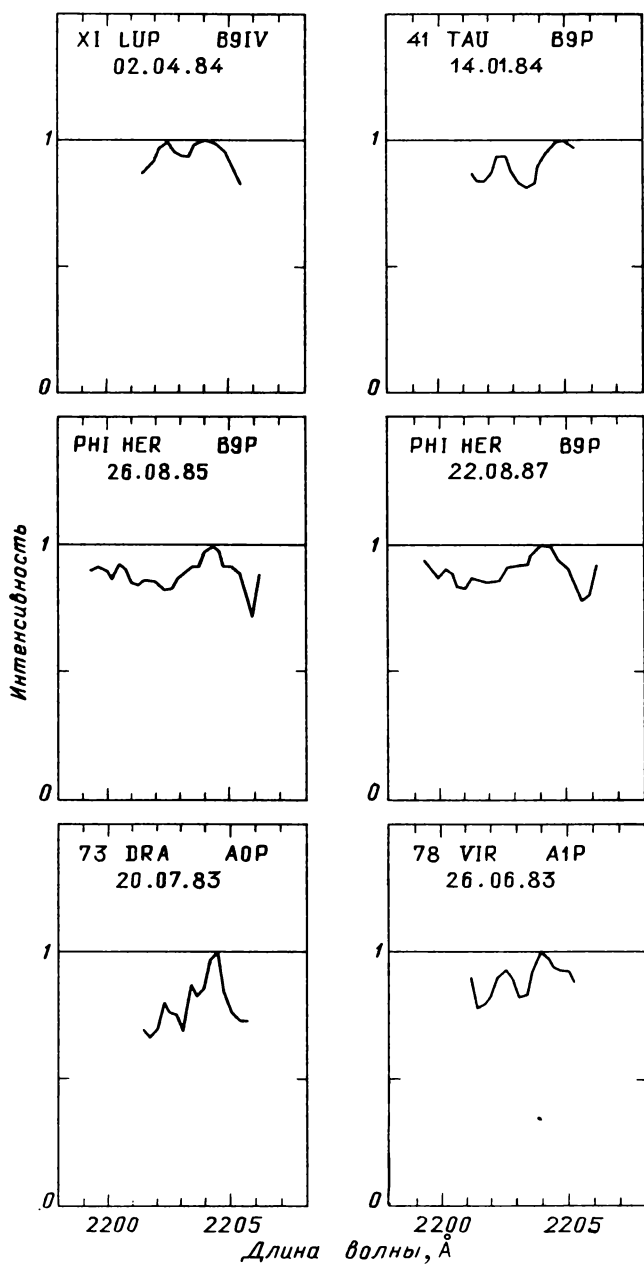
Рис. 47.17. Распределение энергии в спектрах звезд, наблюдавшихся с высоким спектральным разрешением
