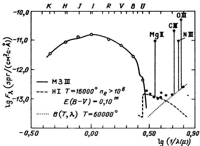
Рис. 43. Результаты наблюдений звезды EG And: черные кружки — «Астрон» 20.12.83, светлые кружки — телескоп АЗТ-11 19.12.83
