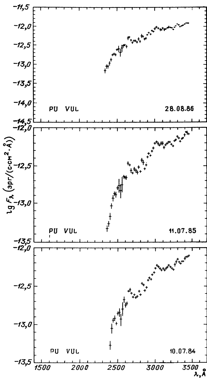
Рис. 31.37. Распределение энергии в спектрах звезд
