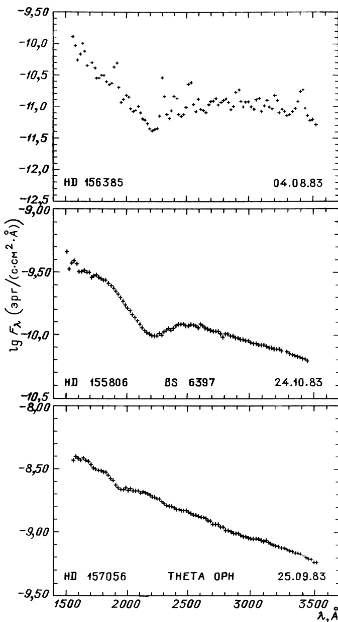
Рис. 31.31. Распределение энергии в спектрах звезд
