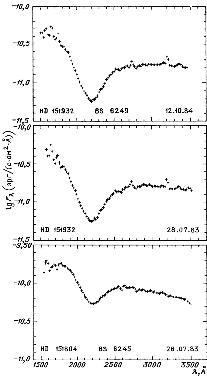
Рис. 31.28. Распределение энергии в спектрах звезд
