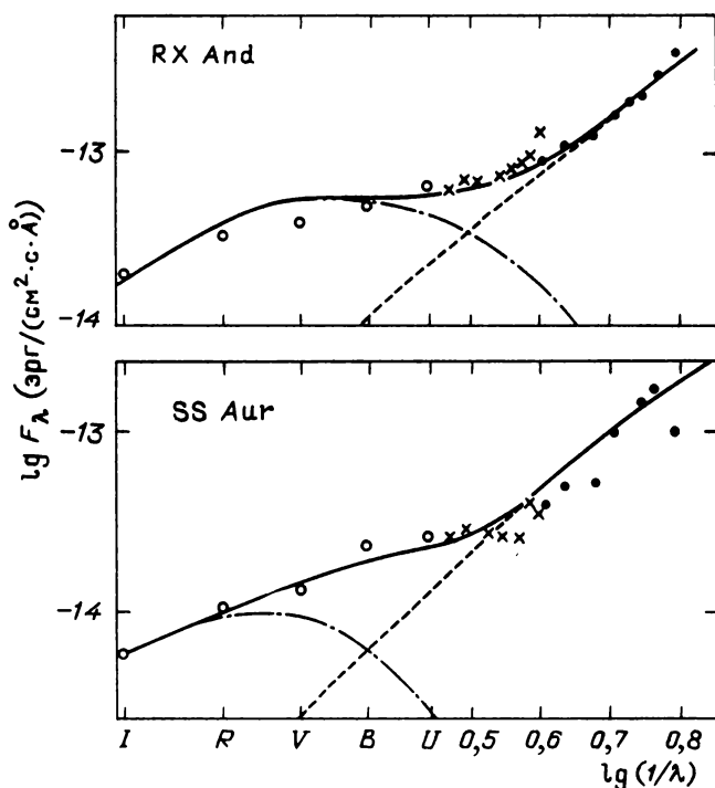
Рис. 44. Распределение энергии в спектрах звезд RX And и SS Aur
