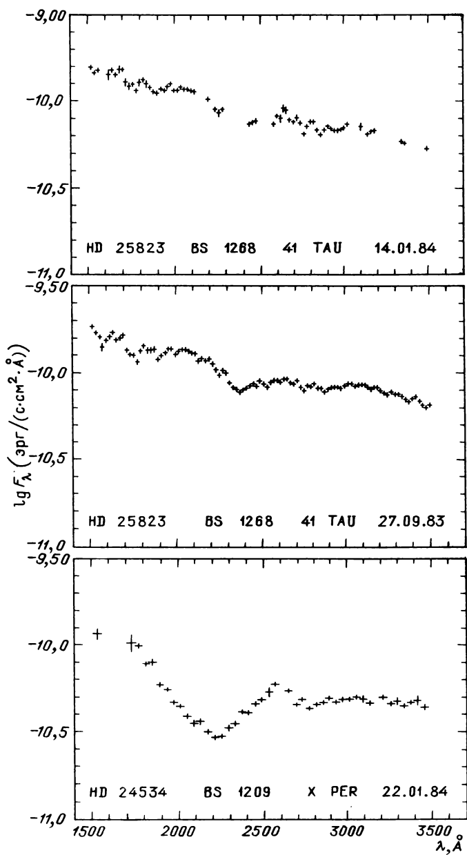
Рис. 31.4. Распределение энергии в спектрах звезд
