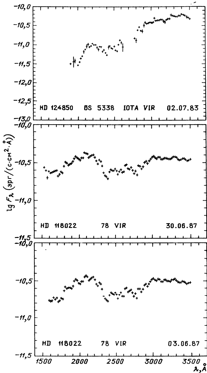
Рис. 31.17. Распределение энергии в спектрах звезд
