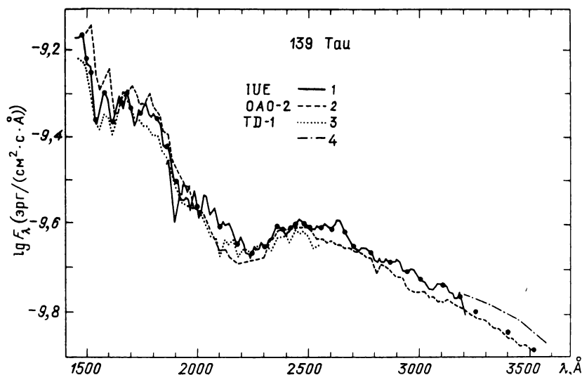
Рис. 20. Результаты наблюдения звезды 139 Тау. Спектральная плотность
