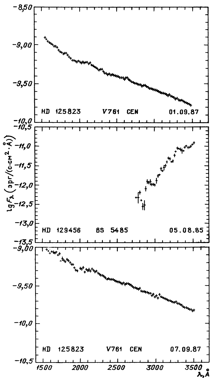
Рис. 31.18. Распределение энергии в спектрах звезд
