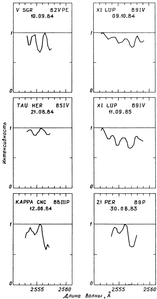
Рис. 47.23. Распределение энергии в спектрах звезд, наблюдавшихся с высоким спектральным разрешением
