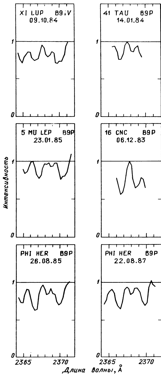
Рис. 47.20. Распределение энергии в спектрах звезд, наблюдавшихся с высоким спектральным разрешением
