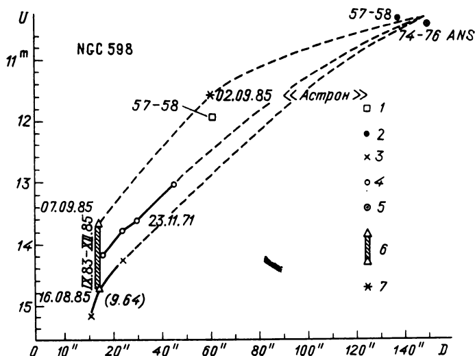
Рис. 57. Яркость галактики NGC 598 (М 33) в разных диафрагмах по наблюдениям разных авторов: 1— [56], 2— [54], 3— [55], 4— [52], 5— [57], 6— [53], 7 — «Астрон»
