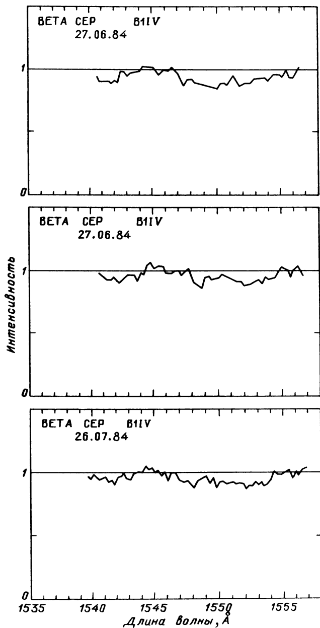
Рис. 47.4. Распределение энергии в спектрах звезд, наблюдавшихся с высоким спектральным разрешением
