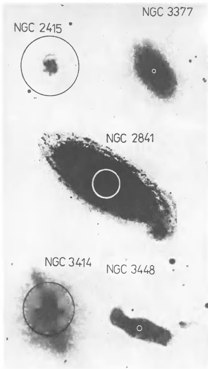
Рис. 48.4. Фотографии наблюдаемых звездных систем. Размеры диафрагмы изображены в виде колец и соответствуют данным столбца «диафрагма» табл. 10: O —офсетная, Ф —фоновая
