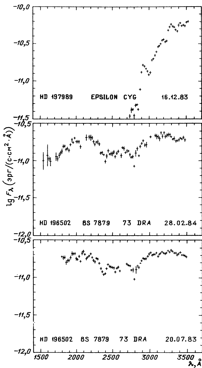
Рис. 31.36. Распределение энергии в спектрах звезд
