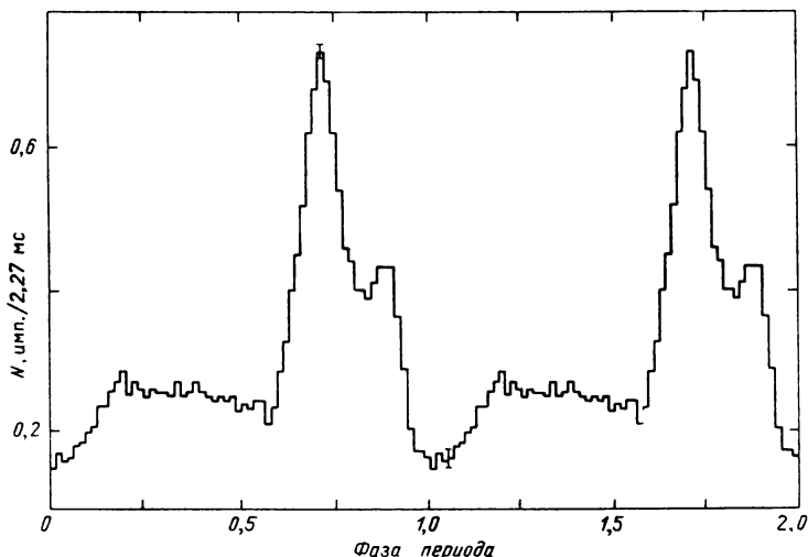
Рис. 86. Кривая блеска пульсара Нег X-1 по данным 07.04.84
