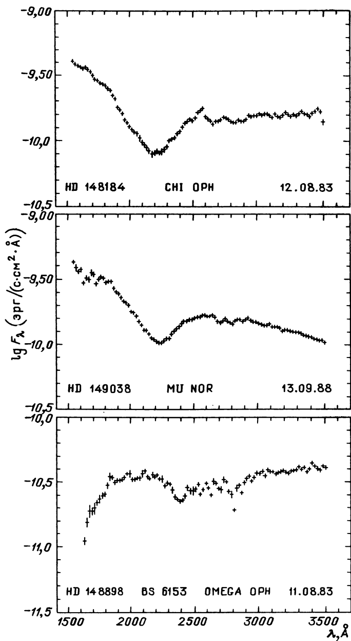
Рис. 31.26. Распределение энергии в спектрах звезд
