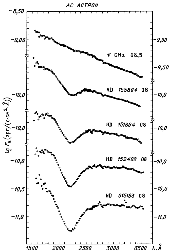
Рис. 34. Спектры звезд класса O8
