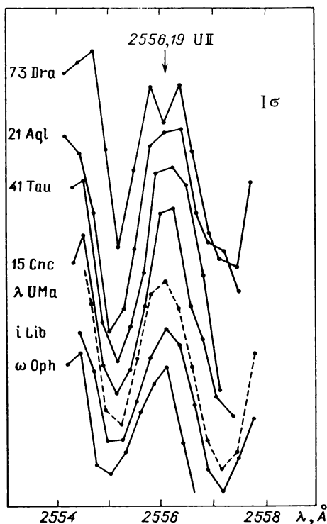
Рис. 35. Спектры в области линии U II, \lambda 2556,19, полученные для нескольких программных звезд. Запись интенсивностей дана в относительных единицах. Кривые, соответствующие разным звездам, для наглядности сдвинуты относительно друг друга
