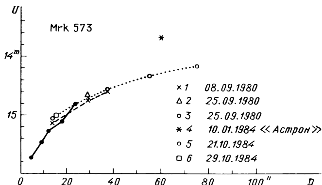
Рис. 56. Яркость галактики Mrk 573 в разных диафрагмах по данным С.И. Неизвестного [51] и наблюдениям на «Астроне»
