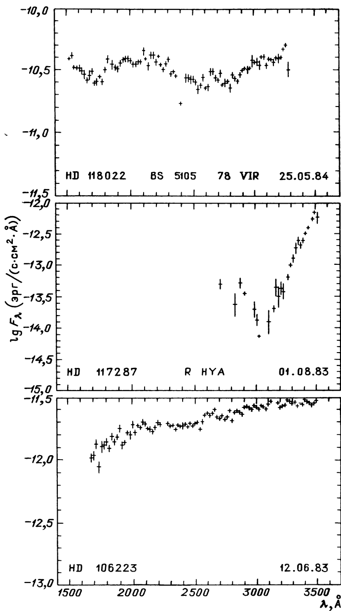
Рис. 31.16. Распределение энергии в спектрах звезд
