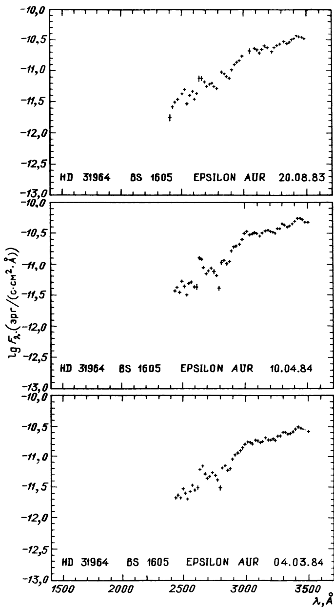
Рис. 31.6. Распределение энергии в спектрах звезд
