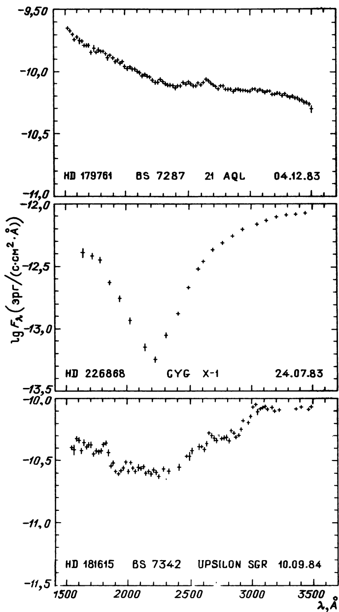
Рис. 31.34. Распределение энергии в спектрах звезд
