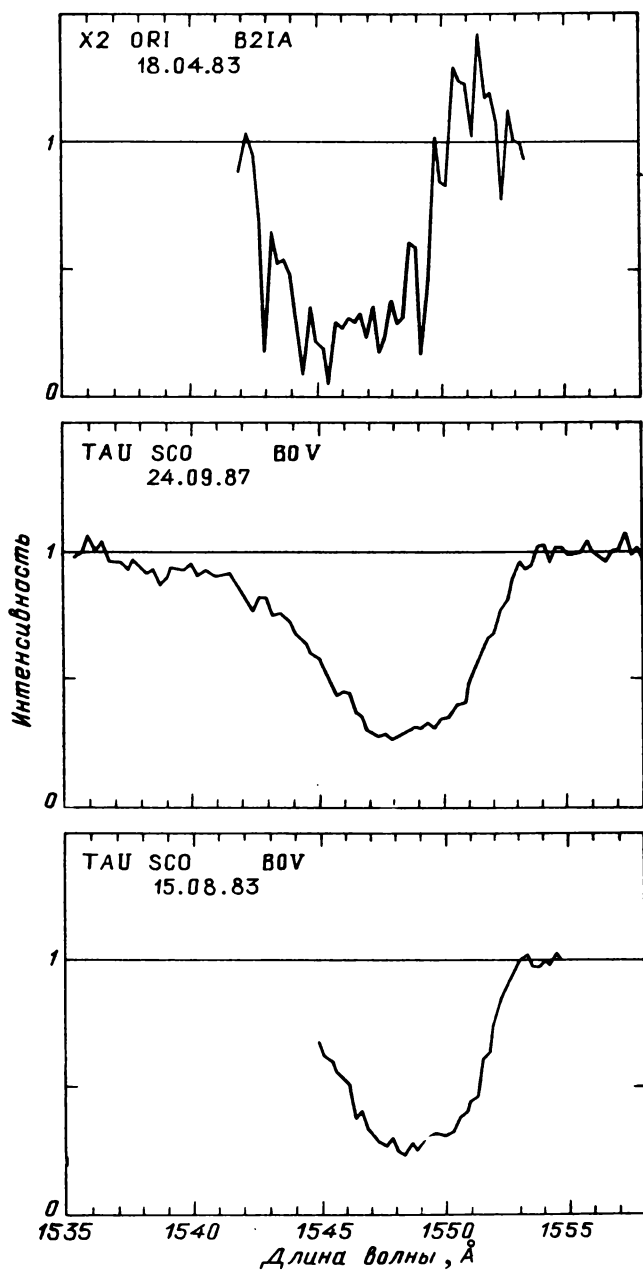
Рис. 47.3. Распределение энергии в спектрах звезд, наблюдавшихся с высоким спектральным разрешением
