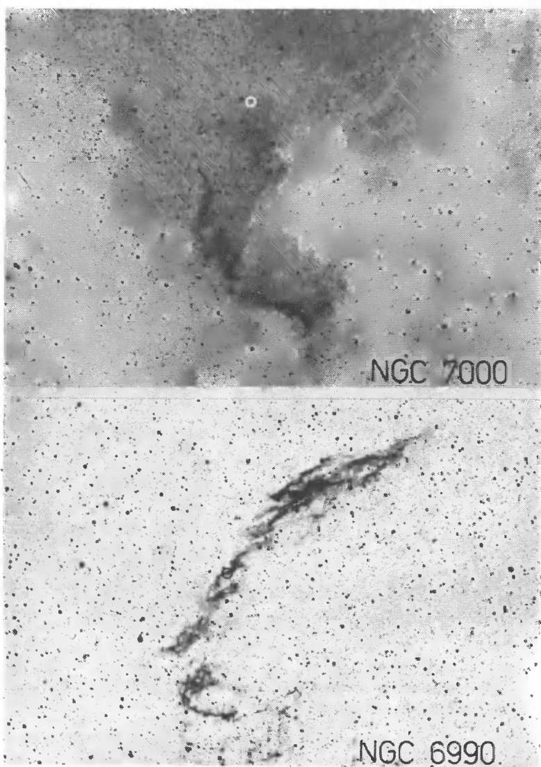
Рис. 63.3. Фотографии газовых туманностей. Размеры и положение колец соответствуют размерам и положениям диафрагм при наблюдениях
