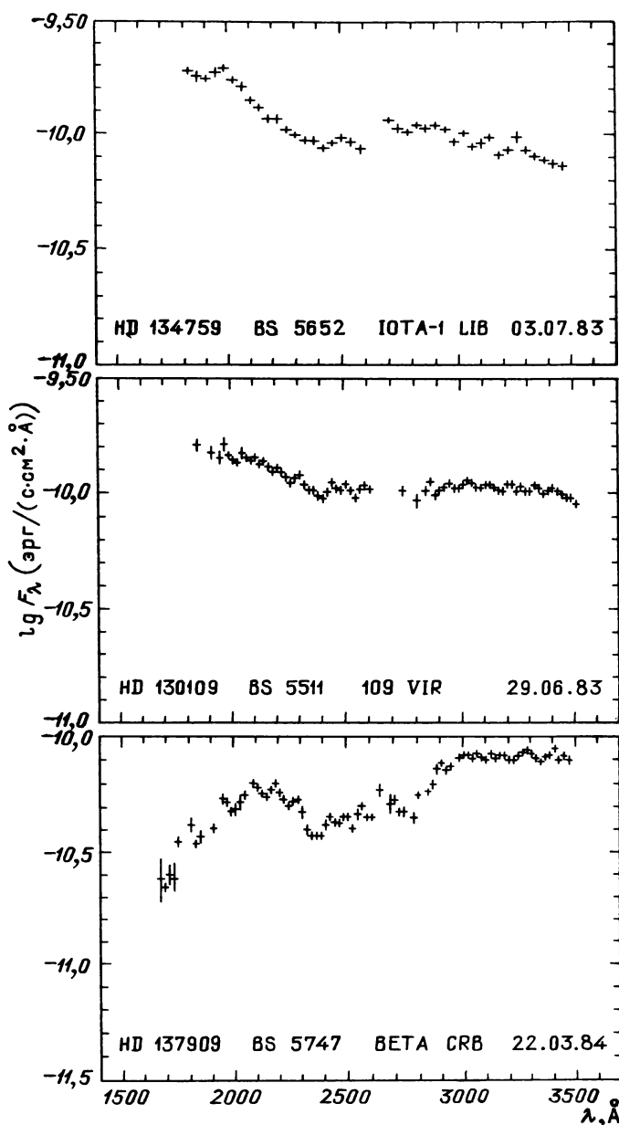
Рис. 31.19. Распределение энергии в спектрах звезд
