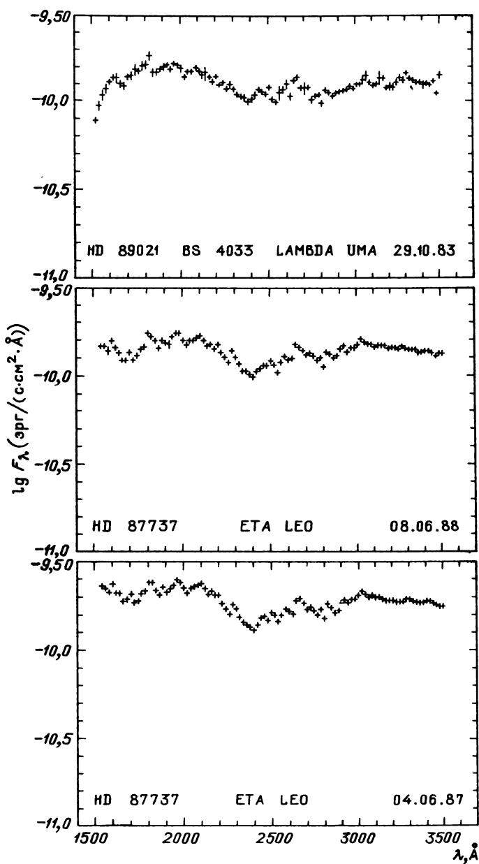
Рис. 31.13. Распределение энергии в спектрах звезд
