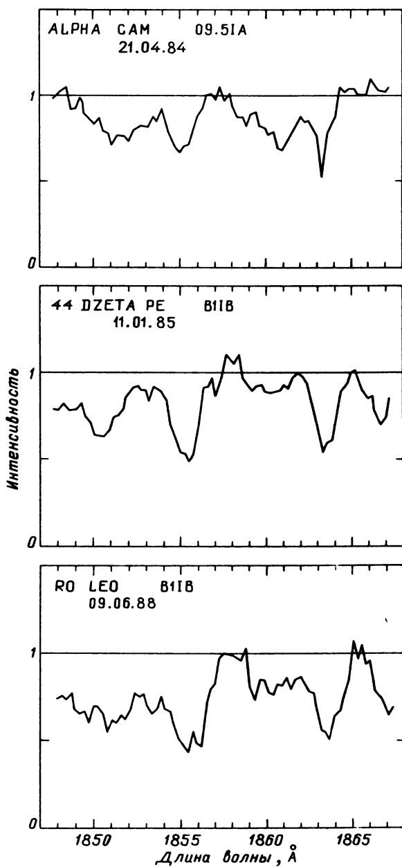
Рис. 47.6. Распределение энергии в спектрах звезд, наблюдавшихся с высоким спектральным разрешением
