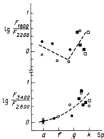
Рис. 59. Сопоставление ультрафиолетовых цветов галактик с их спектральным классом. Обозначения морфологических типов галактик как на рис. 51
