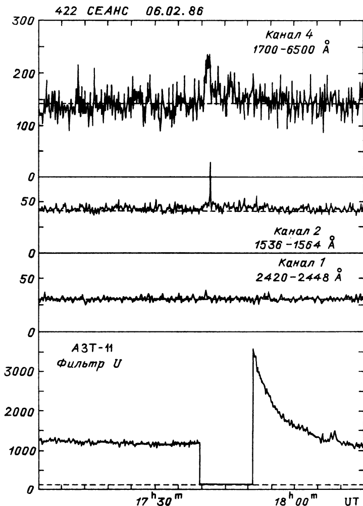
Рис. 46. Вспышка EV Lac 6.02.86. Наблюдения на «Астроне» и на телескопе АЗТ-11 в Крымской астрофизической обсерватории
