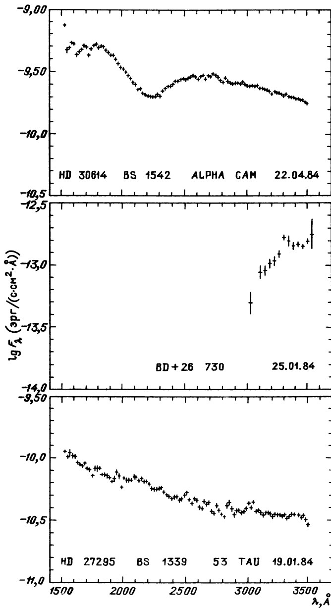
Рис. 31.5. Распределение энергии в спектрах звезд
