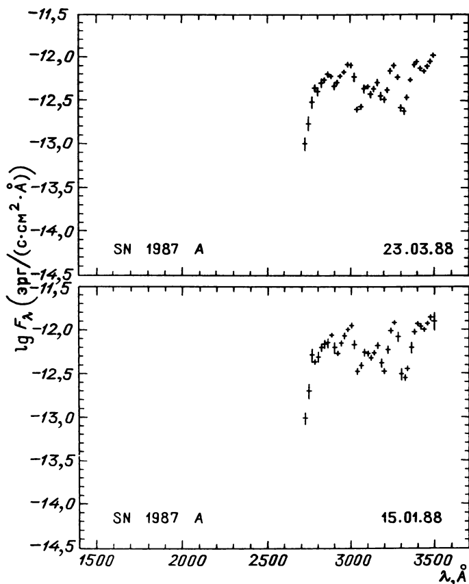
Рис. 31.45. Распределение энергии в спектрах звезд
