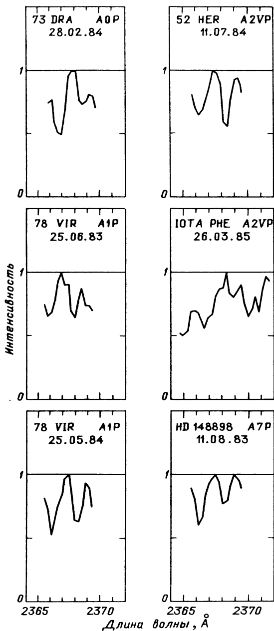
Рис. 47.21. Распределение энергии в спектрах звезд, наблюдавшихся с высоким спектральным разрешением
