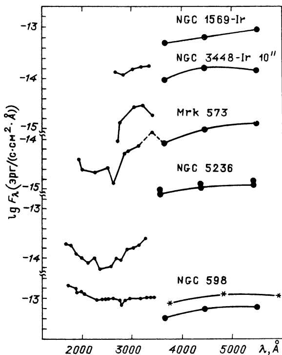
Рис. 55. Спектры галактик, для которых ультрафиолетовый участок спектра не согласуется с видимым
