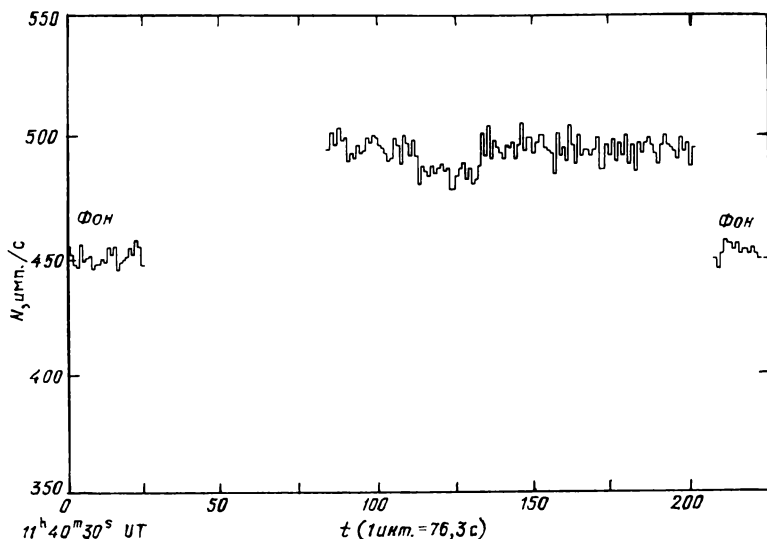
Рис. 89. Скорость счета фотона от пульсара Нег X-1 в диапазоне 2–25 кэВ в состоянии «low on» 08.04
