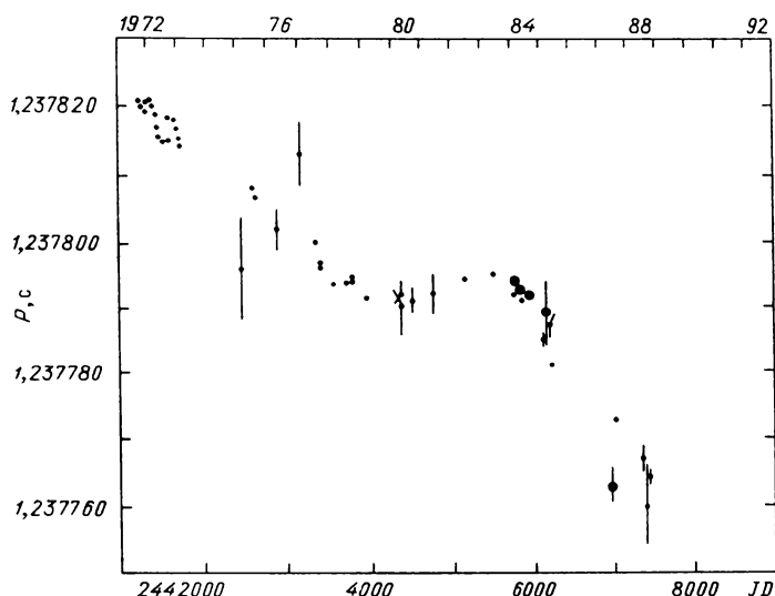
Рис. 92. Изменение периода пульсара Her X-1 за время 1972–1989
