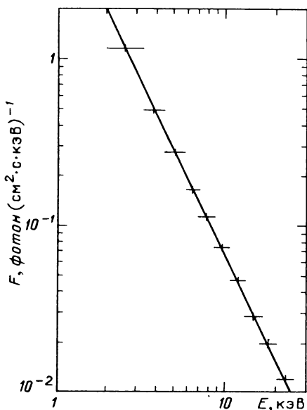
Рис. 74. Спектр рентгеновского излучения Крабовидной туманности, зарегистрированный на АС «Астрон». Сплошная линия — теоретический спектр вида F = AE^{-\alpha} e^{-\sigma N_H} (фотон/ (см 2 · с · кэВ)), где \alpha = 2,13 ; A = 9,4 и N_H = 3 \cdot 10^{21} атом/см 2 .
