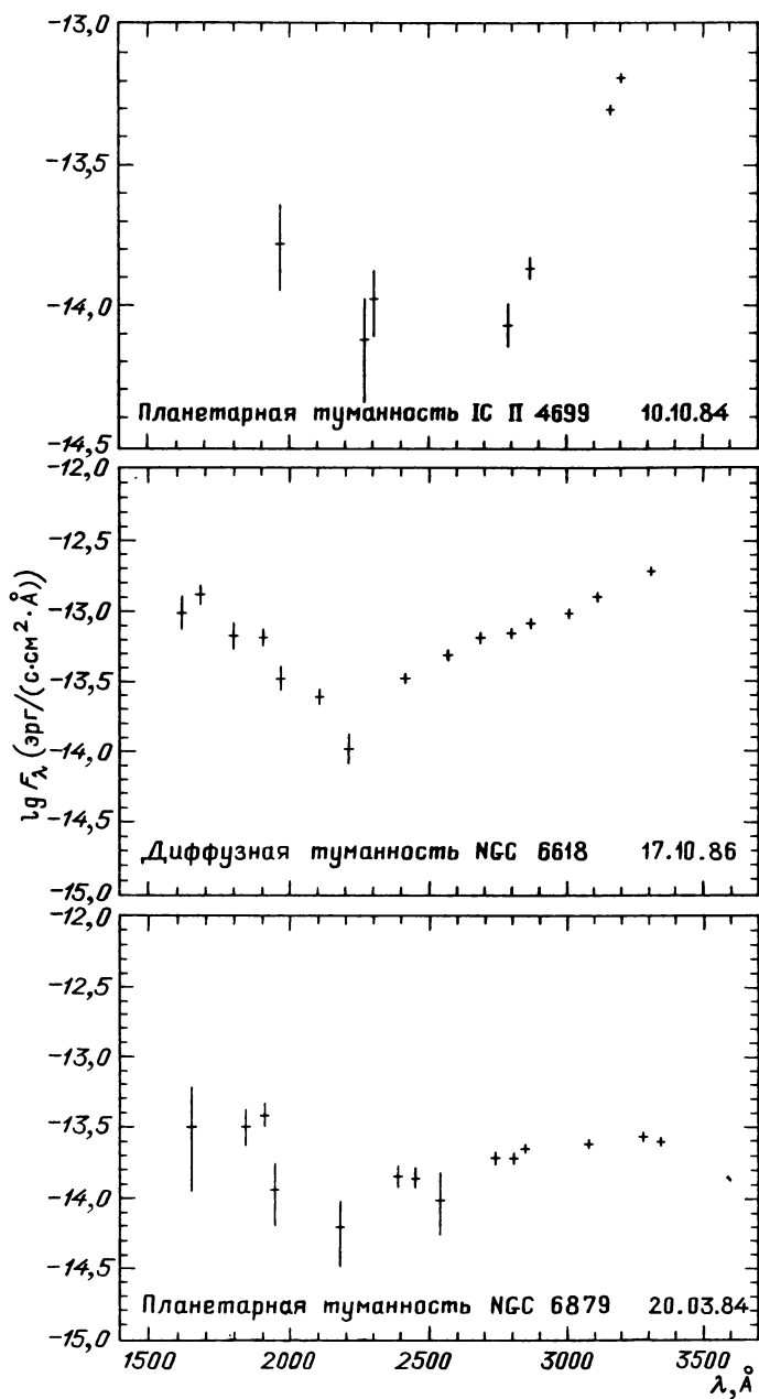
Рис. 64.5. Абсолютные значения потоков излучения газовых туманностей в полосах шириной 28 Å в интервале длин волн 1600–3500 Å
