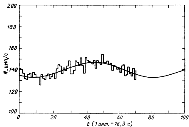
Рис. 84. Вариация среднего потока излучения от источника Her X-1 в сеансе 01.03.84. Синусоидальная кривая проведена методом наименьших квадратов
