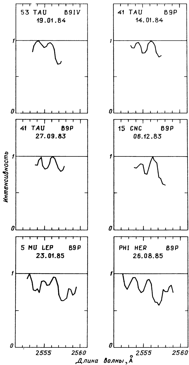
Рис. 47.24. Распределение энергии в спектрах звезд, наблюдавшихся с высоким спектральным разрешением
