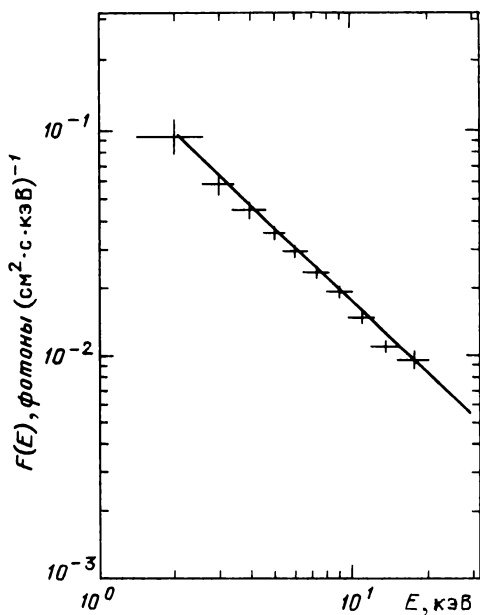
Рис. 88. Спектр Her X-1 в состоянии «high on» в сеансе 25.08. 84
