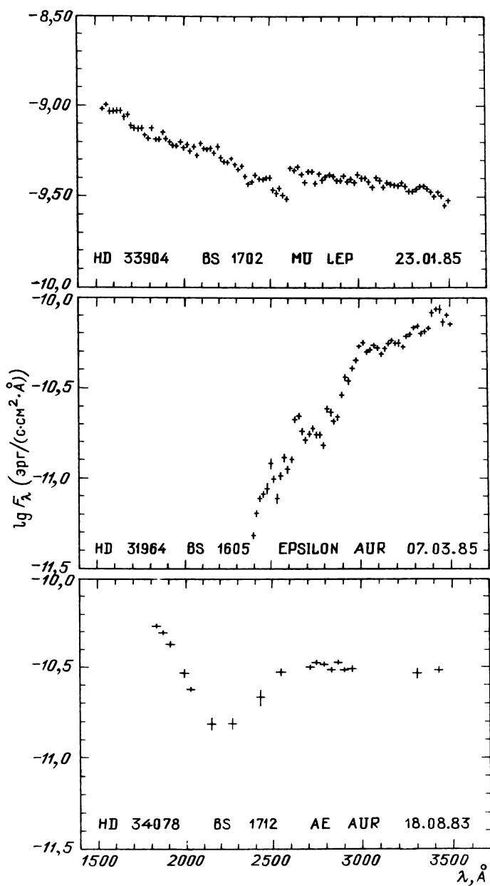
Рис. 31.7. Распределение энергии в спектрах звезд
