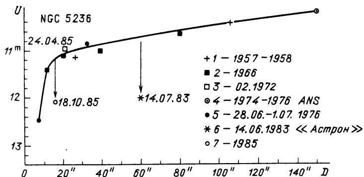
Рис. 58. Яркость галактики NGC 5236 (М 83) в разных диафрагмах по наблюдениям разных авторов: 1 — [58], 2 — [59], 3 — [23], 4 — [57], 5 — [62], 6 — «Астрон», 7 — [61]
