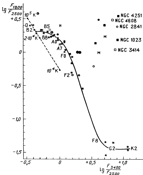
Рис. 61. Двухцветная диаграмма для ультрафиолетового спектра галактик и одиночных непокрашенных звезд главной последовательности. Обозначения галактик те же, что и на рис. 51
