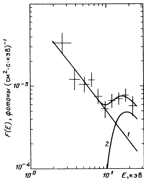
Рис. 82. Спектр Her X-1 в продолжительном «выключенном» («off») состоянии в сеансе 30.06.83
