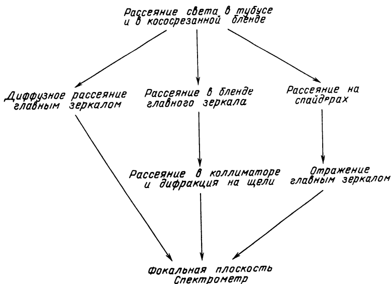
Рис. 11. Схема основных путей распространения рассеянного света в ультрафиолетовом телескопе
