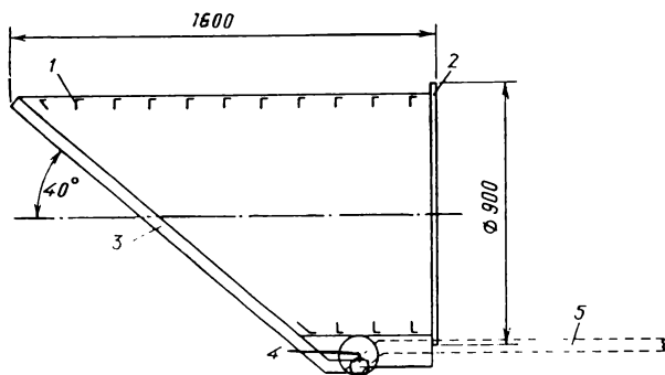
Рис. 7. Наружная блenda: 1 — диафрагмы, 2 — шпангоут, 3 — крышка, 4 — привод крышки, 5 — крышка в открытом положении
