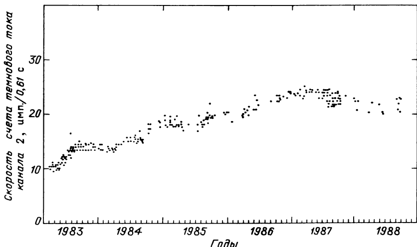
Рис. 27. Температурно однородные оценки темновых токов во 2-м канале
