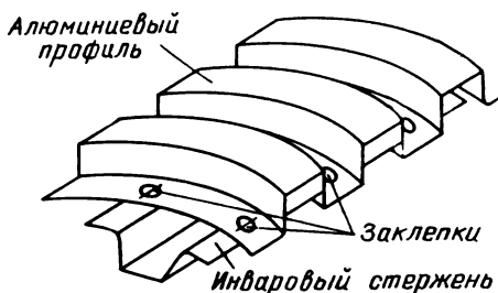
Рис. 9. Специальная форма алюминиевой обо- лочки тубуса и стержней
