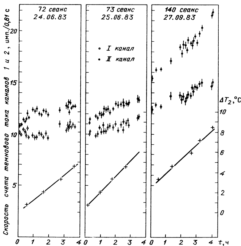
Рис. 25. Измерения темновых токов в 1-м и 2-м каналах
