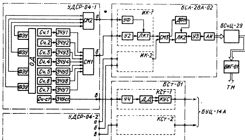
Рис. 71. Функциональная схема спектрометра СКР-02М
