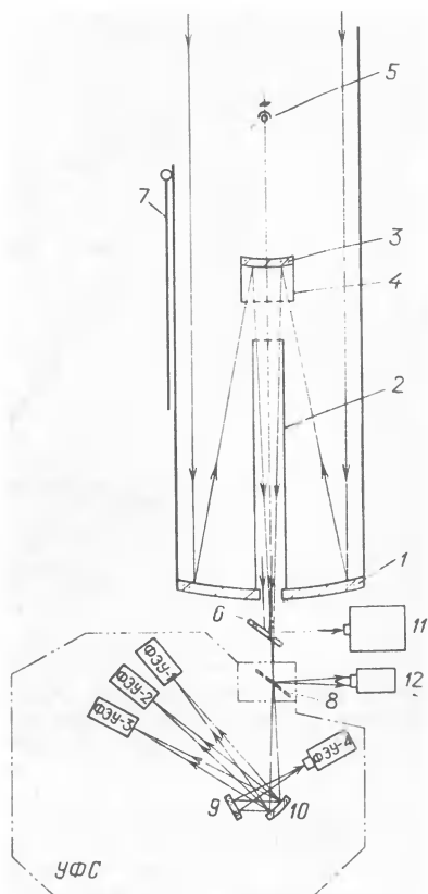
Рис. 3. Общая схема хода лучей в УФС «Спика» и в спектрометре (УФС): 1—главное зеркало, 2—бленда главного зеркала, 3—вторичное зеркало, 4—бленда вторичного зеркала, 5—центр качания вторичного зеркала, 6—диагональное зеркало, 7—свето-защитная крышка телескопа, 8—входные диафрагмы, 9—диагональное зеркало УФС, 10—дифракционная решетка, 11—датчик положения звезды (опорной) (ДПЗО), 12—датчик положения звезды (центральной) (ДПЗД)
