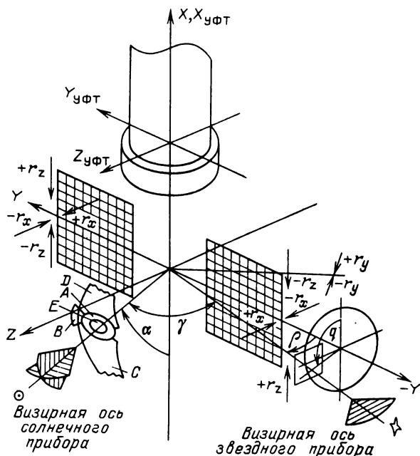
Рис. 2. Кинетическая схема расположения измерительных и исполнительных элементов СУО. Оси УФТ совпадают с осями XYZ станции. A, B, C, D и E — управляющие зоны солнечного прибора; r_x, r_y, r_z — векторы управляющих воздействий исполнительных элементов; \gamma — угол «Солнце-станция-звезда», \alpha — угол установки визирной оси солнечного прибора; \rho и q — углы установки оси звездного прибора
