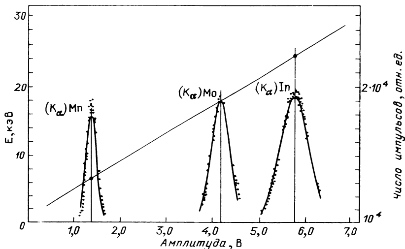
Рис. 72. Зависимость амплитудного распределения импульсов детектора от энергии рентгеновского излучения радиоактивных источников
