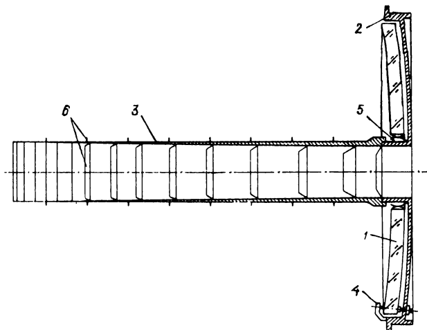
Рис. 10. Узел главного зеркала: 1 — зеркало, 2 — оправа, 3 — бленда главного зеркала, 4 — основные прижимы, 5 — радиальные фиксаторы, 6 — диафрагмы бленды главного зеркала
