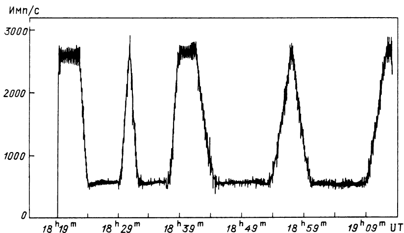
Рис. 73. Изменение сигнала спектрометра СКР-02М во время сеанса юстировки аппаратуры по рентгеновскому излучению от Крабовидной туманности
