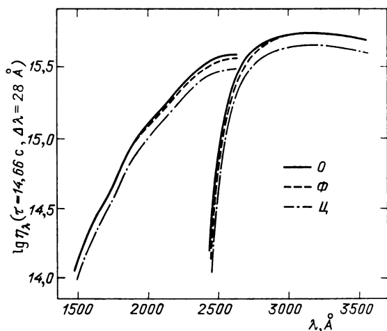
Рис. 21. Зависимость абсолютной спектральной чувствительности \eta_\lambda от \lambda для различных режимов: сплошная линия — режим O с офсетной диафрагмой, штриховая линия — режим Φ с фоновой диафрагмой, штрих-пунктирная линия — режим Ц с центральной диафрагмой
