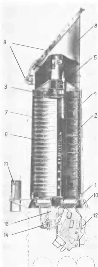
Рис. 6. Общий вид ультрафиолетового телескопа (УФТ): 1 — главное зеркало УФТ, 2 — бленда главного зеркала, 3 — вторичное зеркало, 4 — бленда вторичного зеркала, 5 — узел вторичного зеркала, 6 — бленда УФТ, 7 — корпус УФТ, 8 — герметизирующий кожух, 9 — крышка УФТ с приводом, 10 — коническая проставка, 11 — камера опознавания звездного поля, 12 — ультрафиолетовый спектрометр (УФС), 13 — ДПЗО, 14 — ДПЗЦ
