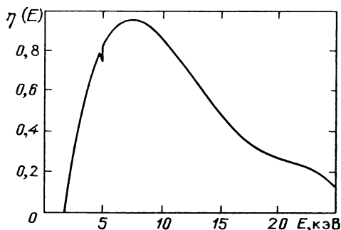
Рис. 70. Спектральная чувствительность спектрометра СКР-02М
