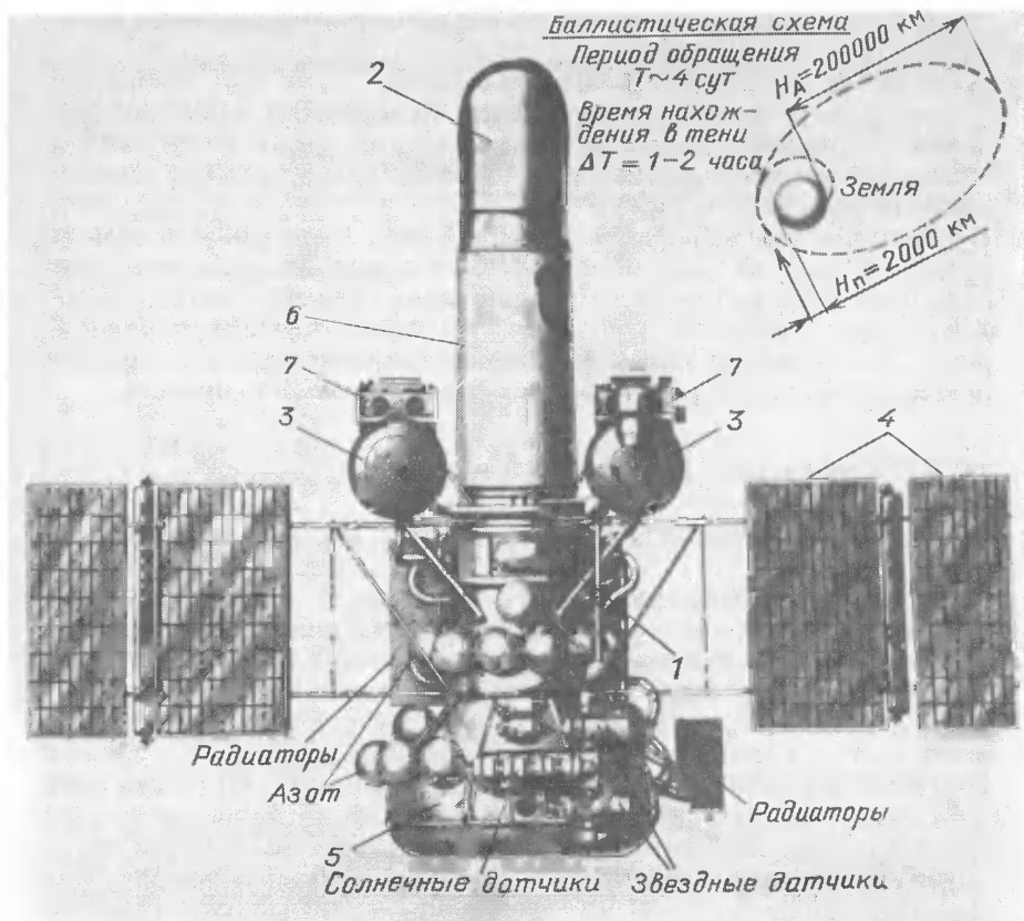
Рис. 1. Общий вид АС «Астрон»: 1 — опорный цилиндр, 2 — крышка ультрафиолетового телескопа, 3 — подвесные контейнеры, 4 — солнечные батареи, 5 — приборный отсек, 6 — герметизирующий кожух ультрафиолетового телескопа, 7 — рентгеновские спектрометры СКР-02М
