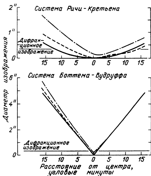
Рис. 4. Размер изображения на фокальной поверхности телескопа при гидировании вторичным зеркалом. Расчет выполнен методом точечной диафрагмы. Сплошная линия — звезда на оси, штриховая — уход звезды с оси на 2' , штрих-пунктир — уход звезды с оси на 5'
