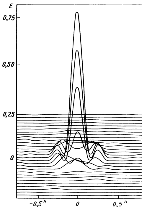
Рис. 5. Интерферограмма главного зеркала, полученная с компенсатором типа Оффнера
