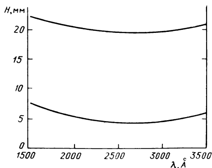
Рис. 15. Высота спектров в интервале длин волн 1500 — 3500 Å для сферической решетки с радиусом кривизны r = 500 мм (верхняя кривая) и тороидальной решетки с r = 404 мм (нижняя кривая)
