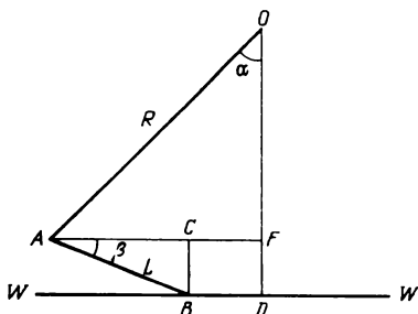
Рис. 17. Кривошипно-кулисный механизм для сканирования спектра: O — центр круга Роуланда, WW — точный микрометрический винт, OA и OB — подвижные плечи механизма
