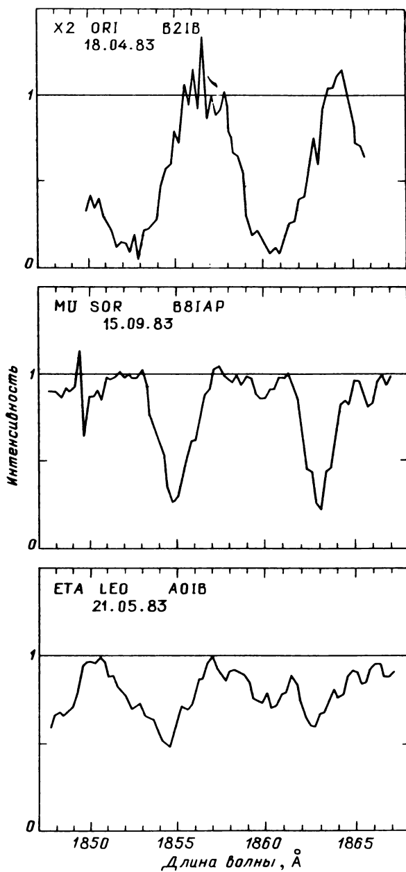
Рис. 47.7. Распределение энергии в спектрах звезд, наблюдавшихся с высоким спектральным разрешением
