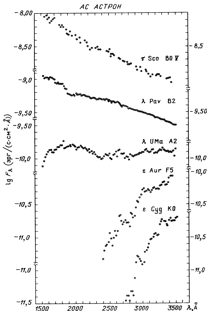
Рис. 32. Распределение энергии в области 1500–3500 Å в спектрах нормальных звезд, начиная со спектрального класса B0 ( T \sim 20\,000\text{ K} ) и до K0 ( T \sim 4500\text{ K} )
