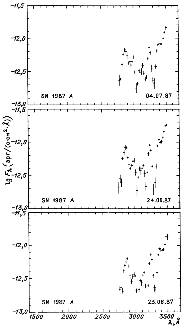
Рис. 31.42. Распределение энергии в спектрах звезд
