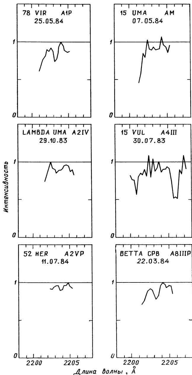
Рис. 47.18. Распределение энергии в спектрах звезд, наблюдавшихся с высоким спектральным разрешением
