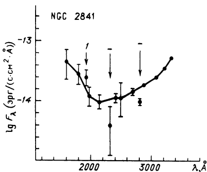
Рис. 50. Ультрафиолетовый спектр NGC 2841, стрелками отмечены абсорбционные полосы \lambda 2800 Å, \lambda 2300 Å и эмиссия CIII] 1909 Å
