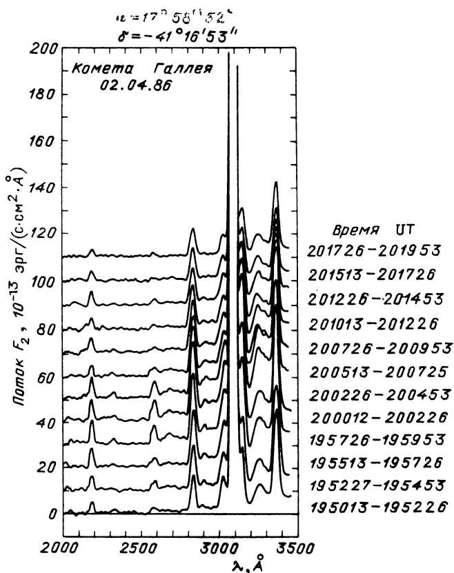
Рис. 66. Серия спектров кометы Галлея, полученных 02.04.86
