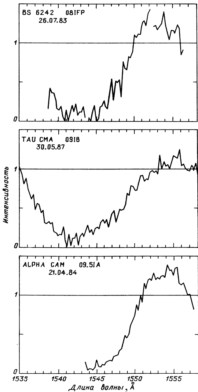
Рис. 47.1. Распределение энергии в спектрах звезд, наблюдавшихся с высоким спектральным разрешением
