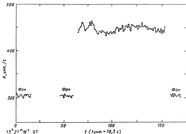
Рис. 83. Скорость счета в диапазоне 2–25 кэВ от пульсара Her X-1 01.03.84
