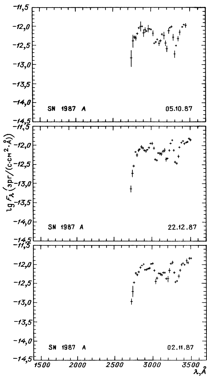
Рис. 31.44. Распределение энергии в спектрах звезд
