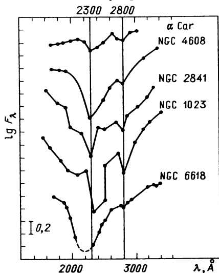
Рис. 53. Сопоставление ультрафиолетовых спектров галактик NGC 2841, NGC 1023 и NGC 4608 со спектрами \alpha \text{ Car} и диффузной туманности NGC 6618
