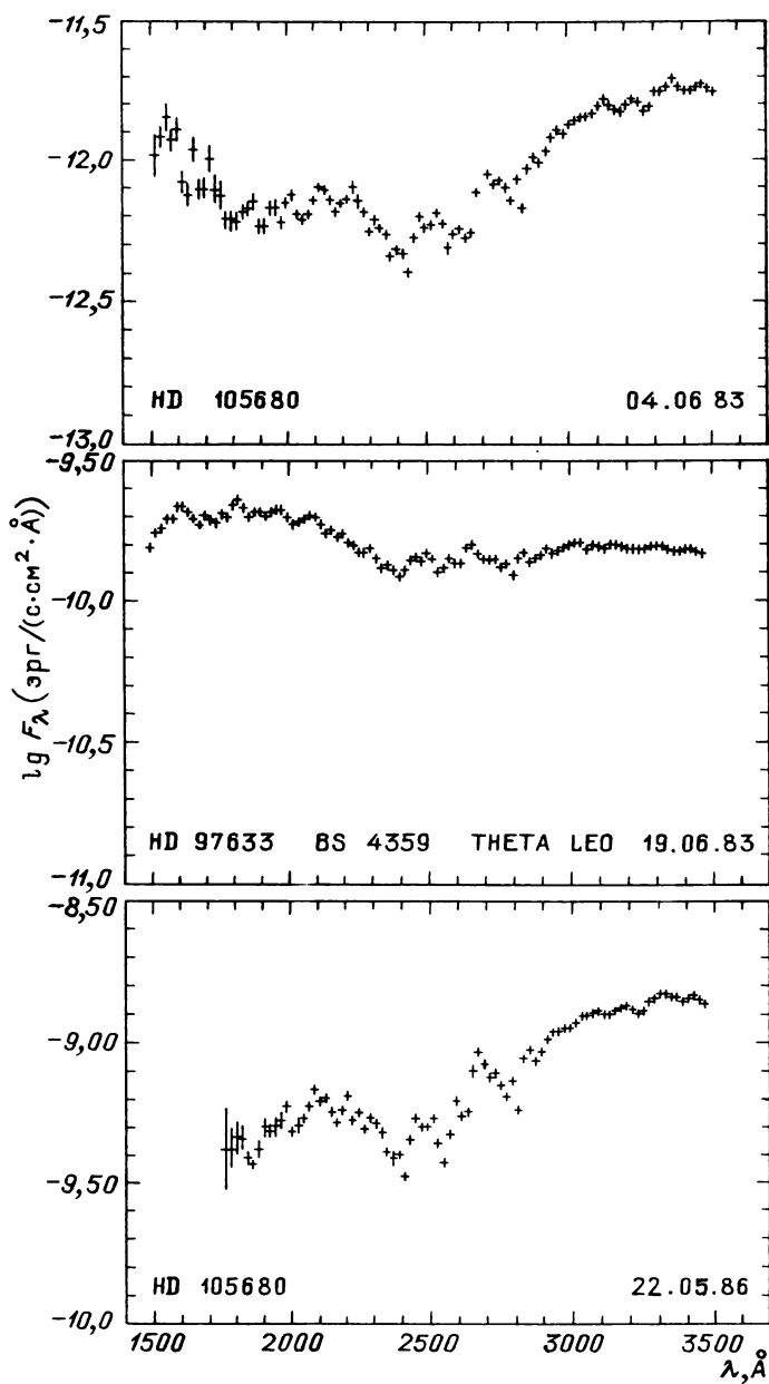
Рис. 31.15. Распределение энергии в спектрах звезд
