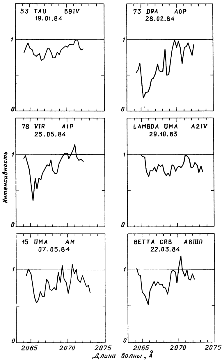
Рис. 47.15. Распределение энергии в спектрах звезд, наблюдавшихся с высоким спектральным разрешением
