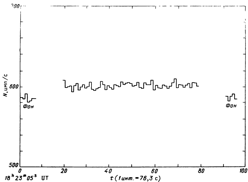
Рис. 81. Скорость счета в диапазоне 2–25 кэВ при наблюдении пульсара Her X-1 30.06.83
