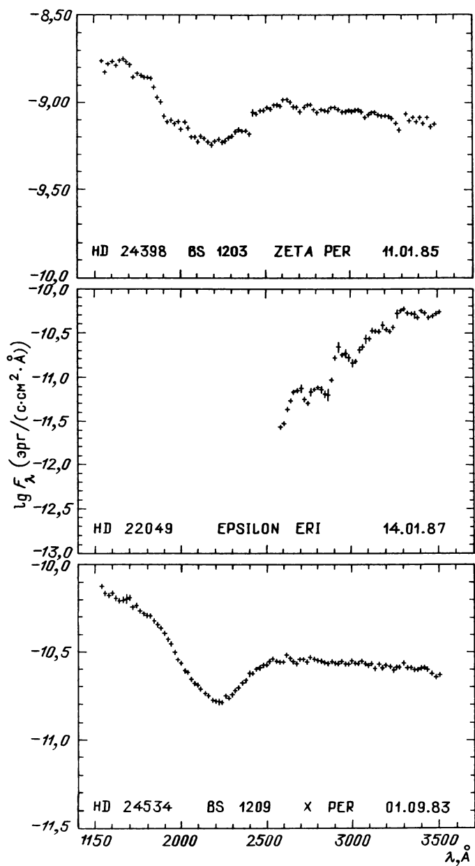
Рис. 31.3. Распределение энергии в спектрах звезд
