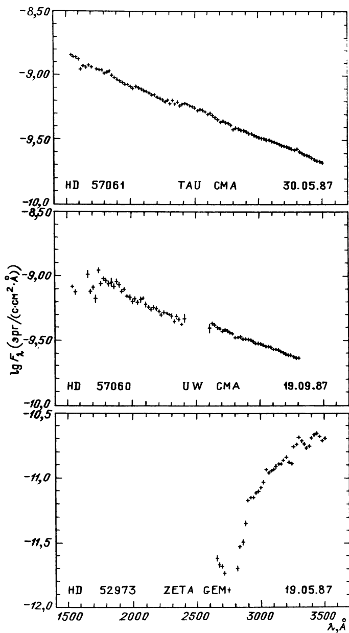
Рис. 31.9. Распределение энергии в спектрах звезд
