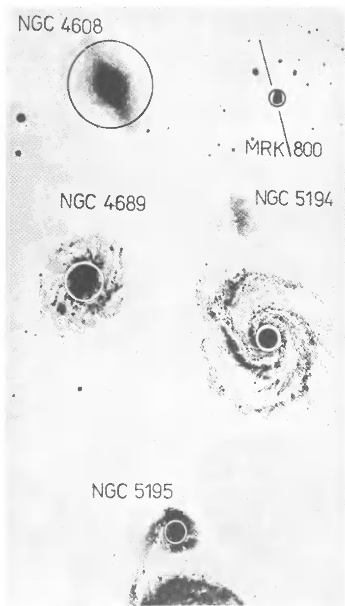
Рис. 48.2. Фотографии наблюдаемых звездных систем. Размеры диафрагмы изображены в виде колец и соответствуют данным столбца «диафрагма» табл. 10: O —офсетная, Ф —фоновая
