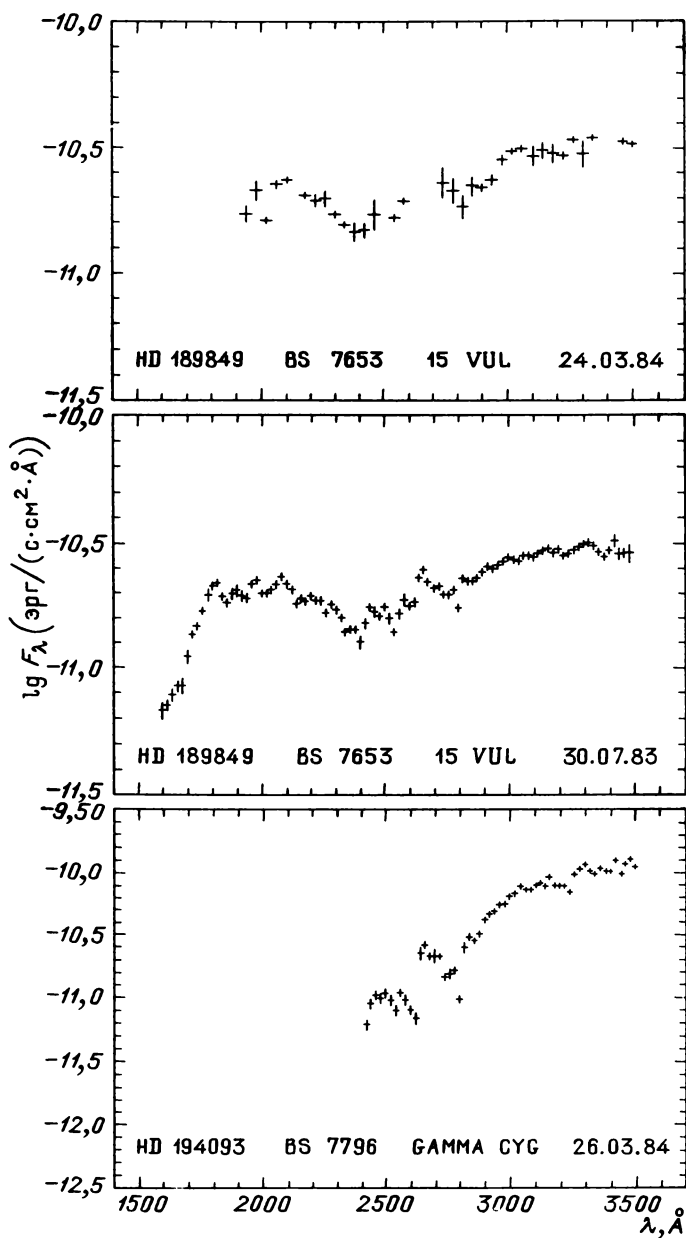
Рис. 31.35. Распределение энергии в спектрах звезд
