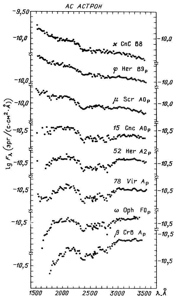
Рис. 33. Распределение энергии в спектрах нескольких магнитных звезд
