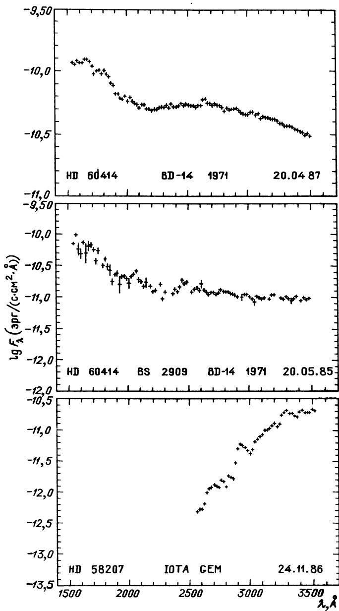
Рис. 31.10. Распределение энергии в спектрах звезд
