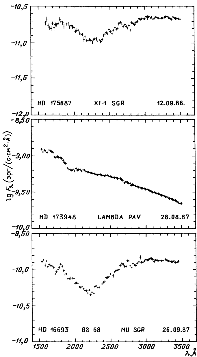
Рис. 31.33. Распределение энергии в спектрах звезд
