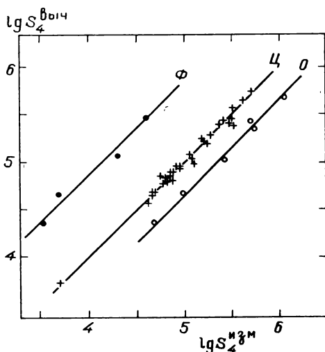
Рис. 24. Сопоставления логарифмов наблюдавшихся значений S_4 с вычисленными по формуле (2.7) с коэффициентами (2.8)
