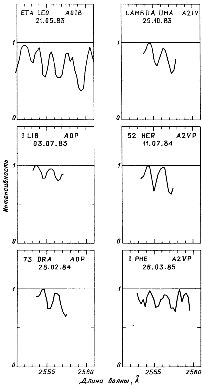
Рис. 47.25. Распределение энергии в спектрах звезд, наблюдавшихся с высоким спектральным разрешением
