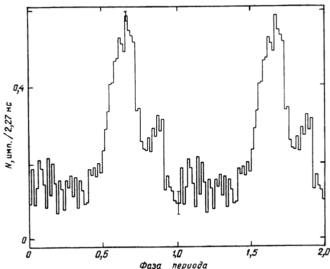
Рис. 91. Кривая блеска пульсара Her X-1 по данным 06.07.87
