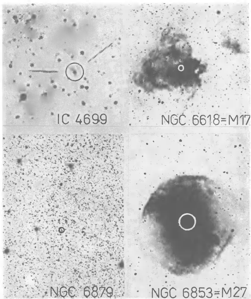
Рис. 63.4. Фотографии газовых туманностей. Размеры и положение колец соответствуют размерам и положениям диафрагм при наблюдениях
