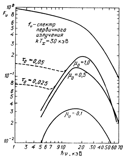
Рис. 93. Спектр рентгеновского излучения, отраженного от атмосферы нормальной звезды (сплошные линии), для различных углов падения \theta_0 = \arccos \mu_0 . Штриховые линии — спектр с учетом излучения, отраженного от внешнего высокотемпературного рассеивающего слоя (короны) с различной оптической толщиной по томсоновскому рассеянию
