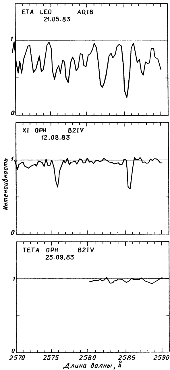
Рис. 47.12. Распределение энергии в спектрах звезд, наблюдавшихся с высоким спектральным разрешением
