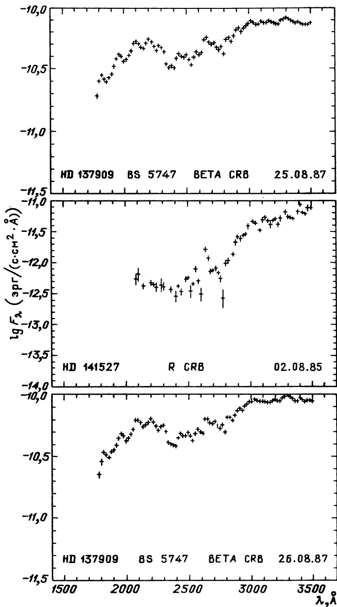
Рис. 31.22. Распределение энергии в спектрах звезд
