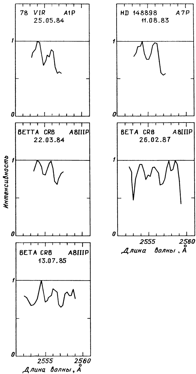
Рис. 47.26. Распределение энергии в спектрах звезд, наблюдавшихся с высоким спектральным разрешением
