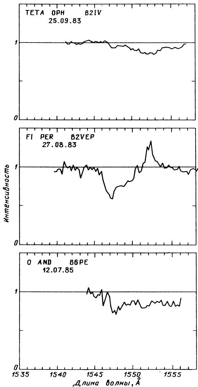
Рис. 47.5. Распределение энергии в спектрах звезд, наблюдавшихся с высоким спектральным разрешением
