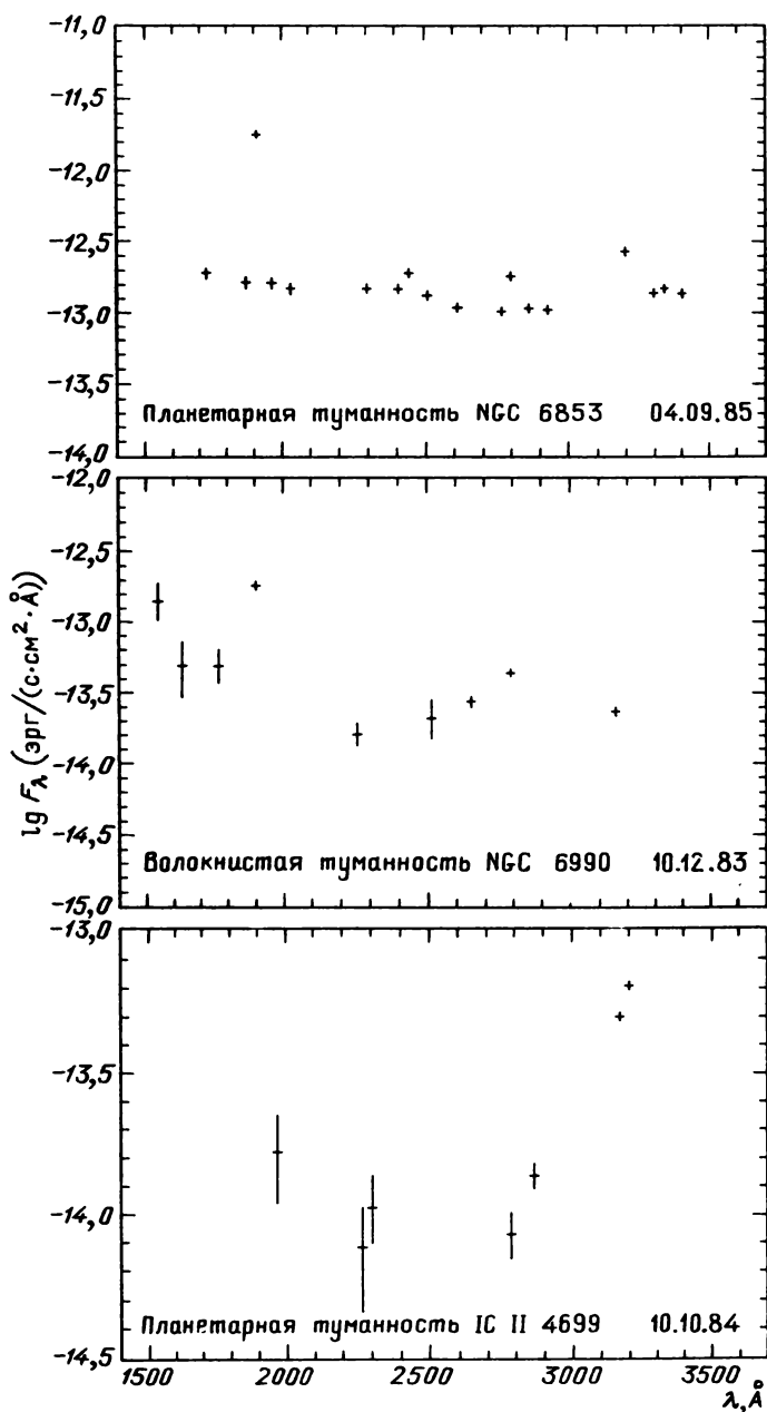
Рис. 64.7. Абсолютные значения потоков излучения газовых туманностей в полосах шириной 28 Å в интервале длин волн 1600–3500 Å
