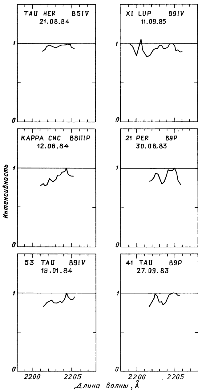
Рис. 47.16. Распределение энергии в спектрах звезд, наблюдавшихся с высоким спектральным разрешением
