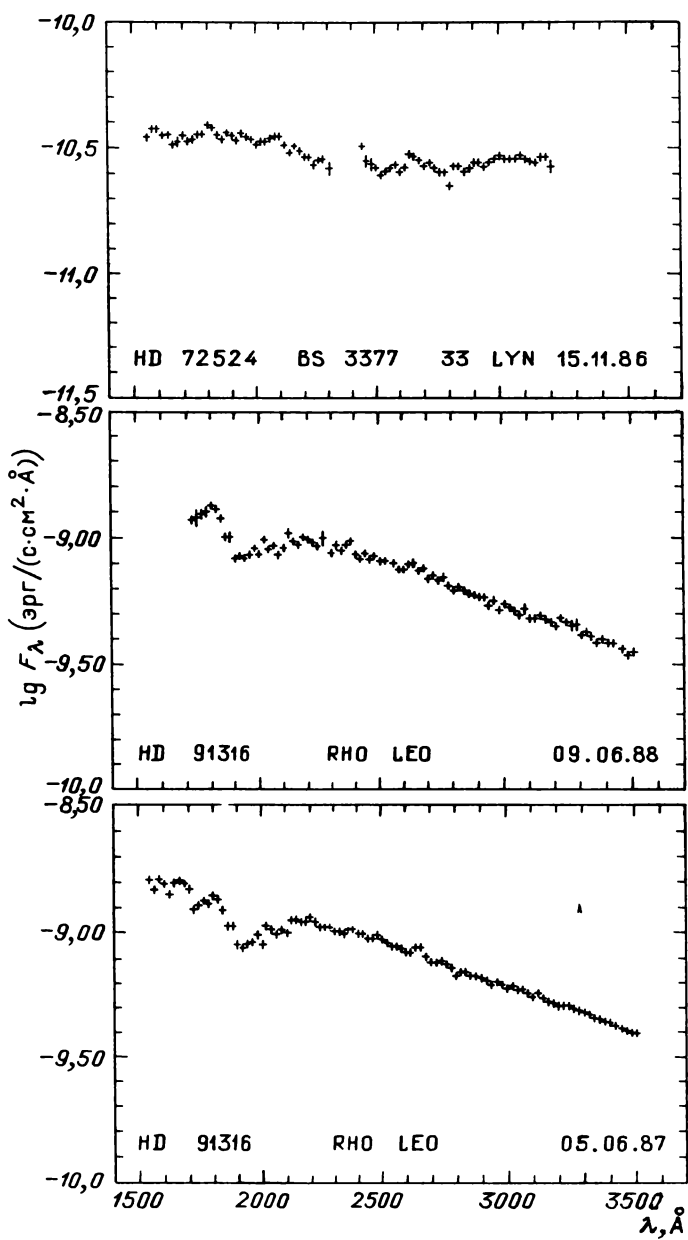
Рис. 31.14. Распределение энергии в спектрах звезд
