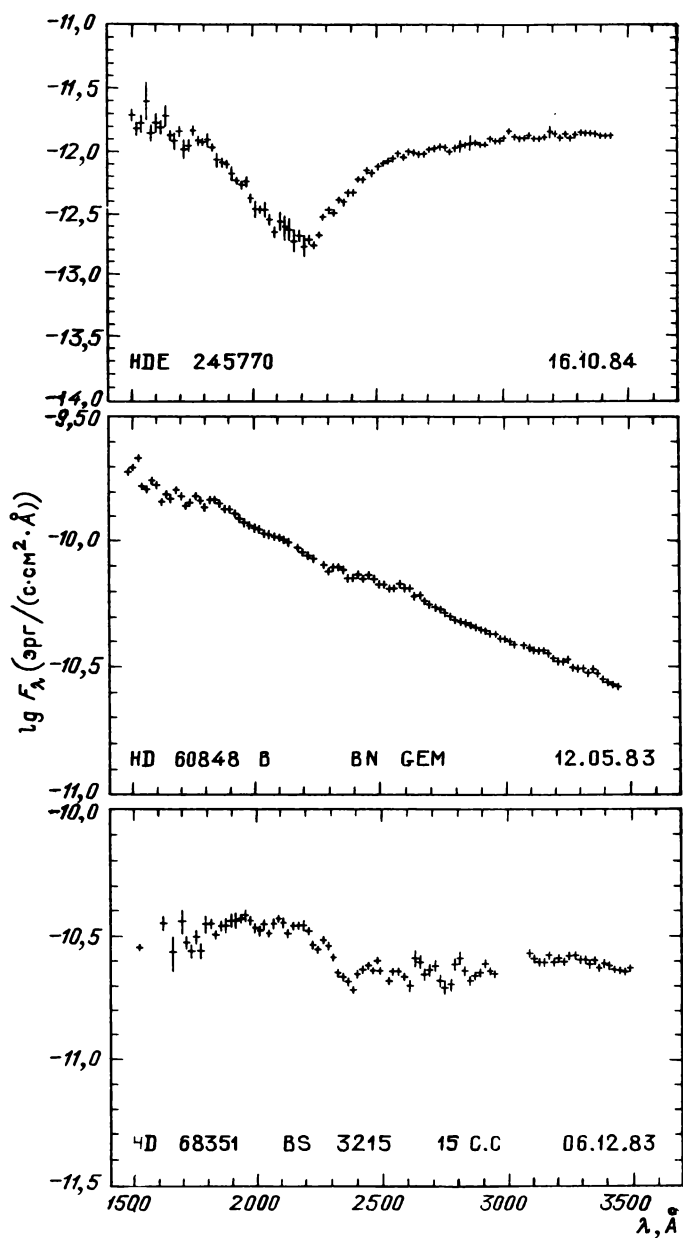
Рис. 31.11. Распределение энергии в спектрах звезд
