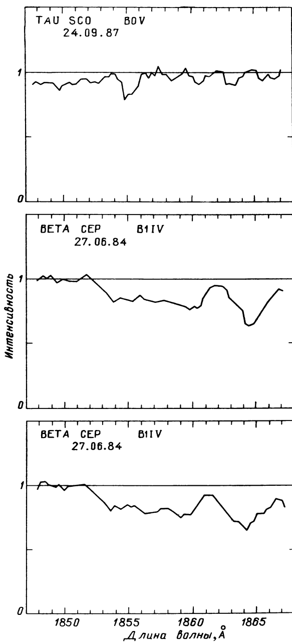
Рис. 47.8. Распределение энергии в спектрах звезд, наблюдавшихся с высоким спектральным разрешением
