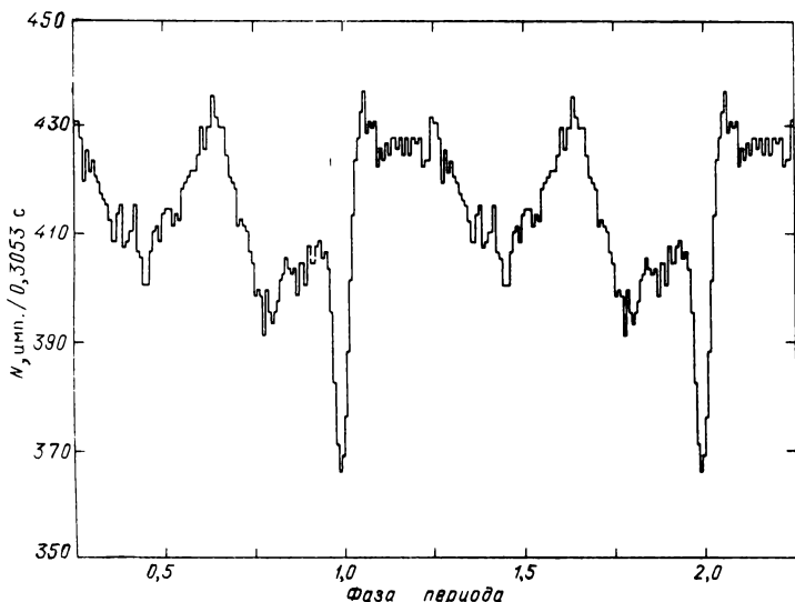
Рис. 76. Кривая блеска 104-секундного пульсара A0535+26
