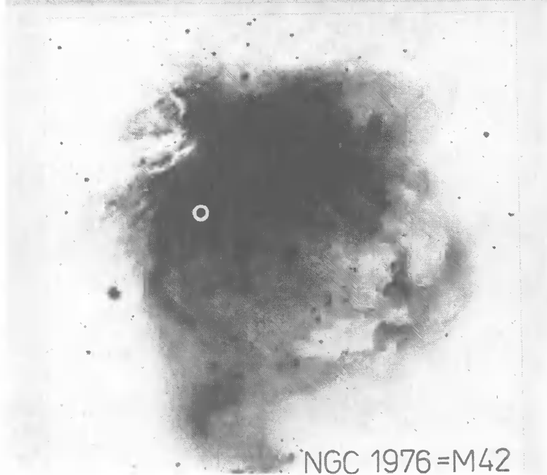
Рис. 63.1. Фотографии газовых туманностей. Размеры и положения колец соответствуют размерам и положениям диафрагм при наблюдениях
