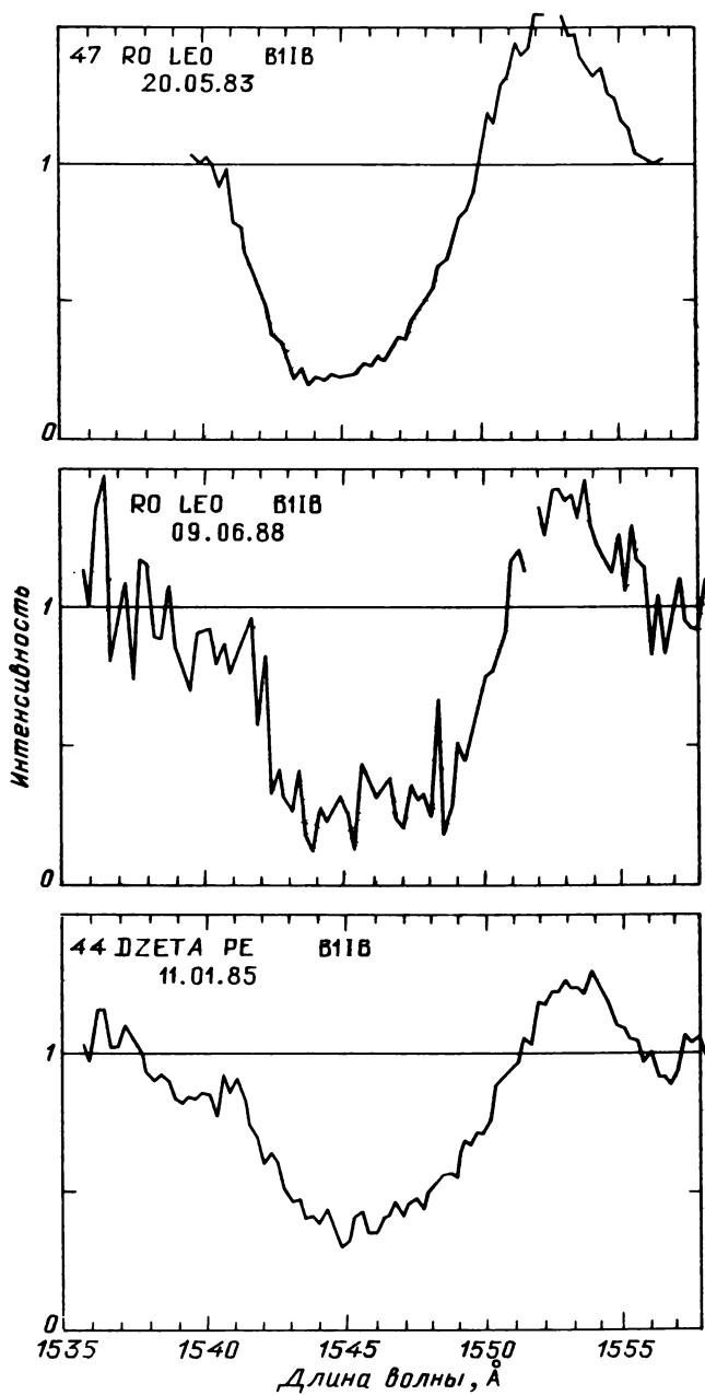
Рис. 47.2. Распределение энергии в спектрах звезд, наблюдавшихся с высоким спектральным разрешением
