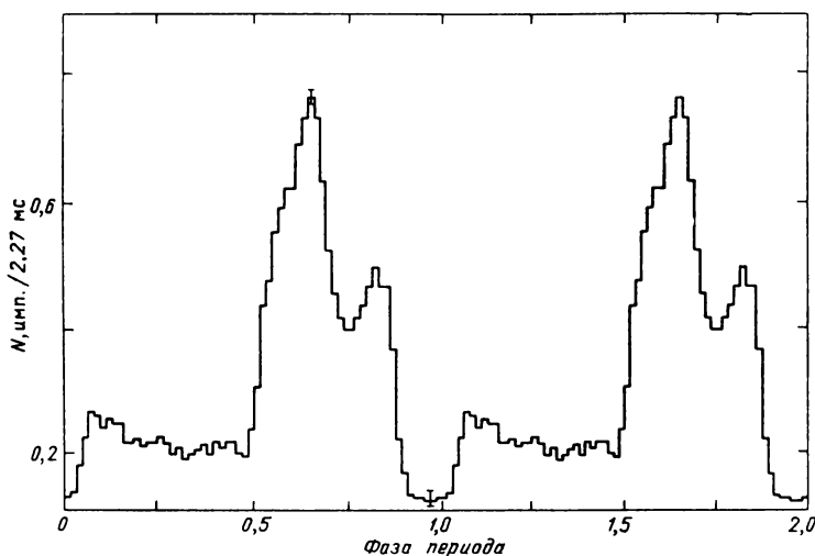
Рис. 85. Кривая блеска пульсара Her X-1 по данным 01.03.84
