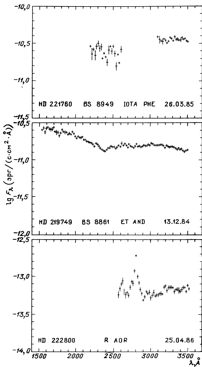
Рис. 31.39. Распределение энергии в спектрах звезд
