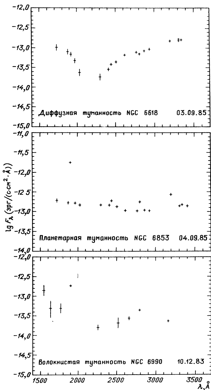
Рис. 64.4. Абсолютные значения потоков излучения газовых туманностей в полосах шириной 28 Å в интервале длин волн 1600–3500 Å
