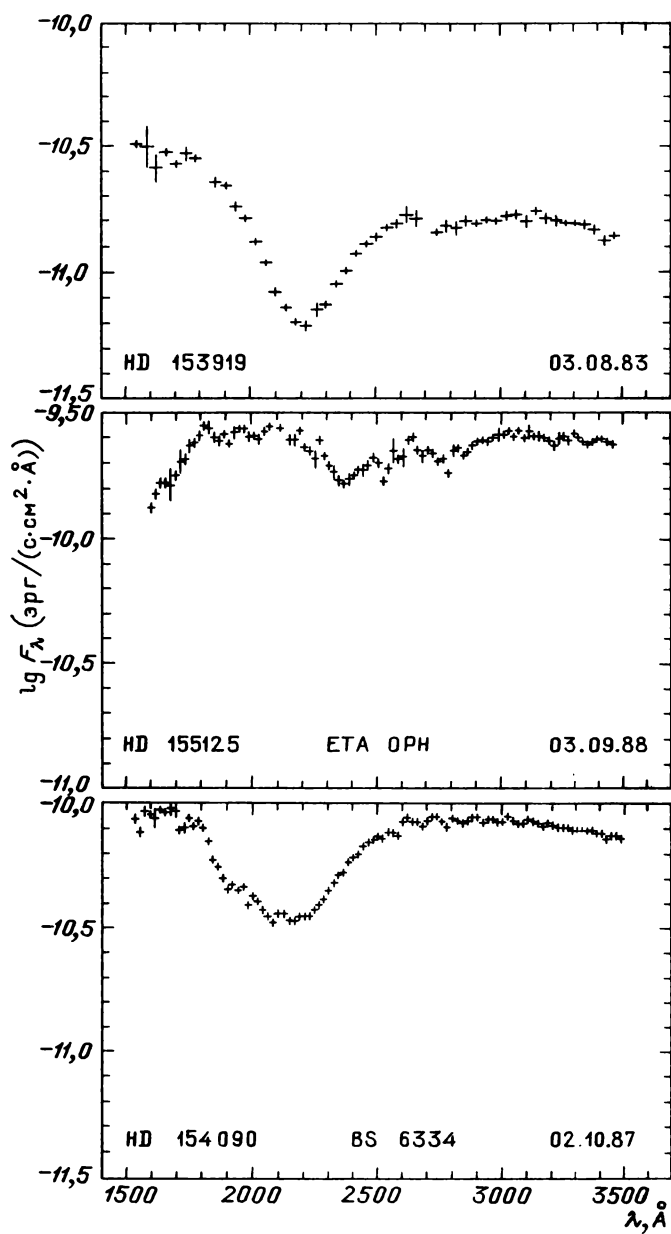
Рис. 31.30. Распределение энергии в спектрах звезд
