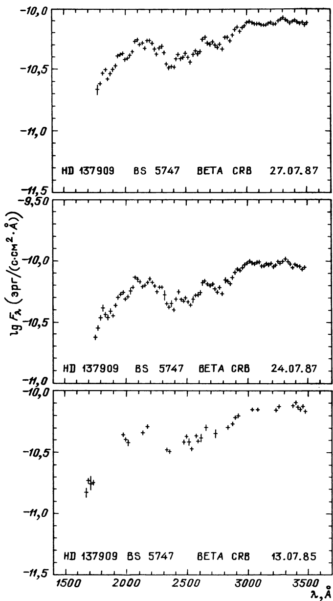
Рис. 31.20. Распределение энергии в спектрах звезд
