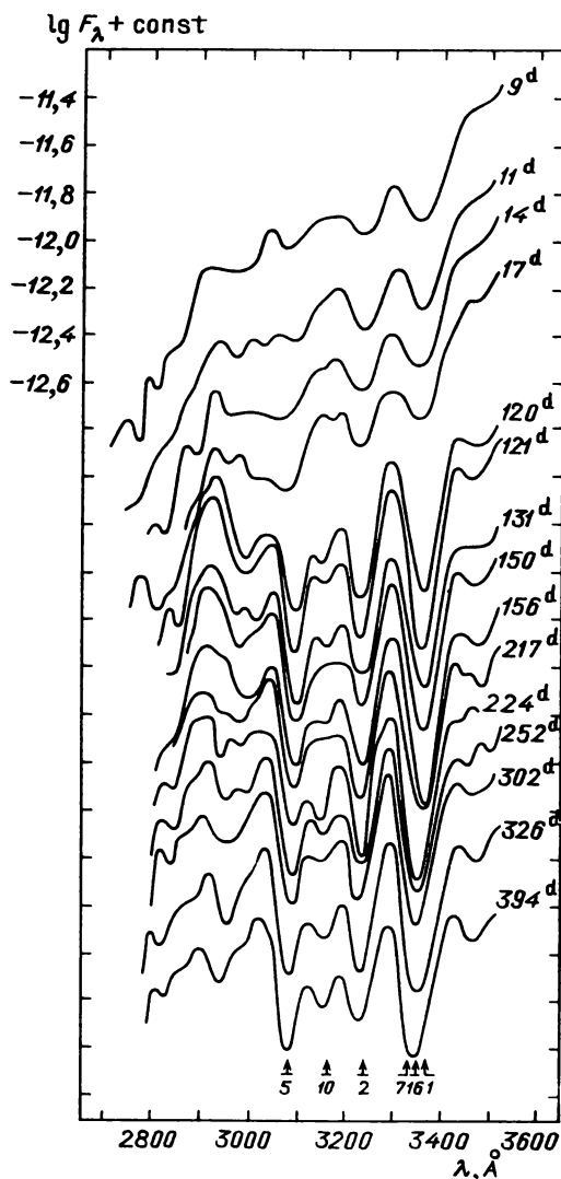
Рис. 40. Спектры SN 1987 A, смещенные вдоль обеих осей — см. текст. Стрелки с числами внизу указывают положения и номера наиболее сильных мультиплетов ионов титана
