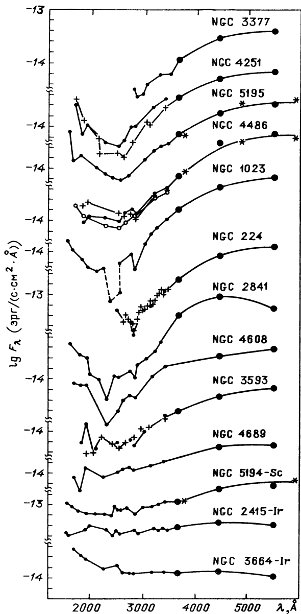
Рис. 54. Спектры галактик, в которых имеется удовлетворительная стыковка ультра-фиолетового и видимого участков
