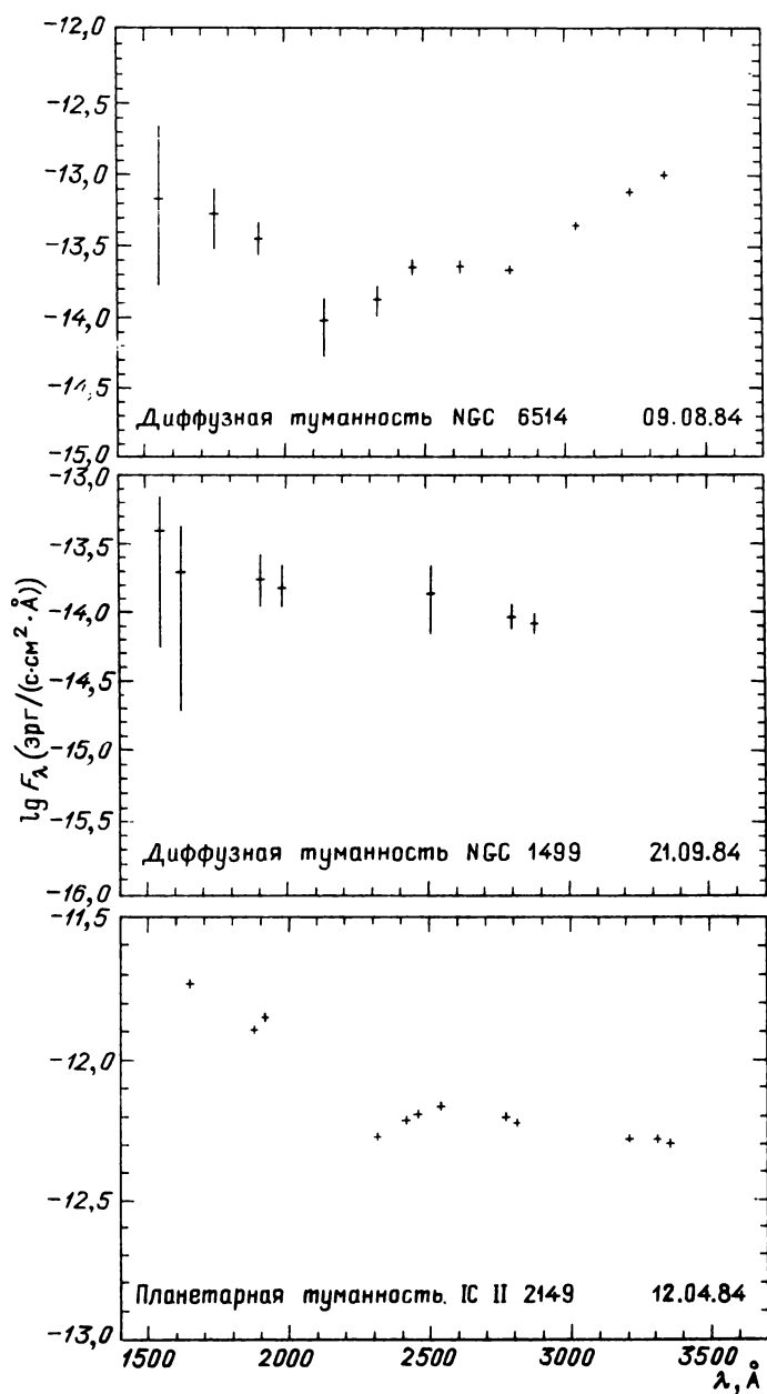
Рис. 64.2. Абсолютные значения потоков излучения газовых туманностей в полосах шириной 28 Å в интервале длин волн 1600–3500 Å
