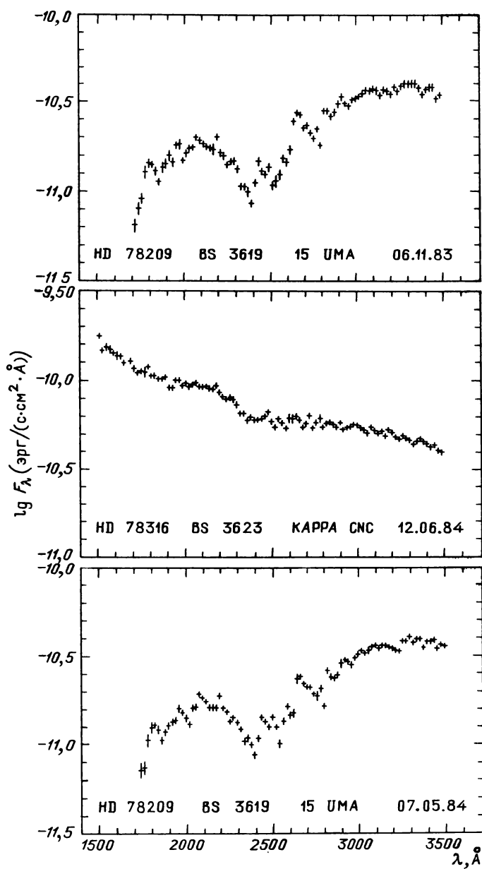
Рис. 31.12. Распределение энергии в спектрах звезд
