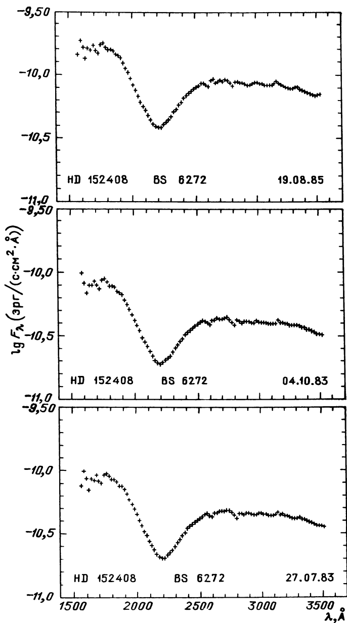
Рис. 31.29. Распределение энергии в спектрах звезд
