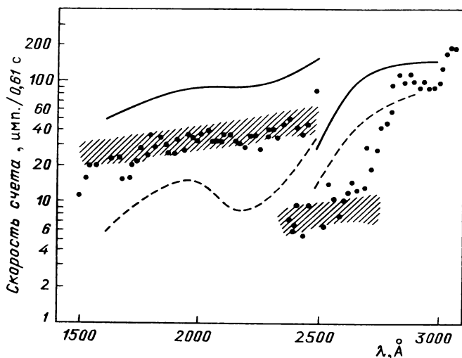
Рис. 37. Наблюдения SN 1987 A и ожидаемое излучение звезды Sk-69°202 в ультрафиолетовом диапазоне длин волн
