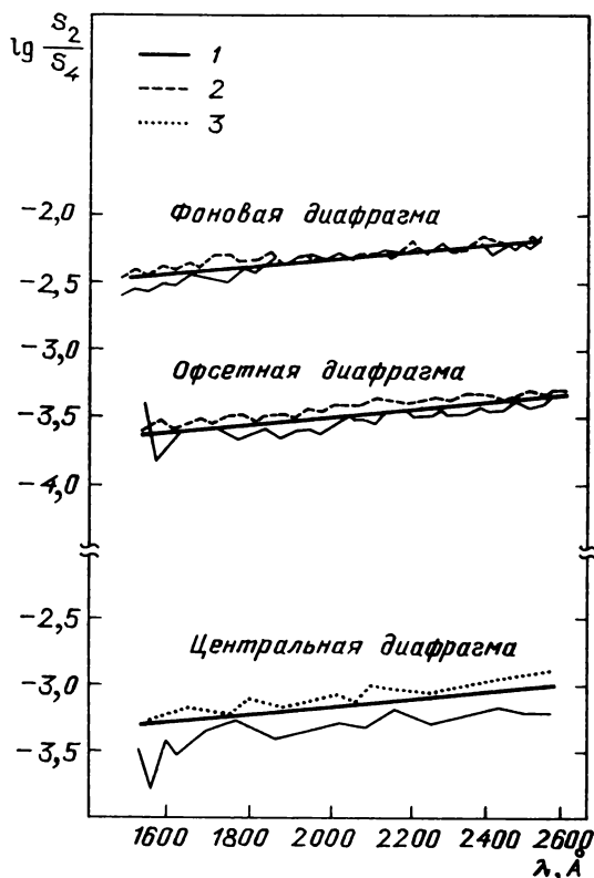
Рис. 29. Зависимость \lg(S_2 / S_4) от \lambda для следующих звезд: 1 — BS 5485 K0 (5.08.85), 2 — 65 And K3 (1.10.85), 3 — \alpha Ari (21.08.85)
