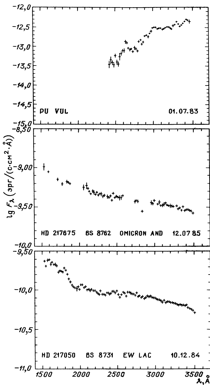
Рис. 31.38. Распределение энергии в спектрах звезд
