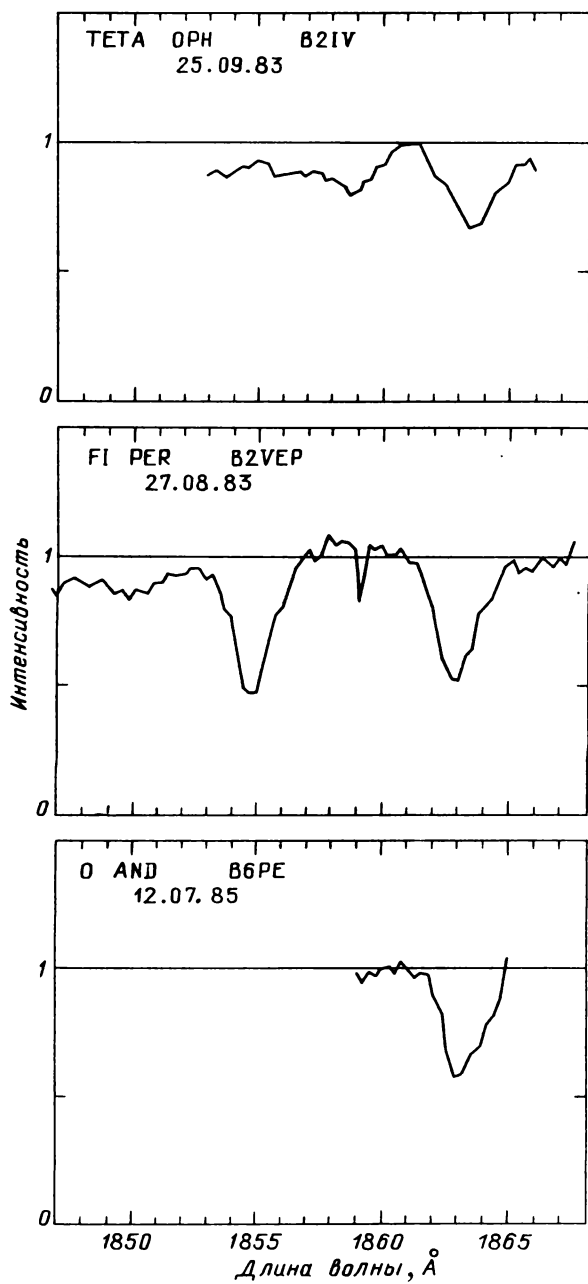
Рис. 47.9. Распределение энергии в спектрах звезд, наблюдавшихся с высоким спектральным разрешением
