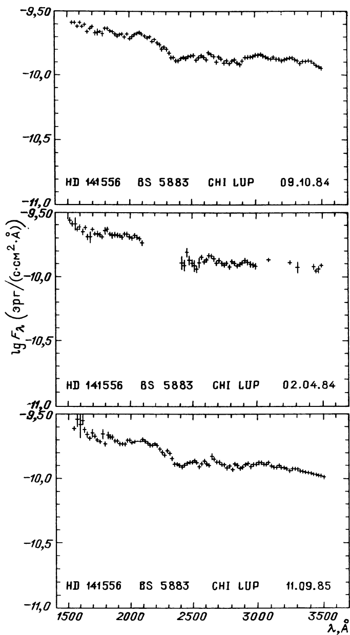
Рис. 31.23. Распределение энергии в спектрах звезд
