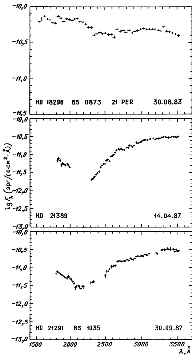
Рис. 31.2. Распределение энергии в спектрах звезд
