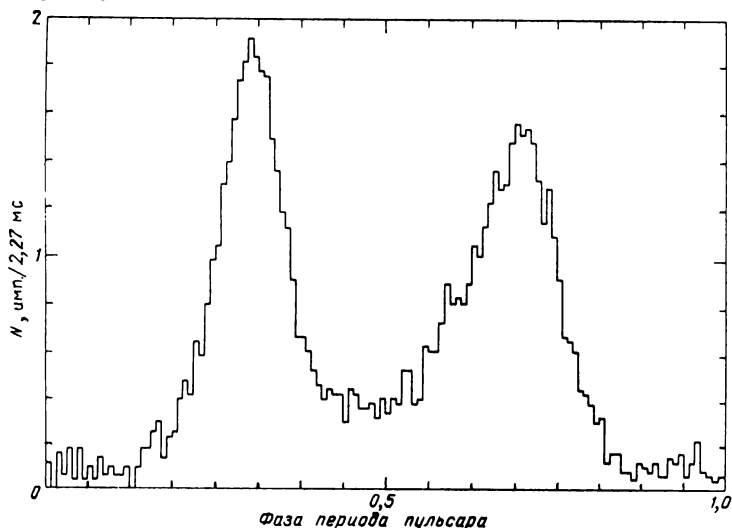
Рис. 75. Кривая блеска пульсара NP 0532 по данным АС «Астрон», полученным 16.03.84
