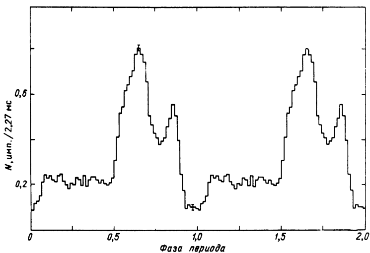
Рис. 87. Кривая блеска пульсара Her X-1 по данным 25.08.84
