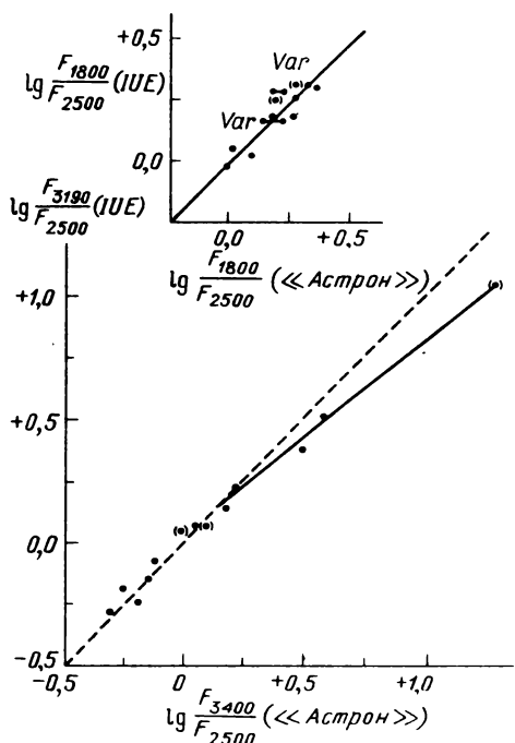
Рис. 62. Сопоставление ультрафиолетовых цветов звезд, полученных по наблюдениям на «Астроне» и на спутнике IUE
