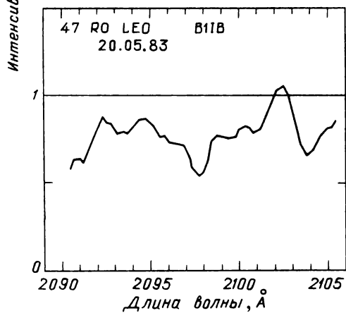
Рис. 47.13. Распределение энергии в спектрах звезд, наблюдавшихся с высоким спектральным разрешением
