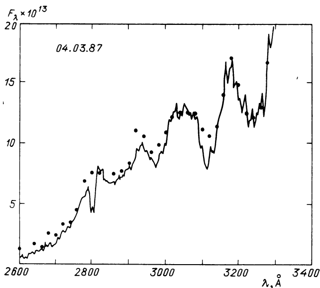
Рис. 22. Абсолютное распределение энергии в спектре Сверхновой 1987а 4 марта 1987 г., полученное по наблюдениям на IUE (сплошная линия) с разрешением 6 Å и на АС «Астрон» (точки) с разрешением 31 Å и с использованием фоновой диафрагмы
