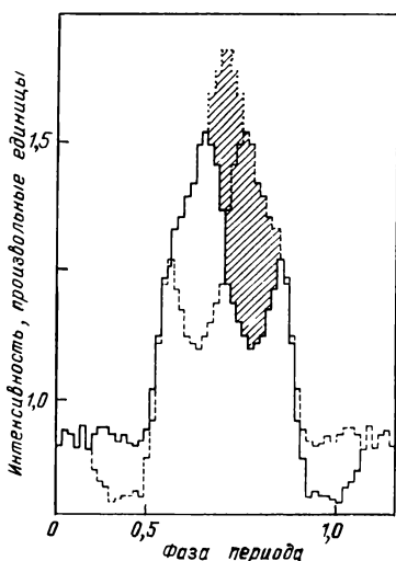
Рис. 95. Вид главного импульса на кривой блеска пульсара Her X-1 (сплошная линия — наблюдения 25.08.84) с наложенным зеркальным изображением импульса (штриховая линия). Точками показана возможная вершина незатененного главного импульса. Заштрихованная площадь — затененная часть главного импульса
