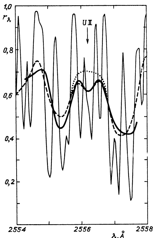
Рис. 36. Сравнение наблюдаемого и теоретического спектров Ар-звезды 73 Dra в области линии U II \lambda 2556,19 . Толстая кривая — наблюдаемый спектр, остальные кривые — теоретический спектр (штриховая — при lg \epsilon(U) = 4,4 ; пунктирная — при lg \epsilon(U) = 0,6 ; тонкая сплошная — без учета инструментального профиля, но с вращением)
