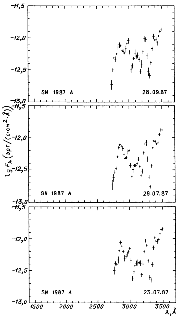
Рис. 31.43. Распределение энергии в спектрах звезд
