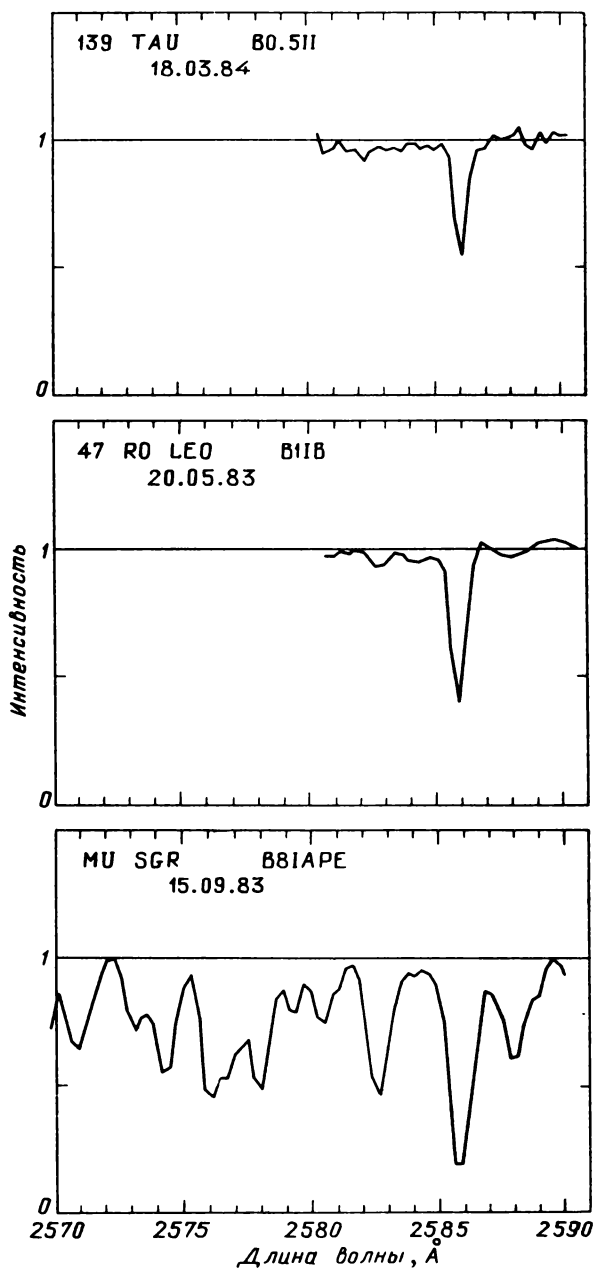
Рис. 47.11. Распределение энергии в спектрах звезд, наблюдавшихся с высоким спектральным разрешением
