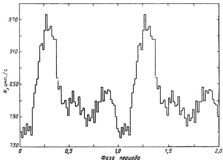
Рис. 80. Кривая блеска пульсара Сеп X-3, полученная 23.05.85
