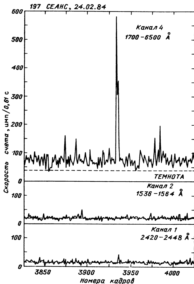
Рис. 45. Вспышка EV Лас 24.02.84. Наблюдения на «Астроне»
