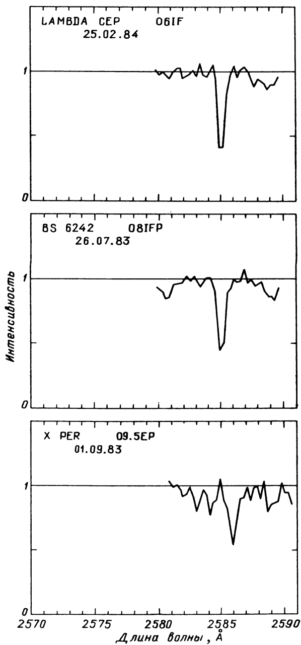
Рис. 47.10. Распределение энергии в спектрах звезд, наблюдавшихся с высоким спектральным разрешением
