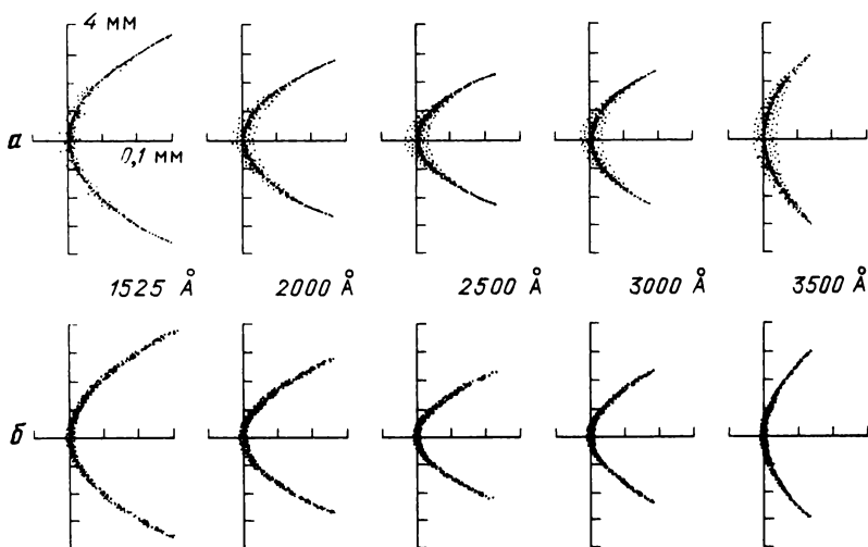
Рис. 16. Структура изображения спектральных линий, даваемых тороидальной вогнутой дифракционной решеткой: а — на круге Роуланда, б — вне круга Роуланда на расстоянии 0,2 мм
