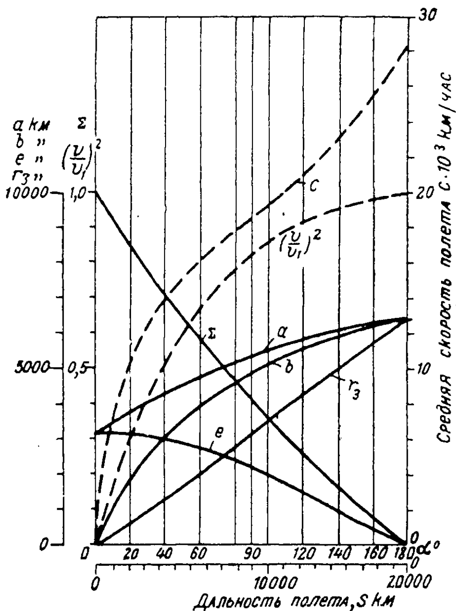
Фиг. 35. Элементы эллиптического пути далеко летящей ракеты.
