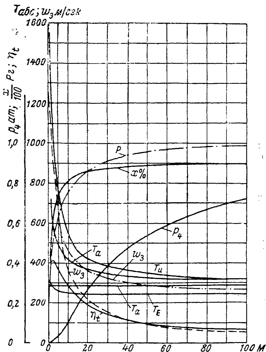
Фиг. 24. Диаграммы к воздушному реактивному двигателю с отдельными циклами.
