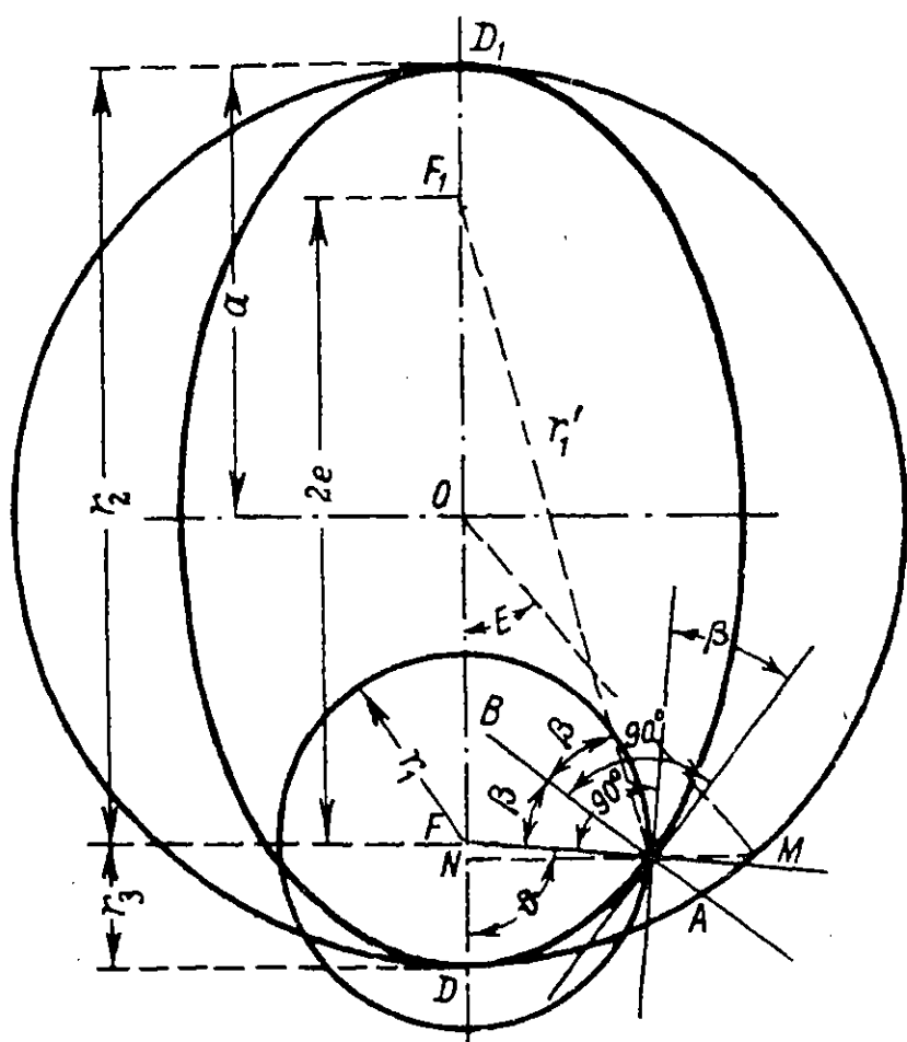
Фиг. 38. К расчету пути далеко летающих ракет.
