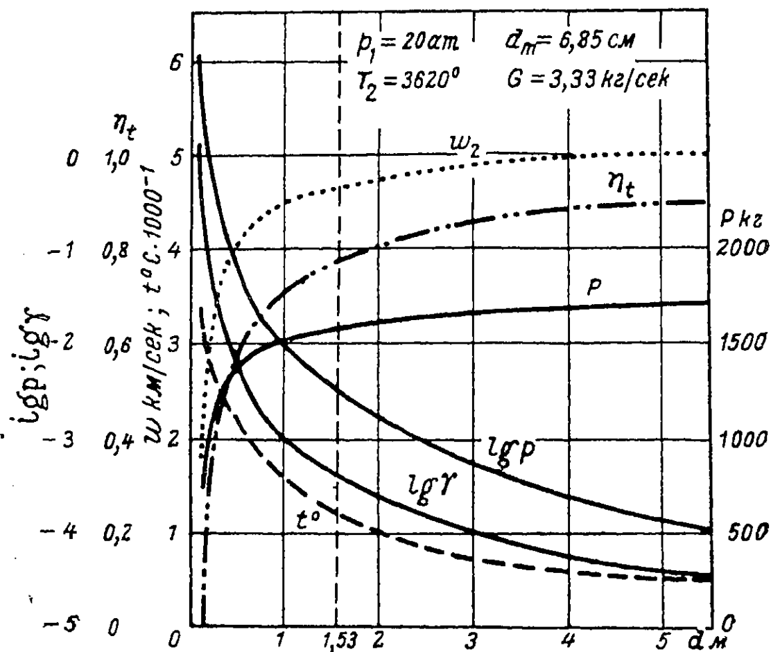
Фиг. 11. Диаграмма состояния и действия газов в водородо-кислородной ракете.
