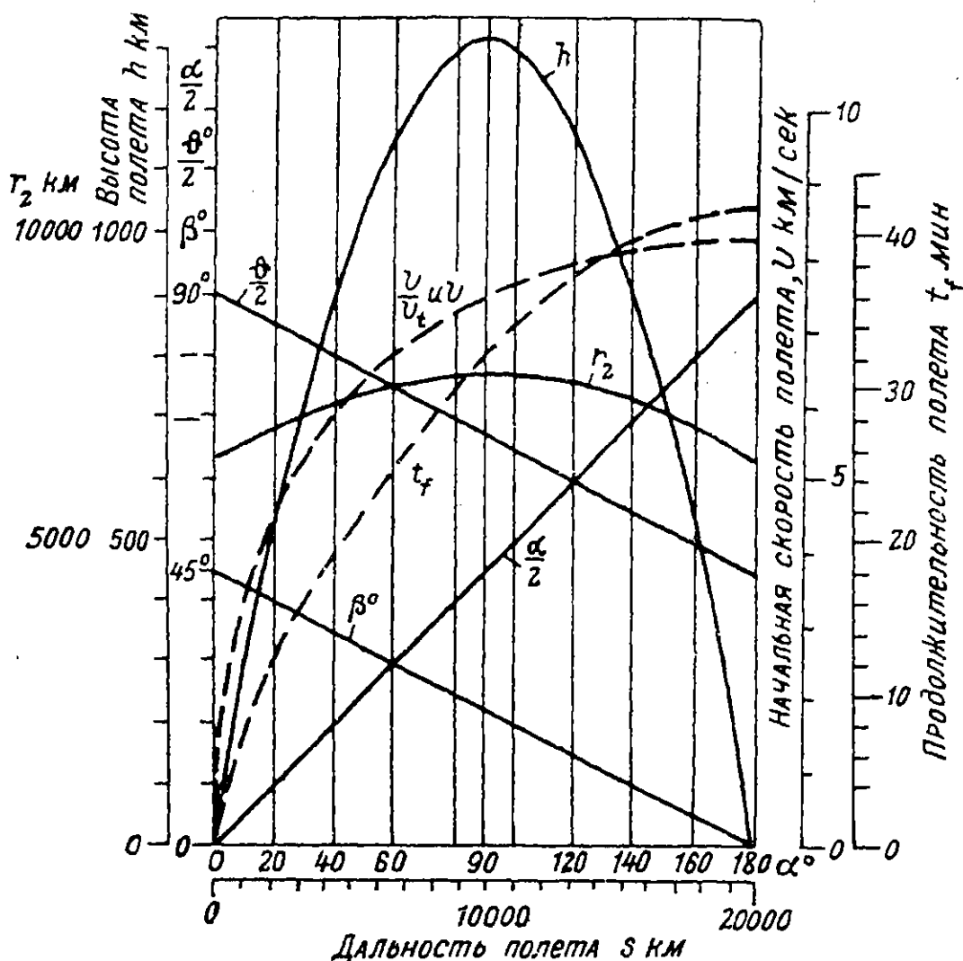
Фиг. 36. Элементы эллиптического пути далеко летающей ракеты.
