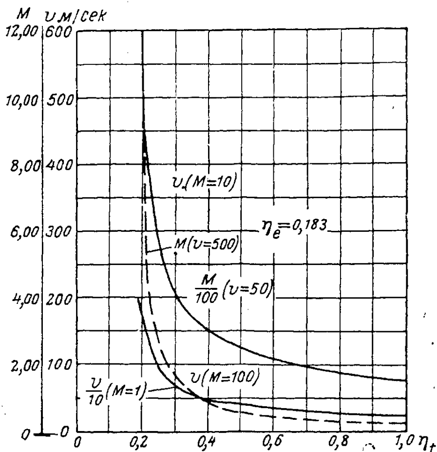
Фиг. 26. Сравнение воздушного реактивного двигателя с двигателем внутреннего сгорания.
