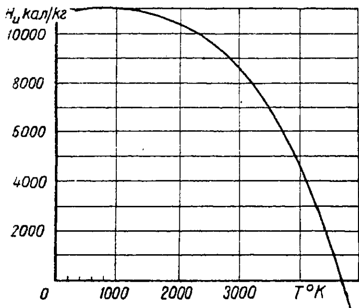
Фиг. 2. Изменение теплотворной способности бензина H_u в зависимости от изменения абсолютной температуры бензина T .
