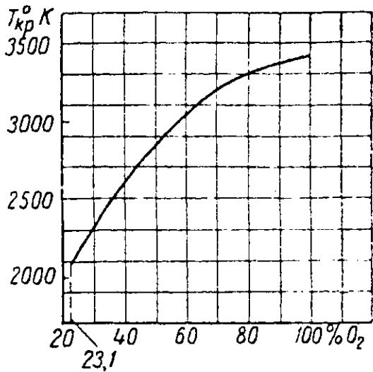
Фиг. 6. Критическая температура в зависимости от содержания кислорода в воздухе.
