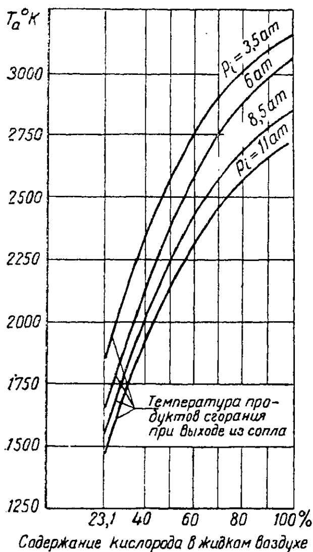
Фиг. 9. Изменение температуры продуктов сгорания у выхода из сопла в зависимости от давления в камере.
