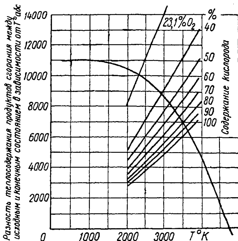
Фиг. 3. Определение температуры сгорания бензина в воздухе, обогащенном кислородом, с учетом диссоциации.
