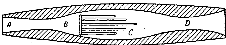
Фиг. 1. Схема воздушного реактивного двигателя Лорена.
