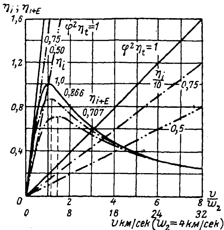
Фиг. 18. Мгновенный к. п. д. реактивного двигателя, работающего лишь продуктами сгорания, при разных скоростях полета.
