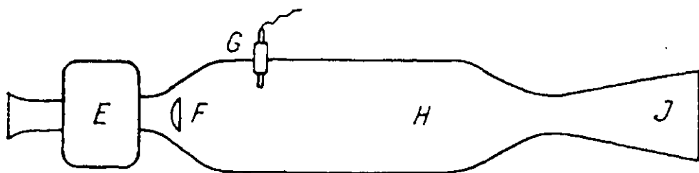
Фиг. 3. Схема воздушного реактивного двигателя непостоянного горения.
