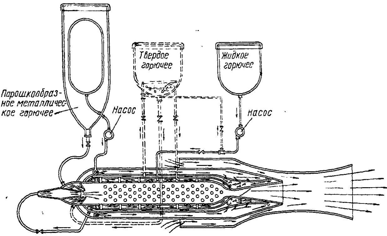
Схема двигателя на твердом горючем.
