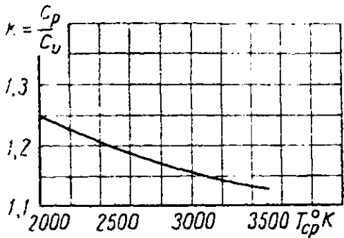
Фиг. 5. Изменение показателя степени адиабаты в зависимости от температуры.
