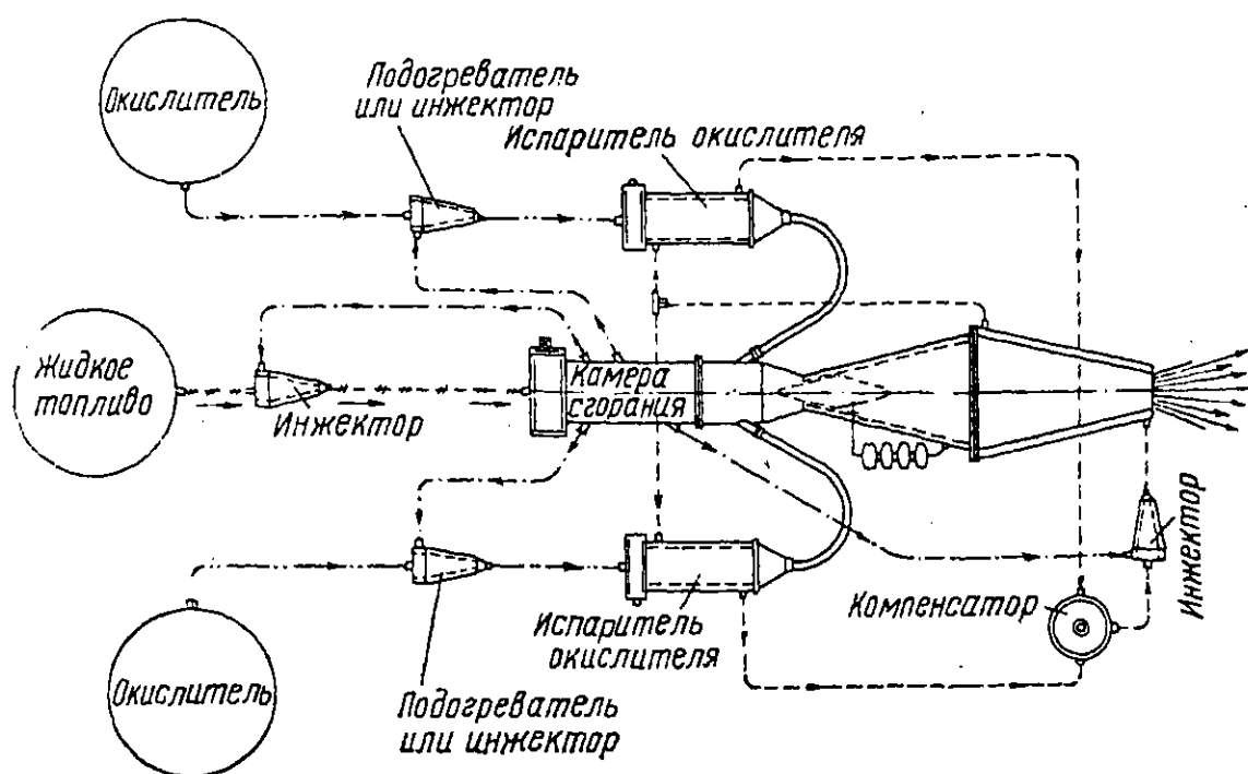
Схема второго варианта реактивного двигателя на 5 т.
