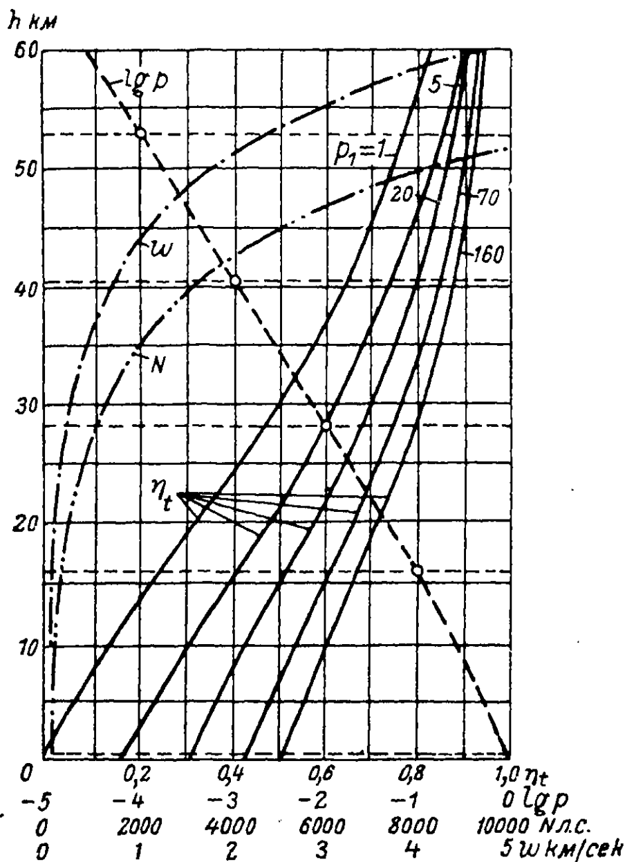
Фиг. 15. Влияние высоты полета на термический к. п. д. ракеты, скорость полета и мощность реактивного двигателя.
