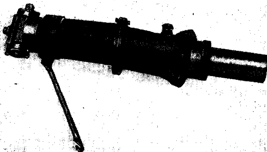
Камеры сгорания ОР-2 с соплом и жиклером.
