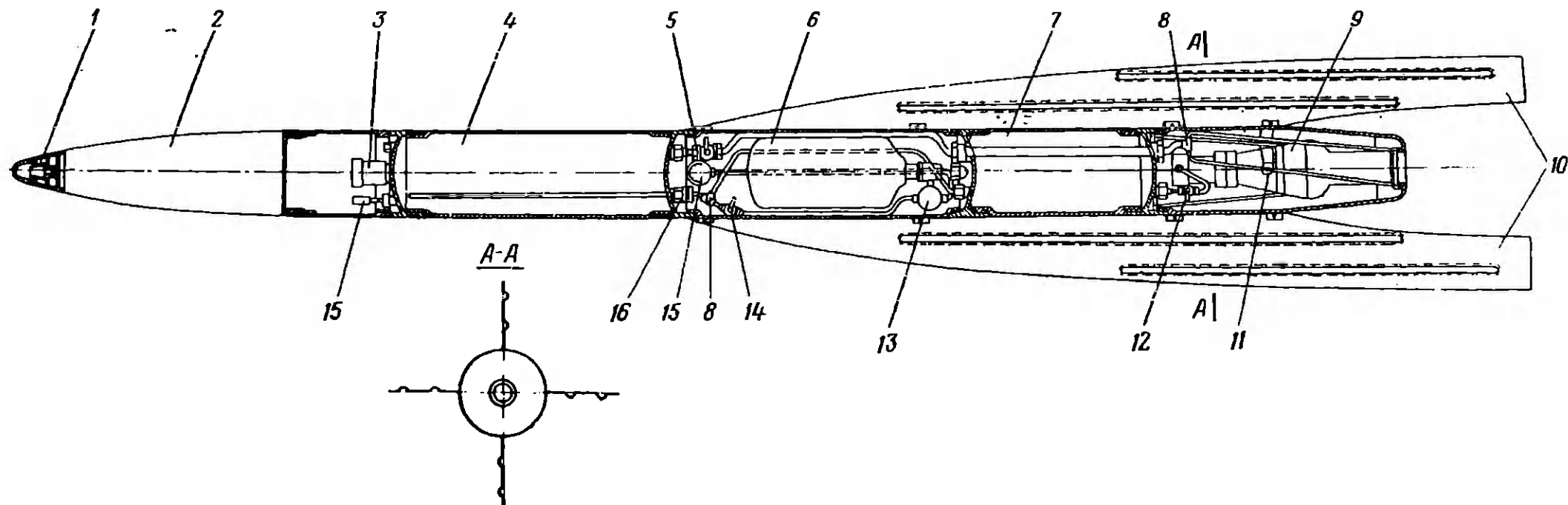
Схема ракеты ГИРД-Х.
