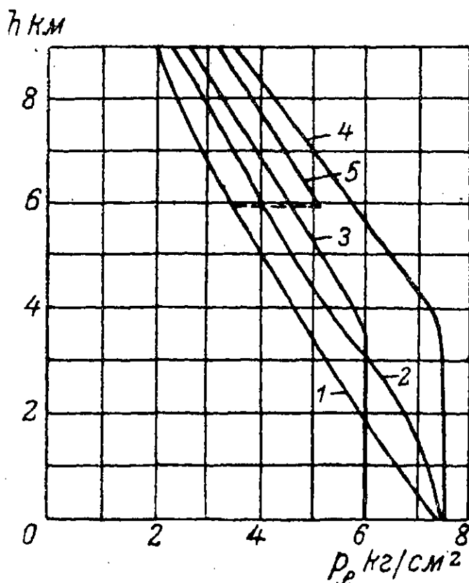
Фиг. 7. Среднее эффективное давление высотных двигателей до высоты 9 км.
