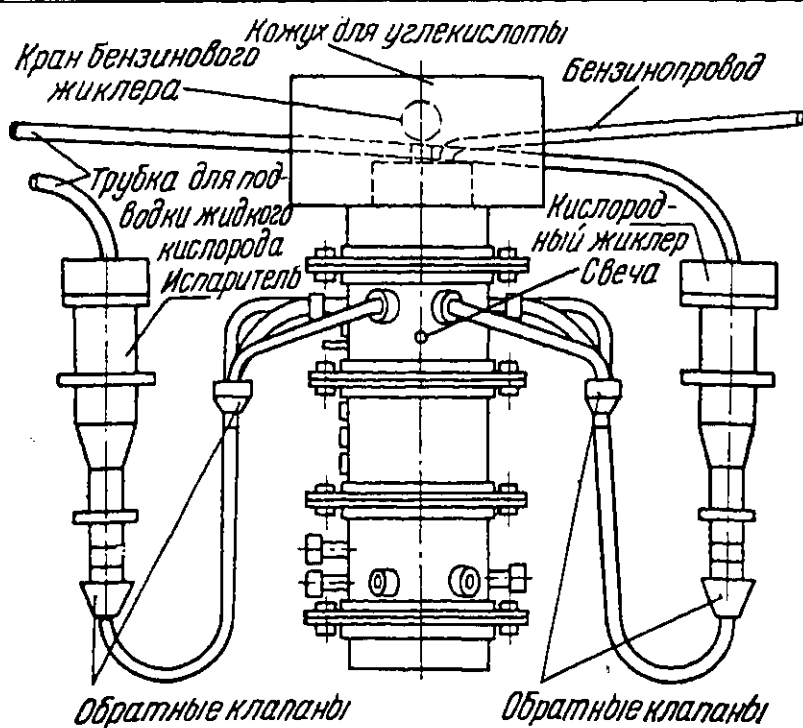
Схема огневой части двигателя ОР-2.
