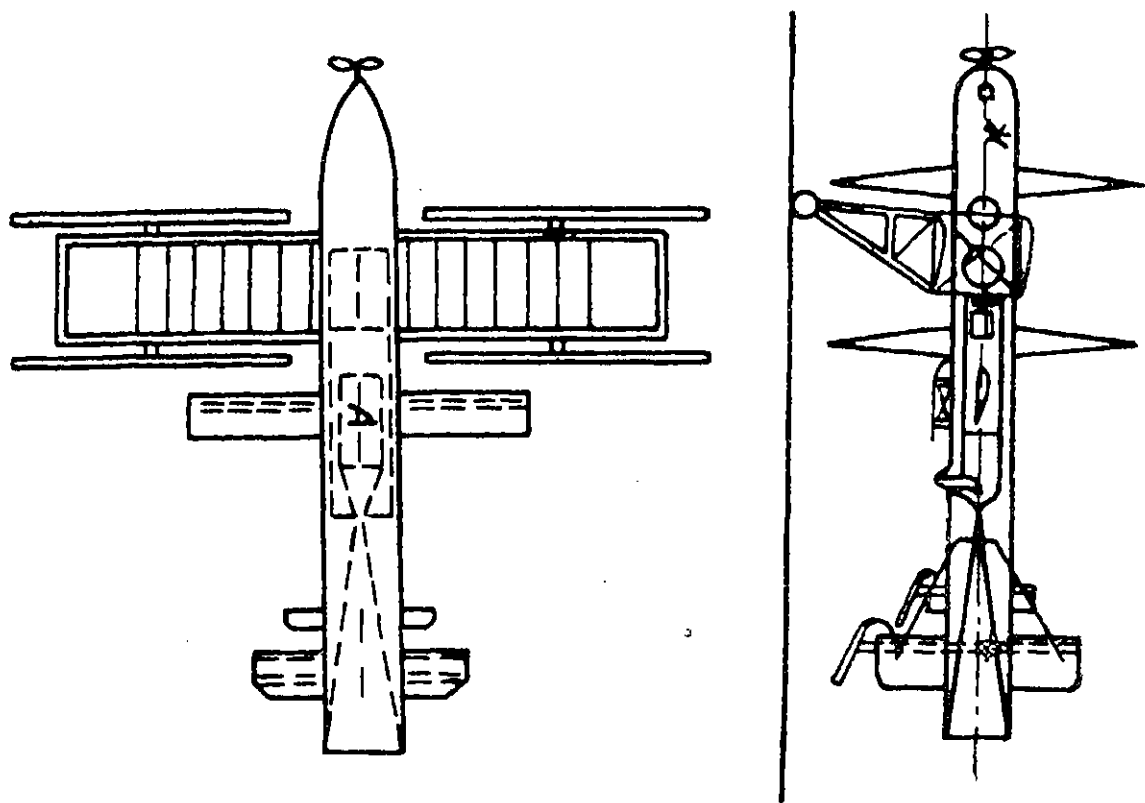
Фиг. 28. Схема аэроплана, приводимого в движение двигателем и ракетой со втягиваемыми частями.
