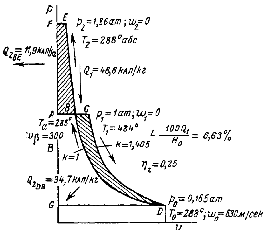
Фиг. 8. Диаграмма R струйного нагнетателя; сжатие воздуха до p_2 = 1,86 ат.
