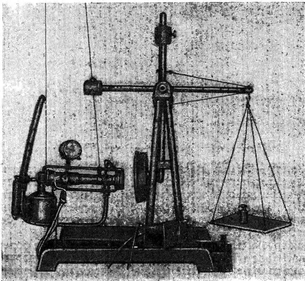
Двигатель ОР-1, подвешенный на двух проволочках, и весы для измерения тяги.
