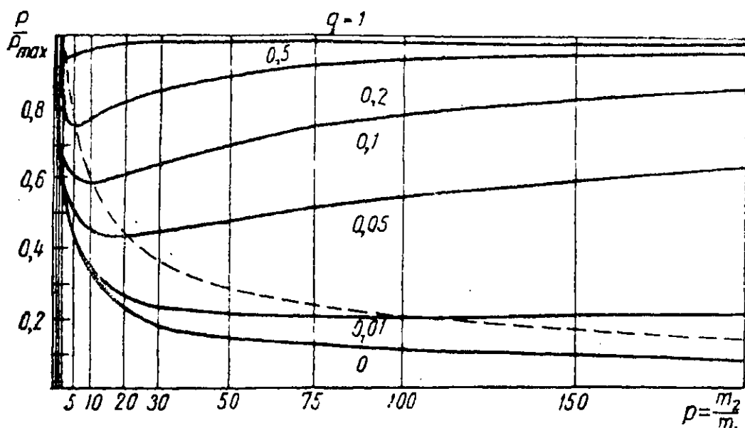
Фиг. 1. Отношение фактической силы реакции струи к теоретической максимальной силе, получающейся при выравнивании скоростей, в зависимости от отношения масс.
