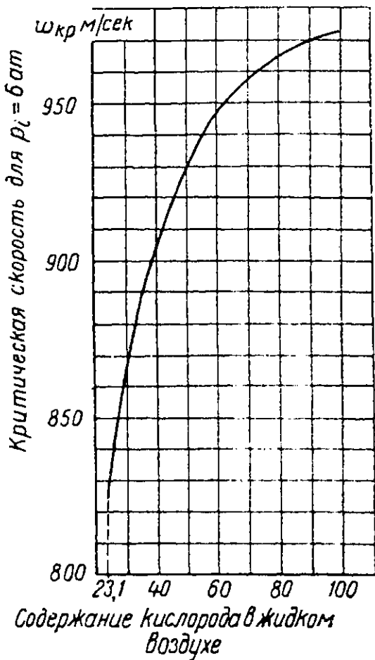
Фиг. 8. Критическая скорость продуктов сгорания в зависимости от содержания кислорода в воздухе.
