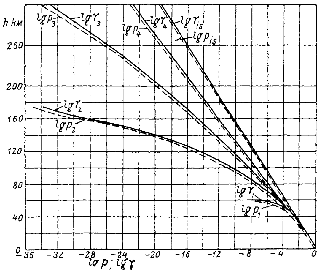
Фиг. 2. Логарифмы давления ( \gamma кг/м 3 ) и плотности ( P ат) атмосферы до высоты 300 км.
