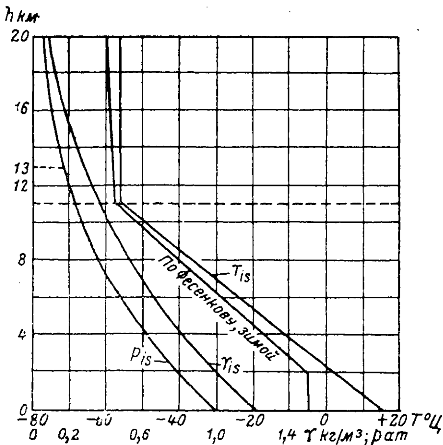
Фиг. 1. Температура, давление и плотность атмосферы до высоты 20 км.
