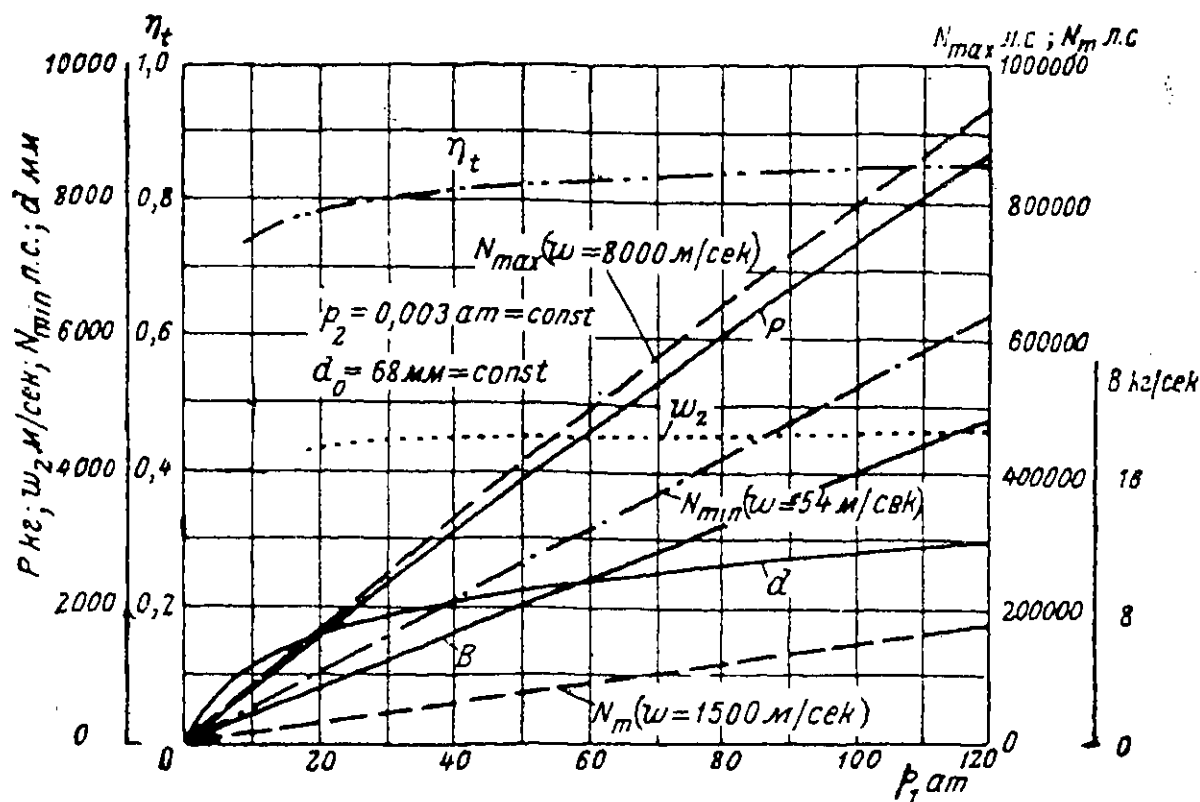
Фиг. 12. Изменение действия ракеты при переменном начальном давлении.
