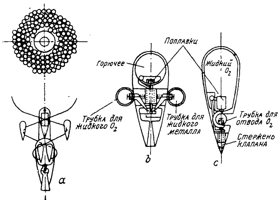
Фиг. 29. Схема одной центральной ракеты со многими боковыми ракетами и сосудами для жидкого горючего и кислорода.
