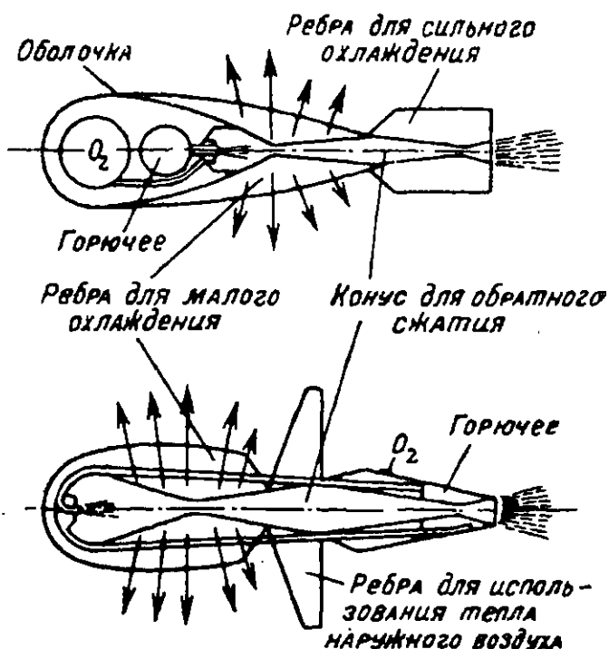
Фиг. 17. Две схемы реактивных двигателей, улучшенных рабочим циклом.
