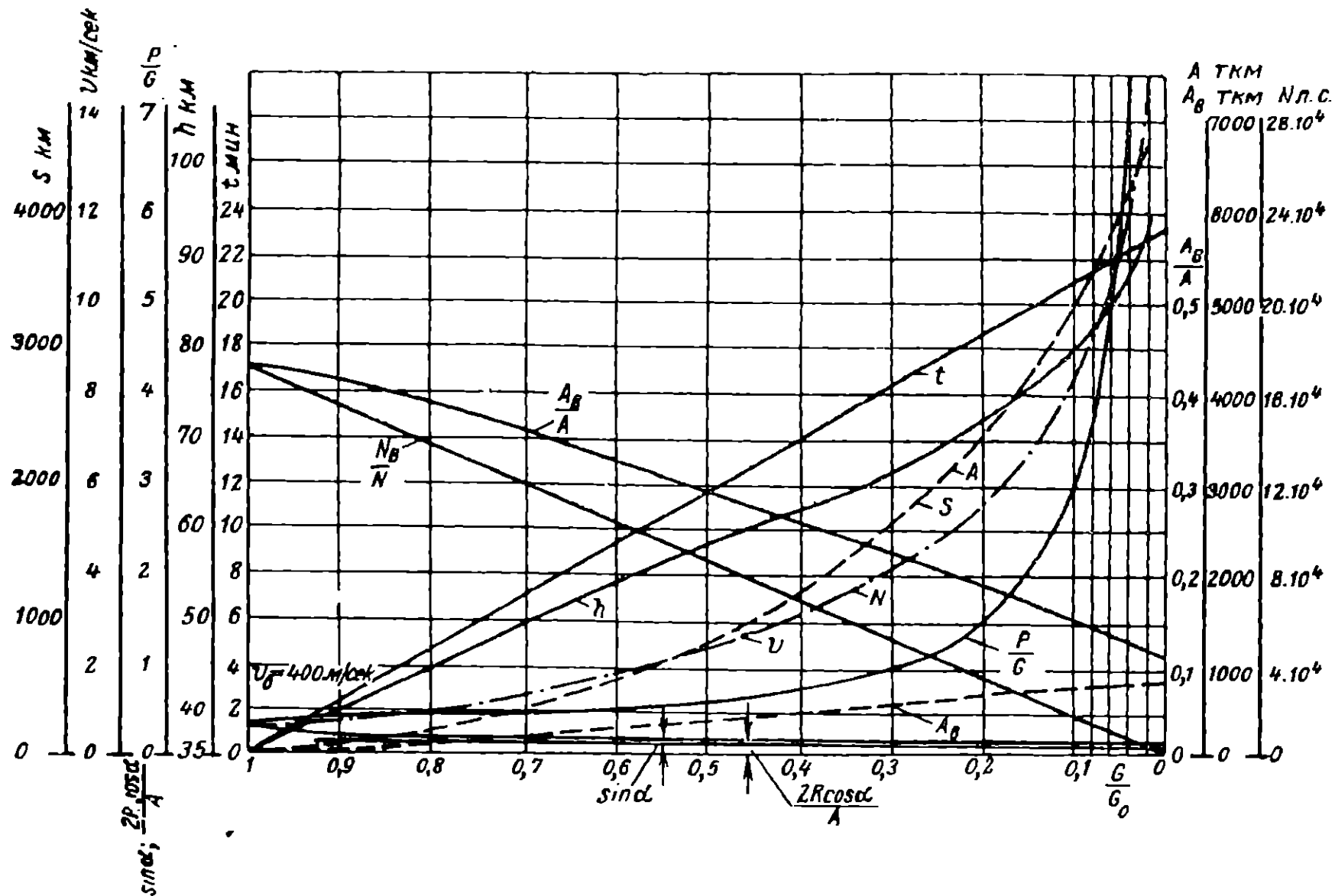
Фиг. 30. Кривые полета ракетного аэроплана.
