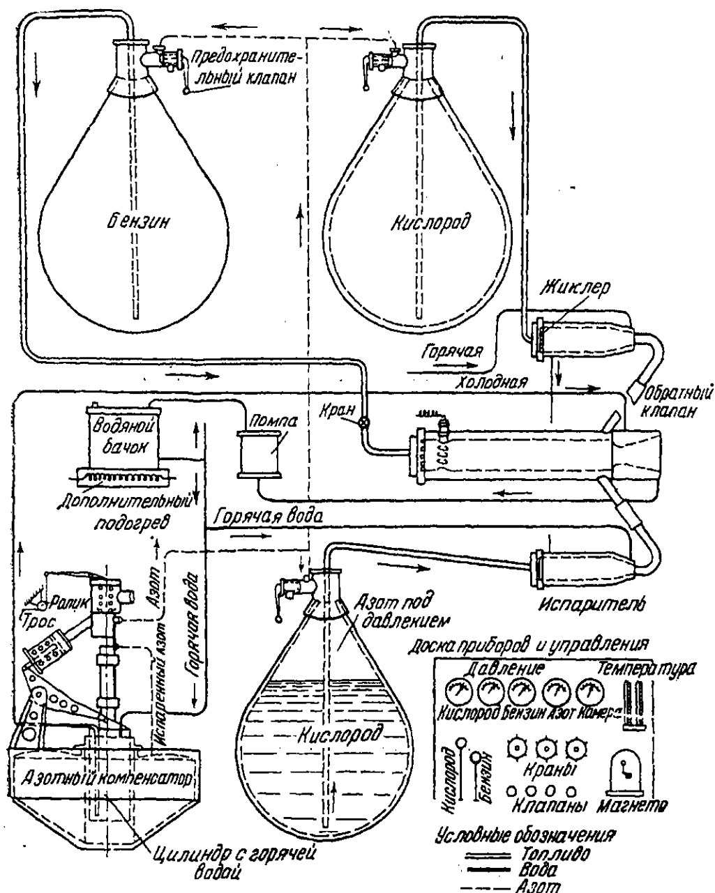
Схема монтажа двигателя ОР-2.
