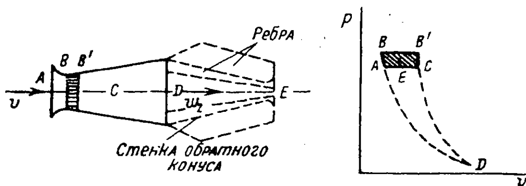
Фиг. 25. Схема обыкновенного воздушного реактивного двигателя.
