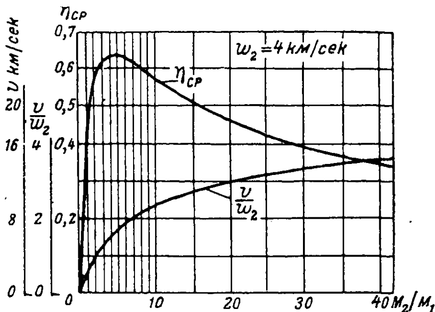
Фиг. 19. Средний к. п. д. и скорость полета ракеты в среде без тяжести.
