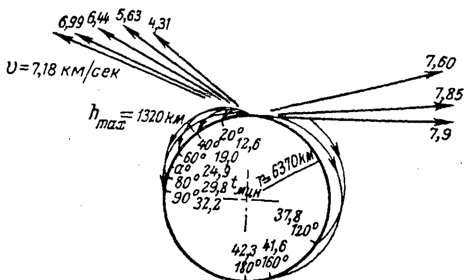
Фиг. 32. Радиусы действия далеко летающих ракет вне атмосферы.
