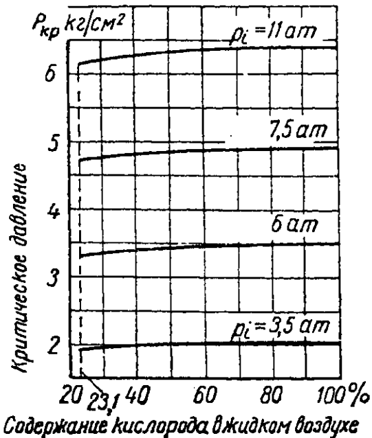
Фиг. 7. Изменение критического давления в зависимости от давления в камере сгорания и от содержания кислорода в воздухе.
