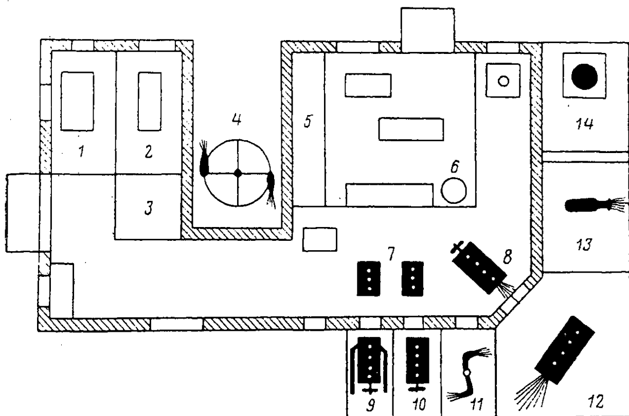
Схема испытательной станции и лаборатории по проекту Ф. А. Цандера.
