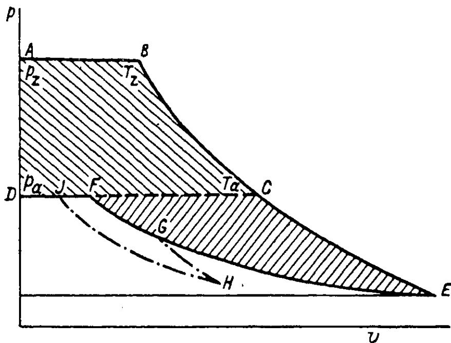
Фиг. 16. Диаграмма p-v реактивного двигателя, улучшенного рабочим циклом.
