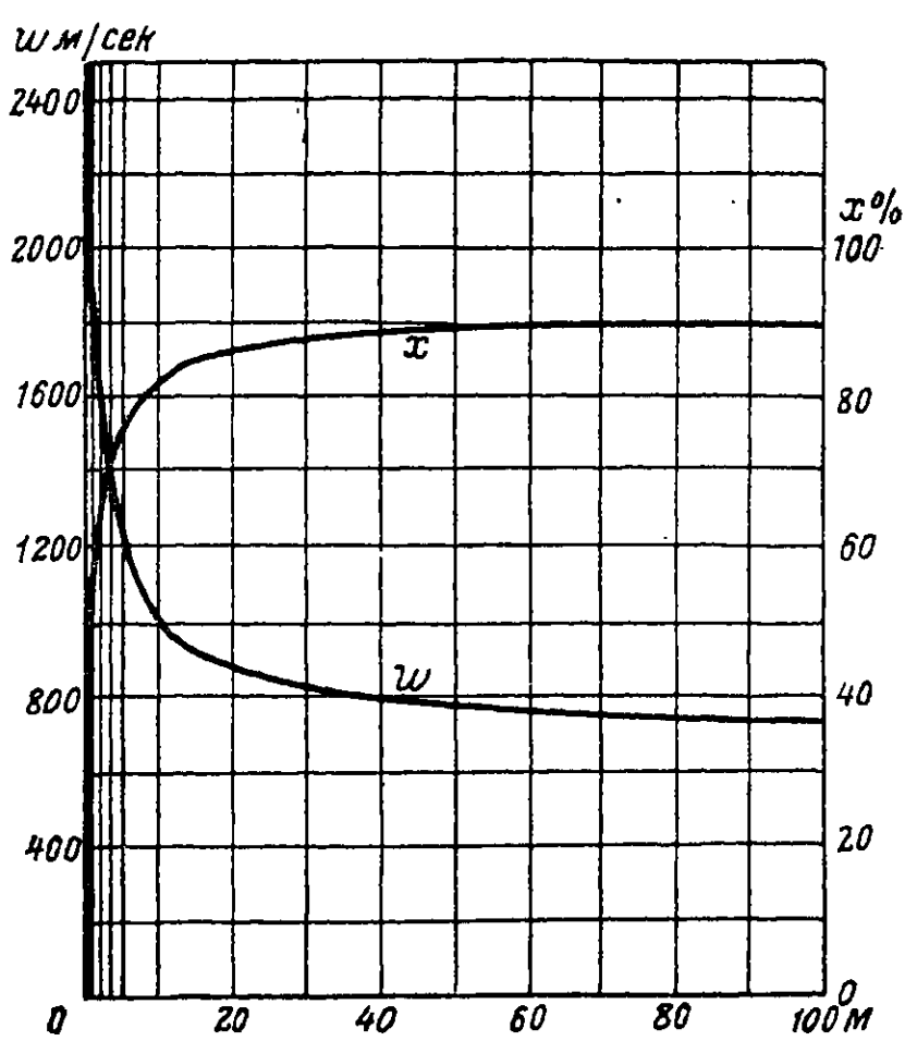
Фиг. 23. Диаграмма к воздушному реактивному двигателю w — общая скорость; x — количество отведенного воздуху тепла в процентах.
