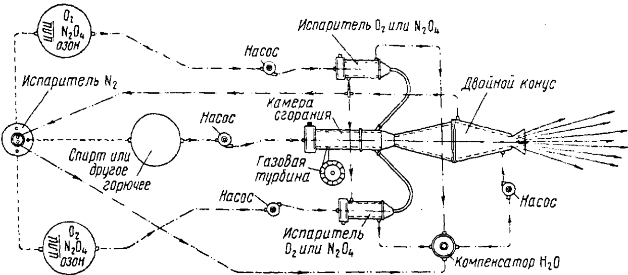
Схема третьего варианта реактивного двигателя на 5 т.
