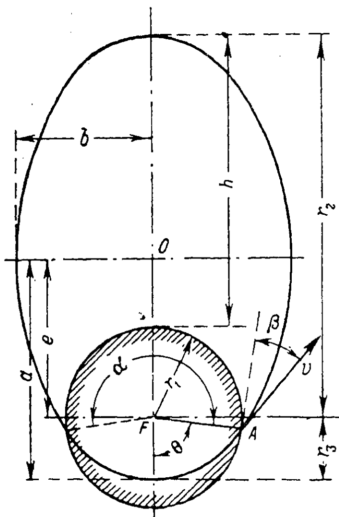
Фиг. 37. К расчету пути полета далеко летающих ракет.
