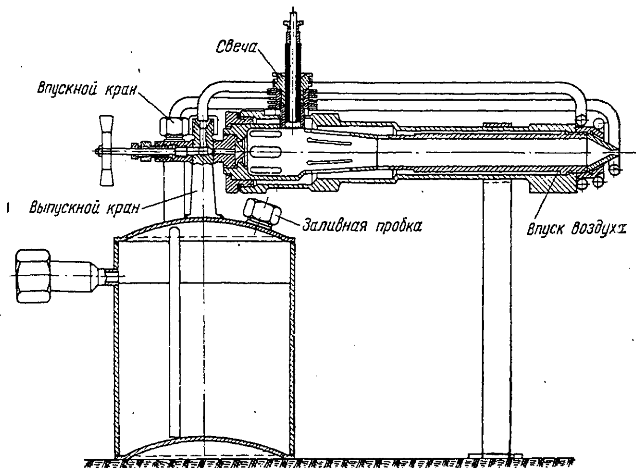
Схема двигателя ОР-1.
