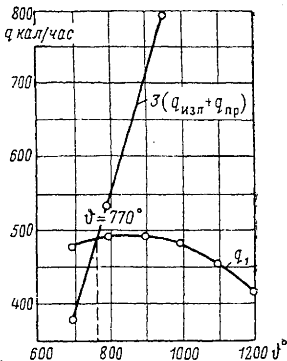
Фиг. 2. Расход тепла при наличии ребер, увеличивающих поверхность теплообмена в три раза.
