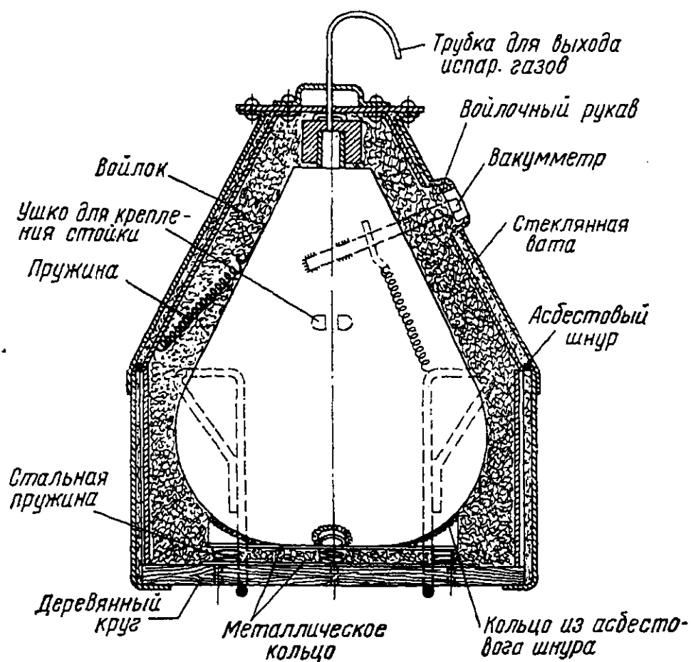
Бак для жидкого кислорода.
