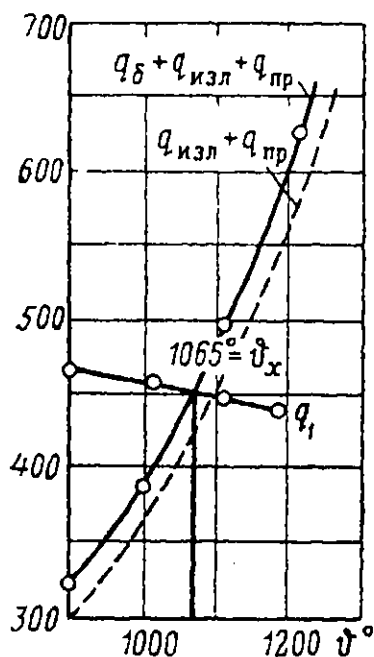
Фиг. 1. Расход тепла через стенки (без ребер).
