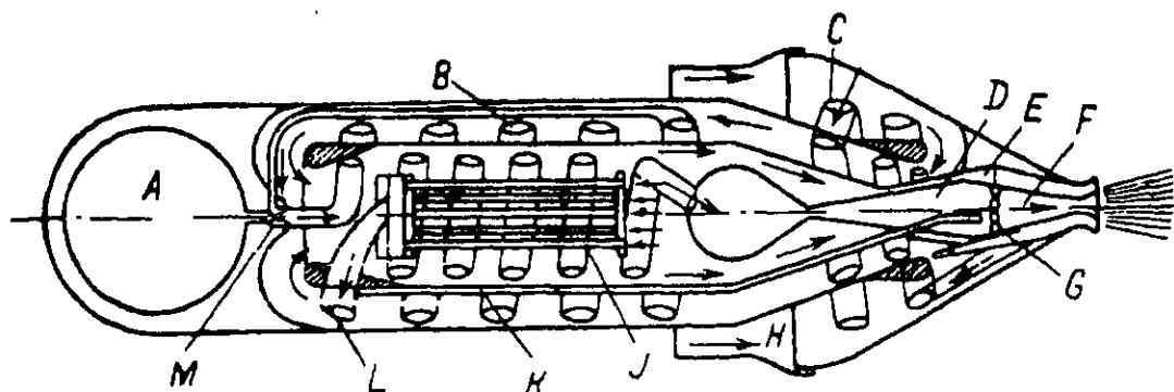
Фиг. 21. Схема воздушного реактивного двигателя с отдельными циклами.
