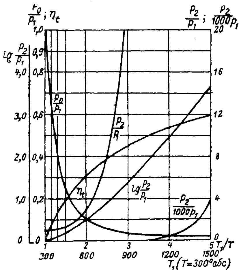
Фиг. 20. Теоретические кривые сжатия воздуха струйных нагнетателей.
