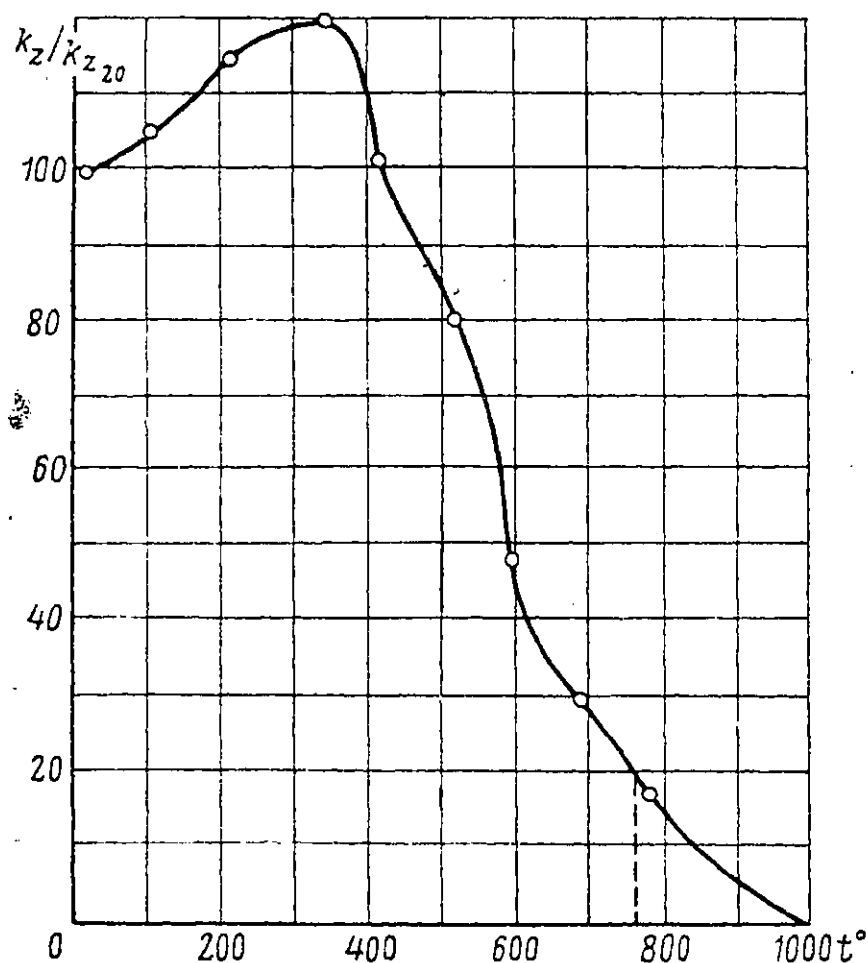
Фиг. 3. Крепость сварочного железа при различных температурах по отношению к крепости при 20^{\circ}\text{C} .
