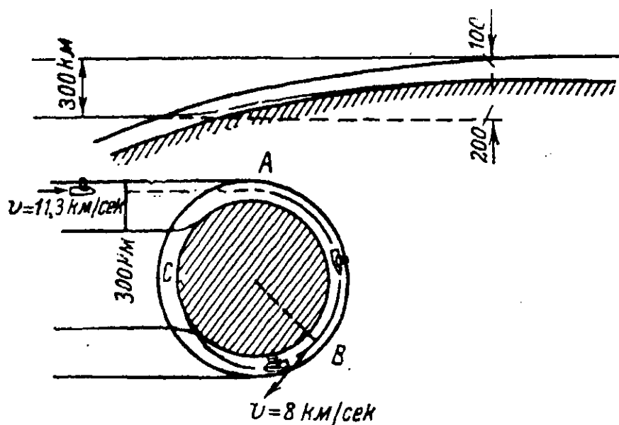
Фиг. 31. Планирующий спуск из межпланетного пространства на землю.
