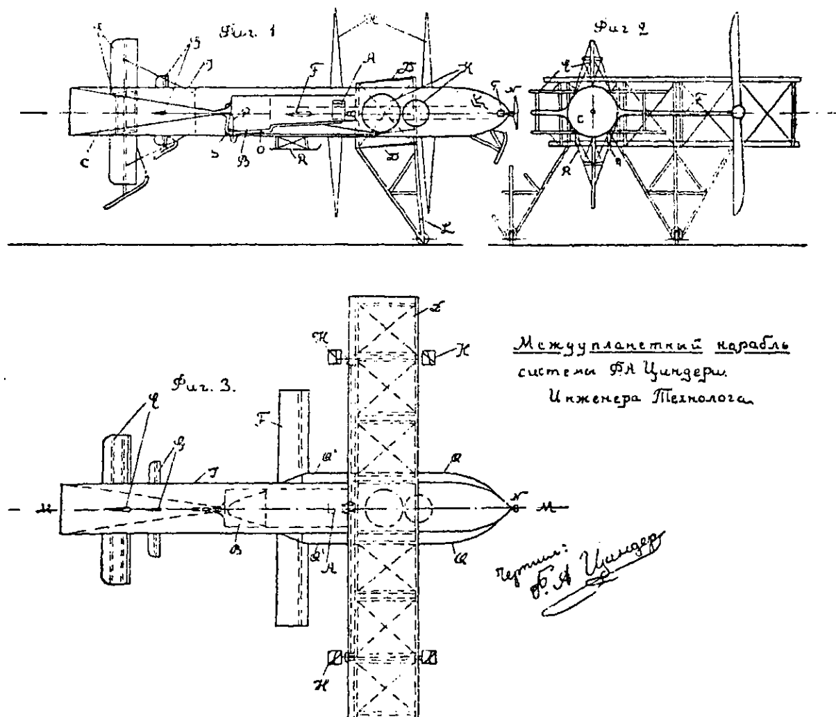
Фиг. 1. Межпланетный корабль системы Ф. А. Цандера (проект).
