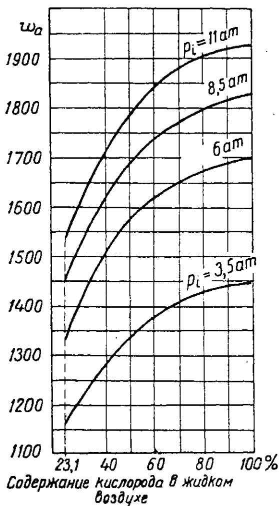
Фиг. 10. Скорость истечения продуктов сгорания из сопла ракетного двигателя в зависимости от давления в камере и содержания кислорода в воздухе.
