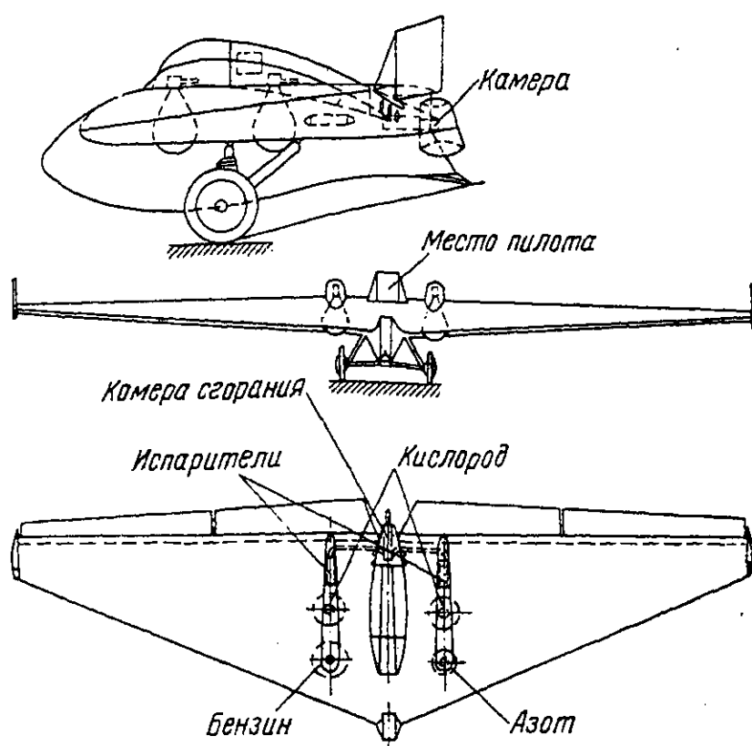
Схема планера РП-1 «Летающее крыло», сконструированного для ракетного двигателя ОР-2.
