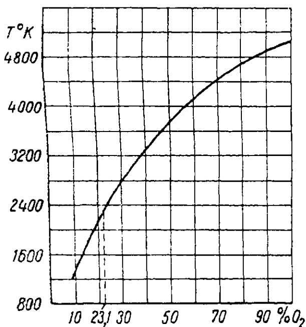
Фиг. 1. Изменение температуры сгорания (без учета диссоциации) бензина в зависимости от содержания кислорода в воздухе.
