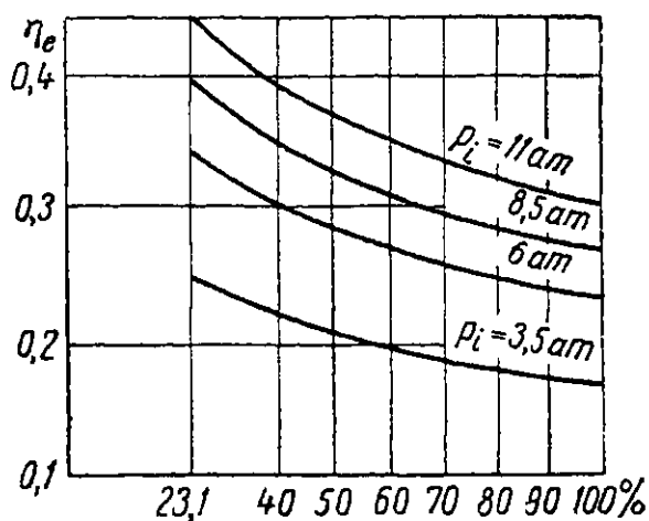
Фиг. 11. Эффективный к. п. д. ракетного двигателя при различном содержании кислорода в воздухе и при различном давлении в камере сгорания.
