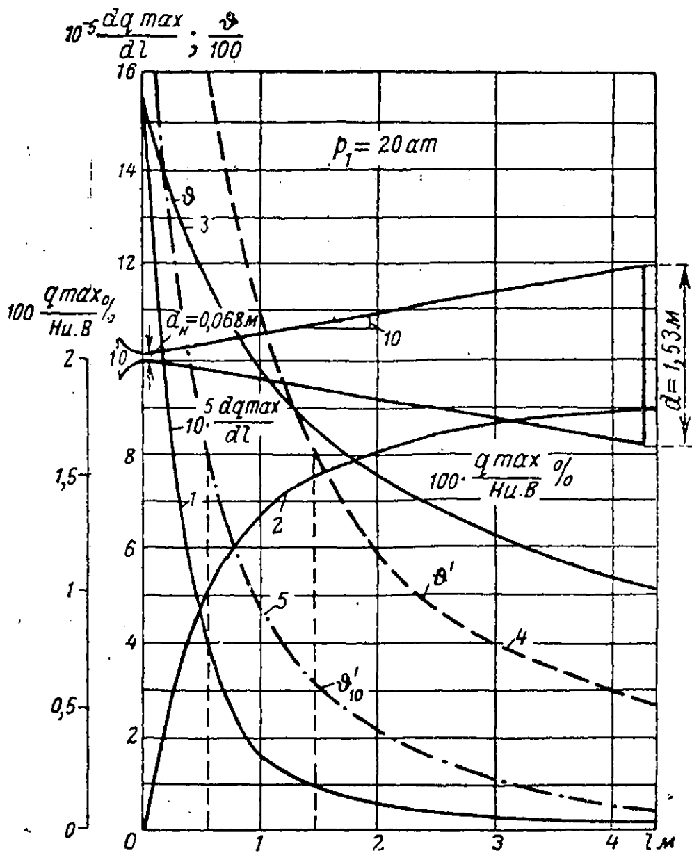
Фиг. 13. Определение прохождения тепла через стенки ракеты.
