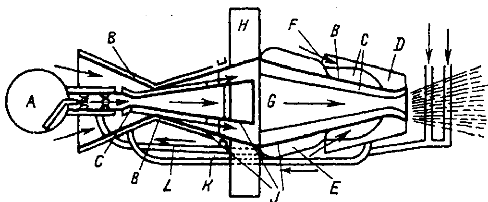
Фиг. 22. Схема воздушного реактивного двигателя, у которого продукты сгорания смешиваются с воздухом без удара.
