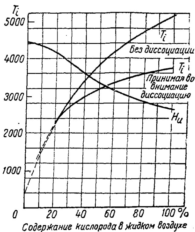
Фиг. 4. Выделение тепла при сгорании бензина. Температура сгорания бензина в зависимости от содержания кислорода в воздухе как с учетом диссоциации, так и без учета ее.
