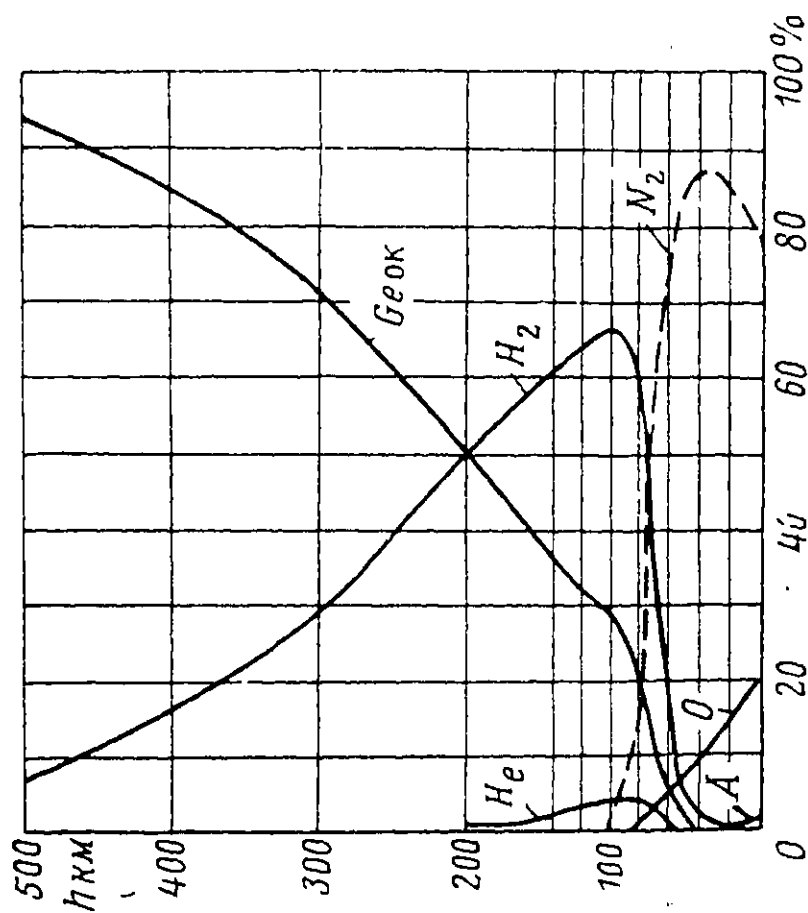
Фиг. 6. Состав атмосферы по Вегенеру.
