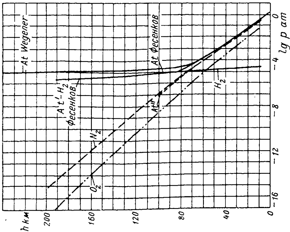
Фиг. 4. Логарифмы давления атмосферы и ее составных частей.
