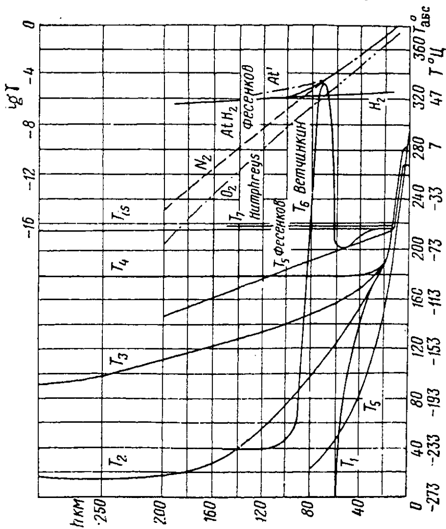
Фиг. 3. Температура атмосферы до высот 300 км и логарифмы плотности атмосферы ( \gamma кг/м 3 ) до 200 км по Фесенкову.
