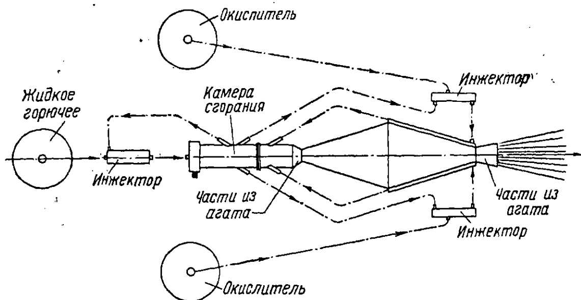
Схема первого варианта реактивного двигателя на 5 т.
