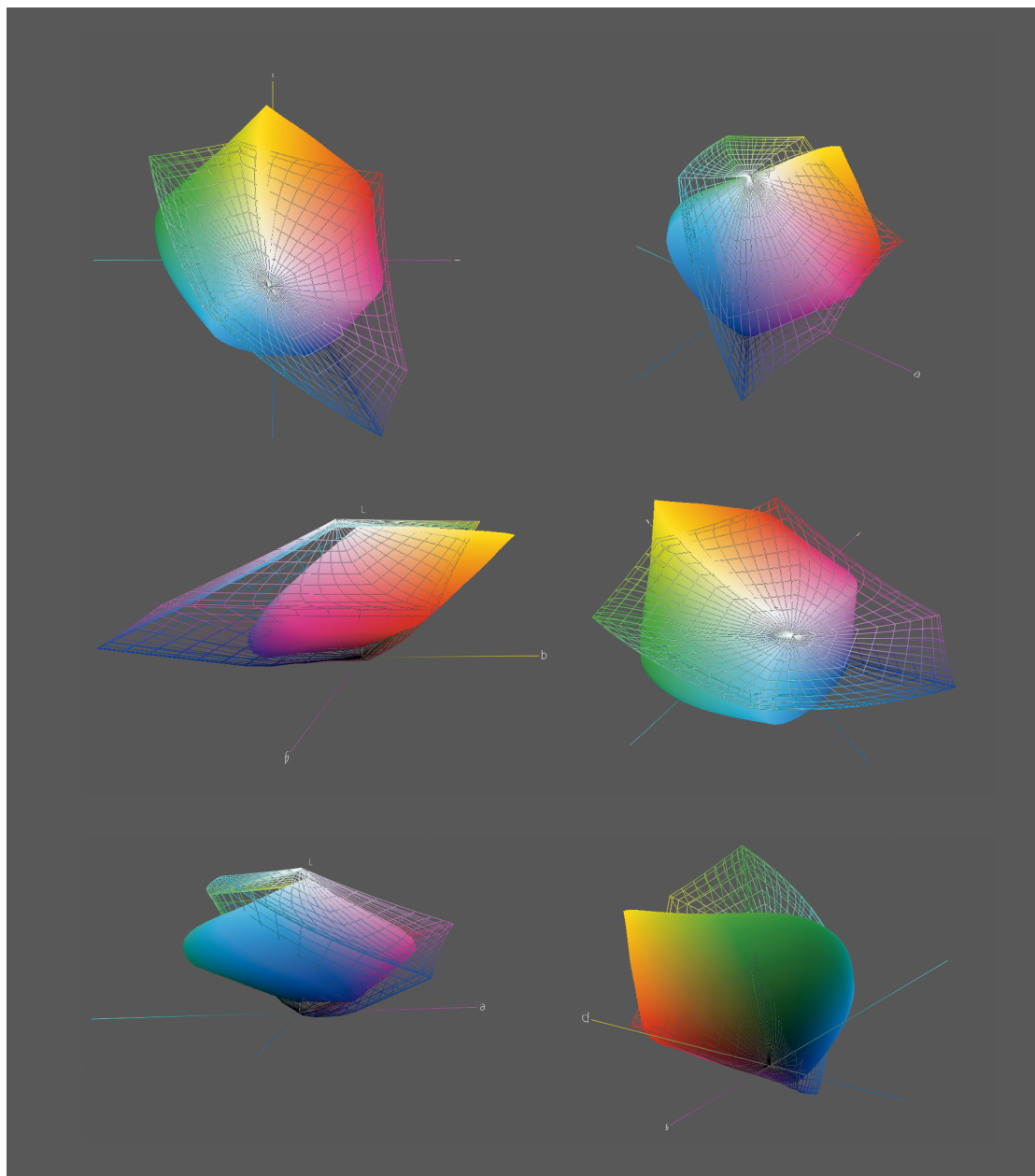
Рис. 19.2 Несколько проекций трехмерного представления цветных охватов двух устройств в цветовом пространстве CIE LAB. Сплошная фигура — охват типичного термотрансферного принтера. Сетчатая фигура — охват типичного CRT-дисплея.
