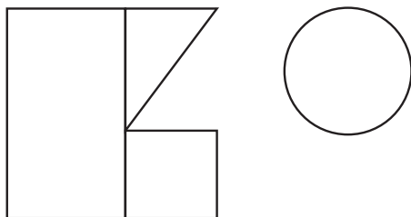
Рис. 1.3. Вопросы землемерия
