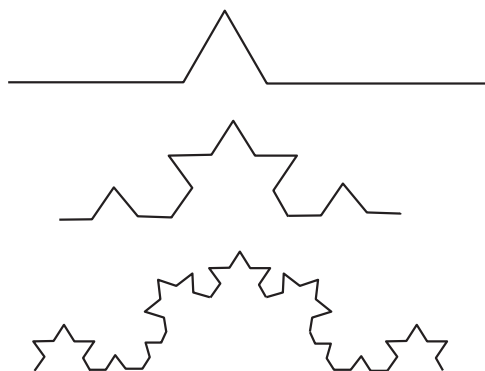
Рис. 11.14. Масштабирование фрактала
