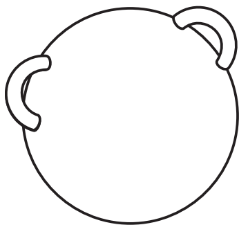
Рис. 10.7. Классификация двумерных многообразий
