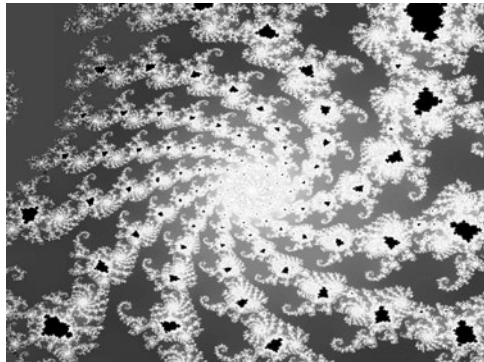
Рис. 11.12. Второй фрактал
