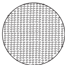
Рис. 5.6. Замкнутый диск
