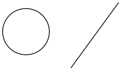
Рис. 10.6. Классификация одномерных многообразий
