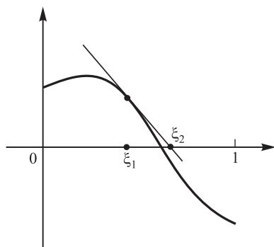
Рис. 5.24. Новое приближение лучше прежнего
