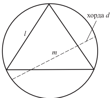
Рис. 5.26. Парадокс Бертрana
