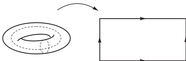
Рис. 6.5. Разрезание тора
