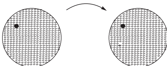
Рис. 5.7. Неподвижная частица сыра
