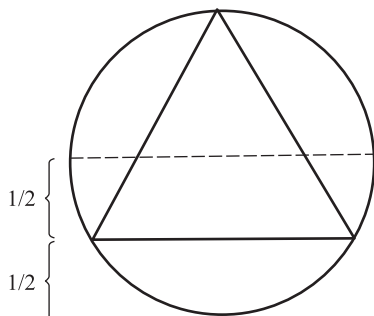
Рис. 5.29. Второе решение парадокса Бертрana
