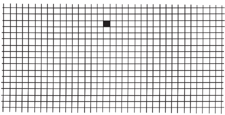
Рис. 11.3. Исходная конфигурация клеточного автомата
