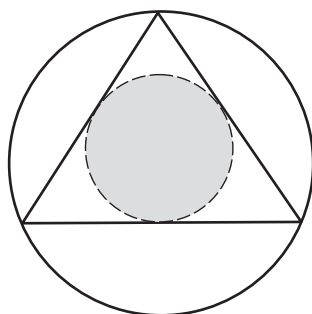
Рис. 5.27. Первое решение парадокса Бертрana
