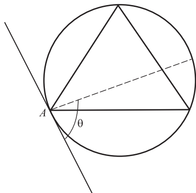
Рис. 5.31. Третье решение парадокса Бертрана. Продолжение
