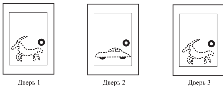
Рис. 5.34. Задача Монти Холла
