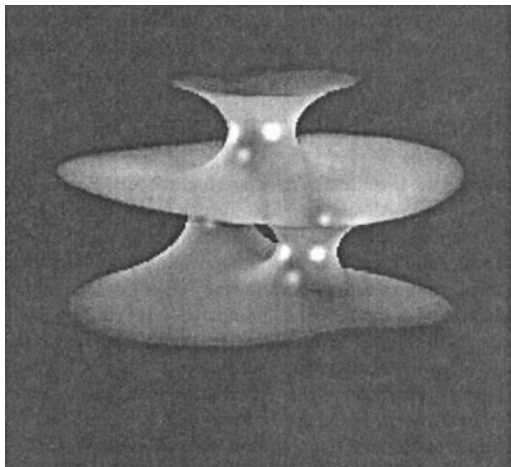
Рис. 8.4. Минимальная поверхность
