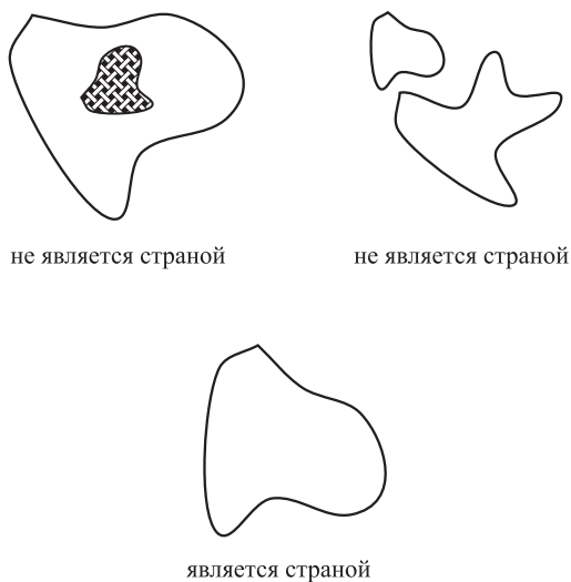
Рис. 6.1. Страна из задачи о четырех красках
