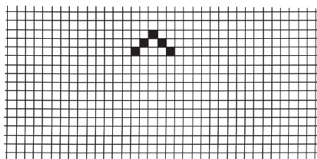
Рис. 11.6. Вторая итерация правила 90
