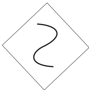
Рис. 5.25. Знак «опасный поворот» Бурбаки
