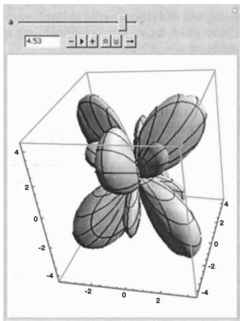
Рис. 8.1. График, созданный в пакете Mathematica
