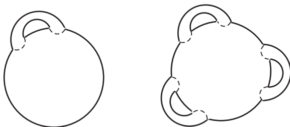
Рис. 6.3. Поверхность на сфере с ручками
