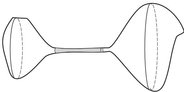
Рис. 10.10. «Сигара» в потоке Риччи
