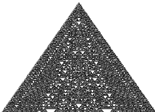
Рис. 11.9. Второй клеточный автомат
