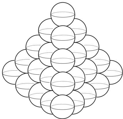
Рис. 10.5. Трехмерный аналог плоской шестиугольной упаковки кругов
