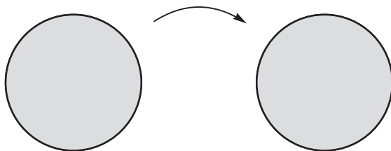
Рис. 5.2. Непрерывное отображение диска на себя
