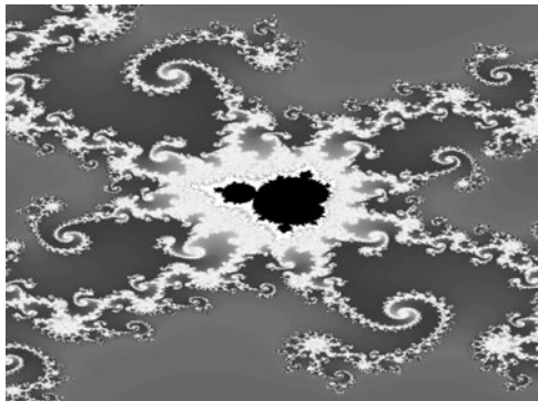
Рис. 11.11. Первый фрактал
