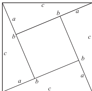
Рис. 2.7. Доказательство теоремы Пифагора
