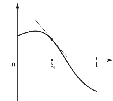
Рис. 5.23. Второй шаг в методе Ньютона
