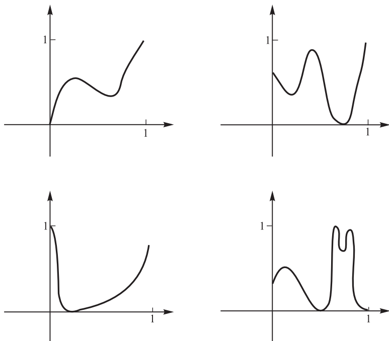
Рис. 5.9. Сложность непрерывной функции
