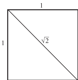
Рис. 8.2. Приближение числа \sqrt{2}
