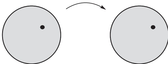
Рис. 5.3. Неподвижная точка
