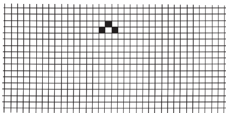
Рис. 11.5. Первая итерация правила 90
