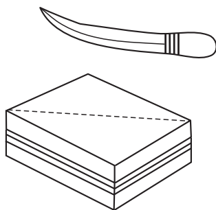
Рис. 5.17. Другой разрез классического бутерброда
