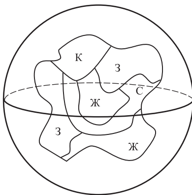
Рис. 6.2. Никакие две соседние страны не раскрашены в один цвет
