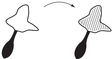
Рис. 8.3. Мыльная пленка
