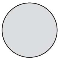
Рис. 5.1. Замкнутый диск
