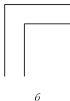
Рис. 2.3. Окружность и прямой угол
