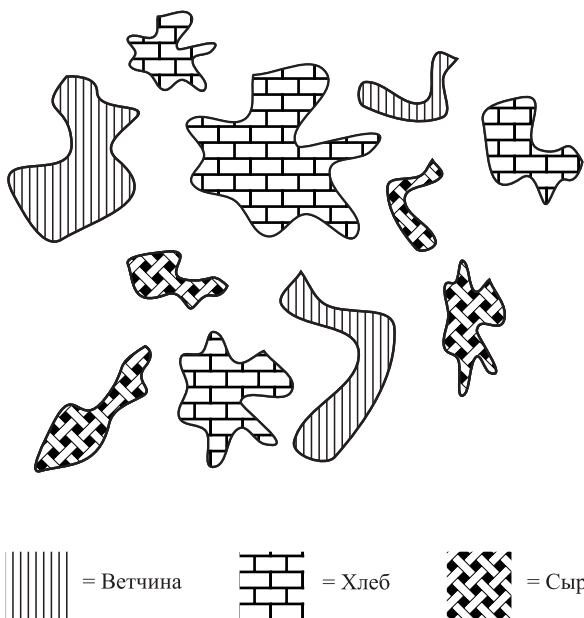
Рис. 5.18. Обобщенный бутерброд с ветчиной
