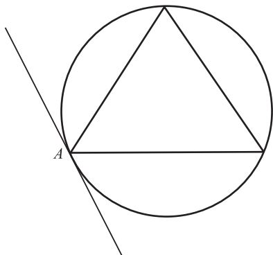
Рис. 5.30. Третье решение парадокса Бертрана
