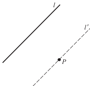
Рис. 2.4. Постулат о параллельных
