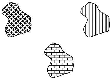
Рис. 5.20. Ограничения на обобщенную теорему о бутерброде в двумерном пространстве
