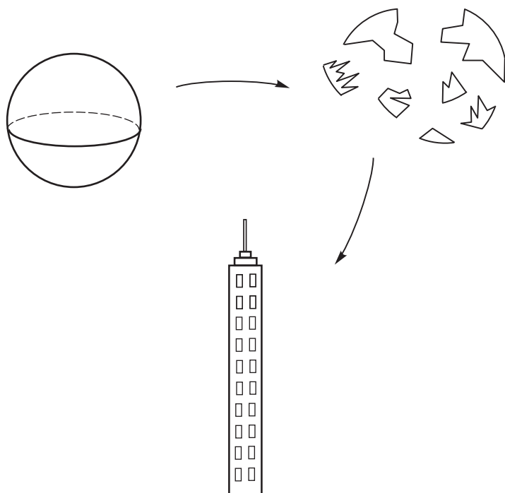
Рис. 5.33. Парадокс Банаха—Тарского. Продолжение
