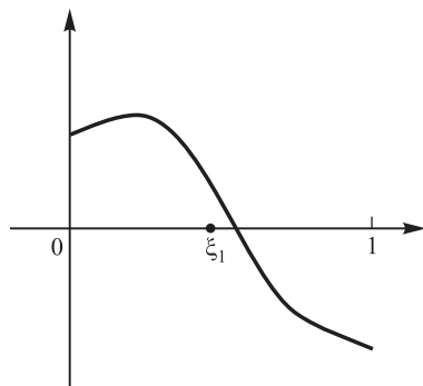
Рис. 5.22. Первый шаг в методе Ньютона
