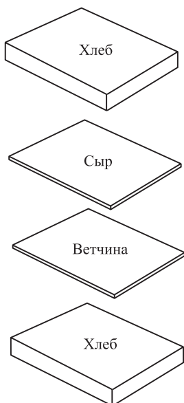
Рис. 5.15. Классический бутерброд с ветчиной
