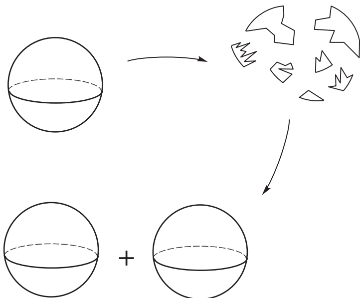
Рис. 5.32. Парадокс Банаха—Тарского
