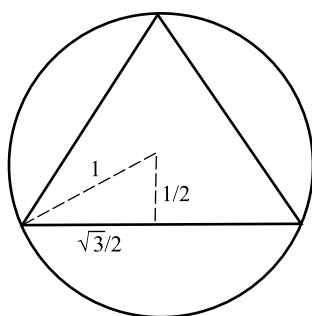
Рис. 5.28. Первое решение парадокса Бертрana. Продолжение
