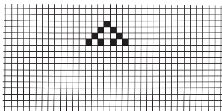
Рис. 11.7. Третья итерация правила 90
