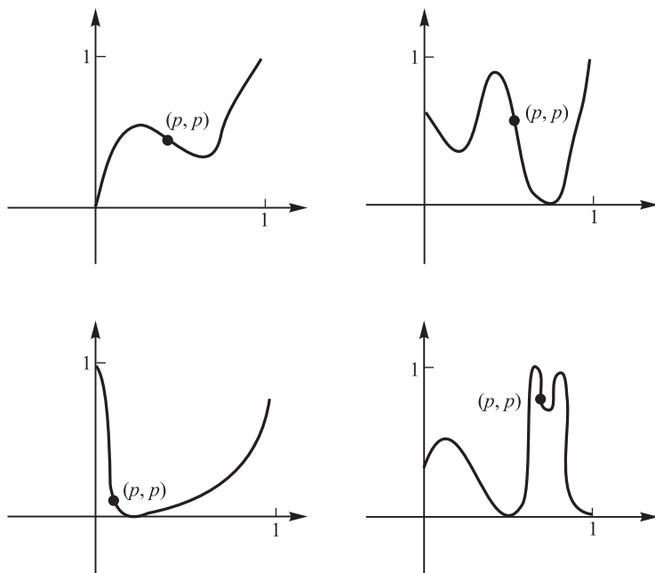
Рис. 5.10. Неподвижная точка каждой непрерывной функции
