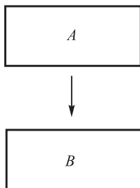
Рис. 1.4. Логический вывод
