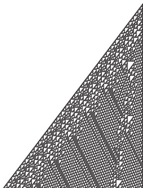
Рис. 11.8. Первый клеточный автомат
