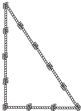
Рис. 2.8. Пифагорова веревка египтян
