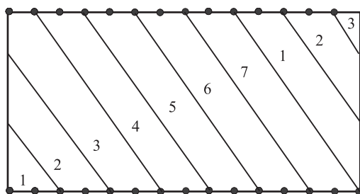
Рис. 6.6. Карта на торе, для раскраски которой требуется семь цветов
