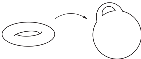
Рис. 6.4. Тор — это сфера с одной ручкой
