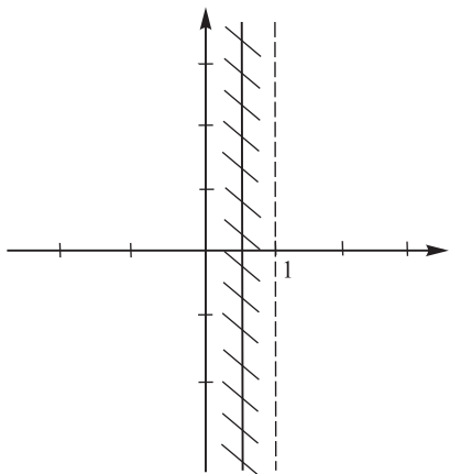
Рис. 11.2. Критическая полоса
