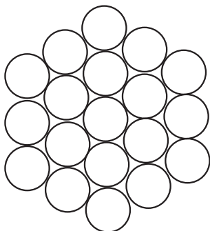
Рис. 10.4. Лучшая упаковка кругов
