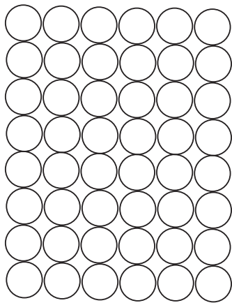
Рис. 10.3. Не лучшая упаковка кругов
