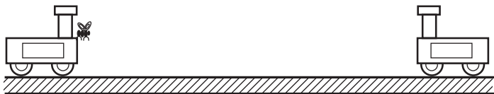
Рис. 7.5. Путешествие мухи от поезда к поезду
