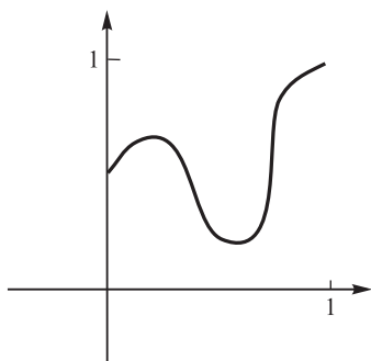
Рис. 5.8. Функция, непрерывная на единичном отрезке
