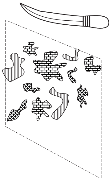
Рис. 5.19. Обобщенная теорема о бутерброде
