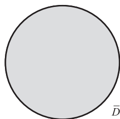
Рис. 5.12. Замкнутый единичный диск
