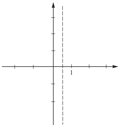
Рис. 11.1. Критическая прямая
