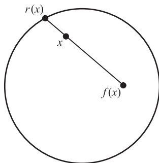
Рис. 5.14. Построение ретракции
