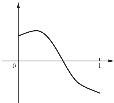
Рис. 5.21. Гладкая функция — подходящий кандидат для метода Ньютона
