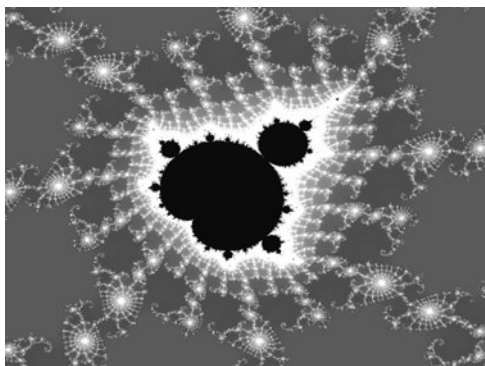
Рис. 11.13. Множество Мандельброта
