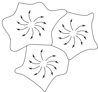
Рис. 10.11. Поток Риччи порождает декомпозицию геометрий
