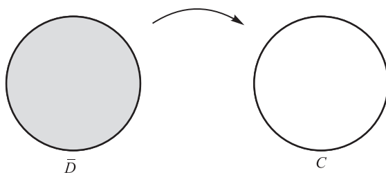
Рис. 5.13. Ретракция
