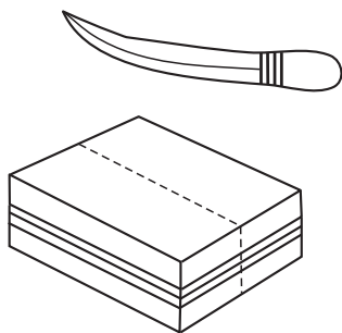
Рис. 5.16. Один разрез классического бутерброда
