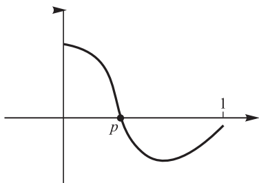
Рис. 5.11. Теорема о промежуточном значении
