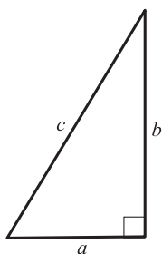
Рис. 2.6. Теорема Пифагора
