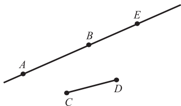
Рис. 2.2. Второй постулат Евклида
