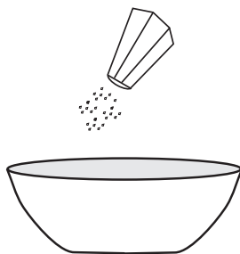
Рис. 5.5. Тертый сыр на поверхности супа
