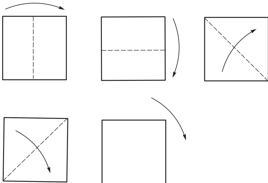
Рис. 10.2. Симметрии квадрата
