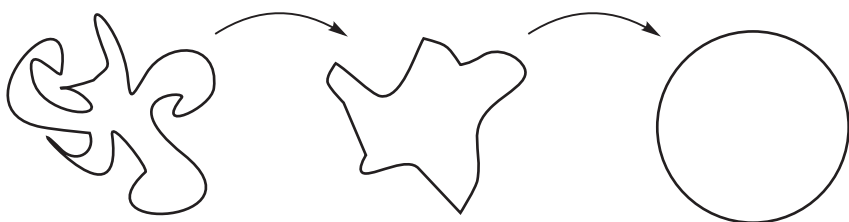
Рис. 10.9. Сингулярности потока Риччи
