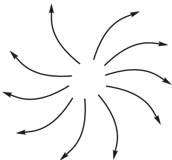
Рис. 10.8. Поток Риччи
