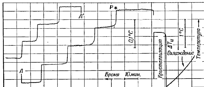
Рис. 7. Результаты криометрических измерений Al[CH_2CH(C_2H_5)C_4H_9]_3 в триизобутилалюминии как растворителя. Тепловой пик загрязнений в точке P отсутствует. Установление фазового равновесия замедленное — закругленные углы, которые видны также при добавке индифферентных эталонных веществ, например изеооктана.
