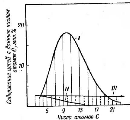
Рис. 1. Рассчитанное распределение по длине цепи продуктов реакции достройки \text{Al}(\text{C}_2\text{H}_5)_3 этиленом.
