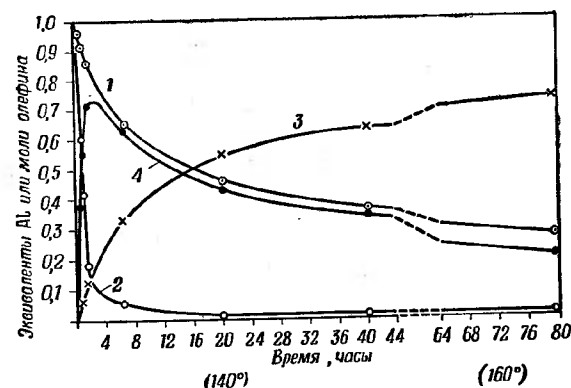
Рис. 3. Изменение состава смеси 1 экв трипропилалюминия и 1 моля пропилена во времени при 140^\circ . 1 — \text{C}_3 связан с Al; 2 — \text{C}_3 свободный; 3 — \text{C}_3 связан с Al; 4 — \text{C}_3 свободный.
