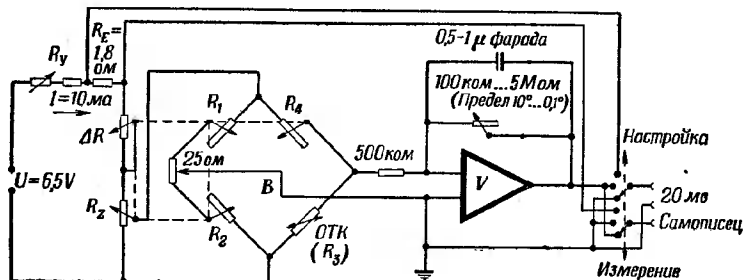
Рис. 2. Схема электрического измерения температуры.
