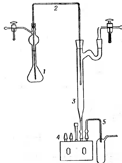
Рис. 4. Приспособление для заполнения проточных ячеек без доступа воздуха (пояснения в тексте).
