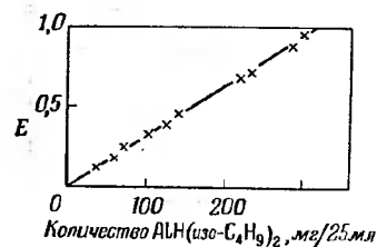
Рис. 2. Применимость закона Ламберта—Беера. Абсцисса: количества АН (изо-С 4 Н 9 ) 2 /25 мл реагента; реагент: бензальанилин; d = 0,05 см, \lambda = 500 мμ. Точки на кривой соответствуют точным значениям отдельных измерений, приведенных в табл. 1.
