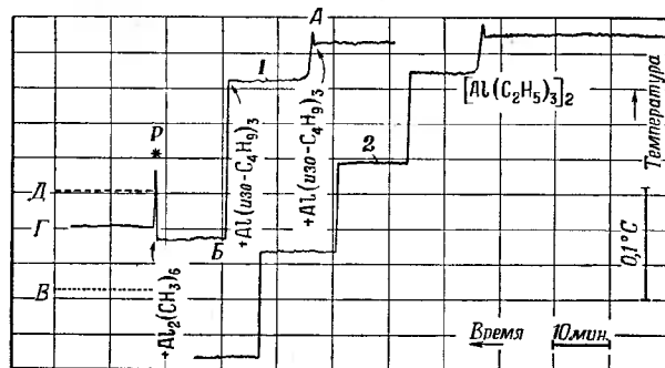
Рис. 6. Результаты криометрических измерений смесей триизобутилалюминия с триметилалюминием в бензоле.
