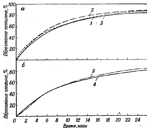
Рис. 3. Отщепление олефина от различных алюминийтриалкилов в присутствии других олефинов (объем во всех случаях \sim 500 мл).
