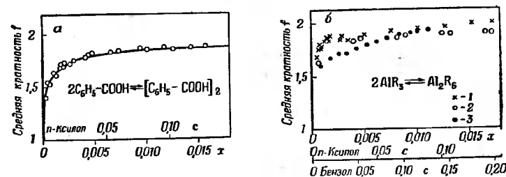
Рис. 5. Зависимость степени ассоциации, найденной криометрическим способом, от концентрации для бензойной кислоты в п -ксилоле (а), а также для триэтил-, три- н -бутилалюминия (б). Константа ассоциации K_x = 6,5 \cdot 10^3 .
