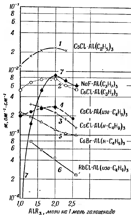
Рис. 2. Изменение электропроводности комплексов хлористого цезия с некоторыми алюминийтриалкилами при молярном отношении \text{AlR}_3/\text{CsCl} > 1 при 100^\circ .
