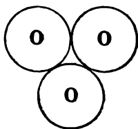
Молекула озона
