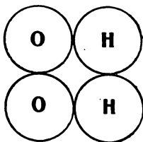
Молекула перекиси водорода
