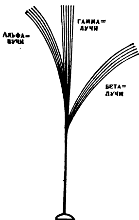
Разделение радиоактивных лучей в магнитном поле
