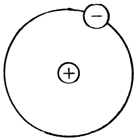
Модель атома водорода
