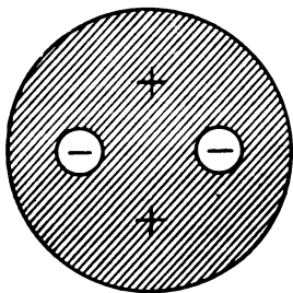
Модель атома по Томсону
