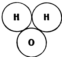
Молекула воды
