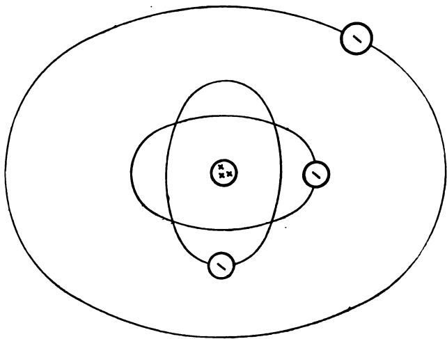
Модель атома лития
