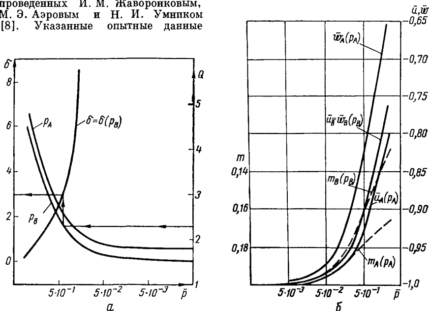
Рис. 13. Рассчитанные замороженная и равновесная ударные адиабаты и ширина фронта ударной волны (а), а также скорости частиц и пористость (б) для грунта начальной пористости: m_0 = 0,2 при \kappa_1 = 3,00, \kappa_2 = 3,00 .
