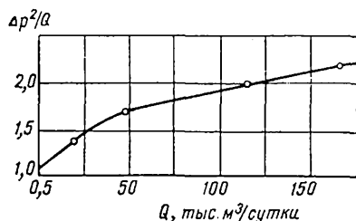
Рис. 41. Зависимость \Delta p^2/Q от Q для скв. 2 Саушинского месторождения.
