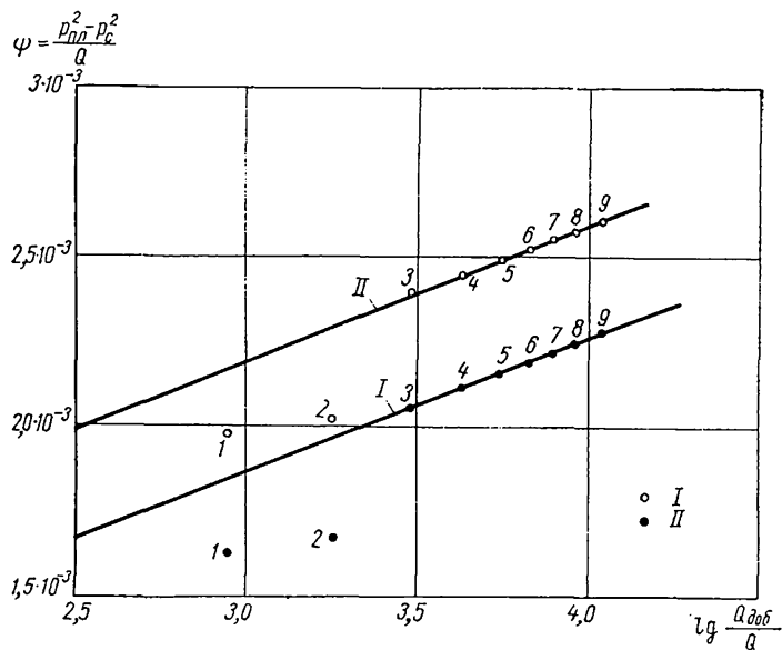
Рис. 47. Зависимость \Delta p^2/Q от \lg \frac{Q_{дсб}}{Q} для скв. 117-III.
