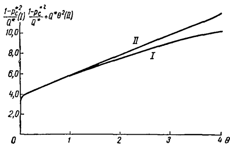
Рис. 51. Зависимость 1 - p_{\xi}^2/Q^* от \theta .
