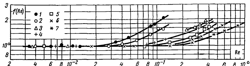
Рис. 2. Представление экспериментальных данных Фенчера, Льюиса и Бернса в виде f = f(Re) :
