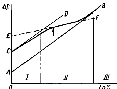
Рис. 57. Характерный вид кривой восстановления давления при учете нелокально-упругих эффектов.
