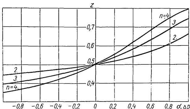
Рис. 37. Зависимость z (\propto \Delta p) при различных значениях n .
