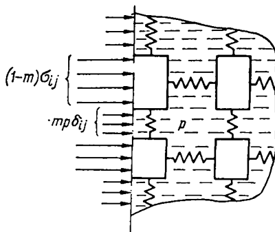
Рис. 1. Схематическое представление контактной передачи импульса в насыщенной пористой среде.
