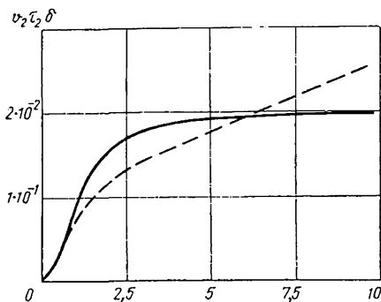
Рис. 11. Зависимость коэффициента затухания от частоты монохроматической звуковой волны в щелевидном канале, v_2 \tau_2 \delta = f(h_2) .
