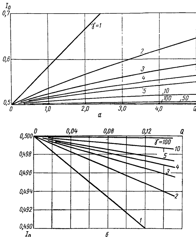
Рис. 31. Зависимость интеграла I от значений параметров \alpha и \gamma для осесимметричной фильтрации:
