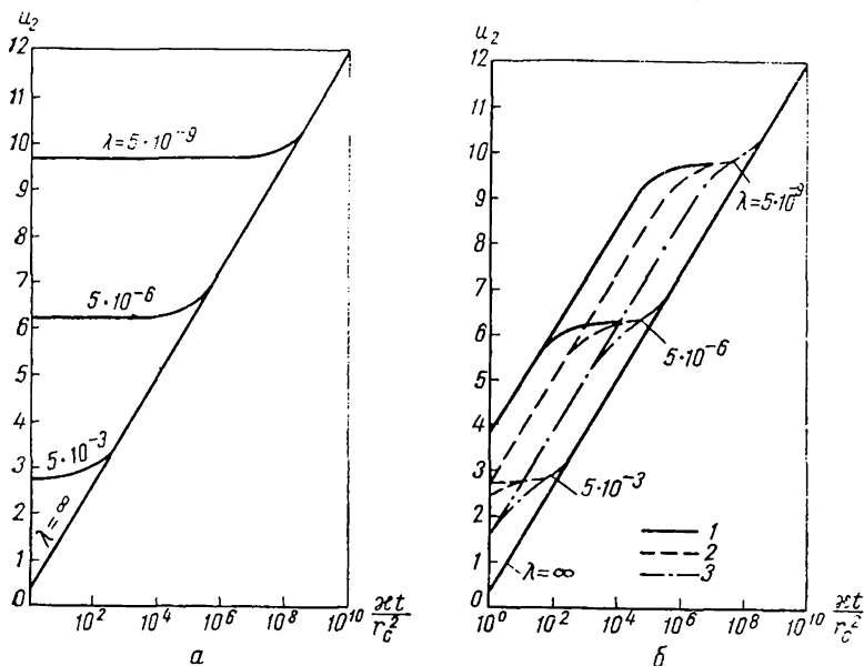
Рис. 32. Зависимость безразмерного давления \bar{u}_2(r_c, t) от параметров \lambda = r_c^2 / \kappa \tau , \omega = \varepsilon_2 (1 + \varepsilon_2)^{-1} :
