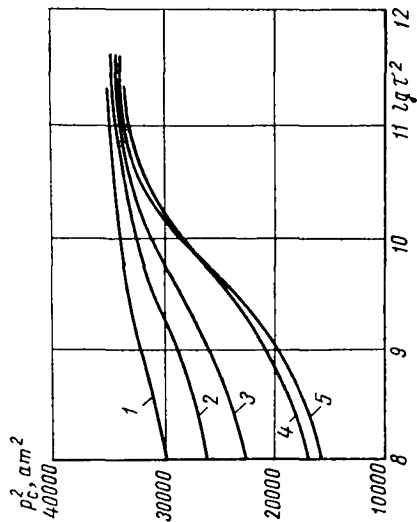
Рис. 49. Результаты обработки серии кривых восстановления давления по скв. 31 в координатах p_c^2 - \lg \tau^2 .
