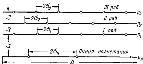
Рис. 44. Схема трех рядов эксплуатационных скважин.
