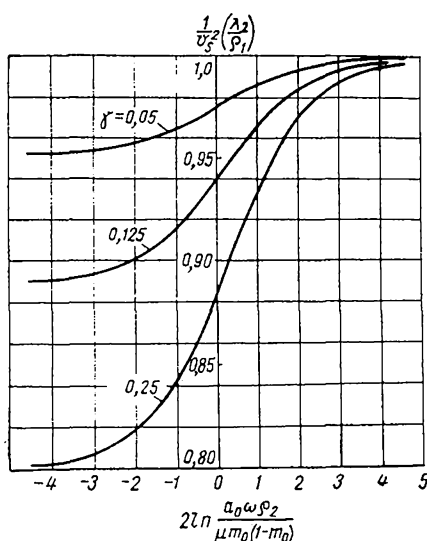
Рис. 4. Зависимость скорости поперечной монохроматической волны v_s от частоты колебаний и параметров среды.
